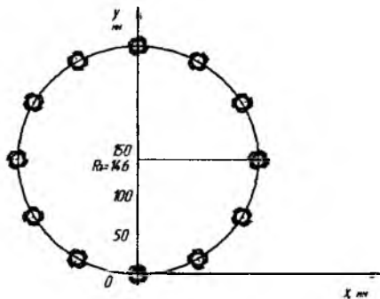
4.3-rasm. Barabanni koordinata o'qlarida joylashtirish sxemasi.
