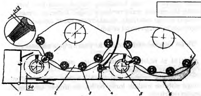
5.18-rasm. Ajratkich va apparat eshiklari holatlarini rostlash:
