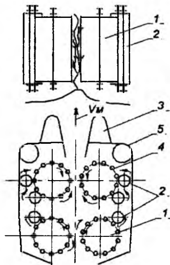
3.3-rasm. Ixtirochi L.M. Rozenblyum tomonidan taklif etilgan VSh paxta terish apparatining prinsipial sxemasi:
