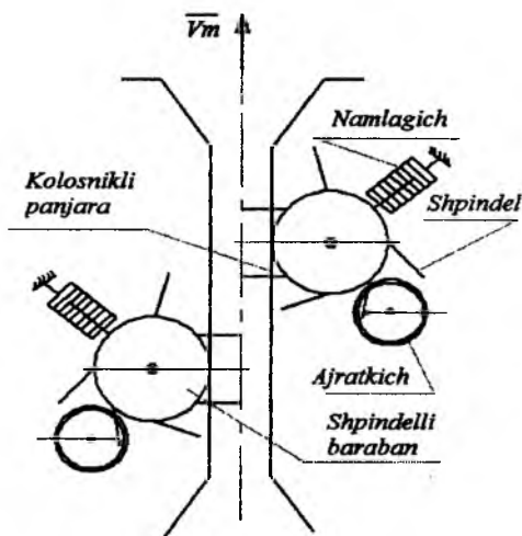
3.8-rasm. G'o'za tuplariga ikki tomondan ishlov beruvchi barabanli GSh PTA prinsipial sxemasi («Case» firmasi mashinalarida qo'llanilgan).
