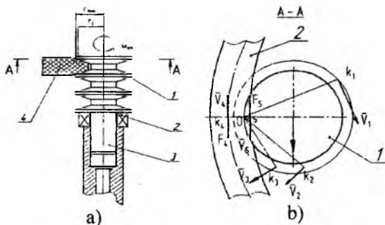
4.1-rasm. VSh PTM shpindel yuritmasi sxemasi:
