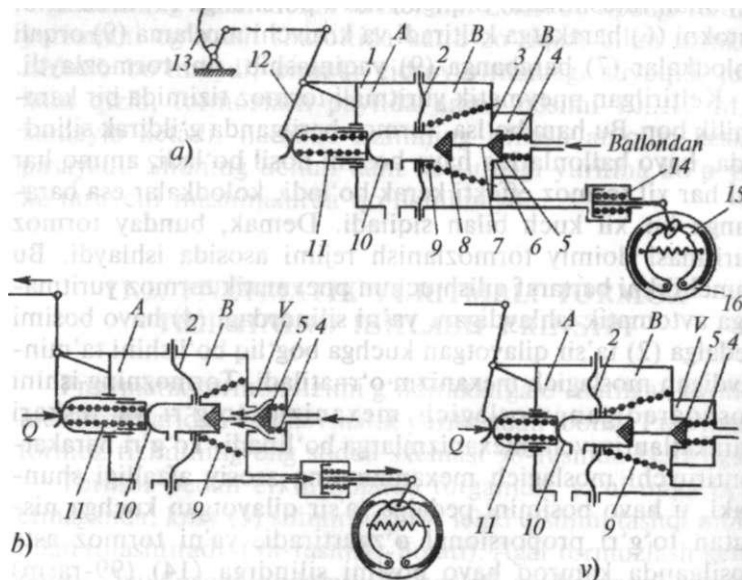
99-rasm. To'g'ri harakatlantiruvchi diafragmalı moslagich mexanizmining sxemasi:
