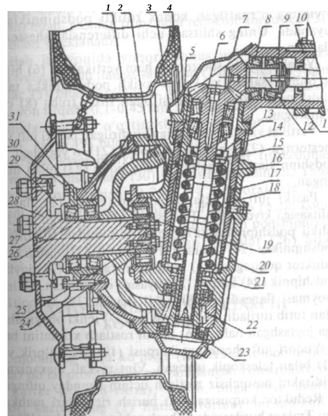
• 67-rasm. MT3-82 traktori oldingi ko'prigi g'ildirak reduktori: Tr, reduktor qopqog'i; 2- pastki juft yetaklanuvchi shesternya; 3, 31- stakanlar 4. 14- stopor halqalar; 5. 30- rostlash vali; 7- qopqog; 24, 27- pod- shipniklar; 9- rostlash gaykasi; 10- ustki konus jufti korpusi; 12- val; 13- zichlama; 15- zichlama oboymasi; 16- zichlama halqa; 17- shkvoren gilzasi; 18- shkvorenli truba; 19- shayba; 20- osma prujina; 21- reduktor korpusi; 22- pastki juft yetakchi shesternyasi; 23- podshipnik qopqog'i; 25- bolt; 26- rostlash halqasi; 28- flanes; 29- zichlash korpusi; 30- bolt; 31- qistirma.
