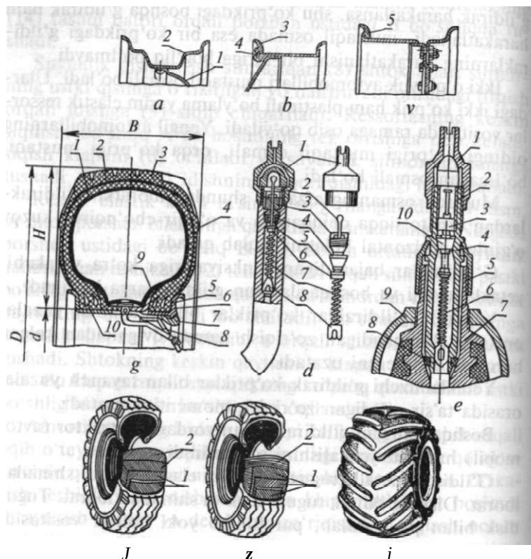
85-rasm. Avtotraktor g'ildiraklari:
