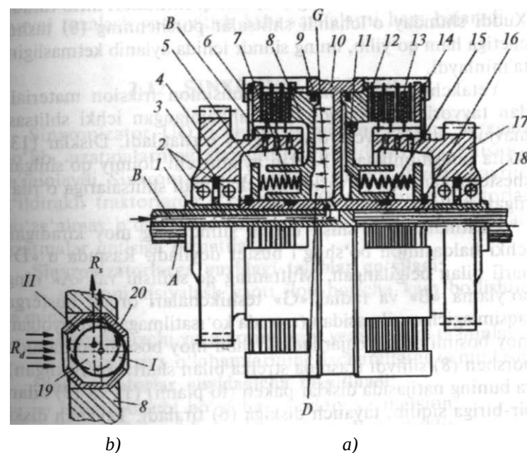
40-rasm. Gidravlik tizimdagi suyuqlik bosimi ta'sirida ishlaydigan ikki barabanli friksion mufta:
