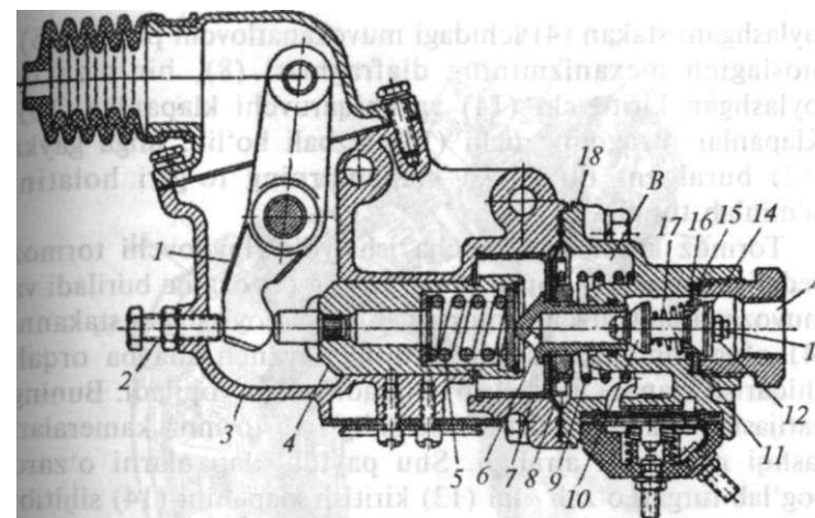
109-rasm. 3MJ1-130 avtomobilining bir mexanizmlı tormoz krani:
