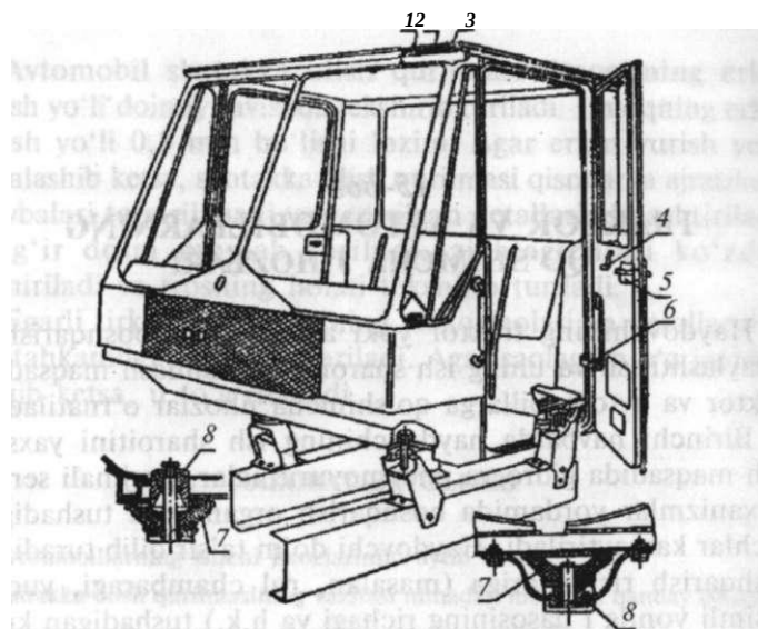
133-rasm. T-150K traktorining kabinasi: 1- mastika qatlami; 2- karton; 3- ekran; 4- oynani ko'tarish dastasi; 5- qulf; 6- oshiq-moshiq; 7- amortizator; 8- bufer.
