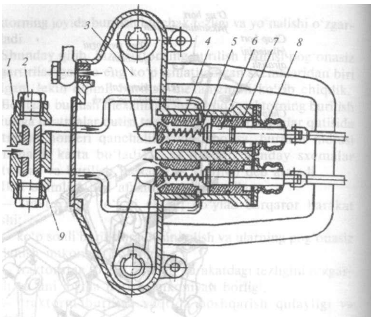
-rasm. Bort friksionini boshqarish gidravlik servouzatmasinin; sxemasi:
