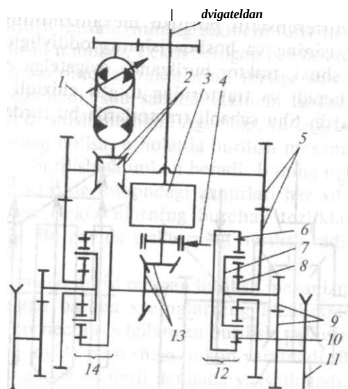
burilish mexanizmi sxemasi- shesternyalari; sheste Z 7 - quyoshsimon shesternya, 9- oxirg, uzatma; 10- satellit; // - yetakchi g'ildirak; 12 va 14- yig'indi planetar qatori; 13- markaziy uzatma.
