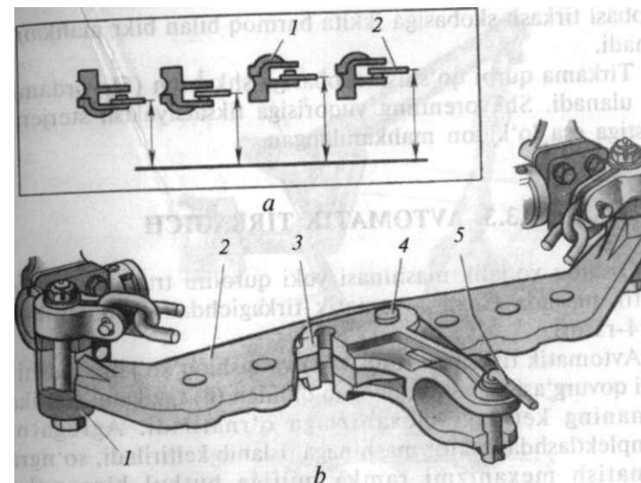
123-rasm. Tirkash qurilmasi:
