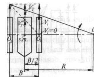
70-rasm. Zanjirli traktorning burilish sxemasi.
