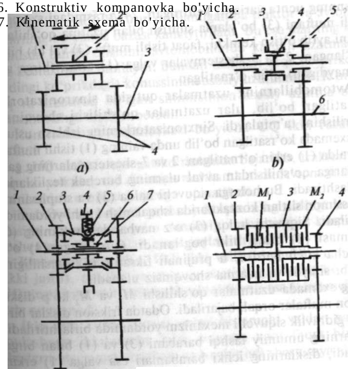
1-rasm. UQ shesternyalari bir-biri bilan tishlashish elementlarining prinsipl sxemalari.
