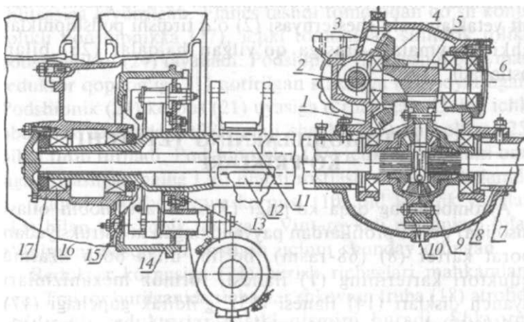
68-rasm. KaMA3 avtomobili orqa ko'prigi:
