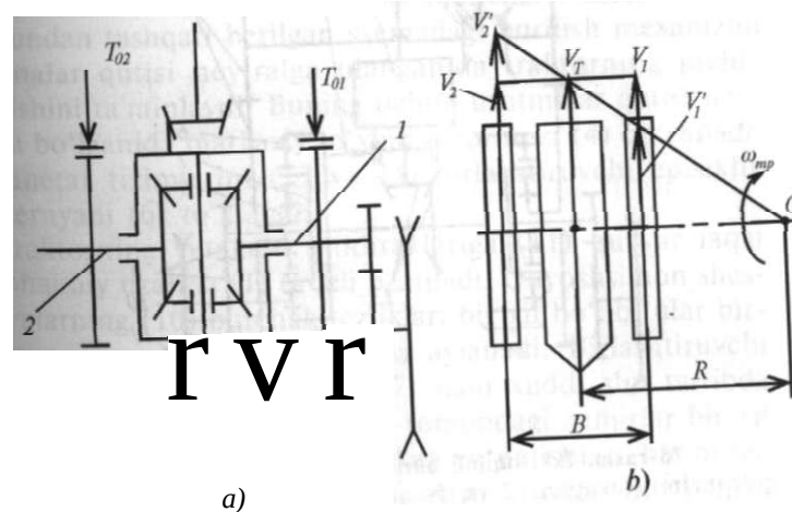
75-rasm. Oddiy differensialli burilish mexanizmi va traktorning burilish sxemasi.
