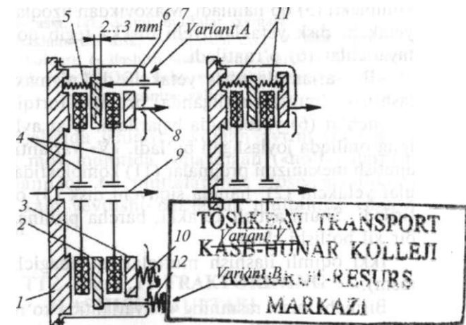
1- dvigatel maxovigi; 2- o'rta yetakchi disk; 3- siquvchi disk; 4- yetaklanuvchi friktsion ustqo'yimli disklar; 5- mufta ajratilganda o'rta yetakchi diskni maxovikdan uzoqlashtiruvchi prujina; 6- o'rta yetakchi diskning maxovikdan uzoqlashishini chegaralovchi rostlash tayanch vinti; 7-ilashish \ muftasining kojuxi; 8- siquvchi diskni boshqarish boltlari; 9- ilashish muftasining yetaklanuvchi vali (transmissiyaning birlamchi) \ ValOJ; 10- siquvchi disk prujinalari; 11- mufta ajratilganida o'rta yetakchi diskni yetaklanuvchi diskarga tegmasdan ushlab turuvchi prujinalar; JA^TET^AJi prujinali rortqi.
