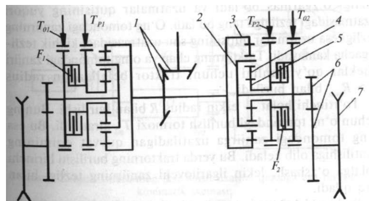
73-rasm. Ikki pog'onali planetar burilish mexanizmi: 1- markaziy uzatma; 2- vodilo; 3- episiklik shesternya; 4- satellit; 5- quyoshimon shesternyasi; 6- oxirgi uzatma; 7- yetakchi g'ildirak.
