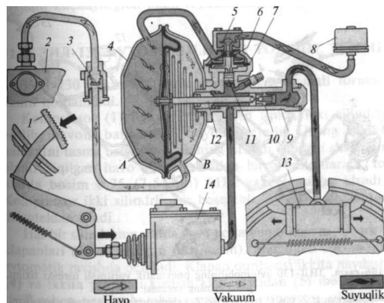
105-rasm. Tormoz yuritmasining gidrovakuum kuchaytirgich sxemasi: A, B — kuchaytirgich vakuum kamerasining bo'shliqlari; 1- tormoz pedali; 2- dvigatelni kiritish (surish) kollektori; 3- berkitish klapani; 4- kuchaytirgichning vakuum kamerasi; 5- havo klapani; 6- vakuum klapani; 7- boshqarish klapanining diafragmasi; 8- havo filtri; 9- kuchaytirgich gidravlik silindri; 10- kuchaytirgich porsheni; 11- boshqarish klapanining porsheni; 12- turtki; 13- g'ildirak tormozi silindri; 14- asosiy tormoz silindri.
