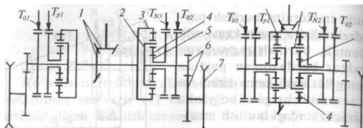
71-rasm. Bir pog'onali planetar burilish mexanizmi: a — planetar qatori ajratilgan; b — bitta korpusga joylashtirilgan planetar qatorli; 1- markaziy uzatma; 2- vodilo; 3- episiklik shesternya; 4- satellit; 5- quyoshsimon shesternya; 6- oxirgi uzatma; 7- yetakchi g'ildirak.
