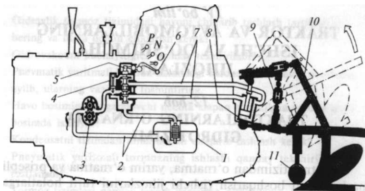
112-rasm. Traktor o'rnatma gidrotizimining sxemasi: 1- bak; 2- past bosimli moy o'tkazgich; 3- moy nasosi; 4- gidrotaqsimlagich; 5- zolotnik; 6- zolotnikni boshqarish richagi; 7- yuqori bosimli moy o'tkaz- gich; 8- gidrosilindr; 9- osma mexanizmi; 10- o'rnatma qurilma; 11- tayanch g'ildirak; P - «Ko'tarish» holati; N - Neytral holat; O - «Majburiy tushirish» holati; PI — «Ishchi yoki suzuvchi» holat.
