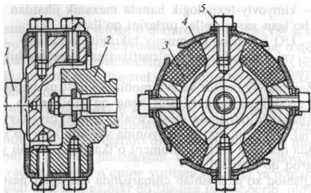
47-rasm. MT3-5M, MT3JIC traktorlarining elastik oraliq birikmasi.
