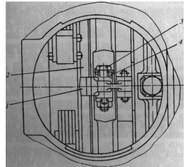
19-rasm. T-100M traktori ilashish muftasini rostlash nuqtasi. - kulachok; 2- siquvchi disk; 3- krestovinani siqib qo'yuvchi bolt; 4- krestovina.
