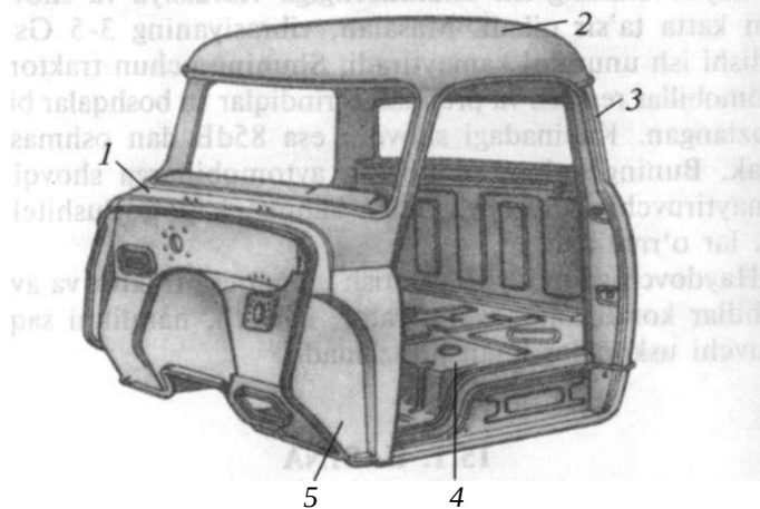
134-rasm. Ikki o'rinli yuk avtomobilining kabinasi: 1- yuqori panel; 2- torn; 3- orqa panel; 4- karkas; 5- yon panel.
