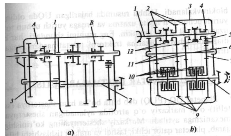
27-rasm. Tarkibli UQlarining kinematik sxemalari.
