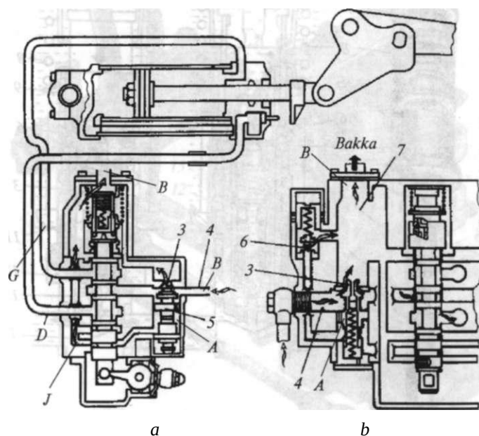
117-rasm. Hidrotaqsimlagichning neytral holatda ishlash sxemasi: a — o'tkazish klapanining ishlash sxemasi; b — saqlash klapanining ishlash sxemasi; 1 va 2- otvod (uzatish) kanallari; 3- o'tkazish klapani; 4- bosh kiritish kanali; 5- kalibrlangan teshik; 6- saqlash klapani; 7- to'kish bo'shlig'i.
