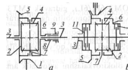
62-rasm. Differensiallar sxemasi: a — blokirovkalanadigan; b — o'z-o'zidan blokirovkalanadigan; 1- yetakchi shesternya; 2- differensialning konus shesternyasi; 3- chiqish vali; 4- satellit; 5- yetaklanuvchi shesternya; 6- differensial korpusi; 7- krestovina; 8- korpus tishlari; 9- tishli mufta; 10, 11- yetakchi va yetaklanuvchi disklar.
