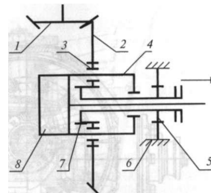
59-rasm. Ikki bosqichli blokrovkalanuvchi planetar qatorli bosh uzatma sxemasi: 1- yetakchi shesternya; 2- yetaklanuvchi shesternya; 3- satellit; 4- vodilo; 5- val; 6- yetakchi ko'priknining qo'zg'almas korpusi; 7- quyoshsimon shesternyaning tishli venesi; 8- differensial korpusi.
