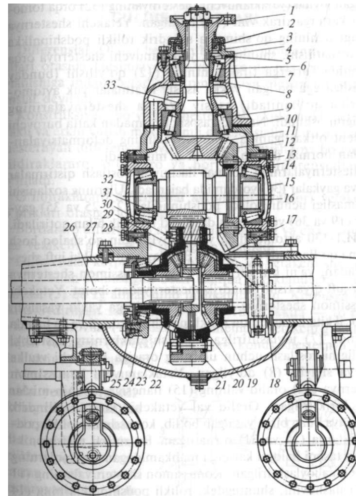
61-rasm. 3MJ1-130 avtomobilining bosh uzatmasi:
