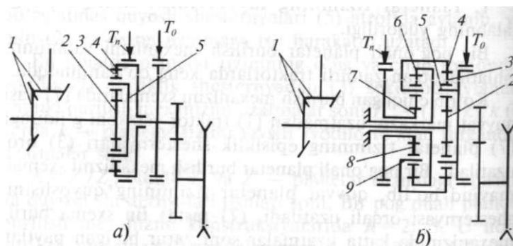
72-rasm. Bir pog'onali planetar burilish mexanizmi sxemalari: 7- markaziy uzatma; 2- quyoshimon shesternyasi; 3- satellit' 4- episiklik shesternya; 5- vodilo; 6, 7, 8 va 9- episiklik shesternya, quyoshimon shesternya, satellit va qo'shimcha planetar qatorining vodilosini; T - burilish tormozi; T_p - to'xtatish tormozi.
