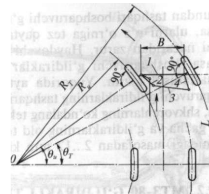
86-rasm. To'rt g'ildirakli mashinaning burilish sxemasi va rul trapetsiyasi: 1- mashinaning oldingi o'qi; 2, 4- burilish sapfalarining richaglari; 3- ko'ndalang rul tortkisi; /, 2, 3, 4- rul trapetsiyasi; 5- bo'ylama rul tortqisi.
