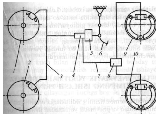
97-rasm. Ikki konturli tormoz yuritmasining sxemasi: 1- oldingi g'ildirak tormozı; 2- oldingi g'ildirak; 3- oldingi g'ildiraklar konturi; 4- asosiy tormoz silindri; 5- vakuum kuchaytirgich; 6- tormoz pedali; 7- orqa g'ildiraklar konturi; 8- tormoz regulyatori; 9- tormoz kolodkasi; 10- tormoz barabani.
