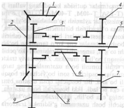
58-rasm. Ikki bosqichli qo'shaloq bosh uzatma sxemasi: 1- yetakchi shesternya; 2- yetaklanuvchi shesternya; 3, 4- silindrik shesternyalar; 5- val; 6- harakatlanuvchi tishli mufta; 7, 9- tishli g'ildiraklar; 8- differensial korpusi.
