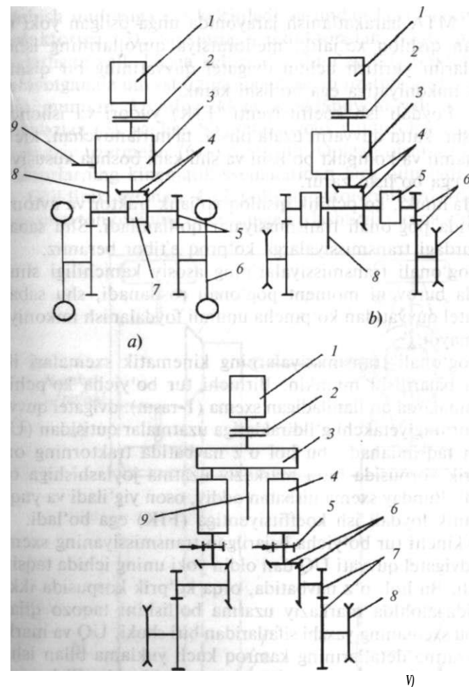
1- rasm. G'ildirakli va zanjirli traktorlarning prinsipial kinematik sxemalari: a) 1- dvigatel; 2- tishlashish muftasi; 3- uzatmalar qutisi; 4- markaziy uzatma; 5- oraliq uzatma; 6- yetakchi g'ildiraklar; 7- differensial; 8- orqa quvvat olish vali; 9- yon quvvat olish vali (QOV). b) 1- dvigatel; 2- tishlashish muftasi; 3- uzatmalar qutisi; 4- markaziy uzatma; 5- burilish mexanizmlari; 6- oxirgi uzatma; 7- yetakchi yulduzcha; 8- orqa QOV. v) 1- dvigatel; 2- tishlashish muftasi; 3- taqsimlash qutisi; 4- uzatmalar qutillari; 5- tornuvlash shkivi; 6- asosiy uzatmalar; 7- oxirgi uzatma; 8- yetakchi yulduzchalar.
