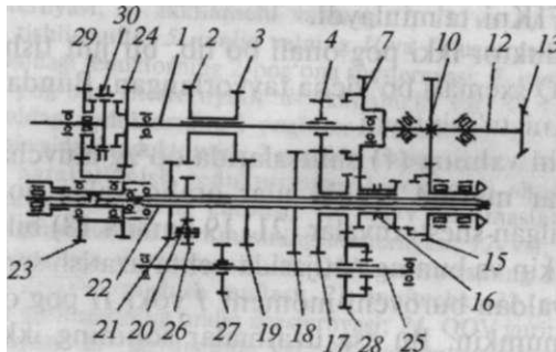
-rasm. MT3-80 traktorining tarkibli UQ kinematik sxemasi.
