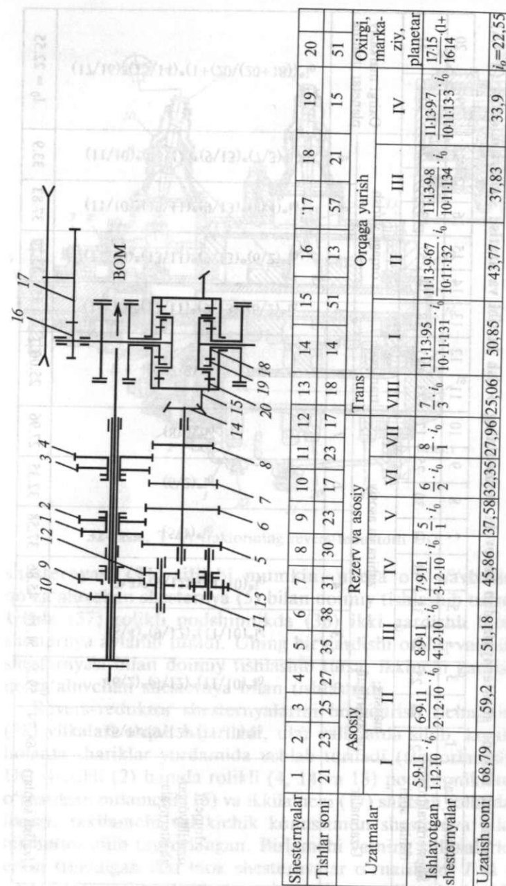
33-rasm. T-4A zanjirli traktorining UQ kinematik sxemasi.
