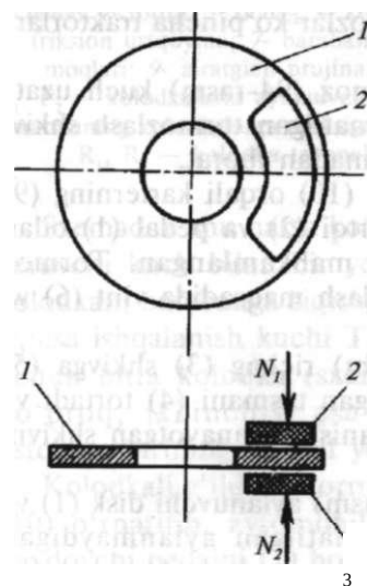
95-rasm. Avtomobillarda o'rnatiladigan diskli g'ildirak tormozı sxemasi: 1- aylanuvchi disk; 2, 3- friksion material qoplangan aylanmaydigan kolodkalar; N 1 , N 2 — diskni ikki tarafdan siquvchi kuchlar.
