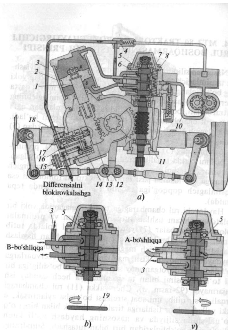
92-rasm. Hidrokuchaytirgichli rul boshqarmasining sxemasi- 1- porshen; 2- silindr; 3- ikki yekali sektor; 4- o'tkazish klapani; 5- zolotnik; 6- taqsimlagich; 7- shayba; 8- polzun; 9- saqlash klapani; 10- gidro- kuchaytirgichga moy haydash yo'li; // - chervyak; 12- soshka; 13- reyka; 14- Prujina; 15- reyka tiragichi; 16- rul chambaragi; A, B - silindr bo shhqan; 17- differensialni blokirovkalash qismi; 18- eksentrik vtulka; 19- zolotnik gaykasi.
