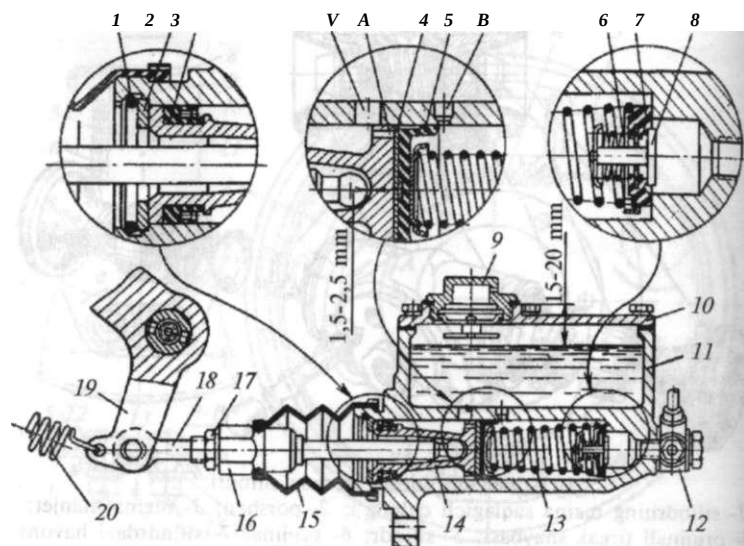
104-rasm. Gidravlik yuritmal TA3-53A avtomobili tormozining asosiy silindri:
