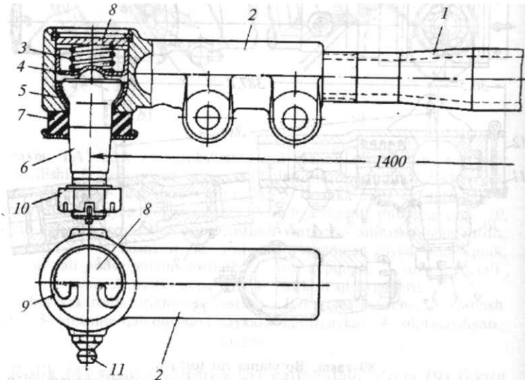
90-rasm. TA3-53A avtomobilining ko'ndalang rul tortqisi: /- ko'ndalang rul tortqisi; 2- uchlik; 3- prujina; 4- prujinaning tayanchi; 5- suxarik; 6- sharnirning kallakli barmog'i; 7- rezina zichlagich; 8- qopqog; 9- siljitmaydigan halqa; 10- gayka; 11- moydon.
