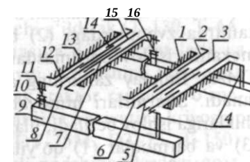
81-rasm. Zanjirli traktorlar yarim bikr to'rt nuqtali osmasining sxemasi:
