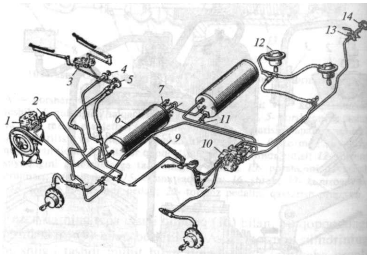
106-rasm. 3MJ1-130 avtomobilining pnevmatik yuritmalı tormoz tizimi jihozlarining sxemasi:
