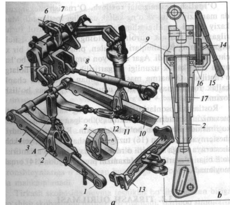
122-rasm. Uch nuqtali o'rnatish mexanizmining sxemasi: a — tuzilishi; b — rostanuvchi kashak; /- sferik (sharli) sharnir; 2- kashak vilkasi; 3- chapki kashak; 4- bo'ylama tortqining oldingi qismi; 5- bo'ylama tortqining o'qi; 6- silindr shtogi; 7- burish richagi; 8- markaziy tortqi; 9- o'ng kashak reduktori; 10- bo'ylama tortqining orqa qismi; // - cheklash zanjiri; 12- zanjirning taranglagichi; 13- tirkash qurilmasi; 14- moydon; 15- dasta; 16- shesternyalar; 17- kashak trubasi.
