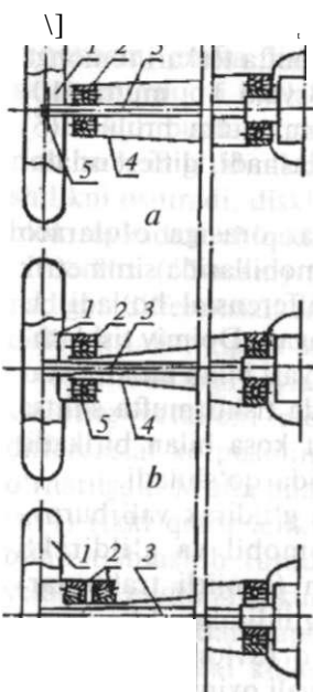
64-rasm. Yarim o'qlar turlari (yetakchi g'ildiraklar vallari):
