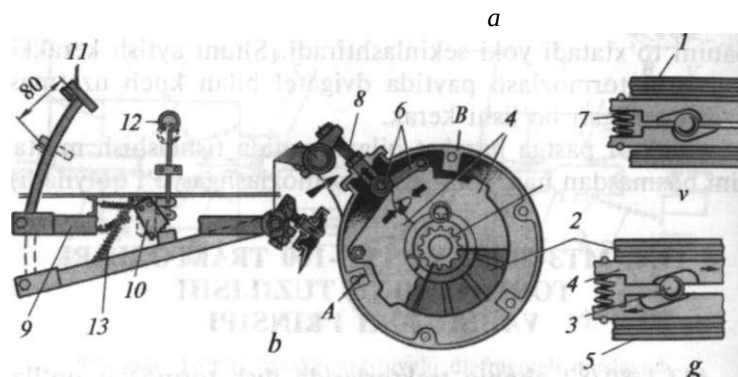
101-rasm. MT3-80/82 va TTZ-100K traktorlarining diskli (gardishli) tormozi:
