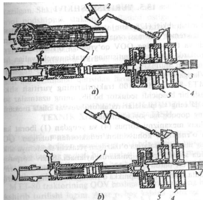
127-rasm. QOVning ishlash sxemasi: a - sinxron QOV yuritmasi (QOV uzilgan); b - mustaqil QOV yuntmasi (QOV ulangan); 1- tishli mufta; 2- QOV ni boshqarish richagi; 3- QOVning chiqqan uchi; 4- vodilo tormozi; 5- markaziy shesternya tormozi.
