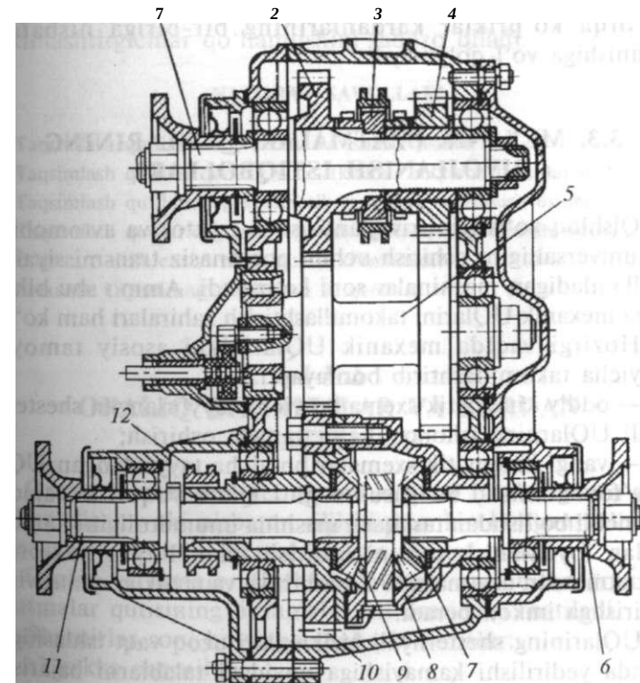
46-rasm. BA3-2121 «HnBa» yengil avtomobilining taqsimlash qutisi: 1- yetakchi val; 2- sekinlashtiradigan uzatma shesternyasi; 3- uzatmalarni almashtiruvchi mufta; 4- yuqori uzatma shesternyasi; 5- oraliq val; 6- orqa ko'priklar yuritmasining vali; 7- shesternya; 8- differensial korpusi; 9- satellitlar; 10- differensial shesternyasi; 11- oldingi ko'priklar yuritmasining vali; 12- differensialni blokirovkalash muftasi.
