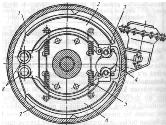
110-rasm. 3HJ1-130 avtomobilining orqa g'ildirak tormozi: /- tormoz barabani; 2, 6- tormoz kolodkalari; 3- kolodka roligi; 4- keruvchi moslama; 5- kolodkalarni bir-biriga tortuvchi prujina; 7- kolodkaning friksion ustqoymasi; 8- kolodkaning tayanch barmog'i.
