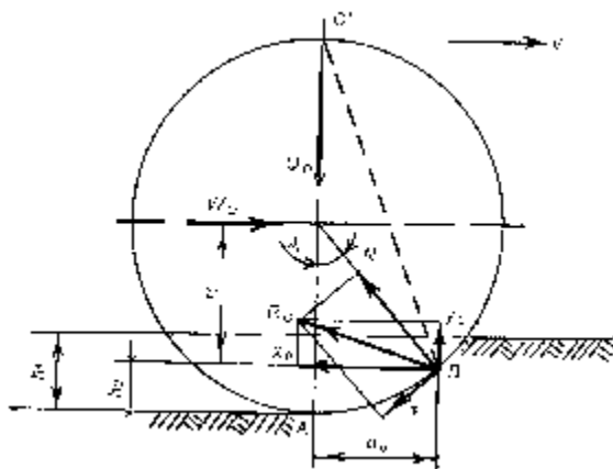
10-chizma. Qattiq gardishli g'ildirakka ta'sir etuvchi kuchlar.
