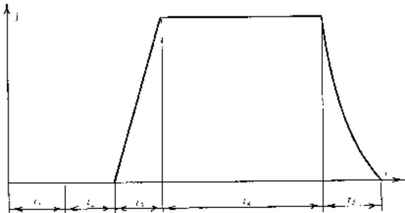
45-chizma. Umumiy tormoz yoʻlining tashkil etuvchilari.
