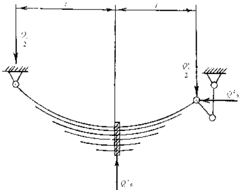
65-chizma. Ressora hisobiga oid shakl.
