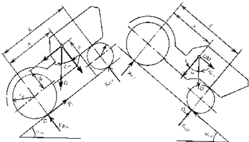
23-chizma. Bo'yлама turg'unlikka oid shakllar.
