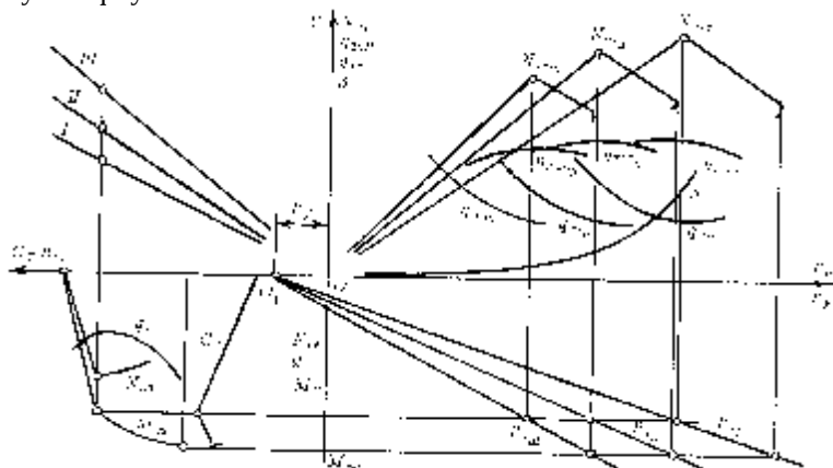
33-chizma. Traktorning tortish kuchi bo'yicha tasnifi.
