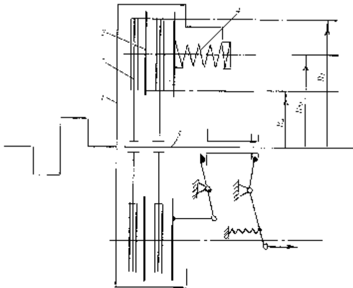
58-chizma. Ikki diskli friksion tishlashish muftasi.
