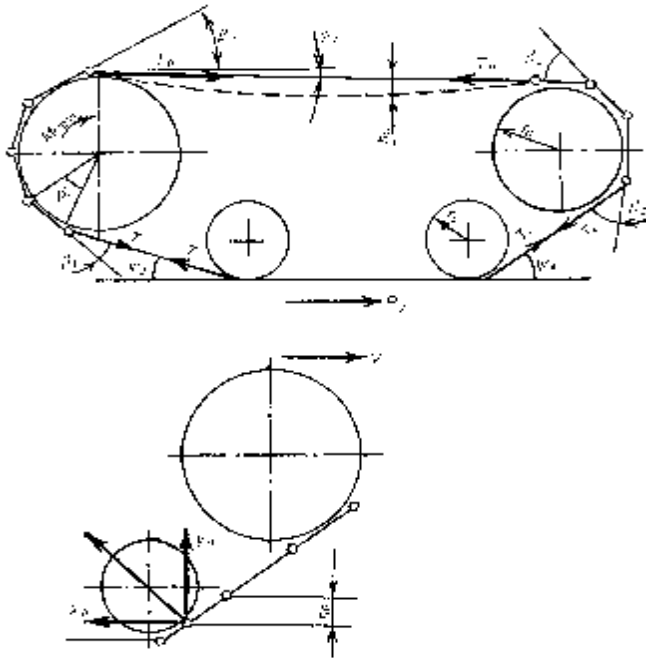
18-chizma. Zanjirli harakatlantirgichning dinamikasiga oid shakl. Taranglovchi qismdagi T kuch quyidagicha aniqlanadi:
