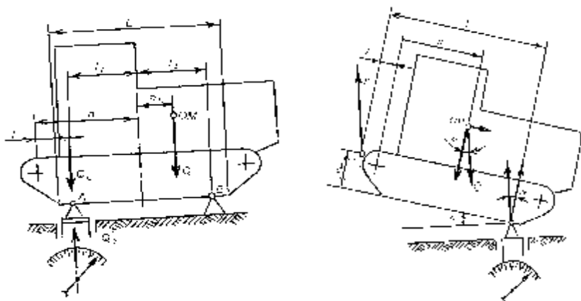
21-chizma. Og'irlik markazining koordinatalarini topishga doir shakl.
