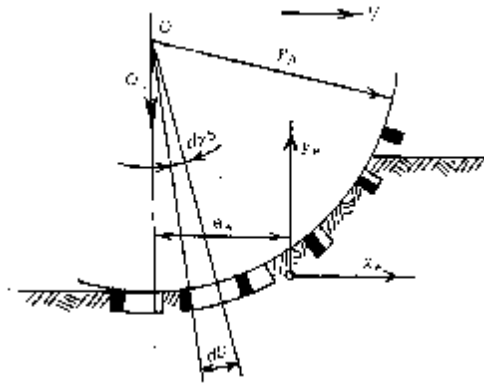
13-chizma. Shataksirash va ilashish ko'effitsiyentlarini aniqlashga doir shakl.
