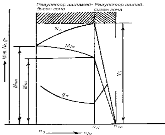
1-chizma. Dizel dvigatelining regulator tasnifi:
