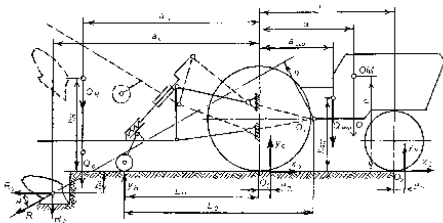
16-chizma. Qishloq xo'jaligi mashinasi bilan ishlayotgandagi vertikal kuchlarni aniqlash.
