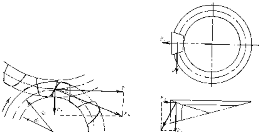
59-chizma. Shesternya tishlariga ta'sir etuvchi kuchlar.
