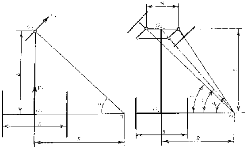
47-chizma. G'ildirakli mashinalarning burilish kinematikasiga doir shakl.
