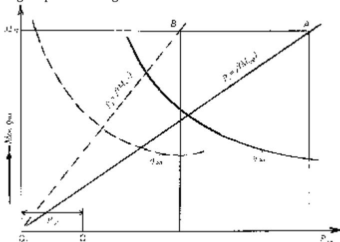
31-chizma. P_u = f(M_{dv}) funksiyaga oid nursimon diagramma.
