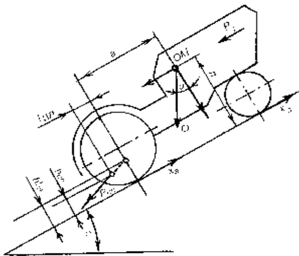
8-chizma. Kuch balansiga doir shakl.
