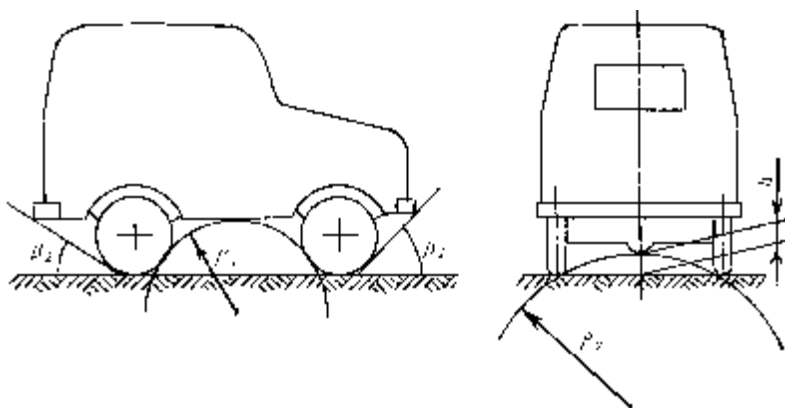
56-chizma. O'tuvchanlik parametrlari.
