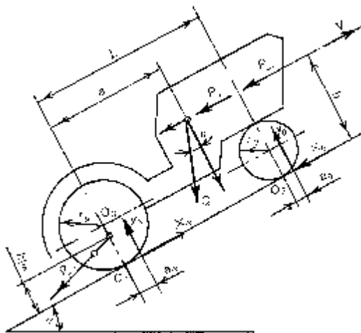
14-chizma. Vertikal (tik) kuchlarni aniqlashga doir shakl.
