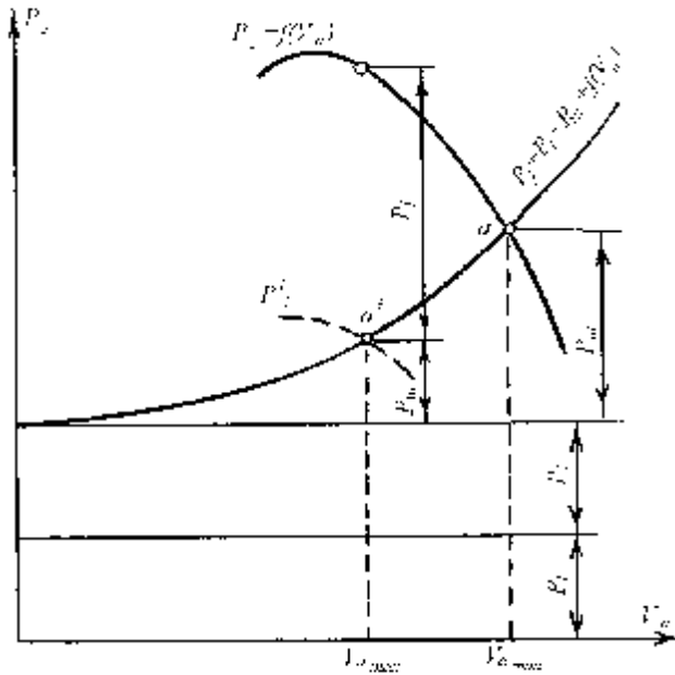
38-чизма. Автомобилнинг куч баланси.
