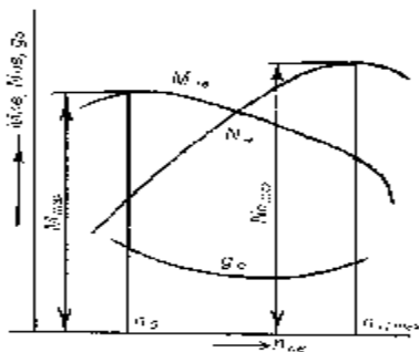
3-чизма. Карбюраторли двигателининг тезликлар таснифи.
