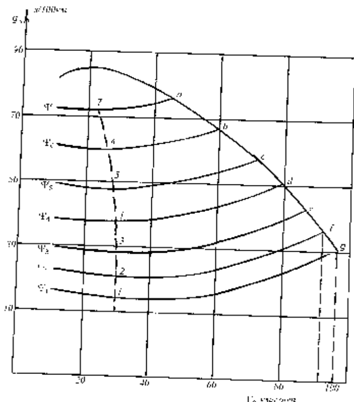
46-chizma. Avtomobilning iqtisodiy tasnifi.
