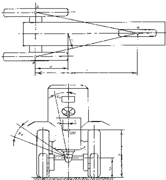
26-chizma. Ko'ndalang turg'unlikni aniqlash.
