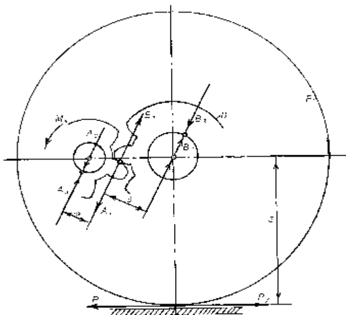
4-chizma. Tashqi va ichki kuchlarni aniqlashga doir shakl.
