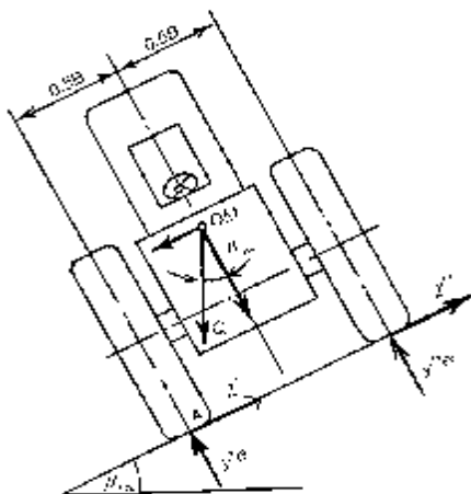
25-chizma. Ko'ndalang turg'unligini aniqlash.
