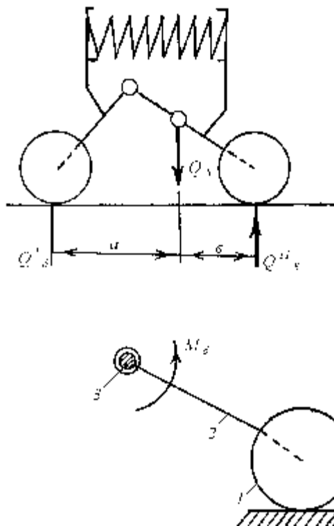
66-chizma. Elastik (a) va torsion osmalar.
