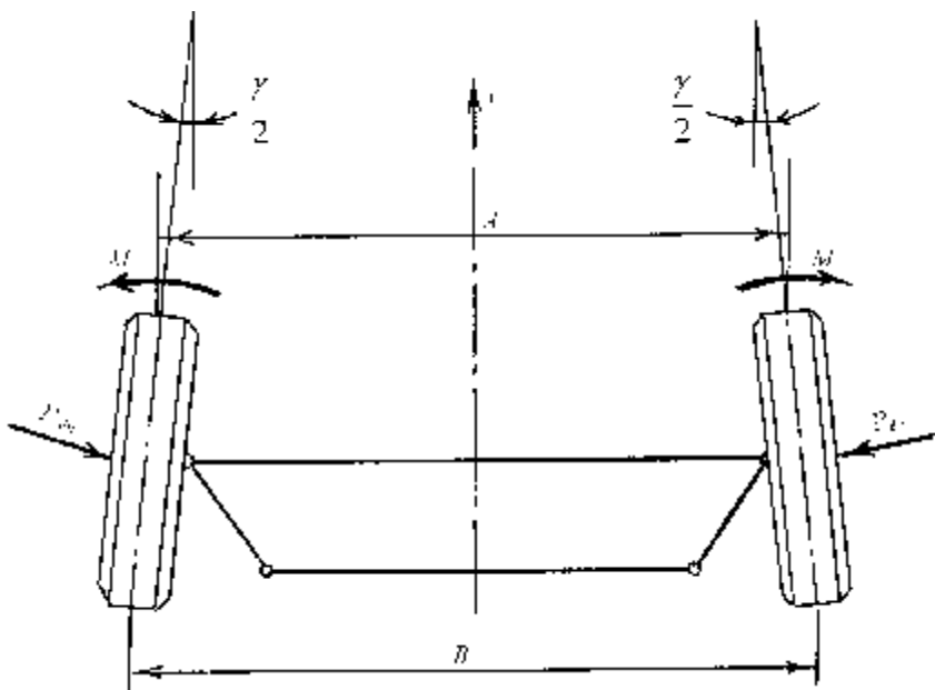
52-chizma. G'ildiraklarning yaqinlashuvi.
