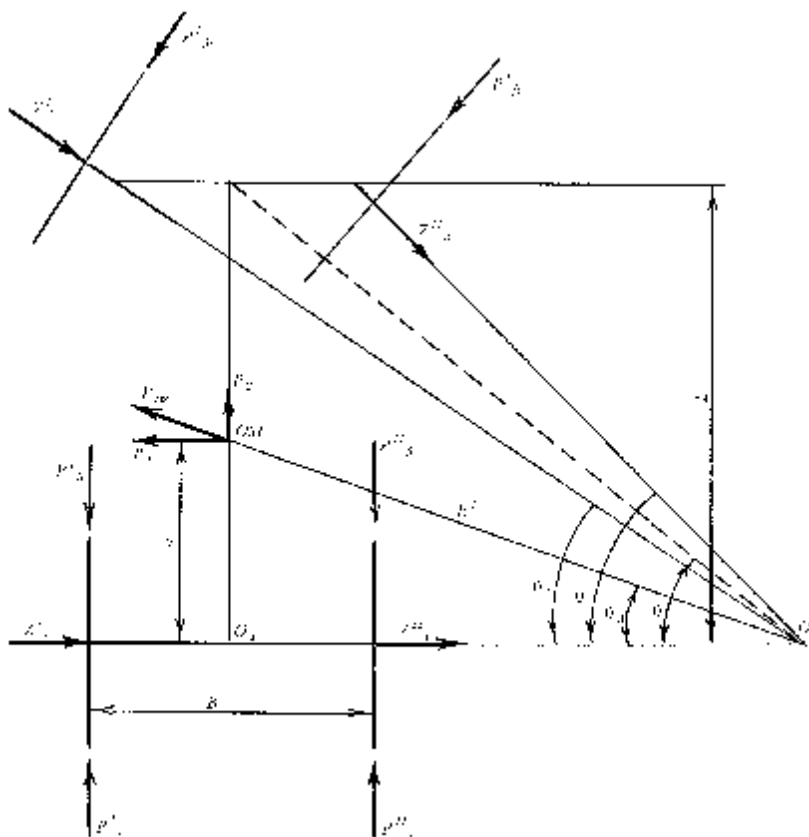
48-chizma. Burilish dinamikasiga doir shakl.
