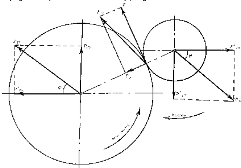
60-chizma. Uzatmalar qutisi o'qlariga ta'sir etuvchi kuchlar.
