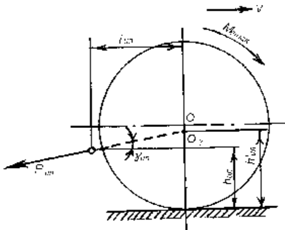
7-chizma. Pritsepning shartli nuqtasini topishga doir shakl.
