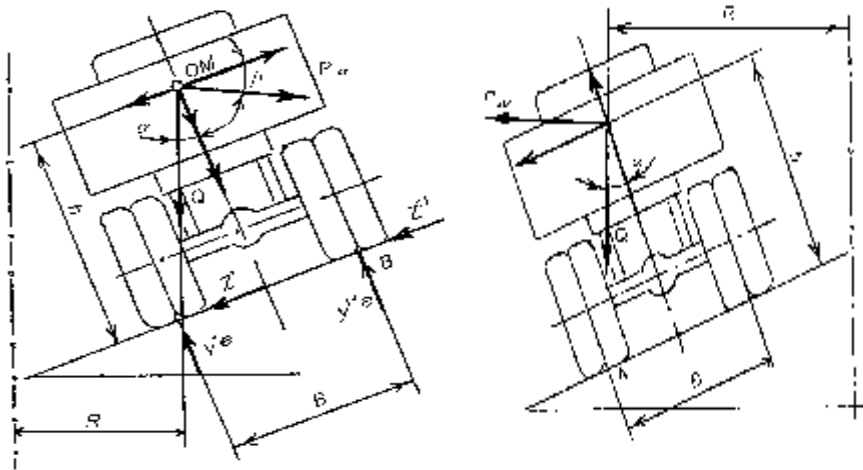
28-chizma. Qiyalikda burilayotgan avtomobilga ta'sir qiluvchi kuchlar.
