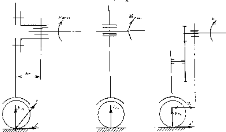
63-chizma. Yarim o'qlarning hisobiga oid shakllar.
