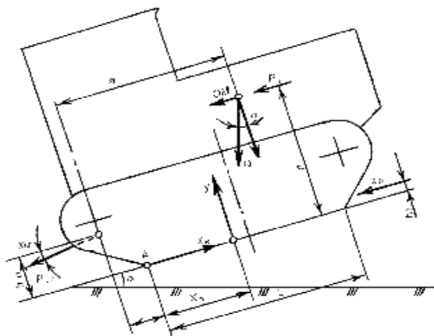
19-chizma. Bosim markazini aniqlash.
