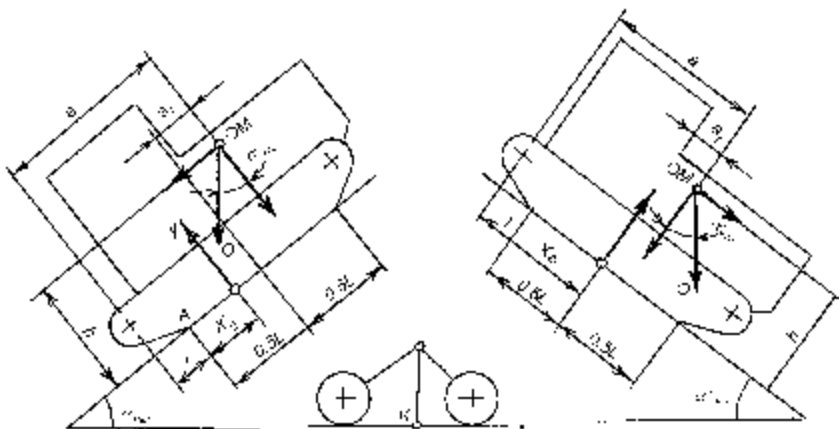
24-chizma. Bo'ylama turg'unligini aniqlash.
