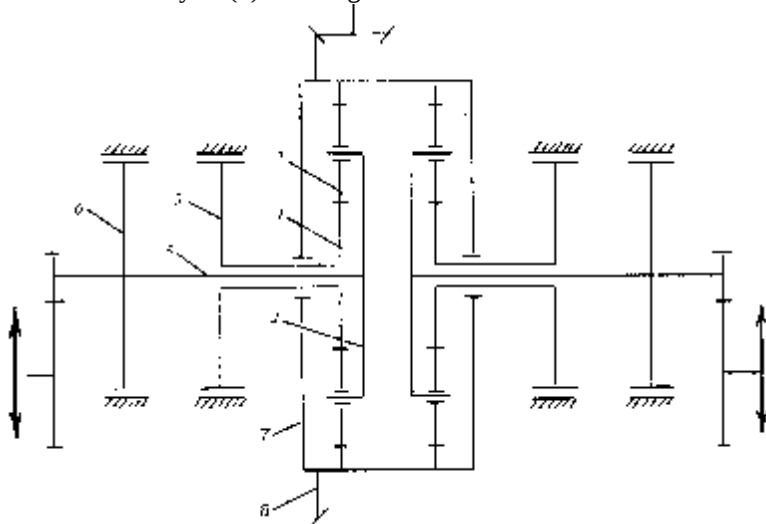
54-чизма. Планетар бурилиш механизми тракторнинг орқа кўприги.
