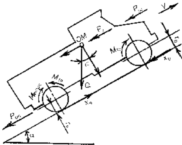
5-chizma. Avtomobilning harakatiga ta'sir etuvchi kuchlar.
