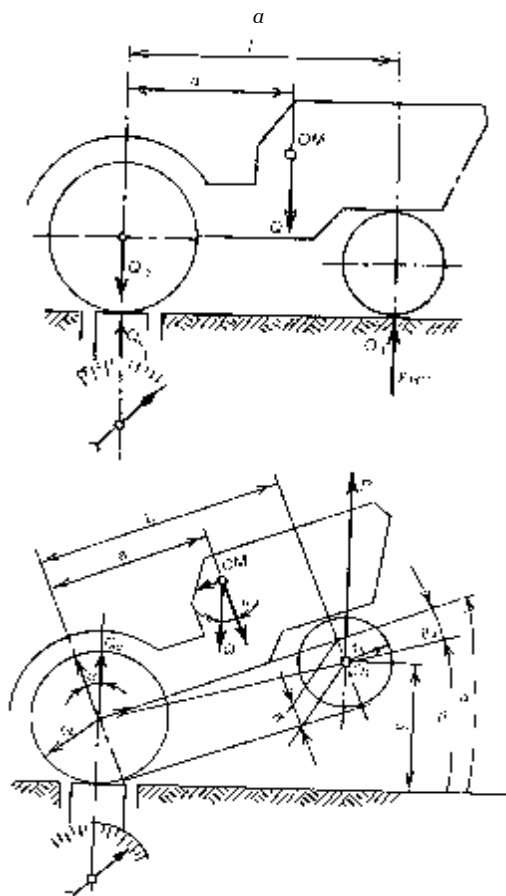
20-chizma. Og'irlik markazi koordinatalarini topish.
