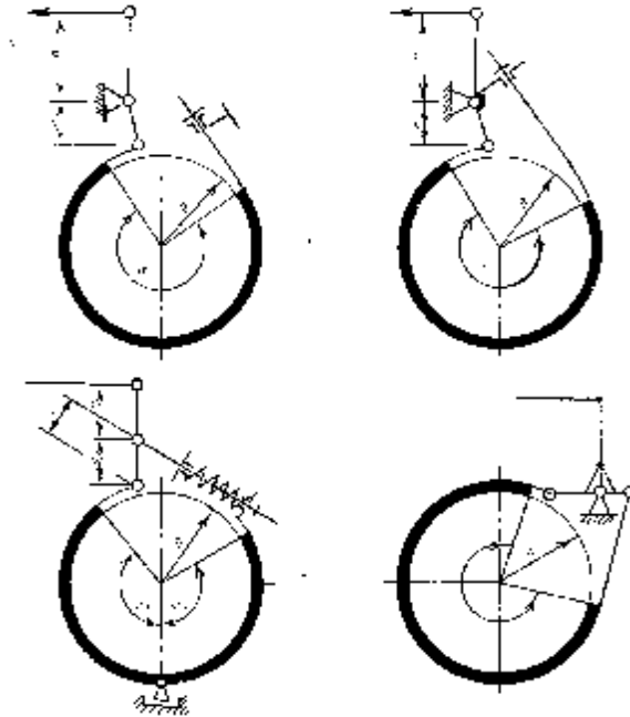
68-chizma. Lentali tormozlar shakli.
