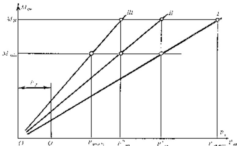
32-chizma. Uzatmalarning geometrik qatoriga oid nursimon diagramma.
