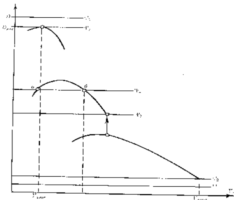
39-chizma. Avtomobilning dinamik tasnifi.
