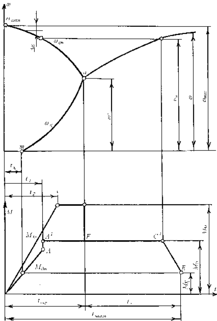
37-chizma. Traktorning shig'ov bilan harakatlanish dinamikasi.
