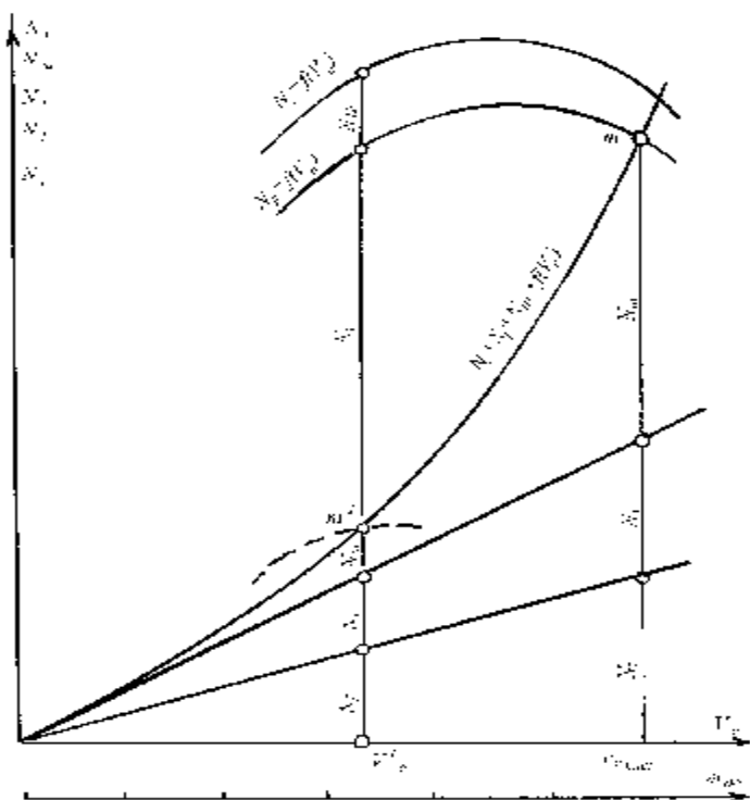
40-chizma. Avtomobilning quvvat balansi grafigi.
