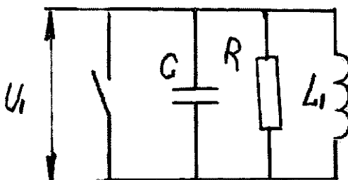
26.5-rasm. Birlamchi cho'lg'amni ekvivalent sxemasi
