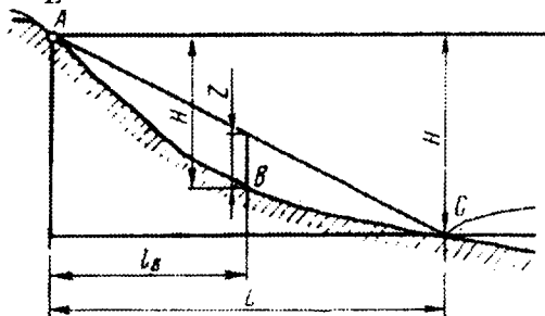
31.43 – расм. Қор кўчкиси тезлигини аниқлашга оид схема: А – кўчкининг ажралиш (узилиш) нуқтаси; С – кўчки ётқиқиқларининг чегараси
