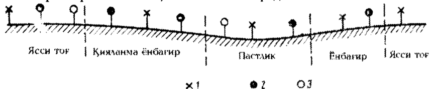
23.7 – расм. Жойнинг релефига қараб шурф ва қазималарни жойлаштириш схемаси: 1 – шурф, 2 – қазималар; 3 – ярим шурф
