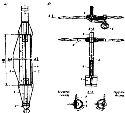
28.3—расм. Торф сынаш учун асбоблар: а—торф намуналари олиш учун ТБ—5 торф бурғуси; б—силжишга қаршиликни ўлчаш учун СК—8 силжиш ўлчагич қанотча; 1—винт; 2—ярим конус; 3—пичок; 4—ўзак; 5—қошиқ; 6—индикатор; 7—қанотча; 8—штангнинг грунтта ишқаланишини ҳисобга олиш қурилмаси; 9—дастали ўлчаш калағи
