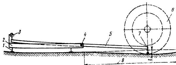
27.9—расм. Йўл тўшамаларининг деформацияларини ўлчаш учун рычагли эгилиш ўлчагичнинг схемаси: 1—асбобнинг ўрнатиш винтлари; 2—асбоб станиниси; 3—асбобнинг қўзғалмас станинасига маҳкамланган, эгилишни ўлчайдиган индикатор; 4—шарнир; 5—ричаг; 6—синов автомобилнинг гиддираги; 7—қопламага таяниб турадиган стержен; 8—йўл тушамаси эгилишининг косаси;
