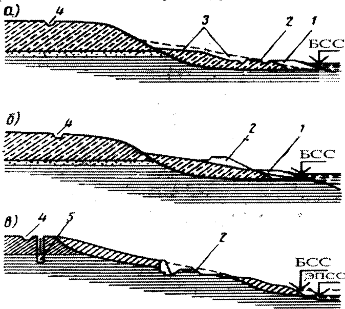
31.37 – расм. Кўчадиган массивларнинг турғунлигини ошириш учун тадбирлар: а – нишабни қиялатиш; б – контрбанкетта грунт тўкиш; в – тирак девор қуриш:
