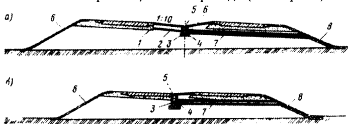
33.6 – расм. Виразларда ажратиш полосасидаги сувни четлатишни таъминлаш схемаси: а – ажратиш полосаси кенг бўлганида; б – ажратиш полосаси энгиз бўлганида; 1 – қум қатламидан сувни йиғиш учун дренаж найчаси; 2 – сувни новга четлатувчи найча; 3 – сув қабул қилгич; 4 – коллектор; 5 – сув қабул қилиш панжараси; 6 – чим ётқизиш; 7 – сувни новдан четлатиш; 8 – қияликдаги бетон нов.
