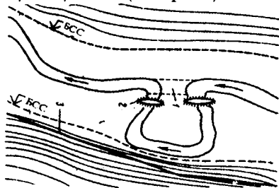
31.4 – расм. Йўл пойининг тагидан ювилиб кетиш хавфини камайтириш учун ўзани тугрилаш: 1 – тўғрилланган ўзан; 2 – дамбалар; 3 – йўл ўқ чизиги
