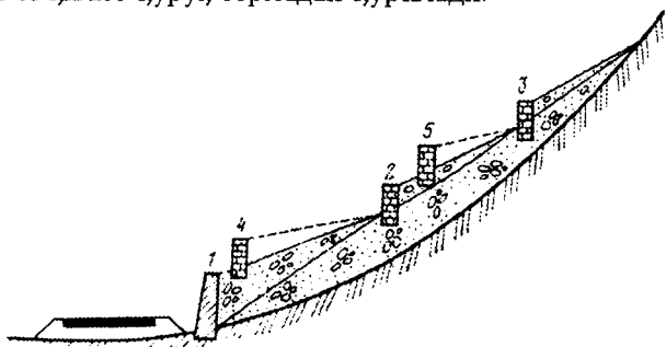
31.30 – расм. Кам кўчадиган тўкманинг шлейфи бўйича ўтадиган йўлни тирак деворлар билан мустаҳкамлаш (рақамлар деворни қуриш кетма – кетлигини билдиради).
