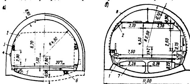
31.21 – расм. Автомобил йўларида туннелларнинг кўндаланг профили: а – шамоллатилмайдиган; б – шамоллатиладиган; 1 – қоплама; 2 – ёритиш асбоблари; 3 – светофор; 4 – телефон ашпарати; 5 – нов; 6 – дренаж; 7 – тоза ҳаво; 8 – ифлосланган ҳаво
