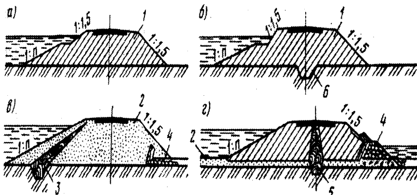
29.6 — расм. Туپроқ тўғонларининг кўндаланг профиллари: а — бир жинсли грунтлардан; б — филтрацияга қарши тишли; в — экранли; г — сув ўтказмайдиган грунтли; 1 — қумлоқ туپроқ; қумлоқ туپроқ; 2 — қум; 3 — экран; 4 — дренаж; 5 — сув ўтказмайдиган ядро; 6 — филтрацияга қарши тиш
