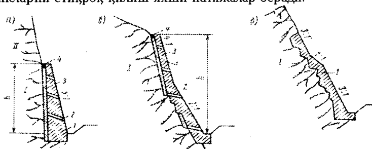
31.27 — расм. Ёпиб (беркитиб) турувчи тирак деворларга мисоллар: а ва б — зах қочирувчи тўкмали деворлар; в — қоя жинсга маҳкамланган девор; 1 — кучсиз қоя; II — мустаҳкам қоя; 1 — ёпиб турувчи девор; 2 — сув чиқариш тешиги; 3 — зах қочирувчи тўкма; 4 — сув ўтказмайдиган қилиб маҳкамлаш
