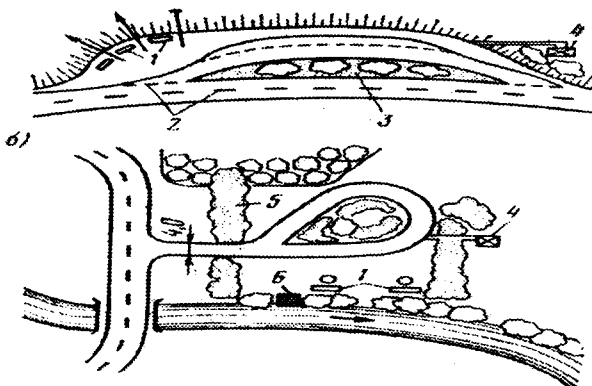
34.1 – расм. Автомобиллар бекати учун майдончани режалаш: а – кўркем кўринишли жойлар яқинидаги дам олиш майдончаси; б – дарё ёнидаги дам олиш майдончаси; 1 – столлар ва скамейкалар; 2 – режалаш қизиги; 3 – бекатни йўлдан ажратиб турувчи оролча; 4 – ҳожатхона ва аҳлатхона; 5 – бутазор; 6 – дарёга олиб тушадиган зинапоя
