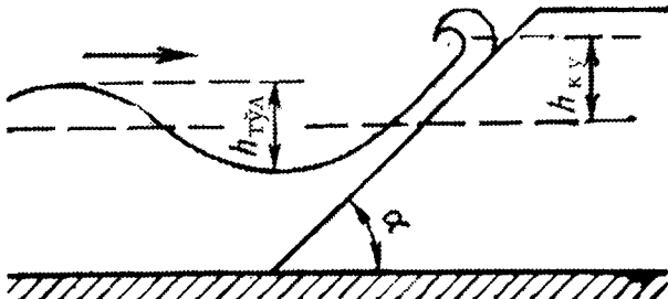
21.2 — расм. Кўтарма ёнбағрига тўлқиннинг келиб урилиши схемаси
