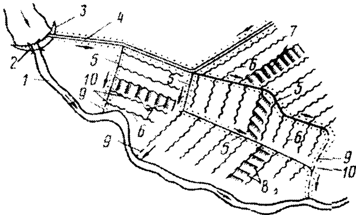
32.1 – расм. Суғориш тизимининг схемаси: 1 – дарё; 2 – тўғон; 3 – сув олиш иншооти; 4 – магистрал канал; 5 – тақсимлаш каналлари; 6 – вақтинчалик суғориш каналлари; 7 – сув чиқариш эгatlари; 8 – суғориш эгatlари; 9 – сув йиғиш каналлари; 10 – йўл бўйича экилган дарахт (бута)лар
