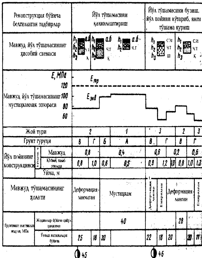
27.10 – расм. Йўл тўшамаси муостаҳкамлигининг графиги: а, б – асфалт – бетон; ч – чақик тош; қ – қум; ш – шағал; с.и. – сирт ишлави; А – енгил қумлоқ тупроқ; Б – қумлоқ тупроқ; В – қумоқ тупроқ; Г – чангсимон қумоқ тупроқ
