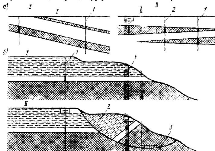
23.8 — расм. Бурғиланган қудуқлар сони етарлича бўлмаганида жойининг геологик қирқими тўғрисидаги нотўғри тасаввурларга мисоллар:
