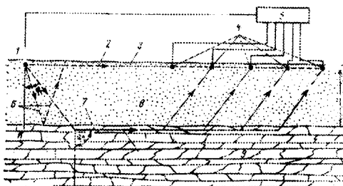
23.10 – расм. Сейсмик усул билан тоғ жинсларининг ётиш чуқурлигини аниқлашга оид схема: 1 – зарб ёки портлаш ўрни; 2 – тўғри тўлқиннинг йўли; 3 – грунт сирти; 4 – геофонлар; 5 – қайд этиш (регистратор); 6 – қайтган тўлқиннинг йўли; 7 – синган тўлқиннинг йўли; 8 – грунтнинг сирт қатлами; 9 – тоғ жинси
