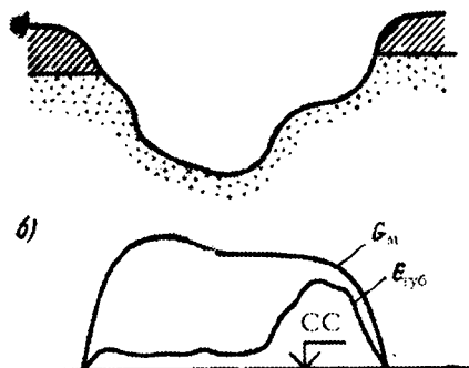
20 2 – расм. Муаллақ ва туб ўтириндилар (чўкиндилар) нинг ўзан эни бўйича тақсимланиш и: а – ўзанининг кўндаланг профили; б – чўкиндилар сарфининг эшо раси;
