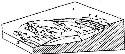
31.35— расм. Кўчкининг тузилиш схемаси: 1— кўчки майдони; 2— асосий поғона (узилиш девори); 3— узилиш дарзи; 4— узилиш қирғоғи; 5— кўчки чўққиси; 6— ички қирғоқ; 7— сирпаниш сирти; 8— кўчки танаси; 9— кўпчиш дарзлари; 10— кўчки сирти релефининг нотекислиги; 11— кўчкининг этаги; 12— кўчки асосининг деформацияси; 13— туб массив
