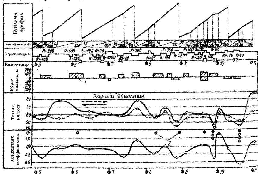
27.3. Йўл бўйича ҳаракатланиш тезликларининг ўзгариш графиги: 1 — текланган кўринишлик зонаси; 2 — йўл — транспорт ҳодисалари юз берадиган жой
