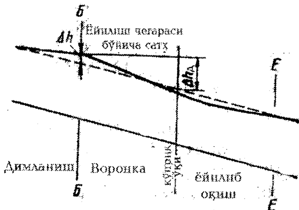
20.19 – расм. Димланишларни (подпор) ҳисоблашга оид схема (кўприк олдида, кўприк остида ва кўприкга келиш йўллари кўтармаси ёнида):
