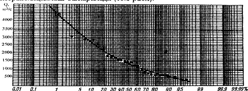
19.3— расм. Максимал сарфларнинг эҳтимоллик эгри чизиғи
