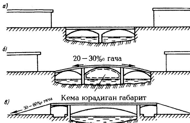
35.16 – расм. Шаҳар кўприкларининг жойлашув вариантлари
