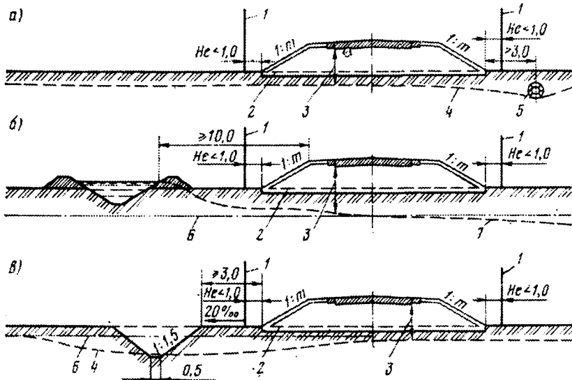
32.2 – расм. Сунъий суғориш ҳудудларида йўларнинг кўндаланг профиллари: а – ёпиқ зовурлар ва коллекторлар бўйлаб; б – магистрал ариқлар бўйлаб; в – очик коллекторлар бўйлаб; 1 – ажратилган жой чегараси; 2 – ўсимликли грунтнинг олиб ташланадиган қатлами; 3 – йўл тўшамаси пастининг ҳисобий кўтарилиши; 4 – сизот сувларининг зовурлар ёки ариқлар билан пасайтирилган сатҳи;
