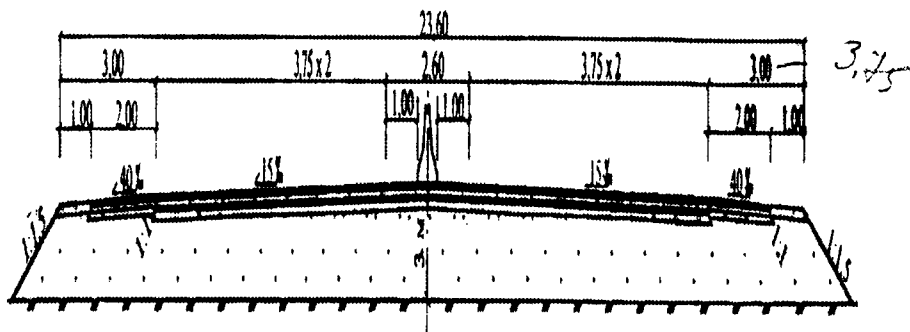
33.3— расм. Ўзбекистон автомагистралларининг кўндаланг профиллари
