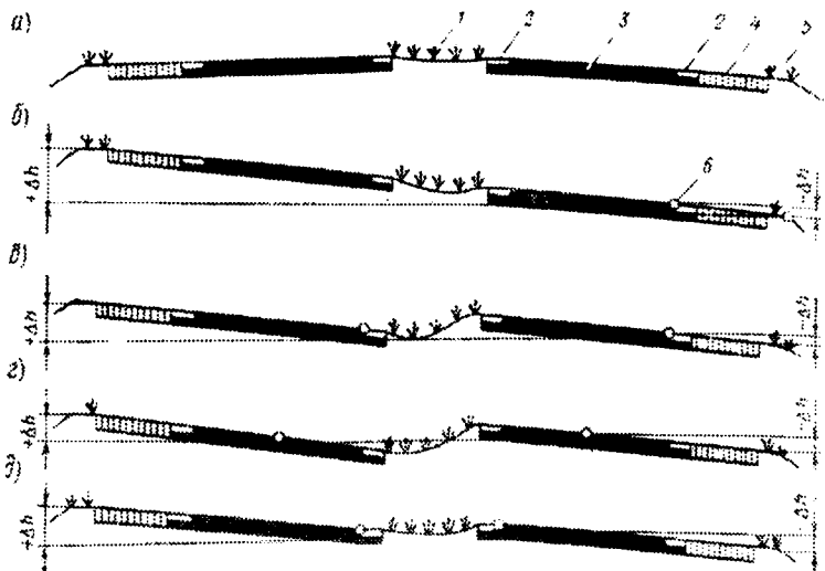
33.5 – расм. Автомобил магистралларида виражлар қуриш усуллари: а – тўғри участкалардаги кўндаланг профил; б – кўндаланг профилнинг йўл пойининг қирғоғига ёки қоплама ички қиррасига нисбатан бурилиши; в – қатнов қисмларининг уларнинг ички қирраларига нисбатан бурилиши; г – қатнов қисмларининг уларнинг ўқларига нисбатан бурилиши; д – қатнов қисмларининг ажратиш полосасига ёндош (туташ) қирраларига нисбатан бурилиши;
