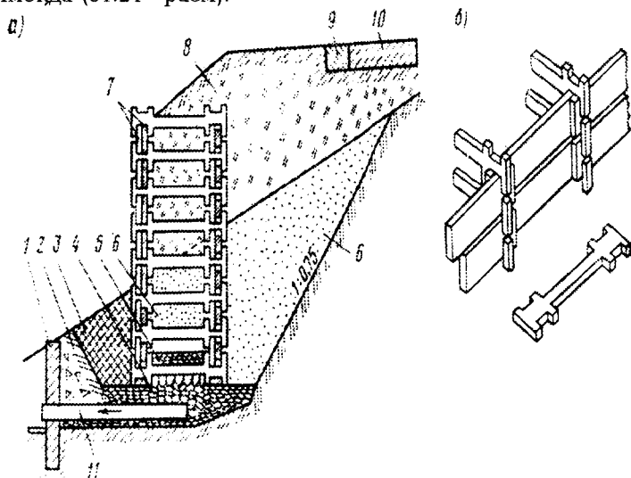
31.24—расм. Сепояли йиғма темир—бетон девор: а—умумий кўриниши; б—йиғиш схемаси 1—қувур каллаги (қувурни ушлаб турувчи деворча); 2—шлак; 3—лой; 4—тош; 5—чақиқ тош ёки шағал; 6—қум; 7—йиғма темир—бетон элементлар; 8—кўтарма; 9—йўл тўшамасининг четки полосаси; 10—йўл тўшамаси; 11—дренаж қузури
