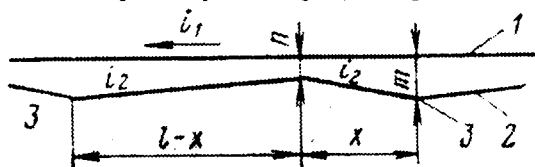
35.14 – Новнинг схематик бўйлама профили: 1 – йўлка қирғоғининг тепаси; 2 – нов туби; 3 – қудуқлар
