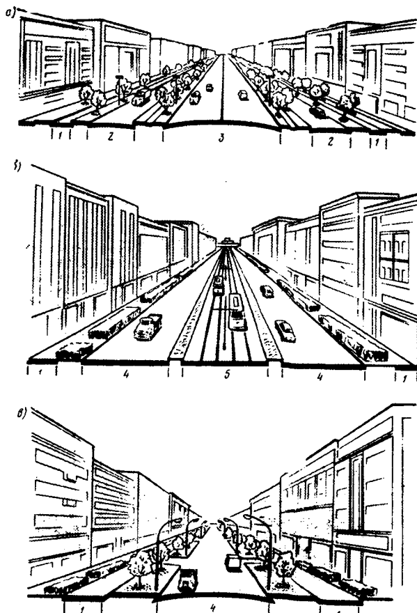
35.5 – расм. Кўчаларнинг кўндаланг профиллари: 1 – йўлка; 2 – маҳаллий ҳаракат; 3 – транзит ҳаракат; 4 – қатнов қисми; 5 – алоҳида трамвай йўли
