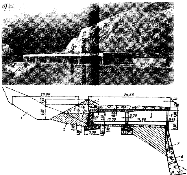
31.32 – расм. Тош тўшадиган участкалардаги ҳимоя галереялари: а – умумий кўриниши; б – галереянинг кўндаланг профили 1 – ушлаб қолувчи ҳандақ; 2 – одатдаги грунт; 3 – шағалли аралашма; 4 – зах қочириш қатлами; 5 – йиғма темир бетон элементлардан қурилган галерея; 6 – пастки тирак девор; 7 – бўйлама бетон тўсинни маҳкамловчи анкер; 8 – метал устун
