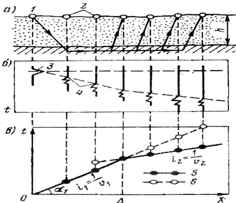
23.11 – расм. Қоянинг ётиш чуқурлигини ҳисоблашга оид схема: а – ашпаратуранинг жойлашиши; б – тўлқинларнинг геофонга келишини ёзиб олиш; в – тўлқинларнинг тарқалиш давомийлигининг геофонгача бўлган масофага боғлиқлиги;
