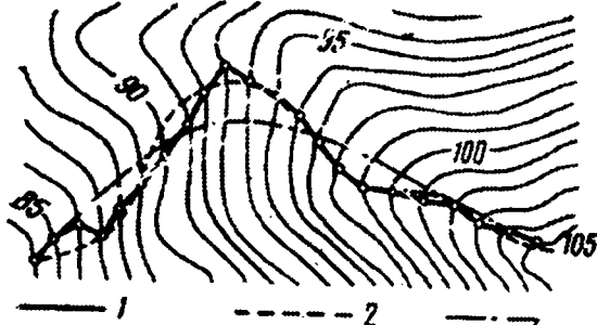
31.11 – расм. План бўйича горизонталларда ўтказилган берилган қияликдаги чизиққа раван трассани мослаштириш: 1 – берилган қияликдаги чизиқ; 2 – берилган қияликдаги чизиққа жуда яқинлашган трасса кичик радиусли эгри чизиқлар билан; 3 – анча раванроқ трасса
