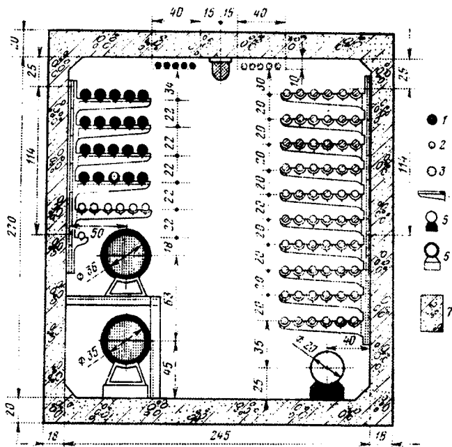
35.4 – расм. Тўғри тўртбурчак кесимли коллекторнинг схемаси: 1 – куч кабеллари; 2 – алоқа кабеллари; 3 – резерв; 4 – кабеллар учун токчалар; 5 – водопровод; 6 – иссиқлик тармоғи; 7 – темир – бетон
