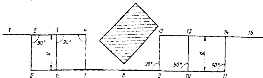
23.3–расм. Қозиқ қоқишда тўсиқларни айланиб ўтиш: 1–15–айланиб ўтишда чизиқларни ўлчаш кетма-кетлиги
