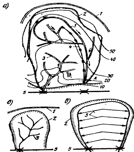
31.36—рasm. Кўчкига қарши тадбирлар мажмуи: а— йўл ёнидаги кўчкига қарши тадбирлар; б— жала ва эриган қор (муз) сувларининг оқиш йўлларидаги ариқлар тармоғи; в— кўчкенинг текисланган сиртидаги ариқларнинг бир текис тармоғи; 1—тепаарик; 2—кўчки чегараси; 3—тош териб маҳкамланган ариқлар; 4—штоля; 5—йўл
