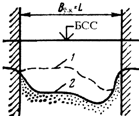
20.10-расм. Энг кам узунликдаги кўприк:
