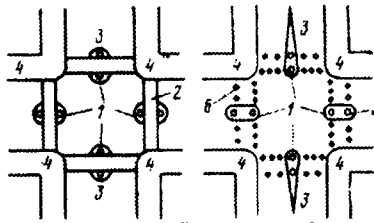
35.11 – расм. Кўчалардан ўтиш жойларида хавфсизлик оролчаларининг схемалари 1 – хавфсизлик оролча; 2 – рангли бетон; 3 – қатнов қисми; 4 – йўлчалар; 5 – ёритиб турувчи тумбалар; 6 – рангли плиталар.
