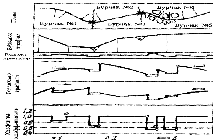
24.4 – расм. Хавфсизлик коэффициентлари графиги:
