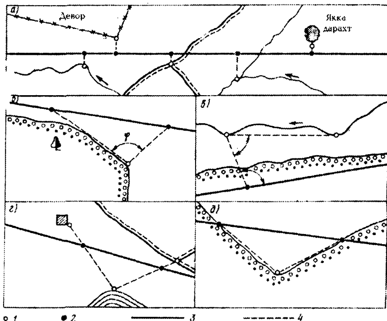
23.1 — расм. Трассани карталар ва аэросуратлардан жойга чиқариш схемаси: а — таниқлиқ нуқталари трасса яқинида жойлашган; б — в — таниқлиқ нуқталаридан нуқталарни трассада геодезик ўлчашлар билан аниқлашда фойдаланилади; г — трасса таниқлиқ нуқталарини бирлаштирувчи чизиқларни кесиб ўтади; д — таниқлик белгилари трасса кесиб ўтадиган контурларда жойлашган; 1 — трассадаги нуқта; 2 — таниқлик нуқтаси; 3 — трасса; 4 — трассани аниқлаш учун ёрдамчи чизиқ.
