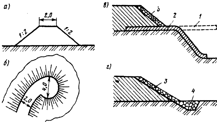
21.19—расм. Оқим йўналтирувчи дамбалар конструкцияларининг деталлари: а — одатдаги кўндаланг кесим; б — дамбанинг бош қисмида чўққисини кенгайтириш; в — дамба ёнбағир этагини тўшак (түфяк) билан мустаҳкамлаш; г — дамба этагидаги рисберма; 1 — ювилишгача түфякнинг ўрни; 2 — ювилишдан кейин түфякнинг ўрни 3 — ёнбағир мустаҳкамлагичи; 4 — рисберма
