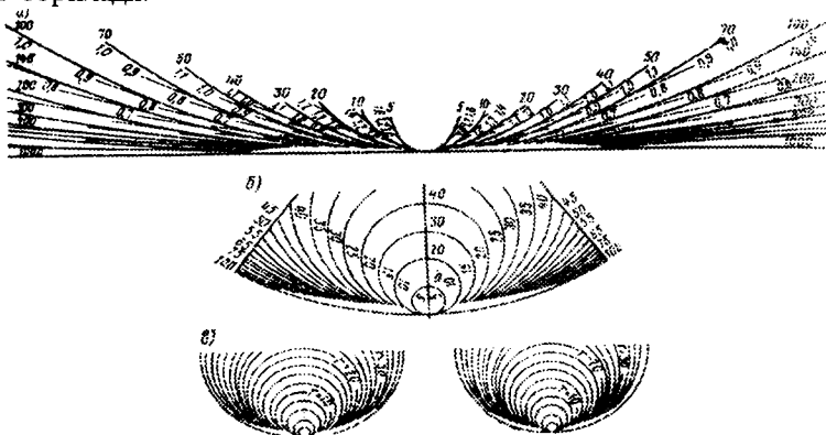
25.5— расм. Жойнинг стереомодели бўйича трасса эгриларини танлаш учун шаффоф андазалар:
