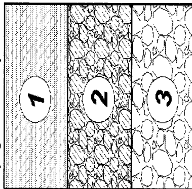
4.35-rasm. Monolit sementbeton qoplama yo'l to'shamasining tavsiya etilgan konstruksiyasi:
