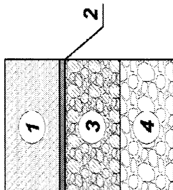
4.34-rasm. Monolit sementbeton qoplamali yo'l to'shamasining mavjud namunaviy konstruksiyasi:
