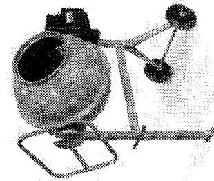
3.1-rasm. Laboratoriyada qorishma tayyorlash uchun ishlatiladigan baraban tipidagi va silindrik idishli betonqoragichlar
