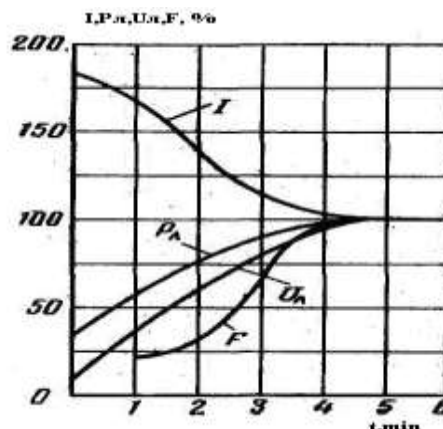
9.3-расм. ДРТ лампасининг асосий қийматларини ўзгариши.
