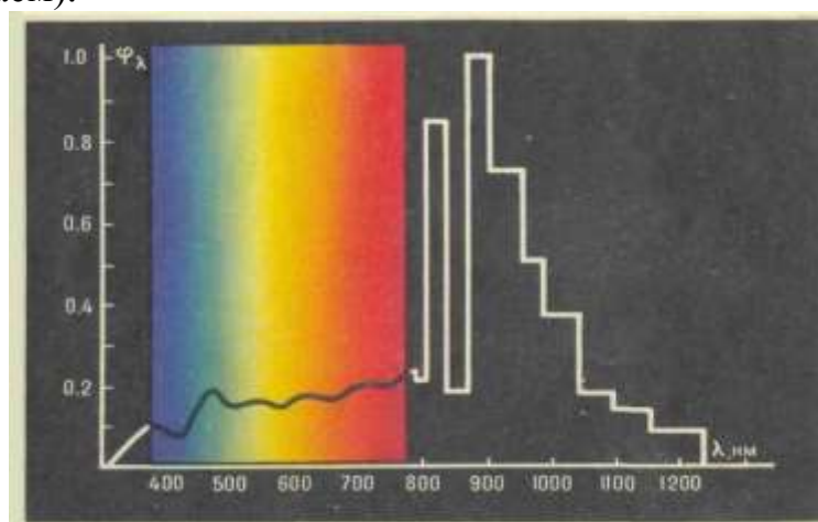
8.10.1-расм. Лампанинг спектр зичлиги.
