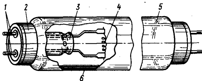
7.1-расм. Люминесцент лампанинг тузилиши.
