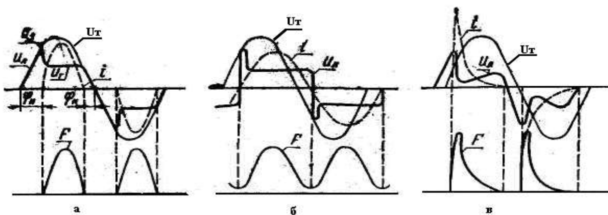
6.5-расм. Газразряд лампанинг кучланиш, ток ва ёруғлик оқимининг бир лахзали қийматларини осциллограммаси:
