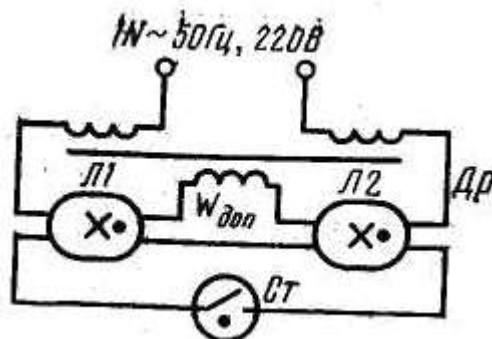
7.8-расм. Люминесцент лампаларини кетма-кет улаш схемаси.
