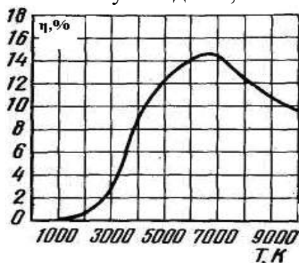
5.2 - расм. Ёруғлик фойдали иш коэффициенти ҳароратга боғлиқлиги.
