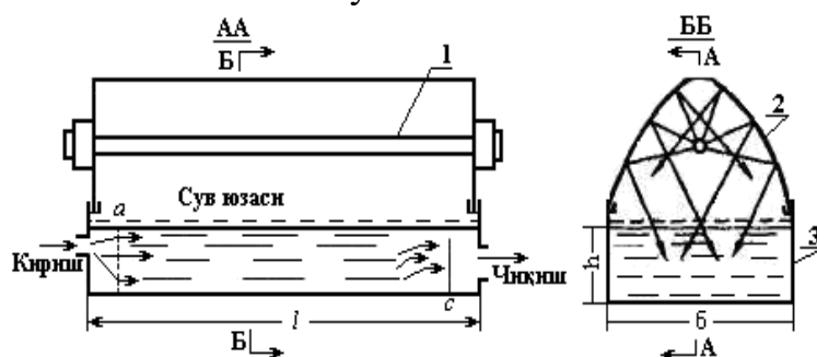
13.12-расм. Сувни ташқарида УБ нурлари билан зарарсизлантириш
