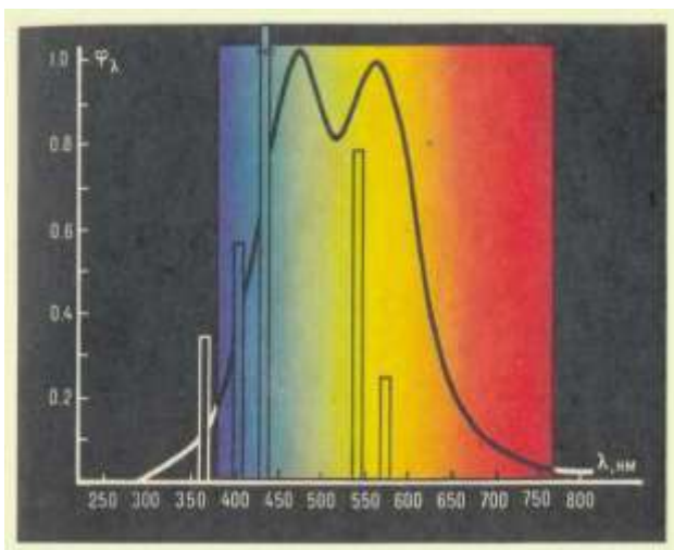
7.4.1 - расм. ЛД лампаси нурланишининг спектр зичлиги.
