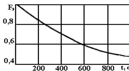
13.10-расм. Эритем лампаларининг нурланиш оқимини ёниш давомийлигига боғликлиги.
