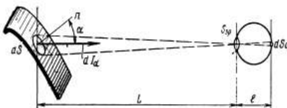
3.4-расм. Юзани равшанлигини аниқлаш.
