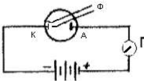
4.4-рasm. Ташқи самарали фотоэлемент:
