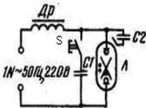
9.2-расм. ДРТ лампасини электр тармоғига улаш схемаси.
