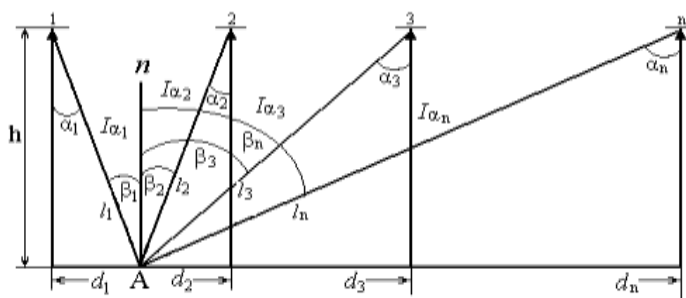
11.2-расм. Шартли ёритилганликни хисоблаш.
