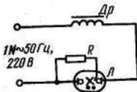
8.2-расм.ДРЛ лампасининг улаш схемаси.
