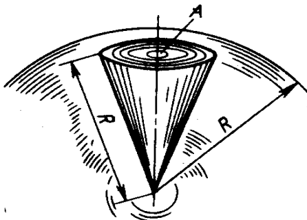
3.2 - расм Фазовий бурчак.
