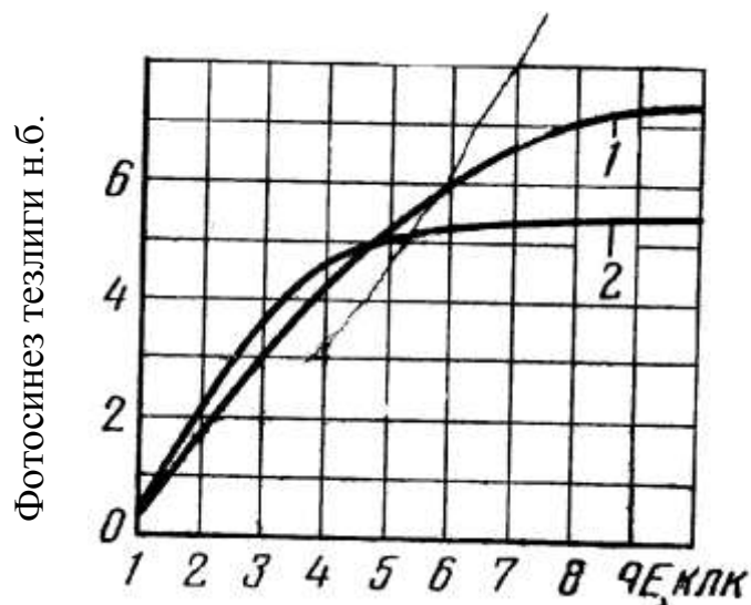
2.2-расм. Фотосинтез жараёнинг ёруғлик эгри чизиқлари:
