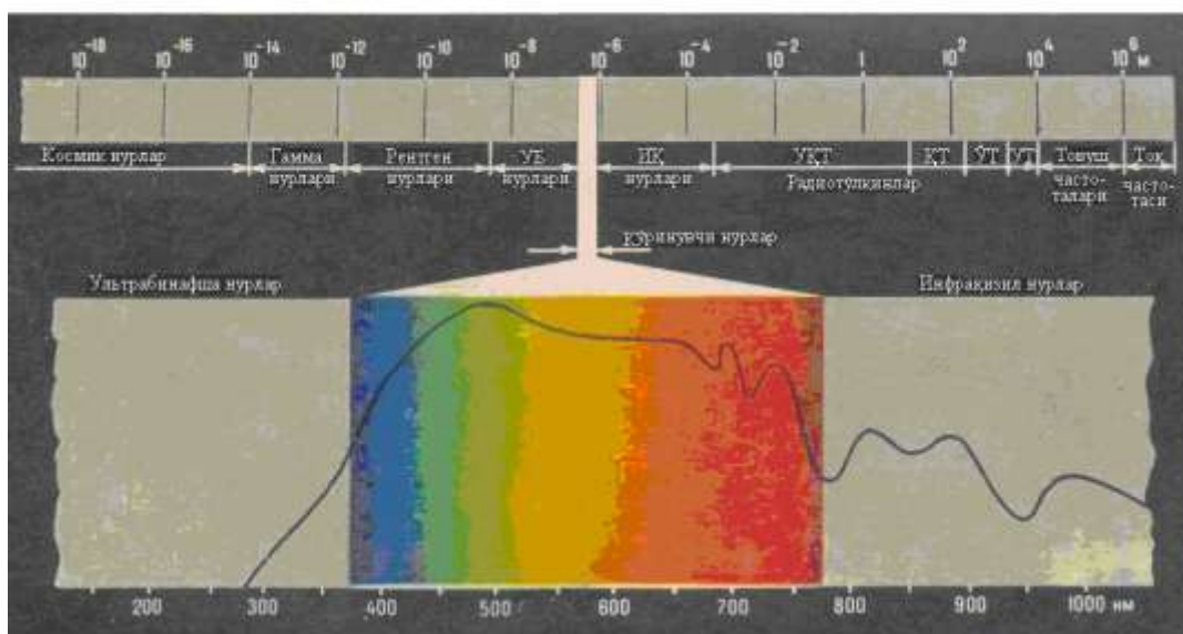
1.1-расм. Электромагнит тўлқинларининг умумий спектри.
