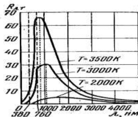
5.1-расм. Абсолют қора жисмнинг ҳар хил ҳароратлардаги нурланиш оқимининг спектр зичликлари.
