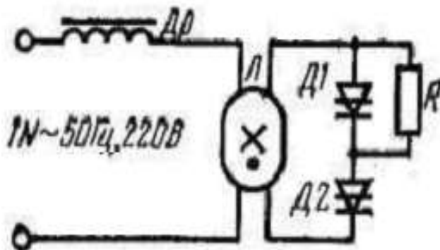
7.9-расм. Люминесцент лампани динистор орқали улаш схемаси. Бу схемада стартер ўрнига D_1 ва D_2 динисторлар ишлатилган.
