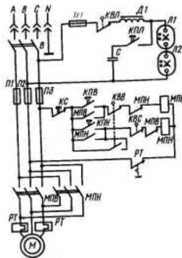
13.5-расм. УОК-1 курилмасининг принципиал электр схемаси.
