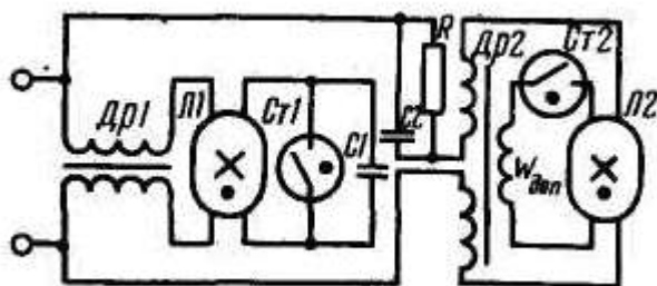
7.5-расм. Люминесцент лампани «фазалари бўлинган» схема билан улаш.
