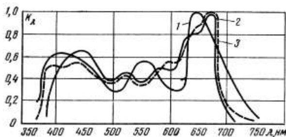
4.10-расм. Фитофотометрларнинг нисбий спектрал сезгирлиги:
