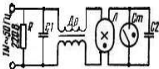
7.2-расм. Люминесцент лампани стартер орқали ўлаш схемаси:
