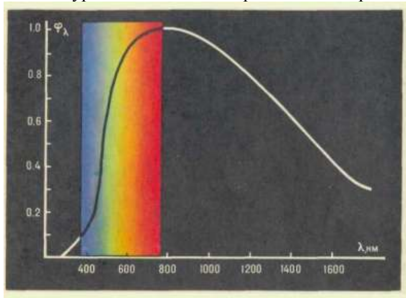
5.4-расм. КГ220-1000 лампаси нурланишининг спектр зичлиги.
