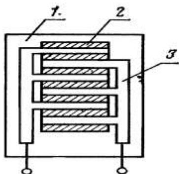
4.6-расм Фоторезисторнинг тузилиши:
