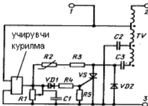
8.6-расм.ИЁҚ принцинал схемаси.
