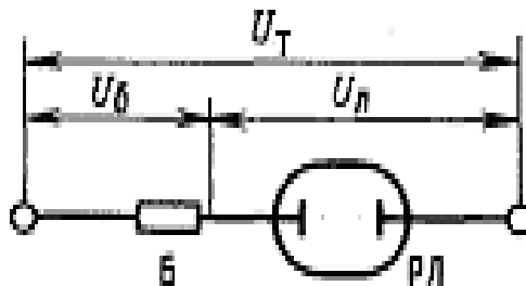
6.2-расм. Газразряд лампани тармоқка улашнинг принцинал электр схемаси.
