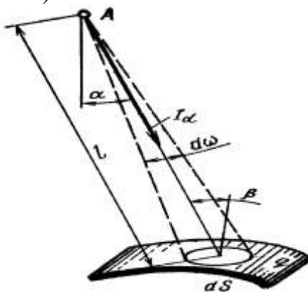
3.3-расм. Ёритилганлик ва ёруғлик кучи орасидаги боғлиқликни аниқлаш.
