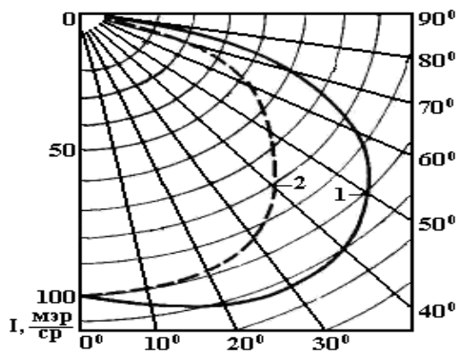
10.7-расм. ЭО 1-30 нурлатгичи УБ нурланиш фазовий зичлигининг нисбий тарқалиши: 1-кўндаланг текисликда; 2-бўйлама текисликда.
