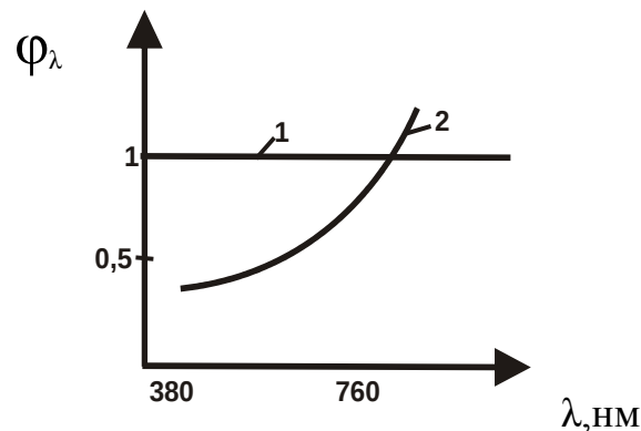
3.1-расм. Қуёш (1) ва чўғланма лампаларнинг (2) нурланиш спектр зичликлари.
