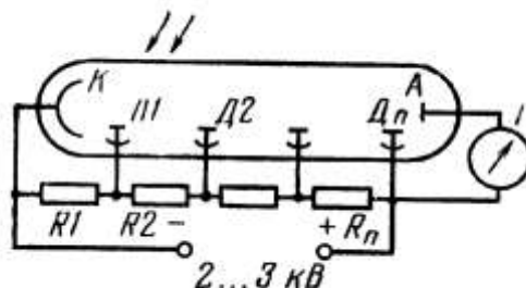
4.5-рasm. Фотоэлектрон кўпайтиргичлар:
