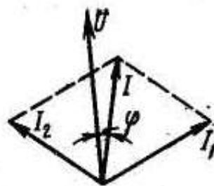
7.6-расм. Лампани «фазаси бўлинган» схема билан улангандаги токларнинг вектор диаграммаси.
