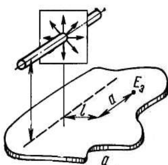
13.1-расм. Стационар нурлатиш қурилмаларини ҳисоблашга оид: а- ҳисобланаётган нукта координатасини аниқлаш; б-чизикли нурланиш манбаи тагидаги тенг нурланишлар эгри чизиклари.
