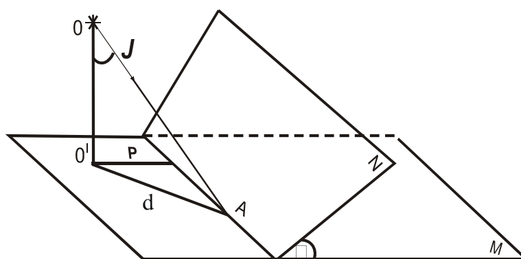
14.4-расм. Оғишган текисликдаги ёритилганликни ҳисоблаш.
