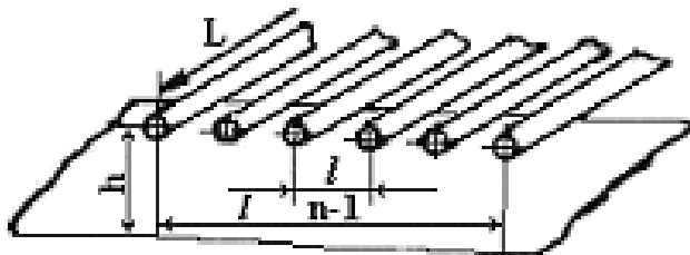
12-4-расм. Люминесцент лампалар блокларни стеллаш юзасида яратилган нурланишини ҳисоблашга доир.
