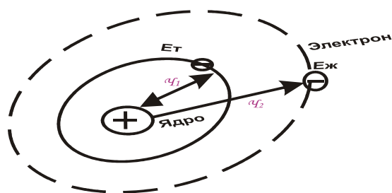
1.2-расм. Водород атомини тузилиши
