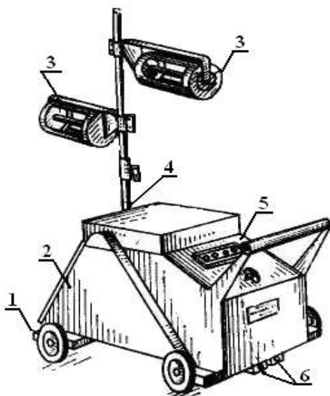
13.4-расм. УОК-1 товукларни нурлатиш учун курилма:
