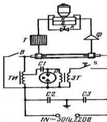
8.10-расм. Лампани принципиал ёқиш схемаси ва уни совутиш системаси.
