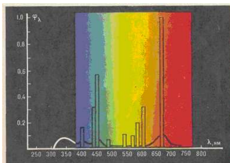
9.1.4-расм. ДРФ 1000 лампанинг нурланиш спектр зичлиги.
