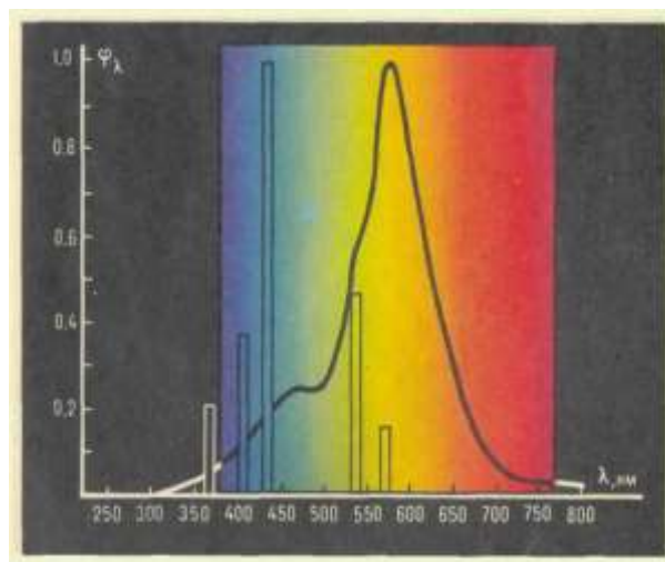
7.4.2 - расм. ЛБ лампаси нурланишининг спектр зичлиги
