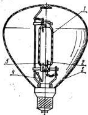
9.4-расм. ДРФ 1000 лампанинг тузилиши:
