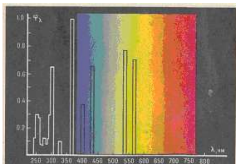
9.3.1-расмда. ДРТ лампаларининг нурланишини спектр зичлиги.
