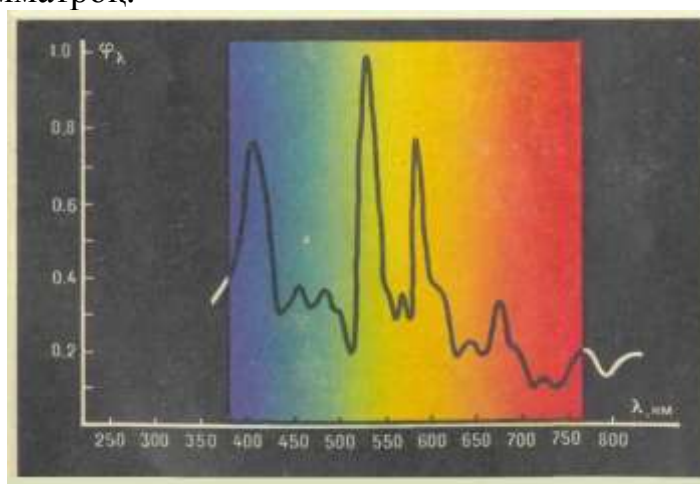
8.7.1-расм. ДРИ лампасининг спектр зичлиги.
