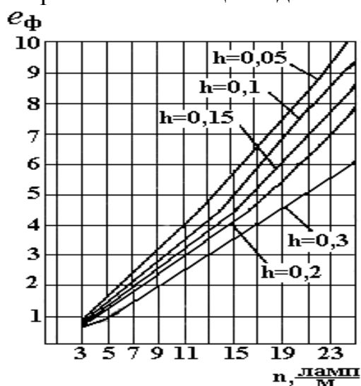
12.5-расм. Нисбий нурлатилганликни блокдаги лампалар сонига ва уларни нурлатилаётган юзага нисбатан жойлашиш баландлигига боғлиқлиги.
