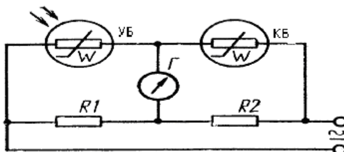
4.2-расмда болометрни улашни кўптрисмон схемаси:
