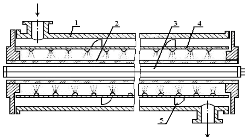
13.13-расм. Сувни ультрабинафша нурлари билан зарарсизлантириш учун ОВУ-6П қурилмаси секциясининг кесими:
