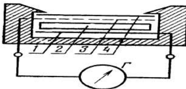
4.8-расм. Винтель фотоэлементининг тузилиши:
