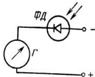
4.7-расм. Фотодиоднинг улаш схемаси:
