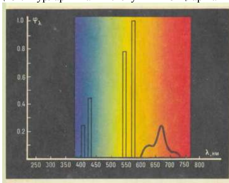
8.3-расм. ДРЛ лампасини нурланиш спектри.
