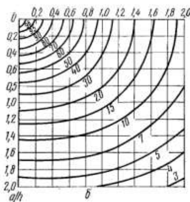
13.1-расм. Стационар нурлатиш қурилмаларини ҳисоблашга оид: а- ҳисобланаётган нукта координатасини аниқлаш; б-чизикли нурланиш манбаи тагидаги тенг нурланишлар эгри чизиклари.
