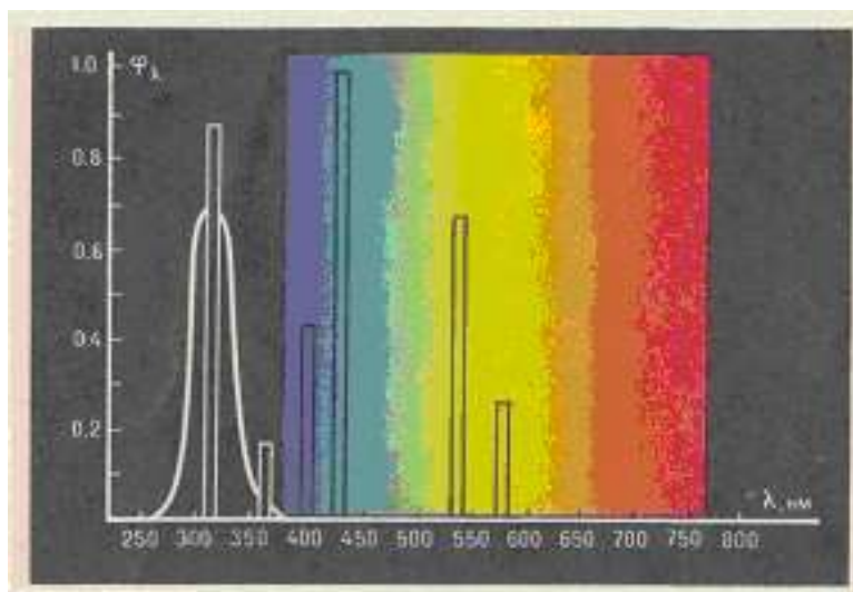
9.0-расм. ЛЭР-40 лампасининг спектр зичлиги.
