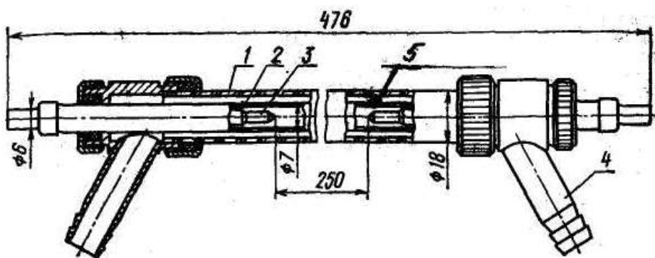
8.9-расм. ДКсТВ6000 лампанинг тузилиши:
