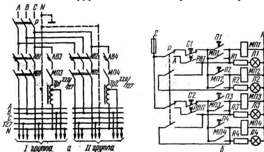
13.23-расм. ИКУФ-1 нурлатиш қурилмасининг принципаал электр схемаси: а-қурилманинг куч қисми схемаси; б-бошқариш схемаси.
