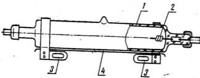
9.1-расм. ДРТ лампасини тузилиши:
