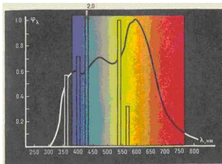
9.3.2-расм. ЛФ 40-2 фотолампасини спектр нурларини зичлиги.
