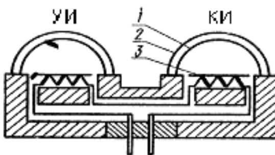
4.3-расм. Термоэлектрик истеъмолчи:
