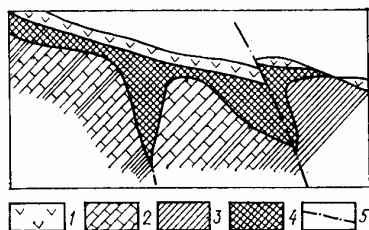
Рис. 5.4. Схематический геологический разрез месторождения Монте-Амиата (по В.И. Смирнову и др.): 1 – трахиты четвертичного возраста; 2–3 – меловые породы: 2 – известняки; 3 – сланцы; 4 – рудное тело (оруденные брекчии); 5 – разломы
