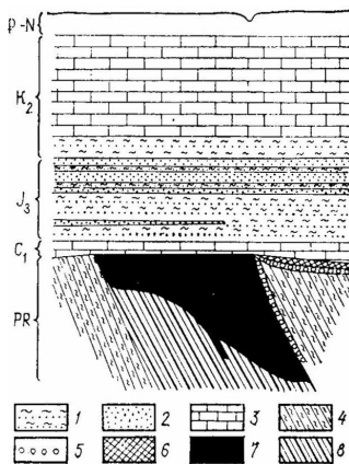
Рис. 12.3. Геологический разрез Яковлевского месторождения КМА (по Я.С. Чайкину): 1 – суглинки, пески, глины; 2 – песчаники; 3 – мел, мергели, известняки; 4 – гнейсы, кварцево-сланцевые сланцы; 5 – бокситы; 6 – 7 – руды: 6 – перекристаллизованные, 7 – богатые; 8 – железистые кварциты
