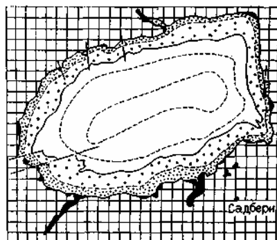
Рис. 3.4. Схема геологического строения лополита Садбери в Канаде (по П. Колеману): 1 – подстилающие породы; 2 – габбро; 3 – нориты; 4 – породы кровли; 5 – сульфидные месторождения; 6 – разрывные тектонические нарушения
