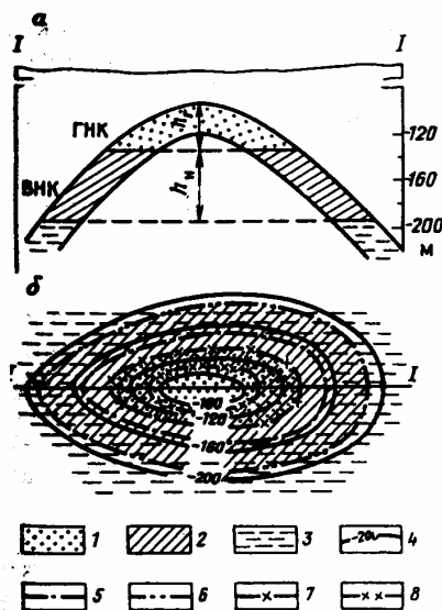
Рис. 15.3. Принципиальная схема сводовой залежи:
