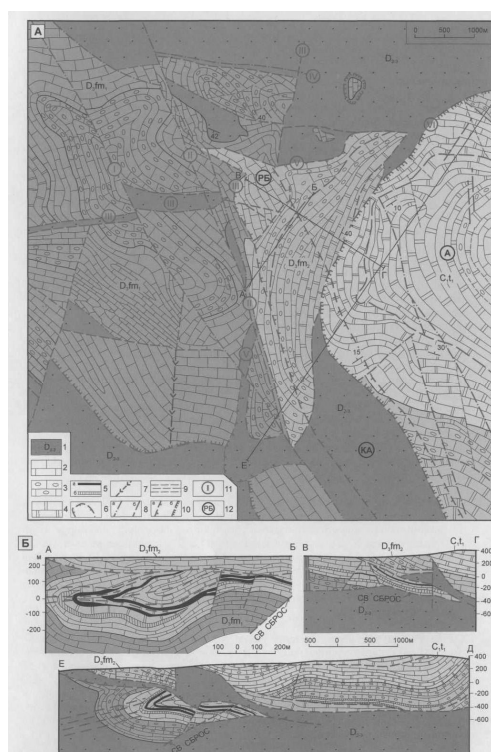
Рис. 12.16. Геологическая карта (А) и разрезы (Б) месторождения Шалкия:
