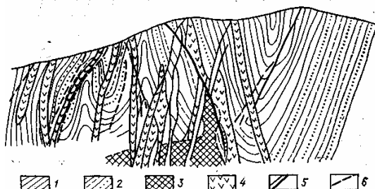
Рис. 12.13. Геологический разрез Хрустального месторождения (по Ф.И. Вольфсону и А.В. Дружинину): 1–алевролиты; 2–переслаивание песчаников и алевролитов; 3–биотитизированные породы; 4–дайки; 5–6 – рудные жилы: 5–касситерит-сульфидные; 6–сульфидные
