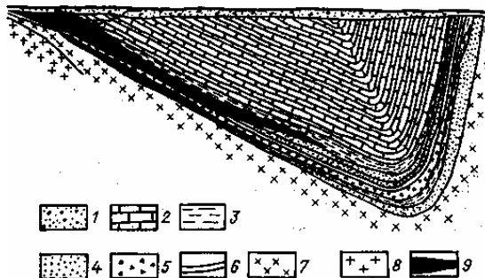
Рис. 12.10. Геологический разрез через синклиналь Нчанга: 1 – слой обломочного кварца и поверхностные отложения; 2 – аргиллиты и доломиты; 3 – полосчатые сланцы; 4 – полевошпатовые кварциты; 5 – полосчатые песчаники; 6 – кварциты и кремнистые сланцы; 7 – аркозы; 8 – граниты; 9 – рудные тела
