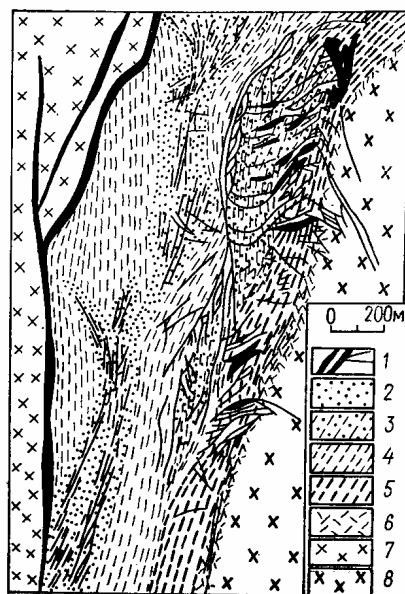
Рис. 5.2. Схема геологического строения медно-порфирового месторождения Чукикамата (по В. Лопесу и В. Перри): 1 – рудные жилы и прожилки; 2–6 – измененные палеогеновые монцититовые порфиры: 2 – окварцованные, 3 – серицитизированные и слабоокварцованные, 4 – интенсивно серицитизированные, 5 – альбитизированные и серицитизированные, 6 – хлоритизированные и альбитизированные; 7–8 – гранодиориты: 7 – палеогеновые, 8 – юрские
