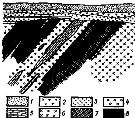
Рис. 12.1. Геологический разрез Сарбайского месторождения (по И.А. Кочергину и В.А. Адамчуку): 1 – пески, сланцеватые глины; 2 – опока; 3 – кварцевые пески и песчаники; 4 – скарны; 5 – ороговикованные карбонатные породы; 6 – порфиры; 7–8 – руды: 7 – скарновые, 8 – магнетитовые
