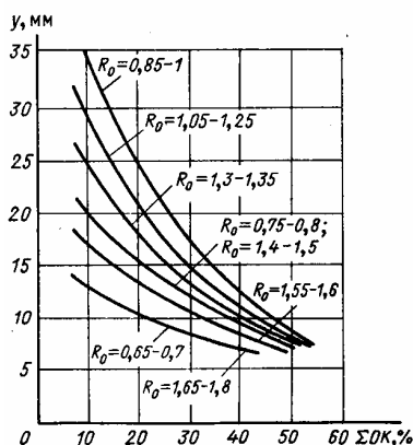
Рис. 14.1. Изменение толщины пластического слоя в зависимости от содержания отощающих компонентов ( \Sigma OK = I_f + 2/3Sv ) в углях различных стадий метаморфизма
