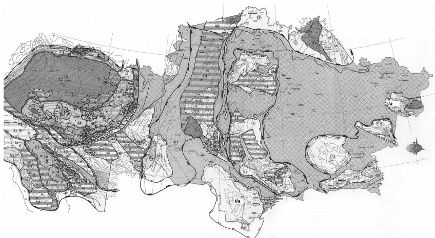
Рис. 15.7. Карта прогноза нефтегазоносности Казахстана (Э.С. Воцалевский и др., 2000). Нефтегазоносные провинции (НГП):
