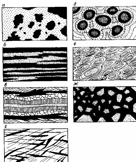
Рис. 1.5. Типы текстур полезных ископаемых (по В.И. Смирнову):
