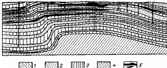
Рис. 9.1. Геологический разрез месторождения Жезказган (по К.И. Сатпаеву): 1 – красноцветная толща нижней перми; 2–4 – каменноугольные образования: 2 – рудоносные серые песчаники, 3 – безрудные красноцветные песчаники и аргиллиты, 4 – песчаники и известняки; 5 – рудные тела
