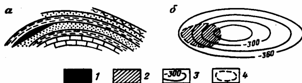
Рис. 15.4. Принципиальная схема нефтяной залежи с наклонным водонефтяным контактом: a —геологический разрез; б —структурная карта;
