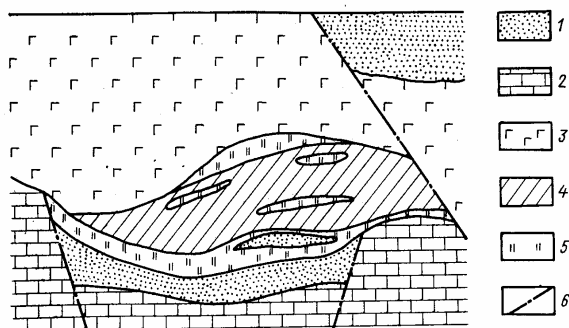
Рис. 12.6. Геологический разрез Талнахского месторождения (по В.Н. Котляру): 1–песчаники; 2–известняки и ангидриты; 3–дифференцированные габбродиориты с вкрапленным оруденением в нижней части; 4–залежь сплошных сульфидных руд; 5–экзоконтактовые вкрапления руды в измененных вмещающих породах; 6–разрывные нарушения
