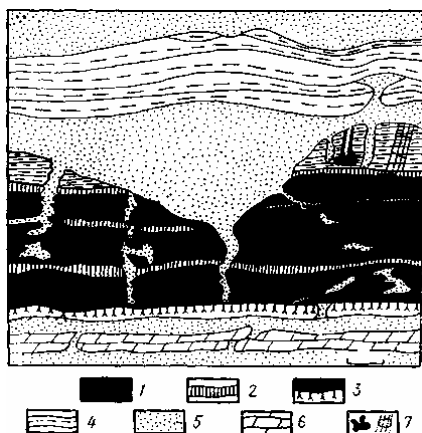
Рис. 14.7. Сводная схема взаимоотношения кластических жил и даек с вмещающими породами и угольными пластами Интинского месторождения Печорского бассейна (по А.Г. Дмитриеву):
