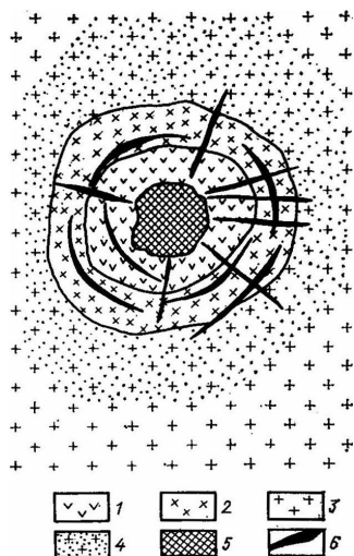
Рис. 3.2. Схема геологического строения карбонатитового месторождения: 1 – щелочные породы; 2 – ультраосновные породы; 3 – гнейсы; 4 – метасоматически измененные сланцы; 5–6 – карбонатиты: 5 – штоки; 6 – жилы (дайки)
