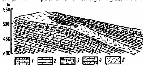
Рис. 13.6. Схематический геологический разрез участка Айдагского месторождения (по А.И. Кулиеву): 1–4 – известняки: 1–2 – кампан-маастрихтские (1 – плитчатые светло-серые, 2 – серые песчаные), 3 – верхнесантонские белые, 4 – с туфогенным материалом; 5 – белые цеолитизированные туфы (собственно Айдагский пласт)
