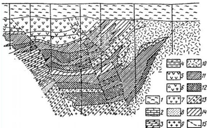
Рис. 12.2. Геологический разрез Качарского месторождения (по
