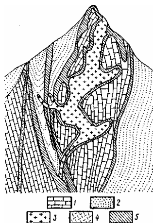
Рис. 6.2. Геологический разрез месторождения Тырныауз (по В.И. Смирнову):
