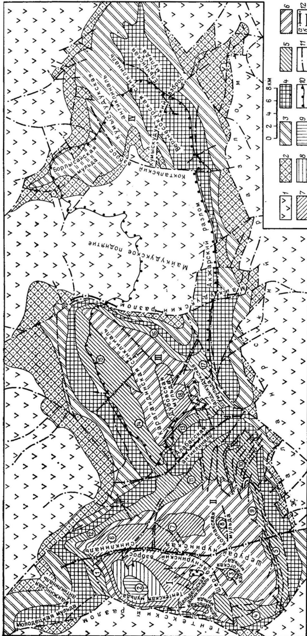
Рис. 14.16. Схематическая геологическая карта Карагандинского бассейна: 1 – дофаменские образования; 2 – фаменский и турнейский ярусы; 3–9 – угленосная толща карбона: 3 – аккулдукская свита ( C_{1,ak} ), 4 – ашляйская свита ( C_{1,as} ), 5 – карагандинская свита ( C_{1,sg} ), 6 – надкарагандинская свита ( C_{2ndk} ), 7 – долинская свита ( C_{2dl} ), 8 – тентекская свита ( C_{2m} ), 9 – шаханская свита ( C_{3sh} ); 10 – контур распространения юрских отложений; 11 – разрывные нарушения; 12 – границы угленосных районов (а) и участков (б). I–IV – геолого-промышленные районы: I – Тентекский, II – Шерубайнуринский, III – Карагандинский, IV – Верхнесокурский. Цифрами в кружках обозначены угленосные участки: 1 – Манжинский, 2 – Тентекский, 3 – Карагогский, 4 – Сасыкольский, 5 – Тазанмвский, 6 – Каражаро-Шаханский, 7 – Долинский, 8 – Колпакский, 9 – Кишинекольский, 10 – Южный, 11 – Центральный, 12 – Северный, 13 – Алабасский, 14 – Саранский, 15 – Промышленный.
