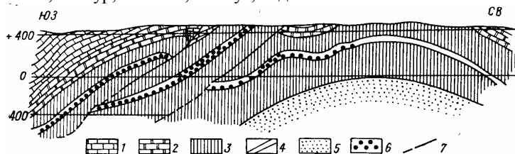
Рис. 12.15. Схематический геологический разрез месторождения Миргалимсай (по материалам Миргалимсайской ГРП ): 1 – известняки ( C_1 ); 2 – доломиты ( C_1 ); 3 – брекчированные известняки ( D_3fm ); 4 – рудоносный горизонт в толще D_3fm ; 5 – аркозовые песчаники ( D_3fr ); 6 – послойные залежи прожилково-вкрапленных барито-свинцовых руд; 7 – разрывные нарушения
