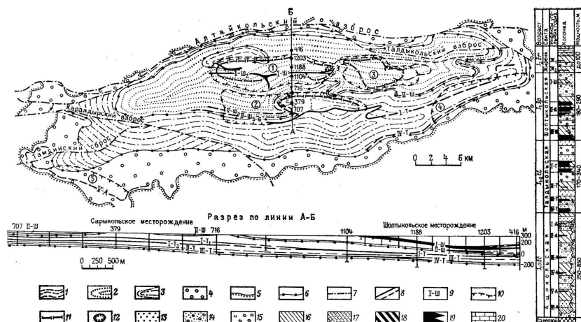
Рис. 14.19. Схематическая геологическая карта Майкюбенского бурогоугольного бассейна. Свиты: 1-жиренкольская ( J_2\dot{z}r ), 2-шоптыкольская ( J_2\dot{s}p ), 3-талдыкольская ( J_{1-2}tl ), 4-ащикольская ( J_1a\dot{s}c ); 5-граница распространения юрских отложений; 6-границы угленосных свит; 7-разрывные нарушения; 8-выходы угольных пластов, установленные и предполагаемые; 9-индексы угольных пластов; 10-границы угольных месторождений с запасами, пригодными для открытых работ; 11-изолинии предельного коэффициента вскрыши ( 10 \text{ м}^3/\text{т} ); 12-действующий карьер; 13-песчаники; 14-гравелиты; 15-конгломераты; 16-аргиллиты; 17-алевролиты; 18-углистые аргиллиты; 19-уголь; 20-известняки. Цифры в кружках - месторождения: 1-Шоптыкольское; 2-Сарыкольское; 3-Талдыкольское; 4-Таскудукское; 5-Тамдинское
