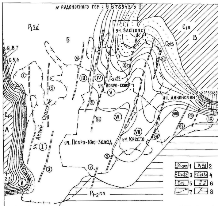
Рис. 12.11. Геолого-промышленная схема Жезказганского месторождения (по материалам Жезказганской ГРЭ). Структуры первого порядка:
