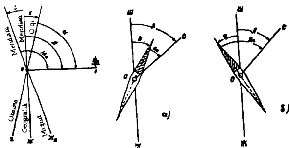
23- rasm. Direksion va azimut (a) hamda rumb (b) burchaklar.
