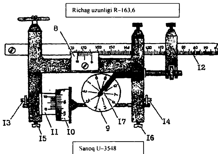
37-rasm. Sanoq olish mexanizmining tuzilishi.
