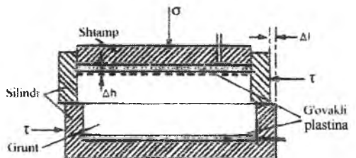
49-rasm. Gruntlarning surilishga qarshiligi- ni aniqlovchi asbobning ishchi qismi.
