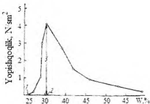
25-rasm. Grunt yopishqoqligining namlikka bog'liqlik grafi: 1 – boshlang'ich yopishqoqlikdagi namlik; 2 – maksimal yopishqoqlikdagi namlik; 3 – gruntlarni maksimal yopishqoqligi.
