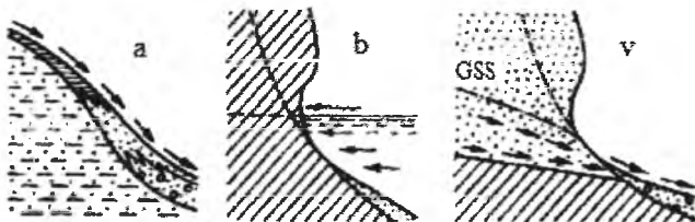
37-rasm. Gruntlarning yuvilishi: a – yuza; b – to'liqli; v – suffoziyli.
