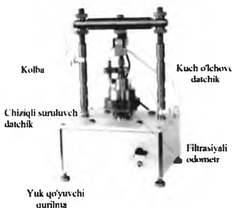
45-rasm. Kompresiya asbobi.
