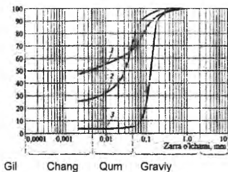
10-rasm. Zarralar tarkibining yeg'indisini egri ko'rinishidagi (komulyativ) grafikli tasviri: 1 – gil; 2 – changli suglinok; 3 – qum.
