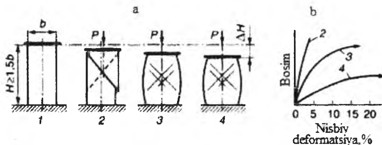
55-rasm. Bir o'qli siqilishda gruntning deformatsiyasi tavsifi: a – namunasining tashqi ko'rinishi: 1 – siqilishdan avval va (2-4)-keyin, 2 – mo'rt buzilish, 3 – yarim mo'rt buzilish, 4 – plastik buzilish; b – “bosim-deformatsiya” diagrammasi.
