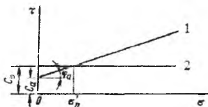
53-rasm. Har xil sinov sxemalari-dagi nam shimgan gilli gruntlarning surilish grafiqi: 1 – konsolidatsiyalashgan-drenajlanmagan sinov; 2 – konsolidatsiyalanmagan-drenajlanmagan sinov.
