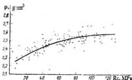
63-rasm. Qumtosh va alevrolitlarning mustahkamlik va zichligi orasidagi o'zaro bog'liqlik.
