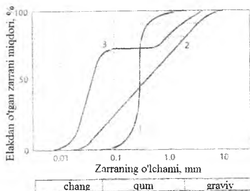
6-rasm. Donalarga ajratilgan yotqizilarning turlari. 1 – yaxshi tasniflangan; 2 – bir jinsli tasniflangan; 3 – uchta oraliqda tasniflangan.
