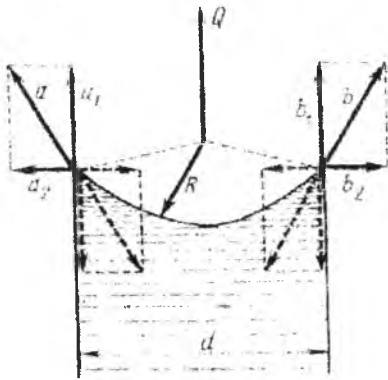
32-rasm. Kapillyar kuchlarining ta'sir chizmasi: a va b – suv va kapillyar devori orasidagi molekullarning o'zaro ta'sir kuchi; d – kapillyar diametri; R – menisk egrisi radiusi.
