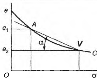
47-rasm. Kompressiya ko'r-satkichlarini hisoblashga oid chizma.
