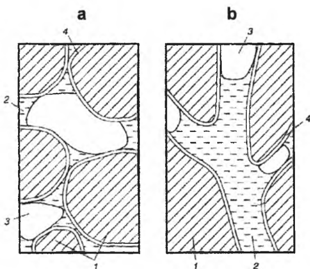
14-rasm. Gruntidagi kapillyar suvning holati: a – kapillyar-kondensirlashgan suv; b – xususiy kapillyar suv; 1 – mineral; 2 – kapillyar suv; 3 – havo; 4 – adsorblashgan suv.
