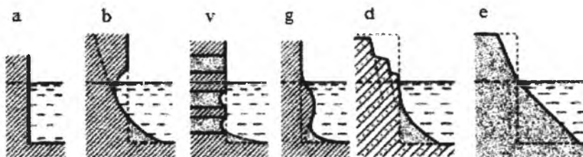
36-rasm. Har xil gruntli kovlanmaning bo'kish tavsifi: a – bo'kmaydigan grunt; b – bo'kadigan grunda oqish va ag'darmaning hosil bo'lishi; v – qatlamli massivda gruntlarning tanlanib bo'kishi; g – ko'pchish bilan bo'kish; d – lyosslarning bo'kishi, cho'kishi va oqishi; e – qumlarning bo'kishi va oqishi.
