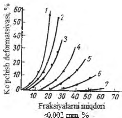
29-rasm. Har xil mineral tarkibli gillning ko'pchish deformatsiyasini undagi gil fraksiyalari miqdoriga bog'liqligi: 1 – bentonit; 2 – bentonit va illit; 3 – kaolinit va bentonit; 4 – illit va bentonit; 5 – illit; 6 – illit va kaolinit; 7 – kaolinit.
