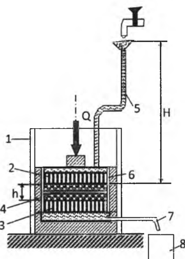
39-rasm. Kompressiya-filtratsiyali asbobning ishlash chizmasi: 1 – korpus; 2 – yuqori g'ovakli shtamp; 3 – ostki g'ovakli shtamp; 4 – grunt namunasi; 5 – pyezometrik trubka; 6 – ishchi halqa; 7 – oqizuvchi; 8 – bo'sh idish; Q – siquvchi kuch.
