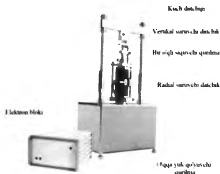
54-rasm. Gruntlarni bir o'qli siqish bilan sinovchi asbob.
