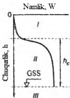
33-asm. Aeratsiya hududida kapillyar kaymaning hosil bo'lishi: I – mustahkam bog'langan suvning hududi; II – kapillyar kayma hududi; III – grunt suvlari; GSS – grunt suvining sathi.
