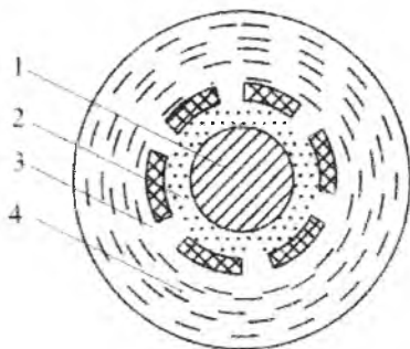
67-rasm. Globulyar agregat-ing tuzilish sxemasi – lyossimon gruntlarning asosiy strukturali ele-menti: 1 – kvarts; 2 – amorfi gel SiO 2 ; 3 – CaCO 3 ; 4 – gilli zarralar + Fe 2 O 3 + amorf SiO 2 + CaCO 3 + kvarts.
