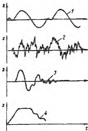
59-rasm. Har xil mashina va mexanizmlarning ishlashida tebranish amplitudasining vaqt davomida o'zgarish turlari: 1 – davriy; 2 – xaotik; 3 – so'nuvchi; 4 – davriy bo'lmagan-uriluvchi.
