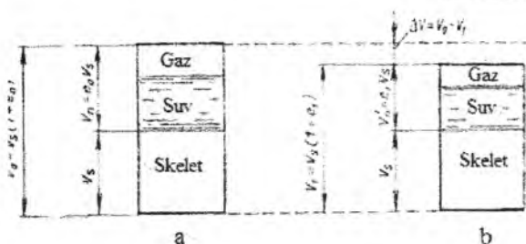
46-rasm. Kopressiya davomida grunt hajmi o'zgarishi: a – boshlang'ich holati; b – kompressiyadan so'ng. V_n – g'ovaklik hajmi, V_s – grunt skeletining hajmi, e – g'ovaklik koeffitsiyenti.
