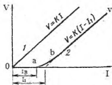
40-rasm. Filtratsiya tezligining bosim gradiyentiga bog'liqlik grafigi: 1 – qumli, 2 – gilli gruntlar uchun.
