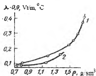
41-rasm. Issiqlik o'tkazuvchanlik koeffitsiyentining skeiet zichligiga bog'liqlik graffi: 1 – qumli, 2 – sug'linokli gruntlar uchun.
