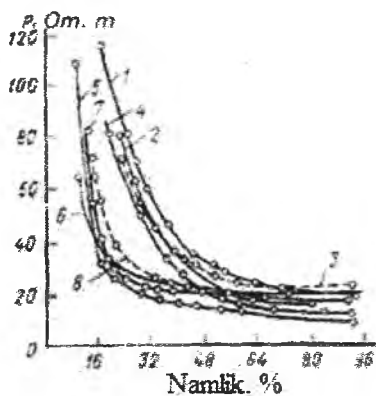
42-rasm. Solishtirma elektr qarshilikning namlikka bog'liqlik grafigi: 1-4 – nozik dispers va 5-8 – yirik dispers gruntlar.
