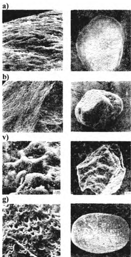
8-rasm. Har xil genetik turdagi qum zarralarining mikrorelyefi shakli va tavsifi: a – eolli, b – allyuvial, v – dengizli, g – dengiz-eolli stallokimyo xususiyati bilan morfologiyasi o'rtasida juda yaqin bog'lanish mavjud bo'lishi kuzatiladi.
