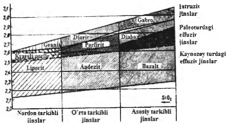
62-rasm. Magmatik tog' jinslari zichligining o'zgarish chegarasi.
