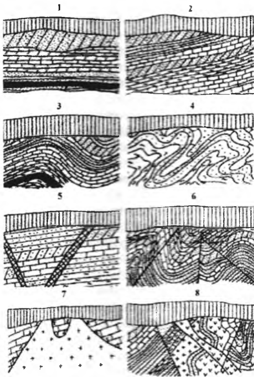
70-rasm. Grunt massivining asosiy tektonik tuzilishi: 1 – gruntlari gorizontal yotgan; 2 – gruntlari monoklinal yotgan; 3 – oddiy buramali tuzilish; 4 – murakkab buramali tuzilish; 5 – uzilgan dislokatsiyali monoklinal yotish; 6 – uzilgan dislokatsiyali murakkab buramali tuzilish; 7 – o'zgargan gruntlar tutash joyidagi oreolli yirik magmatik intruzi; 8 – intrudirlangan magmatik jismi murakkab buramali tuzilish.
