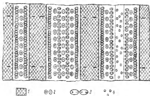
15-rasm. Grunt kapillyarlarida suvning tarqalish chizmasi: 1 – kapillyarlar devori; 2 – ionlar (kation va anionlar); 3 – bog'langan suvning molekulas; 4 – kapillyar suvlar.
