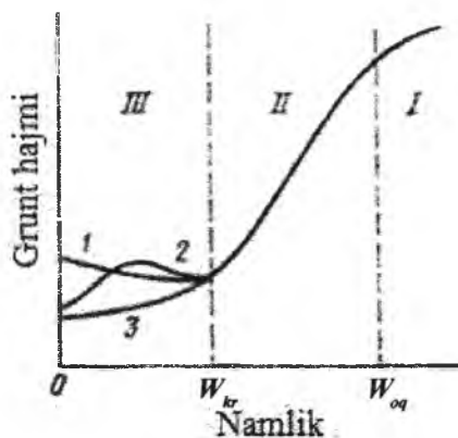
31-rasm. Kirishishda gilli suv shimgan gruntning hajmini o'zgarishi: I – sekinlashgan kirishish bosqichi; II – normal kirishish bosqichi; III – qoldikli kirishish bosqichi; 1, 2 va 3 – qoldiq kirishishning har xil turlari; W_{kr} – kirishish chegarasidagi namlik; W_{oq} – oquvchanlik chegarasidagi namlik.
