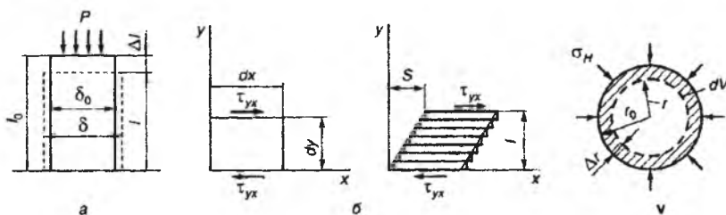
43-rasm. Bir o'qli siqilishda (a), surilishda (b) va har taraflama siqilishda (v) jismlarning deformatsiyasi.
