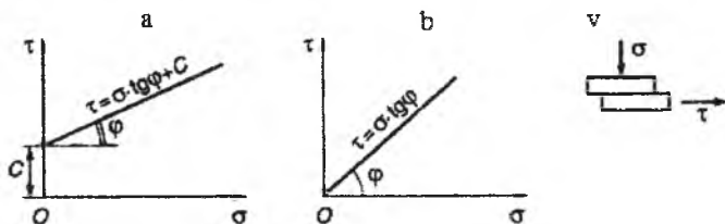
50-rasm. Bog'langan (a), bog'lanmagan (b) gruntlarning surilishga qarshiligining normal bosimga bog'liqligi va sinov chizmasi (v).
