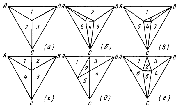
Рис 196 Возможные расположения квазибинарных сечений при наличии одной ( a ) и двух ( b и в ) тройных промежуточных фаз и при сочетаниях одной двойной и одной тройной промежуточной фазы ( г ), двух двойных и одной тройной промежуточной фазы ( д ), одной двойной и двух тройных промежуточных фаз ( е )
