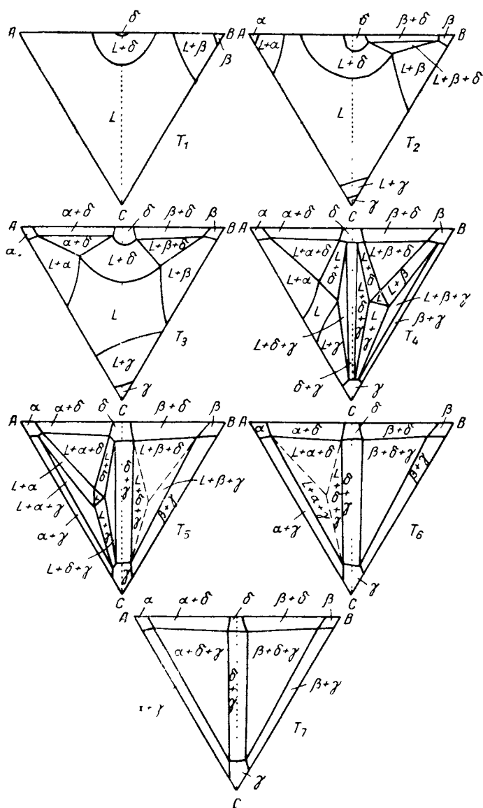
Рис. 187 Изоثرмы пространственной диаграммы, приведенной на рис 185
