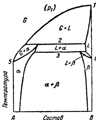
Рис. 260. Сечение TX при t_1 , полученное из PT -диаграммы на рис. 258
