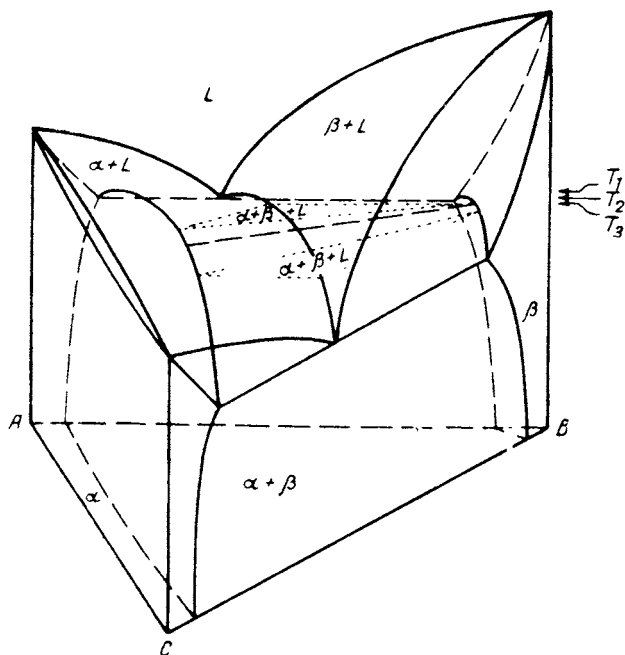
Рис. 144 Трехфазная область сходится в коду при температуре максимума
