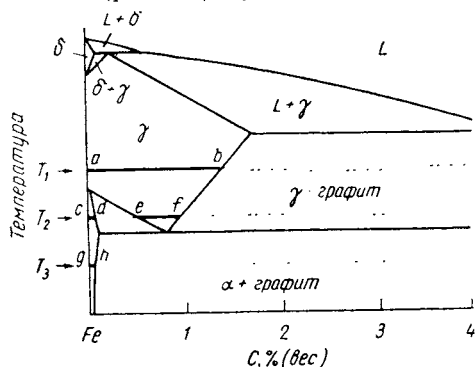
Рис. 57. Диаграмма равновесия стабильной системы Fe—C:
