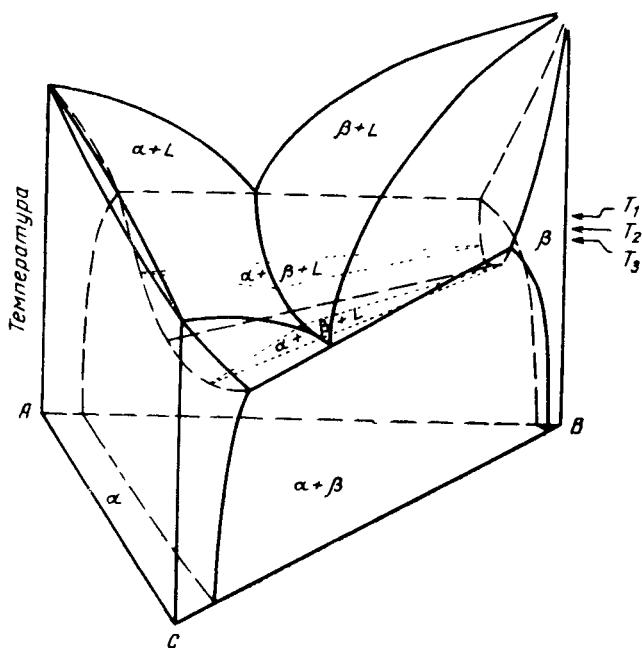
Рис 146 Трехфазная область сходится в коноду при температуре минимума
