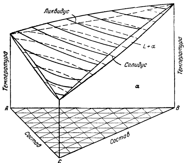
Рис. 101. Пространственная диаграмма: температура—состав тройной изоморфной системы
