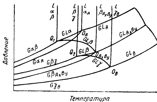
Рис. 262. PT -диаграмма системы с полностью конгруентной промежуточной фазой AxBy
