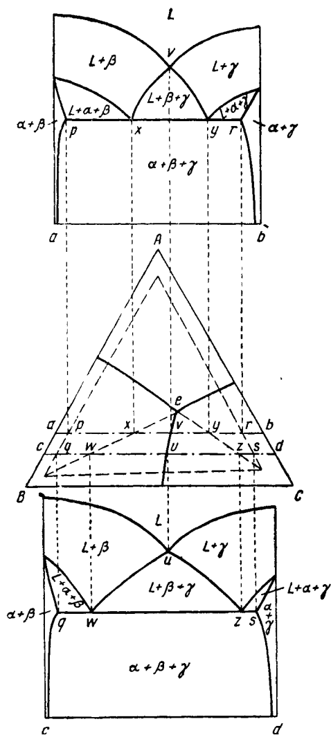
Рис. 277. Модификация рис. 276; построение при помощи двух изоплет без каких-либо допущений относительно растворимости в твердом состоянии
