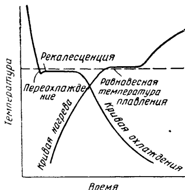
Рис. 270. Реальные кривые охлаждения и нагрева чистого металла
