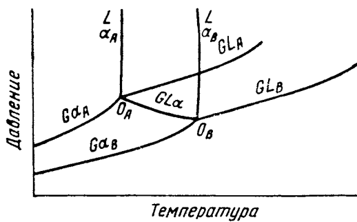
Рис 240 РТ -диаграмма изоморфной двойной системы на рис 1
