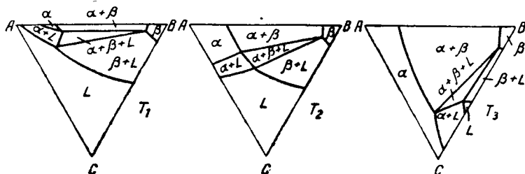
Рис. 135. Изотермы пространственной диаграммы на рис. 133
