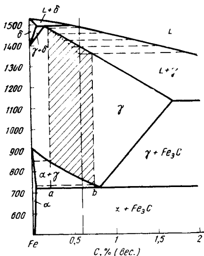
Рис. 95. Диаграмма равновесия метастабильной системы Fe—C. Заштрихована зона концентраций в ликвированном сплаве с 0,6% С непосредственно после окончания затвердевания перед эвтектондным превращением
