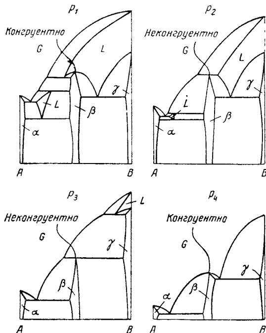
Рис. 265. Сечение температура-концентрация, полученные из РТ-диаграммы на рис. 264
