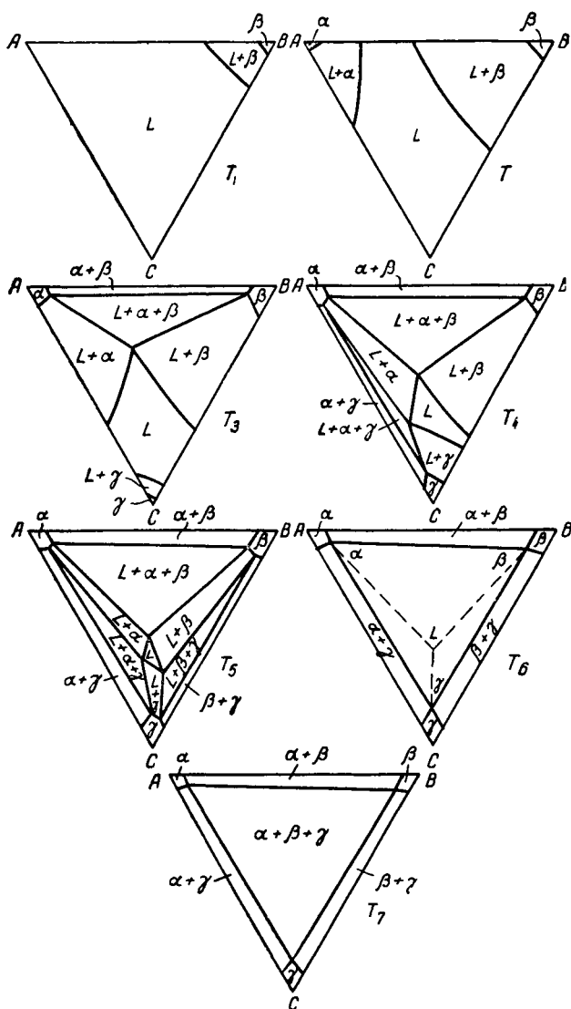
Рис 155. Изоثرмы пространственной диаграммы, приведенной на рис 153
