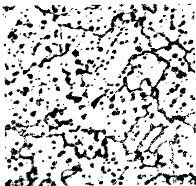
Рис. 63. Домонотектический сплав \text{Cu}+5\% \text{Pb} в литом состоянии
