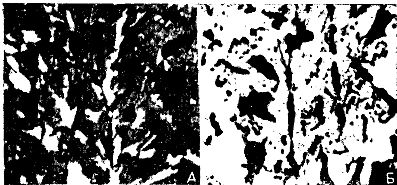
Рис. 233 Микроструктура четверной эвтектики в системе Bi—Pb—Sn—Cd, состоящей из следующих четырех фаз: висмута (светлая матрица, лучше всего видна на Б); свинец (мелкие, темные, извилистые частички, придающие серый цвет матрице на А); олово (большие белые массы, лучше всего заметные на А), кадмий (большие черные частицы). Увеличение: А — \times 100 ; Б — \times 500
