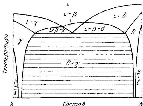
Рис 189 Вертикальное сечение пространственной диаграммы, приведенной на рис 188
