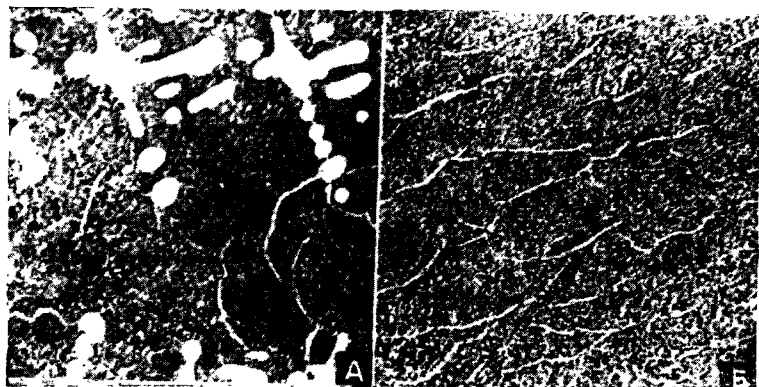
Рис 38 Эвтектический сплав Al-Si, модифицированный натрием ×100:
