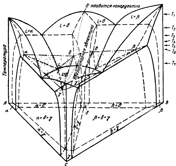
Рис. 185 Диаграмма температура — состав тройной системы с квазибинарным вертикальным сечением между компонентом C и конгруэнтно плавящейся \delta -фазой
