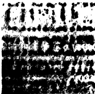
Рис. 32. «Стерлинговое серебро» (7,5% Cu) в литом состоянии.
