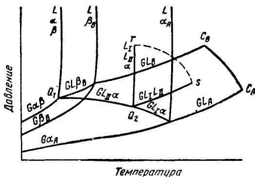
Рис. 257. PT -диаграмма системы с двойным моноотектическим равновесием при Q_2
