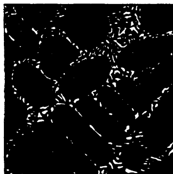
Рис 124 Схема процесса затвердевания сплава 90% Pb+5% Bi+5% Sb, обозначенного точкой X на рис. 126 (а—д схемы, рисунки, е — микроструктура при комнатной температуре). \times 100
