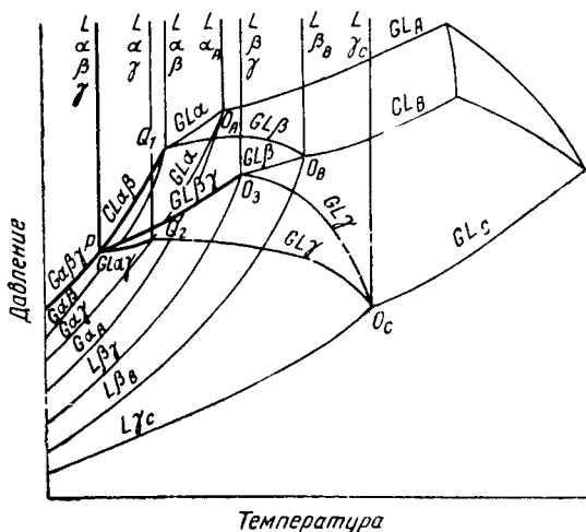
Рис. 266. PT -диаграмма тройной эвтектической системы класса I
