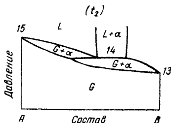
Рис. 248. Сечение PX при t_2 , полученное из PT -диаграммы на рис. 241
