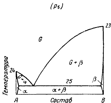
Рис 255. Сечение TX при p_5 , полученное из PT -диаграммы на рис. 249
