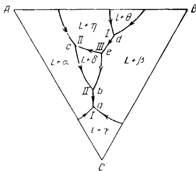
Рис. 204 Проекция поверхностей ликвидус сложной тройной системы
