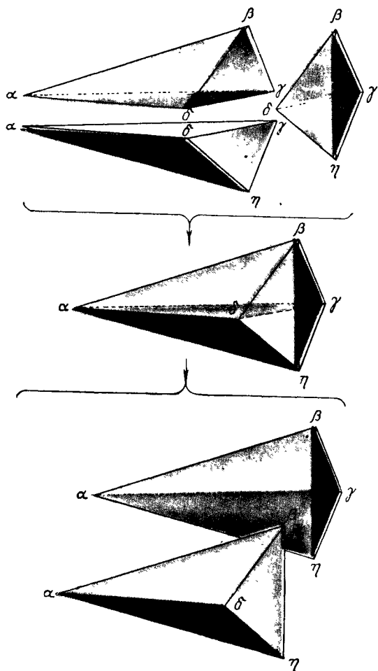
Рис. 215 Схема пятифазного равновесия II класса Геометрически обратная картина даст равновесие III класса
