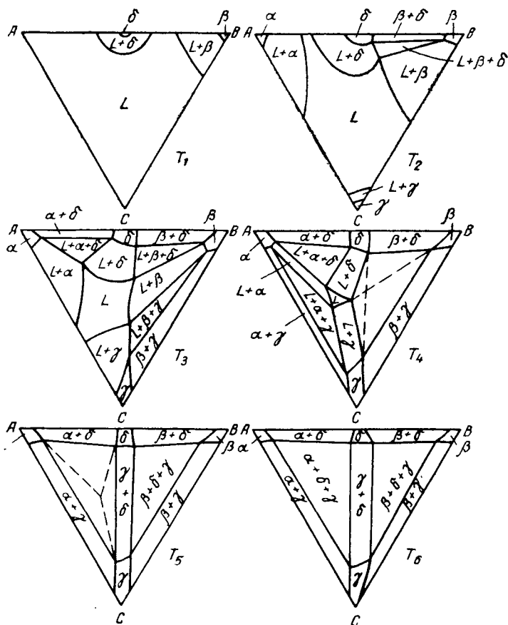
Рис. 191 Изотермы пространственной диаграммы, приведенной на рис. 188
