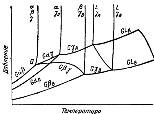
Рис. 256. PT -диаграмма системы с двойным эвтектондным равновесием при Q
