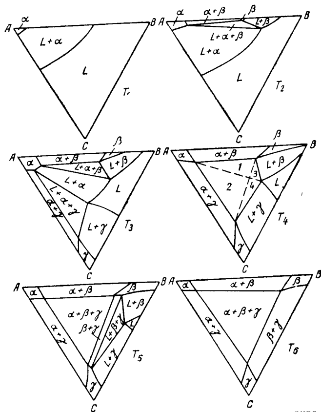
Рис. 169. Изотермы пространственной диаграммы, приведенной на рис 167
