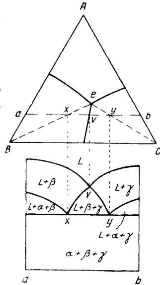
Рис. 276. Определение состава тройной эвтектики путем определения одного вертикального сечения и в предположении нерастворимости в твердом состоянии
