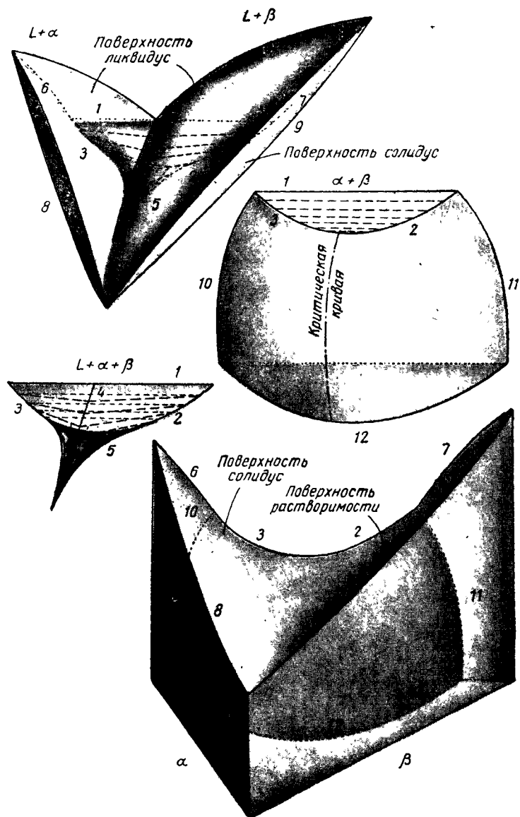
Рис. 137. Разъемная модель диаграммы на рис. 136
