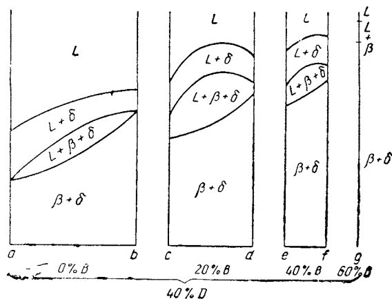
Рис. 229. Изоплеты четверной диаграммы равновесия на рис. 226
