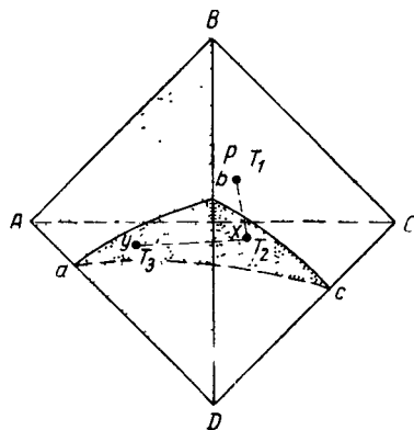
Рис. 227 Проекция ликвидус четверной диаграммы на рис. 226
