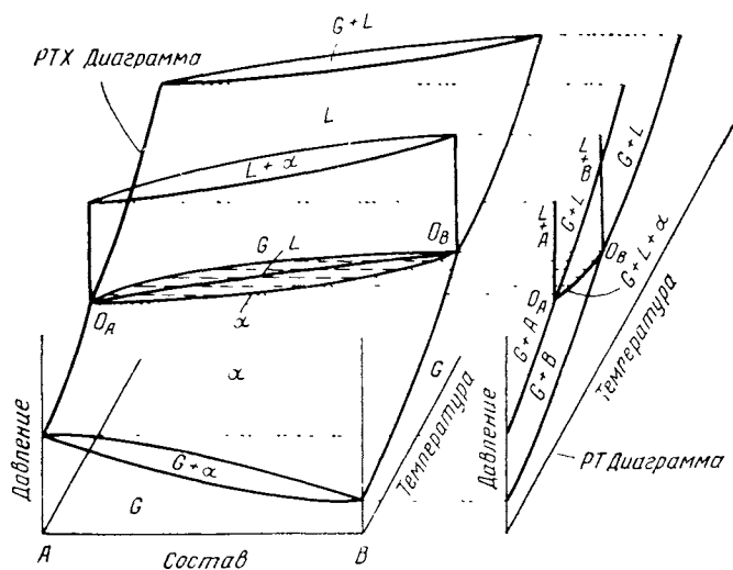
Рис 239 Диаграмма РТХ изоморфной двойной системы показывающая, как получается РТ -диаграмма при проецировании всех одновариантных и безвариантных равновесий на плоскость РТ
