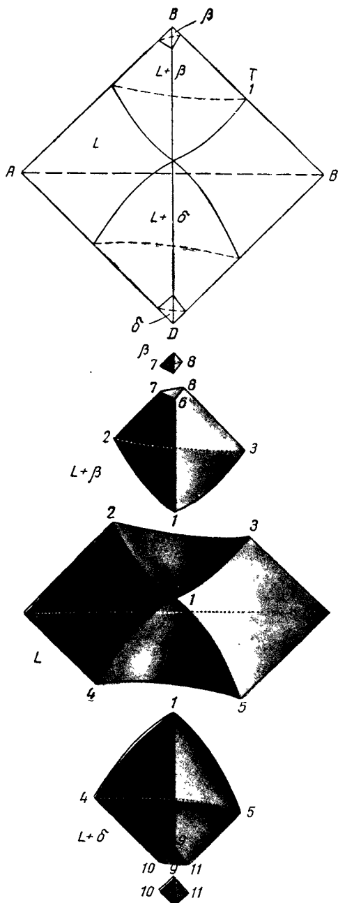
Рис 226, а Шесть изотерм четверной системы, в которой трех- фазное равновесие L+\beta+\delta с понижением температуры рас- пространяется по диаграмме от двойной эвтектики BD при T_1 до двойной эвтектики AD , лежащей между T_5 и T_6
