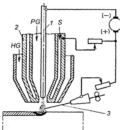
15.7 - rasm. Plazma-kukunli eritib qoplash tok uzatuvchi qo‘shimcha sim bilan:
