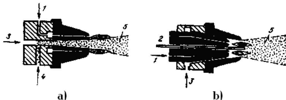
16.2-rasm. Gaz alangasida changlatish sxemasi:
