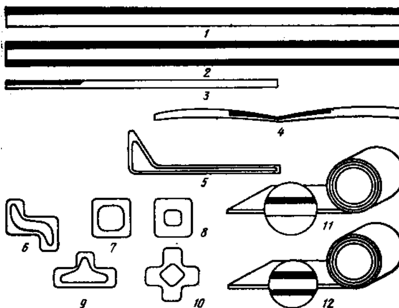
13.5-rasm. Payvand birikmalarning ko'ndalang kesim profillari:
