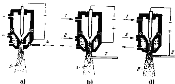
16.4-rasm. Plazmali changlatish sxemasi:
