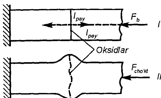
10.5-rasm. Qarshilik bilan uchma-uch payvandlashda birikma hosil bo'lish sxemasi ( F_b – boshlangich kuch; F_{cho'kt} – cho'ktirish kuchi).
