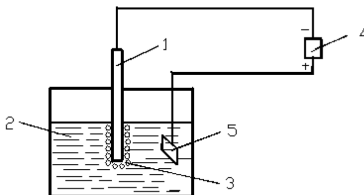
17.6-rasm. Qarshilik bilan kavsharlashning prinsipial sxemasi:
