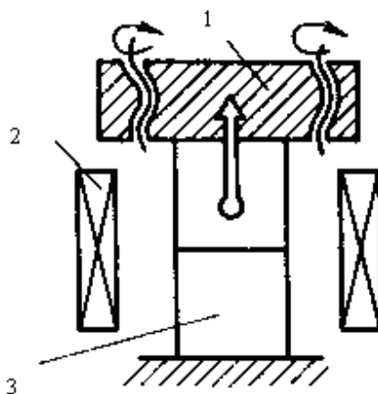
11.5-rasm. Majburiy deformatsiyalash sxemasi bo'yicha diffuzion payvandlash:
