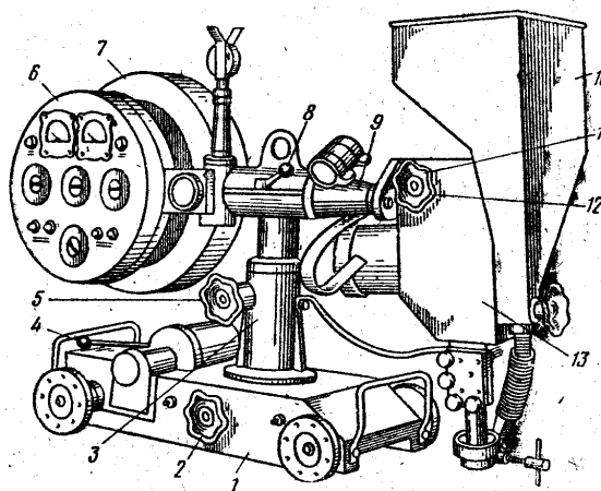
3.3-rasm. Payvandlash traktori:
