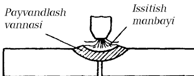
1.3-rasm. Erirtib payvandlash chizmasi.
