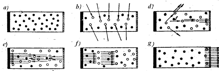
8.2-rasm. Tashqi qoʻzgʻatish taʼsirida rubin kristalida fotonlar sharrasini koʻchkisimon oʻsish sxemasi.
