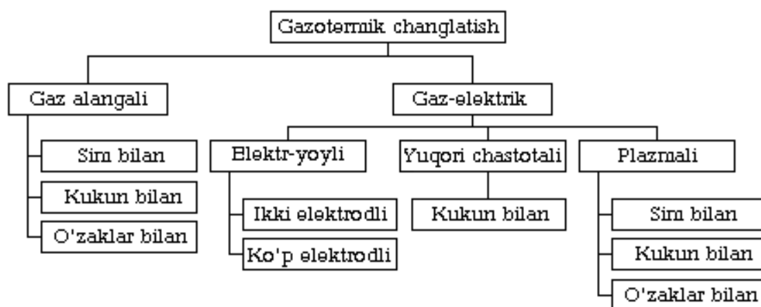
16.1-rasm. Gazotermik changlatish usullarining klassifikatsiyasi.
