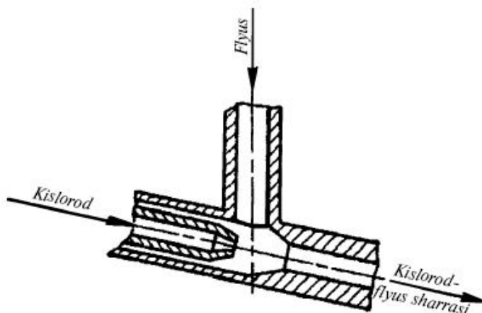
9.5-rasm. Kislorod-flyusli kesish sxemasi.
