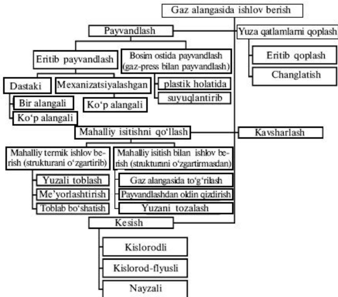
9.1-rasm. Metall va nometall materiallarga gaz alangasida ishlov berish usullarining klassifikatsiyasi.
