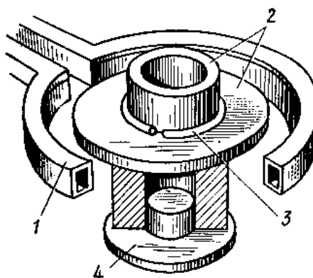
17.5-rasm. Induksion kavsharlashning prinsipial sxemasi:
