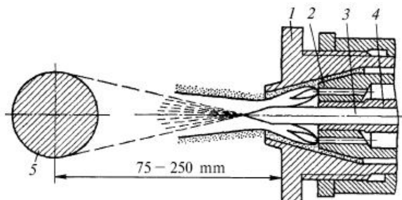
9.7-rasm. Gaz bilan changlatish sxemasi:
