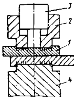
11.3-rasm. Payvandlanayotgan detalni bir tomonli deformatsiyalash bilan sovuq holatda nuqtali payvandlash chizmasi.
