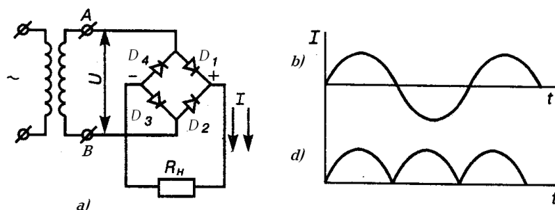
5.5-rasm. Bir fazali ikki yarim davrli ko'priqli to'g'rilash sxemasi:
