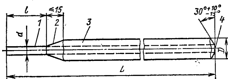
2.3-rasm. Qoplamali elektrod:
