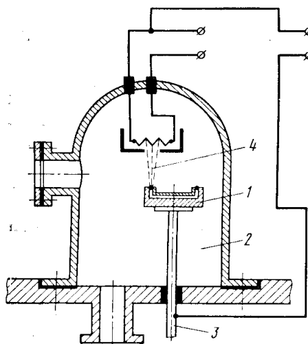
7.1-rasm. Elektron-nurli payvandlash sxemasi:
