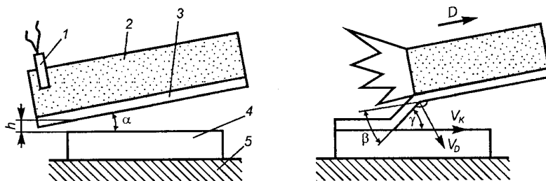
14.1-rasm. Portlatib burchak ostida payvandlash sxemasi:
