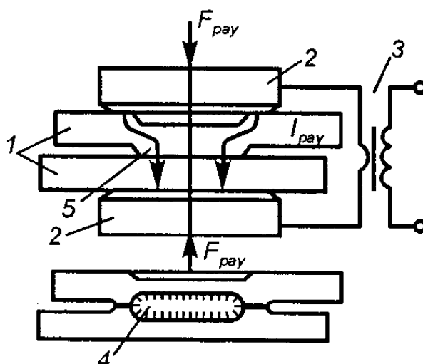
10.3-rasm. Relyefli payvandlash sxemasi:
