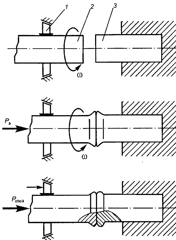
12.2-rasm. Uzluksiz yurg'izib ishqalab payvandlash sxemasi:
