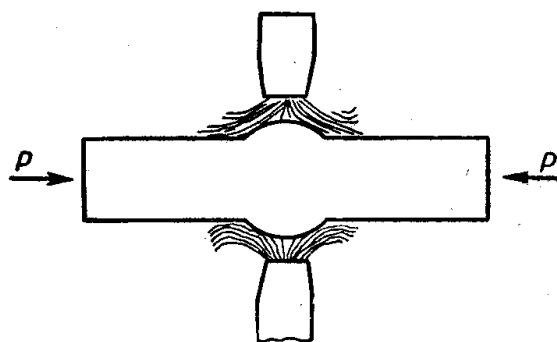
1.4-rasm. Bosim ostida payvandlash chizmasi.
