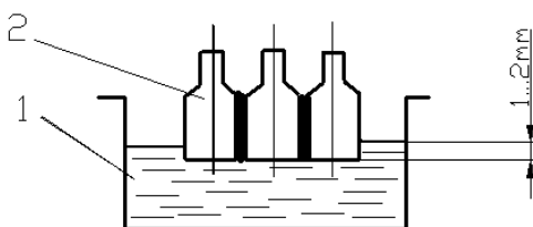
17.7-rasm. Eritilgan kavsharga detalni cho‘ktirib kavsharlash sxemasi:
