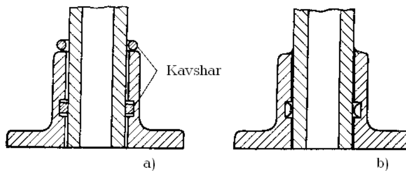
17.2-rasm. Kapillar usulda kavsharlash sxemasi:
