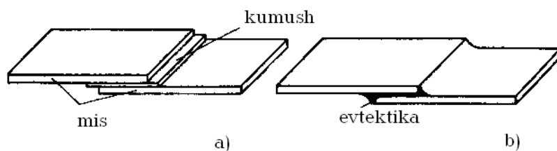
17.3-rasm. Kontaktli reaksiyon kavsharlash sxemasi:
