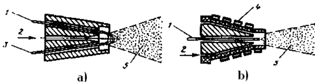
16.3-rasm. Elektr metallizasion changlatishning sxemasi:
