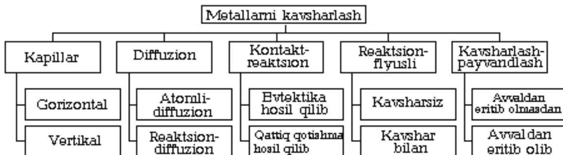
17.1-rasm. Kavsharlash usullarining klassifikatsiyasi.
