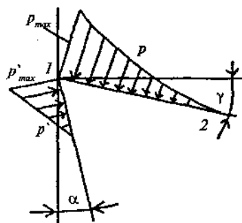
6.1-rasm. Keskich tig'i old va orqa yuzalarida bosimning
