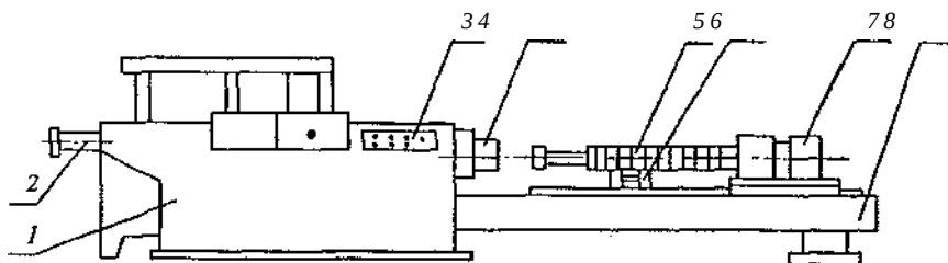
13.6-rasm. 7523 modeli gorizontalsidirish yarim avtomat stanogi: 1-asosiy stanina; 2- gidrosilindr; 3- boshqarish pulti; 4-planshayba; 5-protyajka; 6- rolik; 7- karetka; 8- qoʻshimcha stanina.
