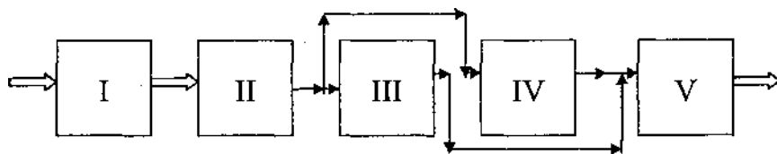
Parallel- ketma-ket ishlov beruvchi siklli avtomatik liniya
