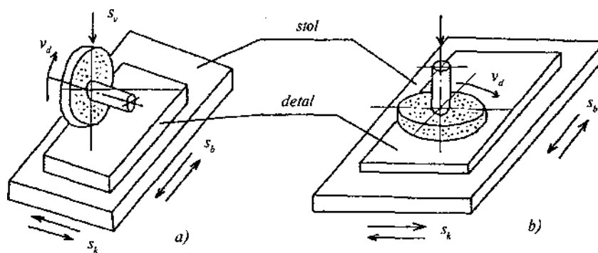
16.11-rasm. Yassi jilvirlash sxemalari.
