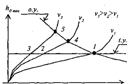
6.8 -rasm. Yedirilish mezonlari. gan qatlam qalinligi H ko'rsatiladi (6.9-rasm).
