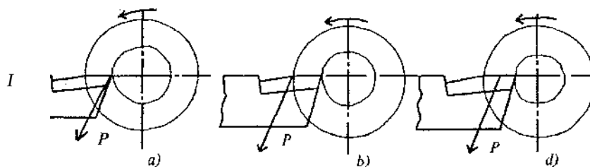
4.2-rasm. Keltirilgan kesish kuchi P ning asosiy kesuvchi tig'ga qo'yilish sxemasi.
