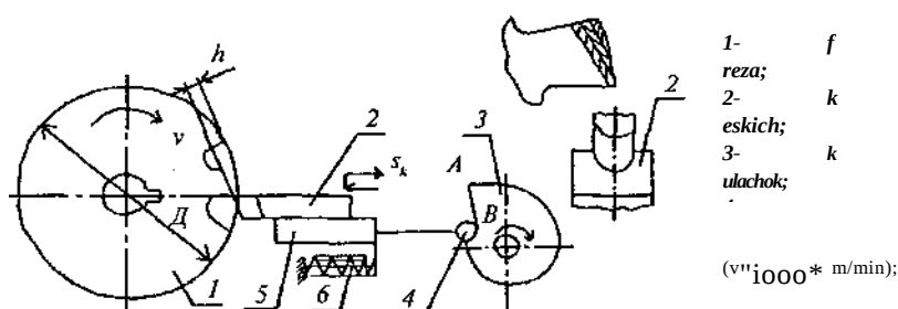
10.1- rasm. Freza orqa yuzasini gardanlash sxemasi.
