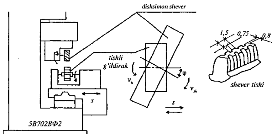
14.16-rasm. Shevinglash stanogi va shevinglash sxemasi.
