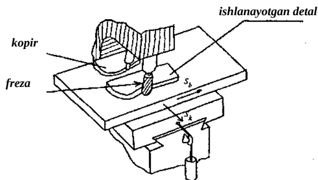
12.8-rasm. Kontur bo'yicha frezalash sxemasi. 109
