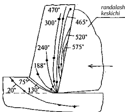
5.7-rasm. Qirindidagi temperatura maydoni.
