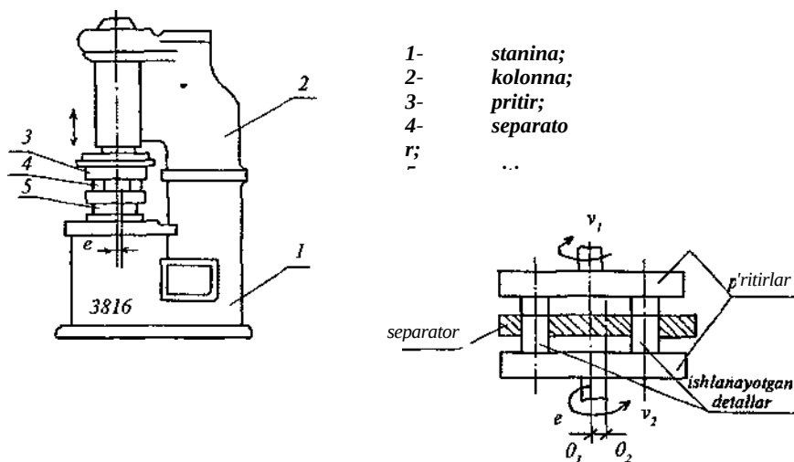
16.15-rasm. Pritirkalash stanogi va pritirka qilish sxemasi.
