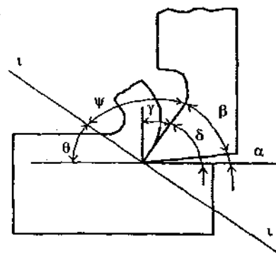
3.2-rasm. Yorilish tekisligi vaziyatini aniqlovchi burchaklar (6, y).
