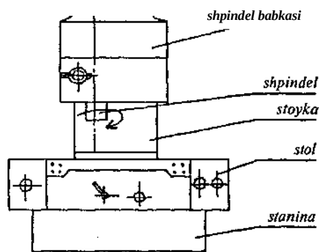
11.6-rasm. Koordinat- teshik kengaytirish stanogi.
