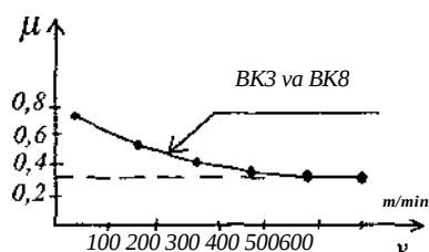
6.2-rasm. Quruq tashqi ishqalanish koeffitsiyenti.
