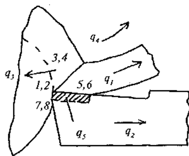
5.3-rasm. Kesish zonasidan materialining yupqa qatlamida issiqlikning chiqib ketish sxemasi. yig'ilib qolishi sabab bo'ladi.
