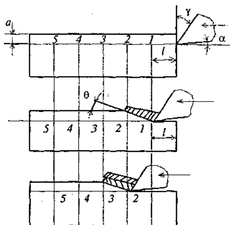
3.1-rasm. Yorilish qirindisining hosil bo'lish sxemasi.
