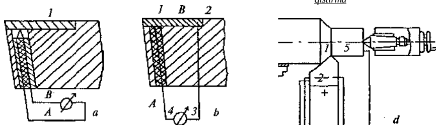
5.5- rasm. Keskichning temperaturasi sun'iy (a), yarim sun'iy (b), va tabiiy (d) termojuftlar yordamida o'lchash.
