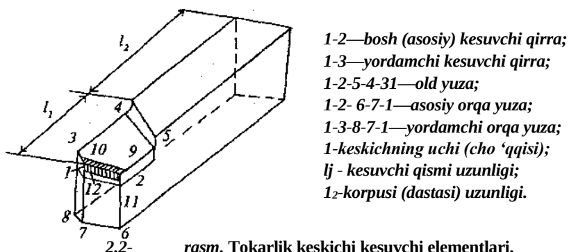
rasm. Tokarlik keskich kesuvchi elementlari.
