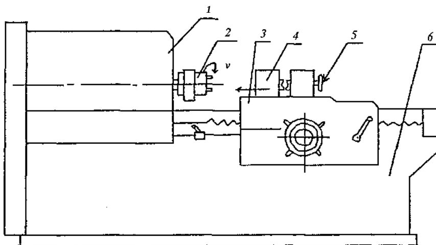
15.6-rasm. Boltlarga rezba ochish stanoklari: 1-tezliklar qutisi; 2-rezba ochish kallagi; 3-support; 4-tiski; 5-maxovik; 6-stanina.
