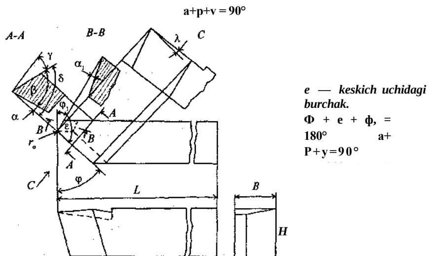
2.6-rasm. Oddiy ko'rinishdagi tokadik keskichining chizmasi.
