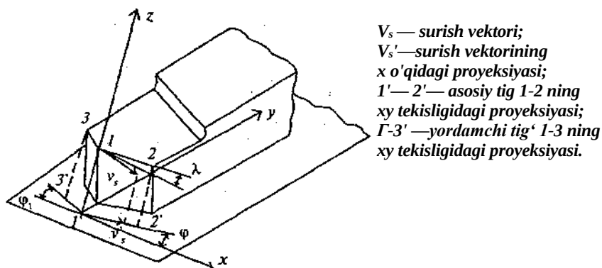
2.3-rasm. Keskich kesuvchi qismining geometrik parametrlari.
