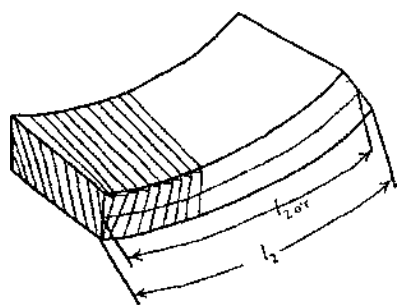
3.7-rasm. Qirindining uzunligini uning kirishuvini hisoblash uchun o'lchash sxemasi.
