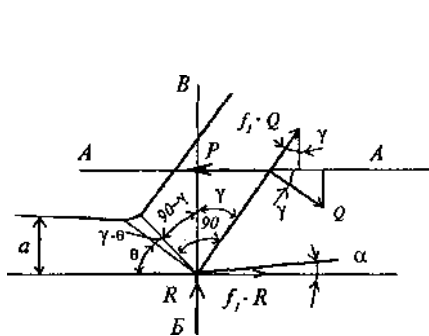
4.5-rasm. Qirindi hosil qilishdagi 4.4- deformatsiya va buzilishga
