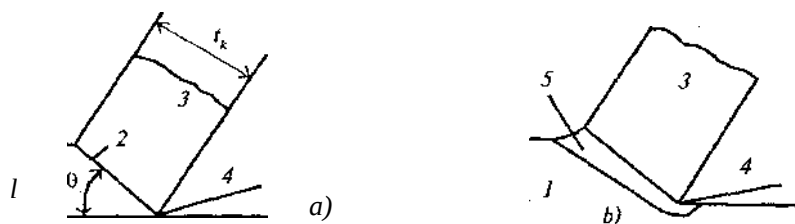
3.3- rasm. Kesishda deformatsiya zonasining sxematik tasviri: a) bir surilish tekisligiga ega bo'lgan model; b) rivojlangan zonaga ega bo'lgan model;
