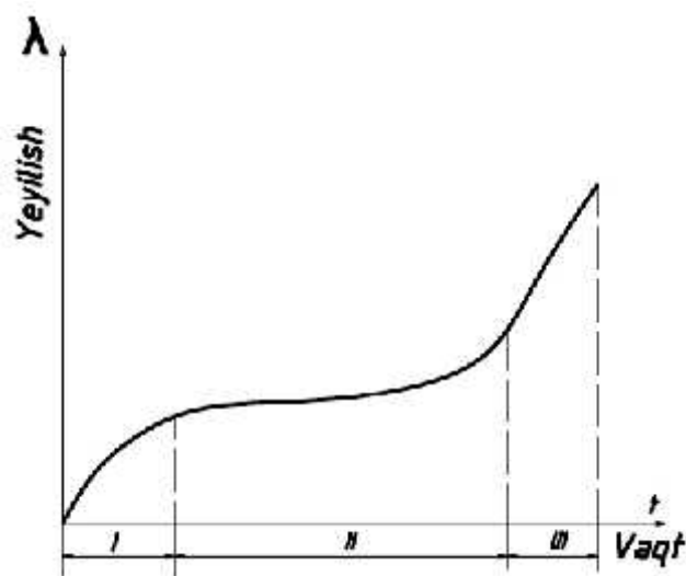
5.1.3-rasm. Yeyilishning vaqt bo'yicha o'zgarishi
