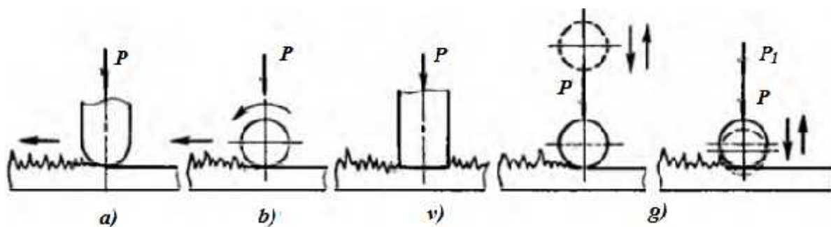
14.1.1-rasm. Sirtlar turli xil usullarda plastik deformatsiyalanganda asbobning ishlov beriladigan sirt bilan o'zaro ta'siri xarakteri
