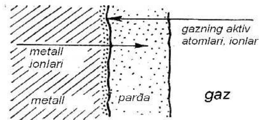
6.1.3-rasm. Kimyoviy korroziya vaqtida atomlarinig (ionlarining) ikki tomonlama diffuziyalanish sxemasi.
