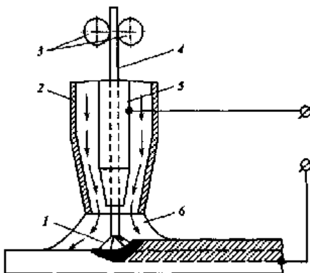
11.1.13-rasm. Himoyalovchi gazlar muhitida suyultirib qoplash sxemasi:
