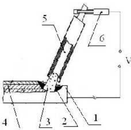
11.1.7-rasm. Qoplangan elektrod yordamida dastaki elektr yoyli suyultirib qoplash sxemasi:
