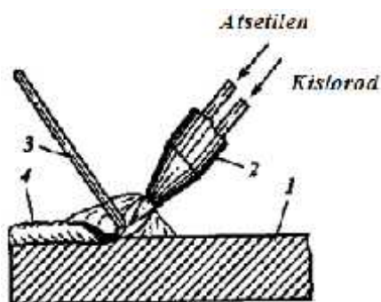
11.1.4-rasm. Gazli suyultirib qoplash sxemasi: 1 – suyultirib qoplanadigan detal; 2 – gaz yondirgichi (gorelka); 3 - qo'shiladigan material; 4 – suyultirib qoplanadigan metall.
