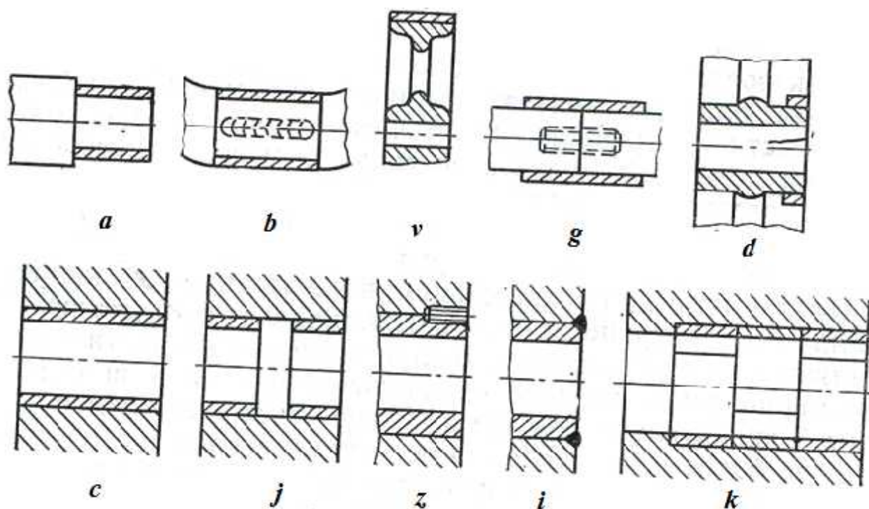
10.2.1-rasm. Detallarni ta'mirlashda halqalash.
