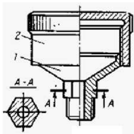
8.2.4-rasm. Qalpoqchali moydon.
