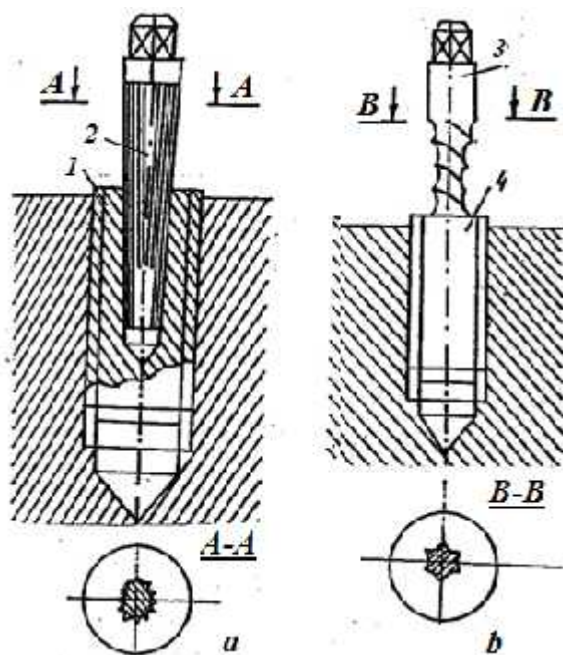
9.3.1-rasm. Vintlarni echib olish usullari.
