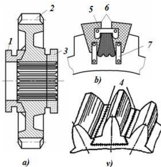
13.4.6-rasm. Tishli g'ildiraklarni ta'mirlash sxemalari:
