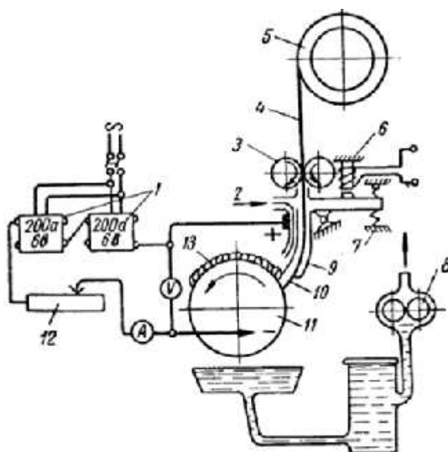
11.1.14-rasm. Avtomatik tebranma yoyli suyultirib qoplash uchun qurilmaning sxemasi
