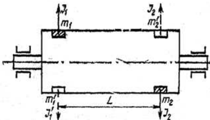
9.4.4-rasm. Dinamik nomuvozanatlik sxemasi.
