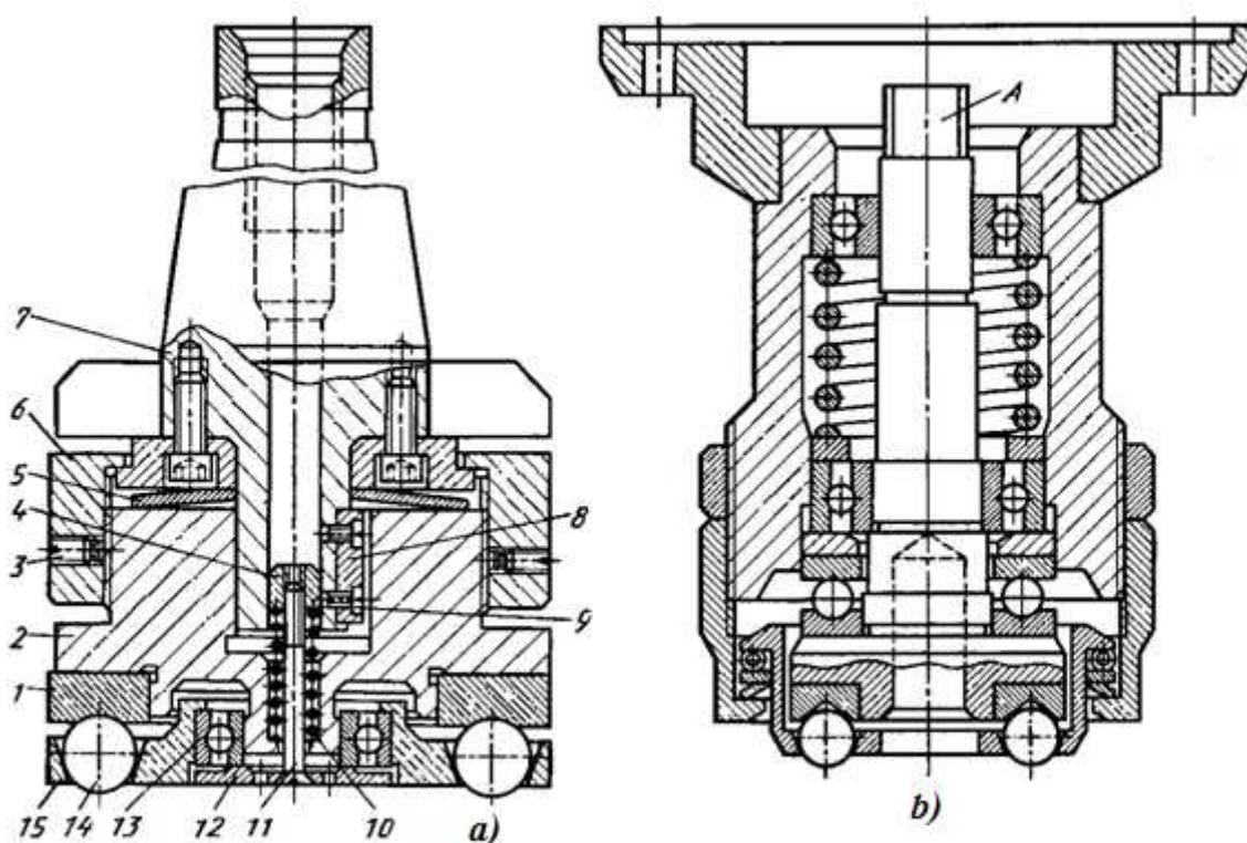
14.1.13-rasm. Tekis sirtlarga ishlov berish uchun kallaklar:
