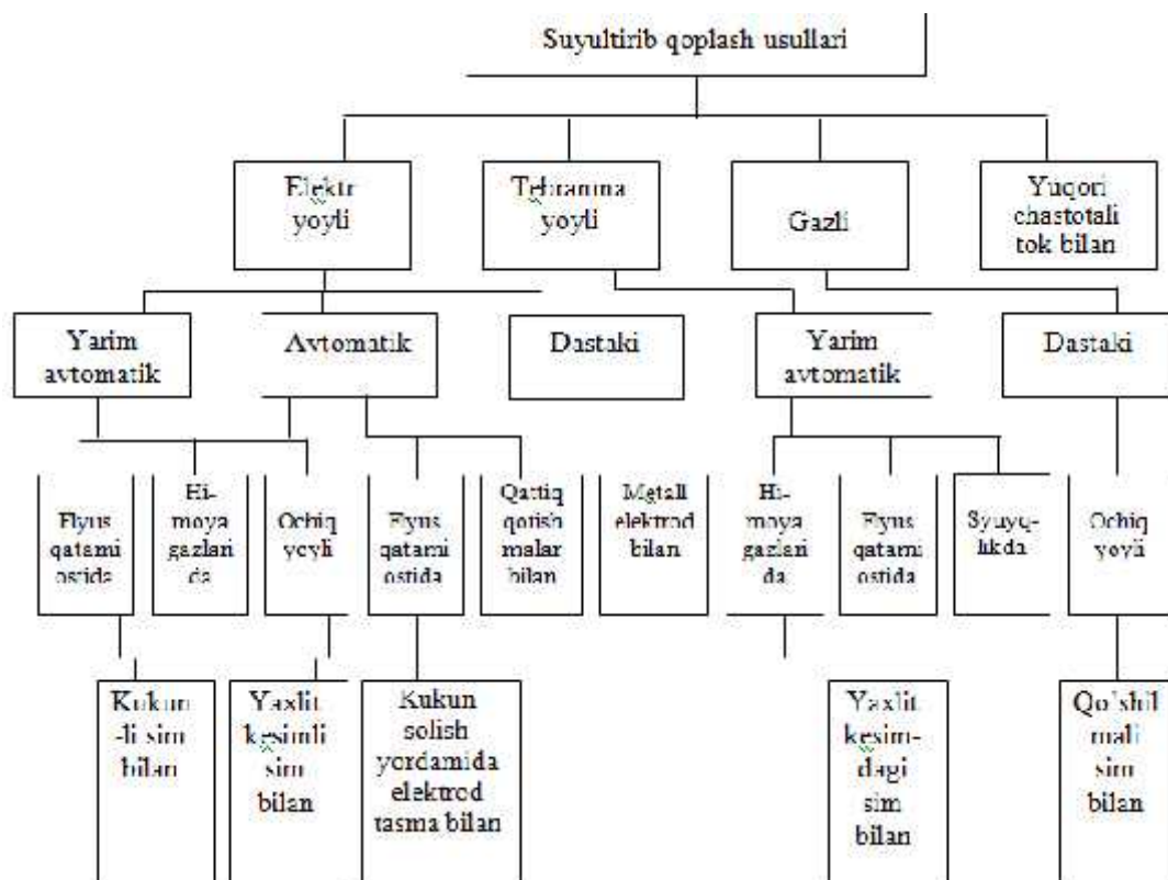
11.1.1-rasm. Yeyilgan detallarni suyultirib qoplash usullarida tiklash sxemasi
