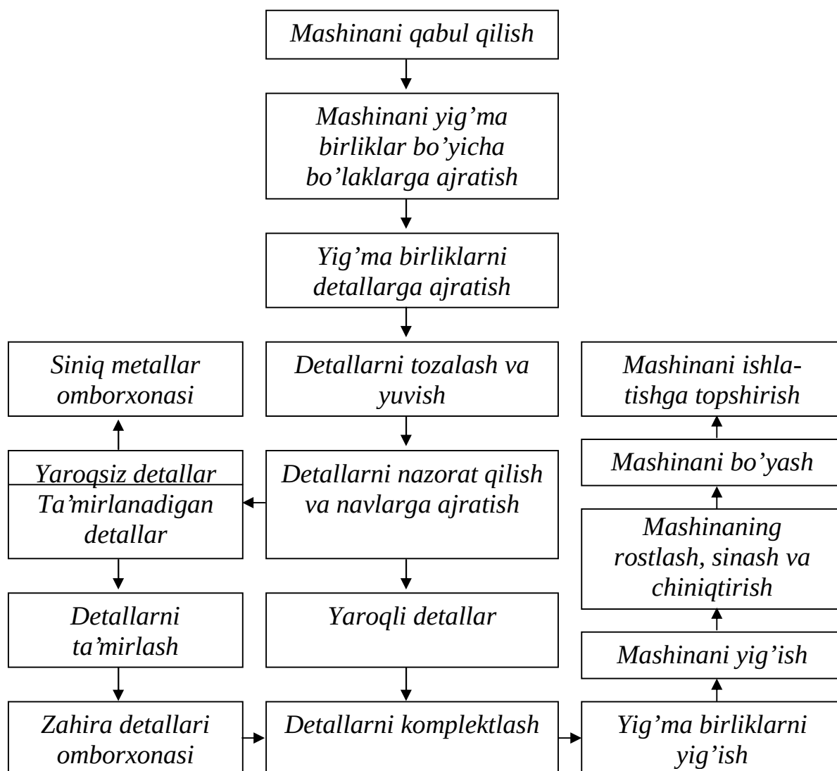
9.1.1-rasm. Mashinalarni ta'mirlash texnologik jarayoni.
