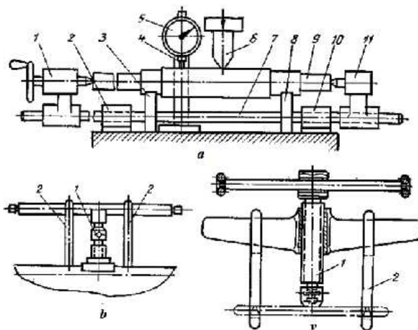
13.1.2-rasm. Statik egish bilan to'g'rilash usullari
