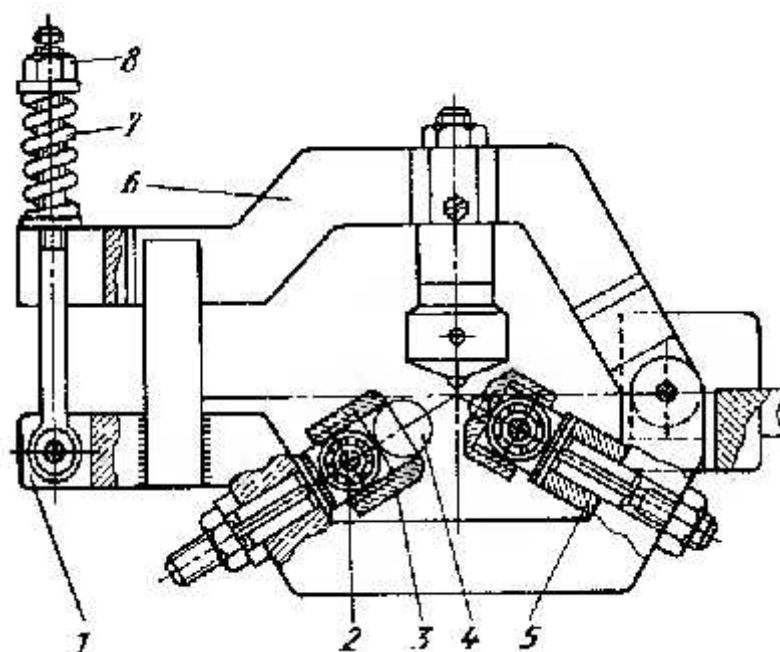
14.1.7-rasm. Elastik ta'sir qiluvchi ko'p zoldirli dumalatgich:
