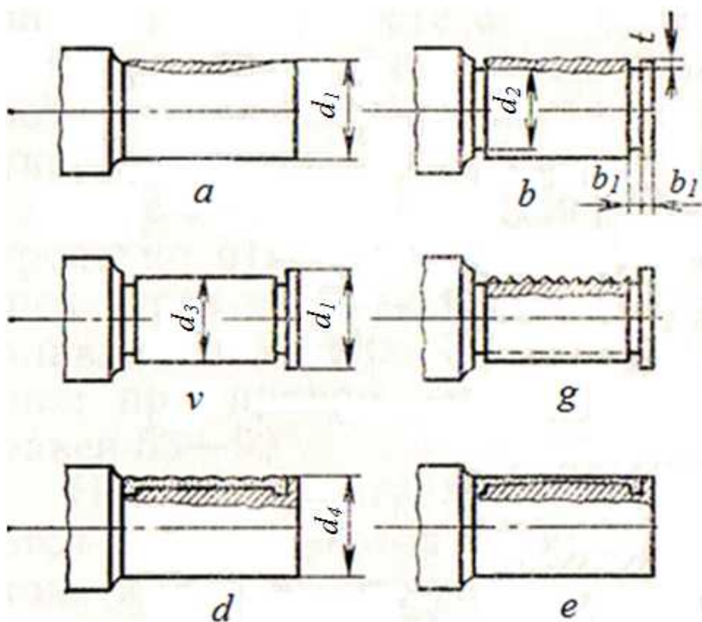
13.1.7-rasm. Gazotermik purkash usulida vallarni tiklash:
