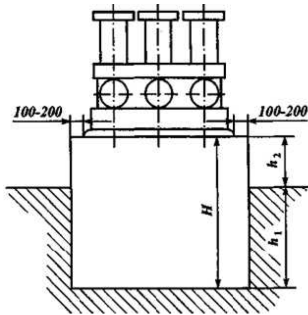
2.2.3-rasm. Poydevorning geometrik xarakteristiklari.
