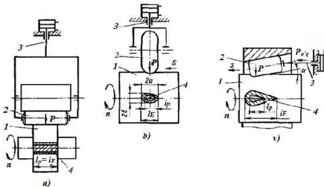
14.2.1-rasm. Rolikli dumalatishning xarakterli sxemalari:
