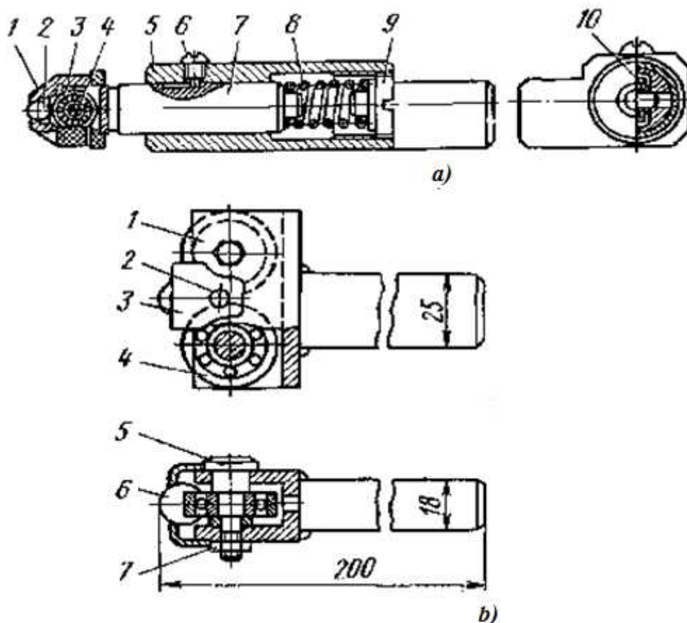
14.1.4-rasm. Bir zoldirli dumalatgichlar:
