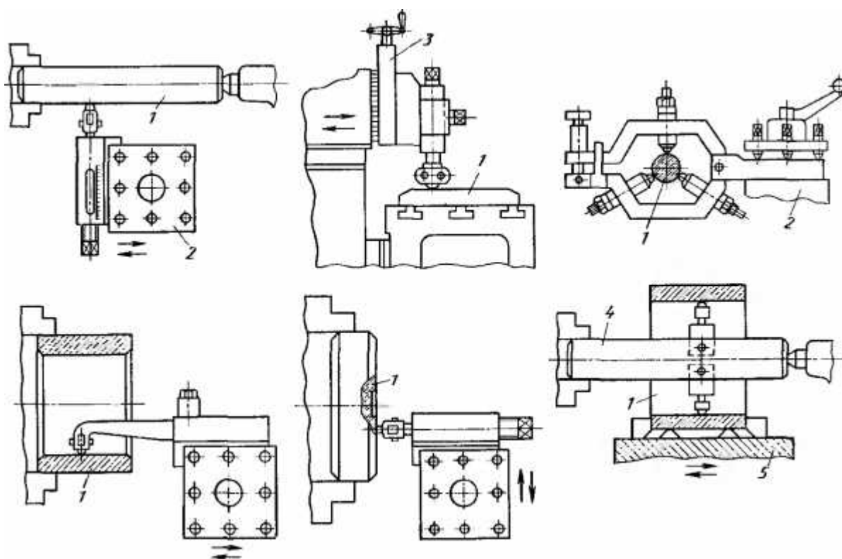
14.1.14-rasm. Detallar sirtini turli xil universal metall kesuvchi stanoklarda dumalatib puxtalash sxemalari:
