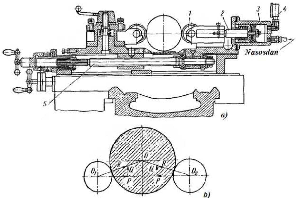
14.2.9-rasm. Ikki rolikli moslama (a) va kuchlar sxemasi (b): 1 – rolikli kallak; 2 – shtok; 3 – gidrosilindr; 4 – manometr; 5 – vint
