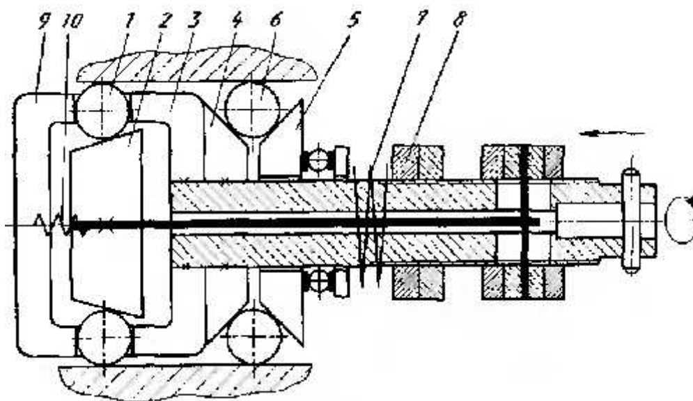
14.1.11-rasm. Kombinatsiyalashtirilgan ikki qatorli elastik-qattiq dumalatgich: 1 – birinchi qator zoldirlar; 2 – qattiq konus; 3 – separator; 4 – qo'zg'almas konus; 5 – prujinalangan konus; 6 – ikkinchi qator zoldirlar; 7 – prujina; 8 – gayka; 9 – halqa; 10 – prujina
