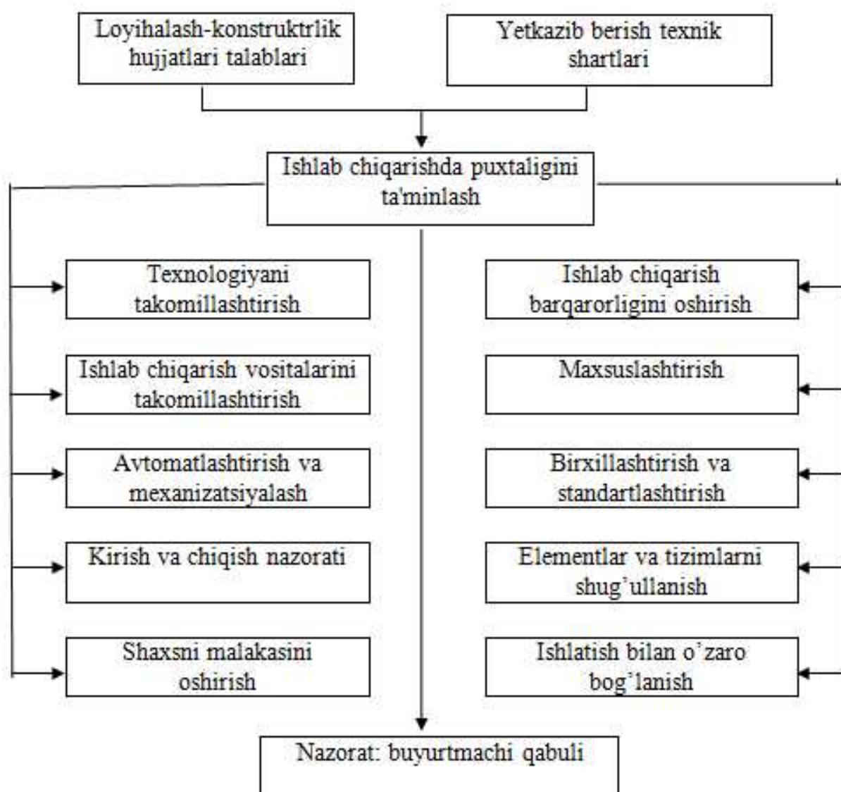
3.3.1-rasm. Ishlab chiqarishda jihozning puxtaligini ta'minlash bo'yicha tadbirlar strukturasi.
