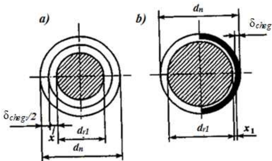
10.1.2-rasm. Ta'mir o'lchamini aniqlash sxemasi:
