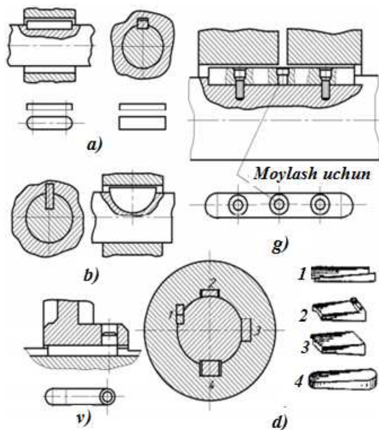
13.5.1-rasm. Shponkalarining konstruksiyalari:
