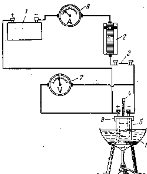
11.3.4-rasm. Elektrolitik xromlash uchun qurilma sxemasi:
