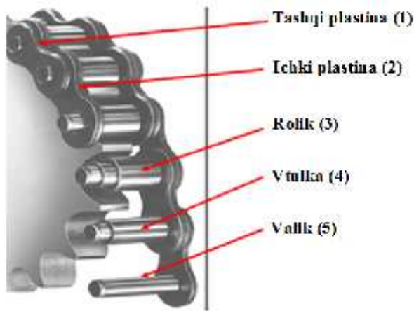
10.1.1-rasm. Vtulka-rolikli zanjir sxemasi
