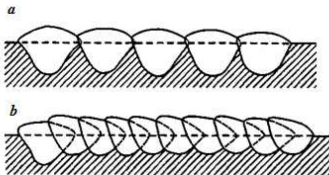
11.1.12-rasm. Valiklarni suyultirib qoplash sxemasi: a – qoplashning katta qadami; b – qoplashning kichik qadami
