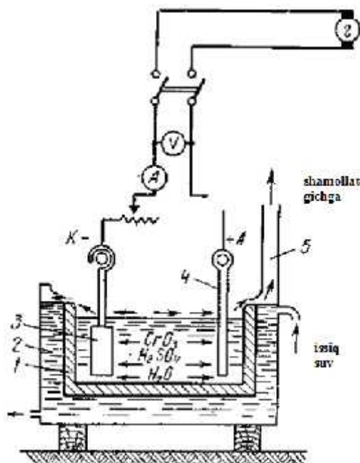
11.3.3-rasm. Xromlash uchun elektrolitli vanna sxemasi:
