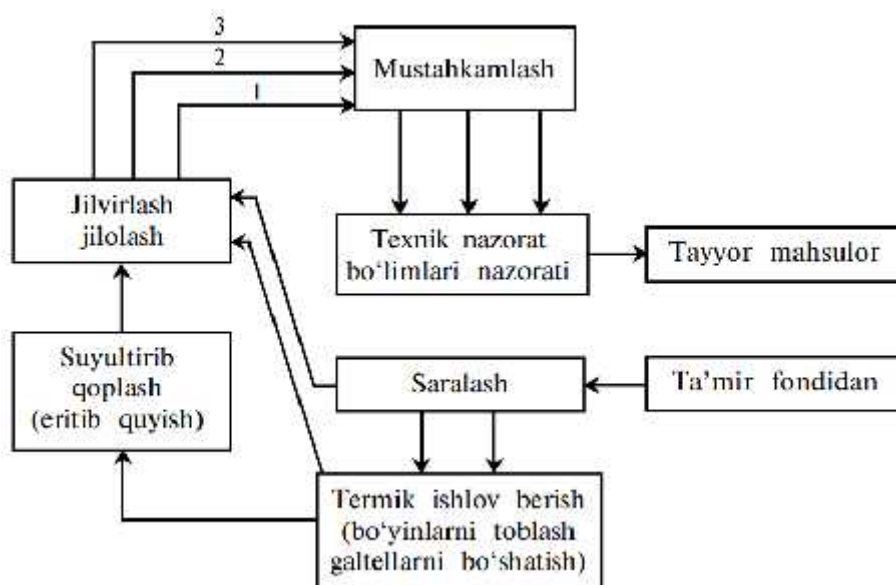
13.1.4-rasm. Tirsakli val bo'yinlarini yo'nalishlar bo'yicha ta'mirlash texnologik jarayonining sxemasi.
