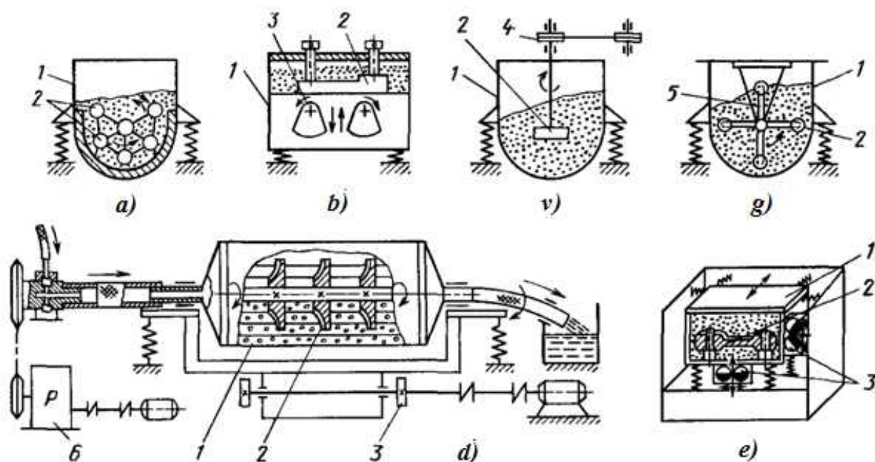
14.3.2-rasm. Detallarga konteynerga qotirib ishlov berish sxemasi:
