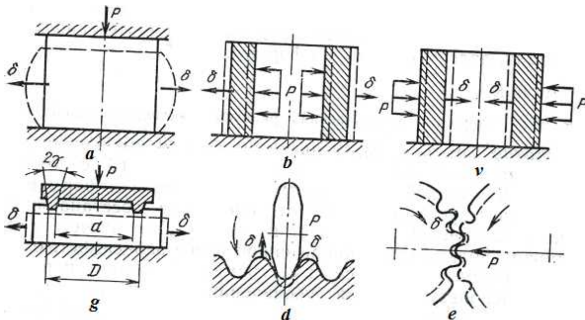
10.2.2-rasm. Yeyilgan detallarni metallni plastik qayta taqsimlash usulida tiklash:
