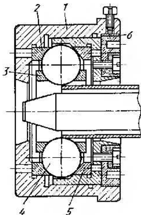
14.1.8-rasm. Qattiq ko'p zoldirli dumalatgich:
