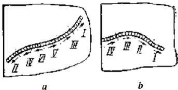
11.1.9-rasm. Mashina detallaridagi darzlarni payvandlab tuldirishda choklarni yotqizish tartibi:
