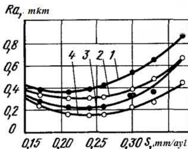
14.2.5-rasm. Ra ni rolkning bo'ylama uzatishdan bog'liqligi:
