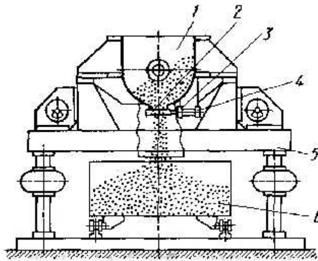
14.3.7-rasm. Yordamchi ishlarni mexanizatsiyalashtirish uchun konteyner
