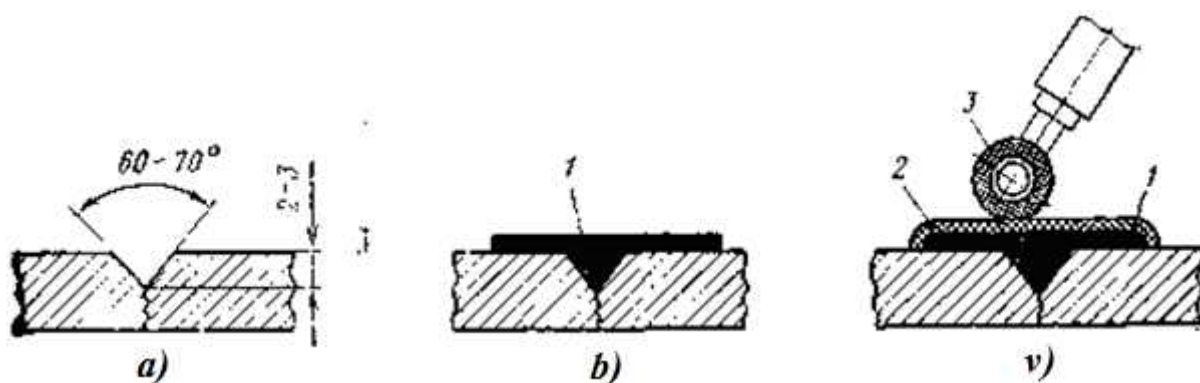
11.4.2-rasm. Darzlarni yamash sxemasi:
