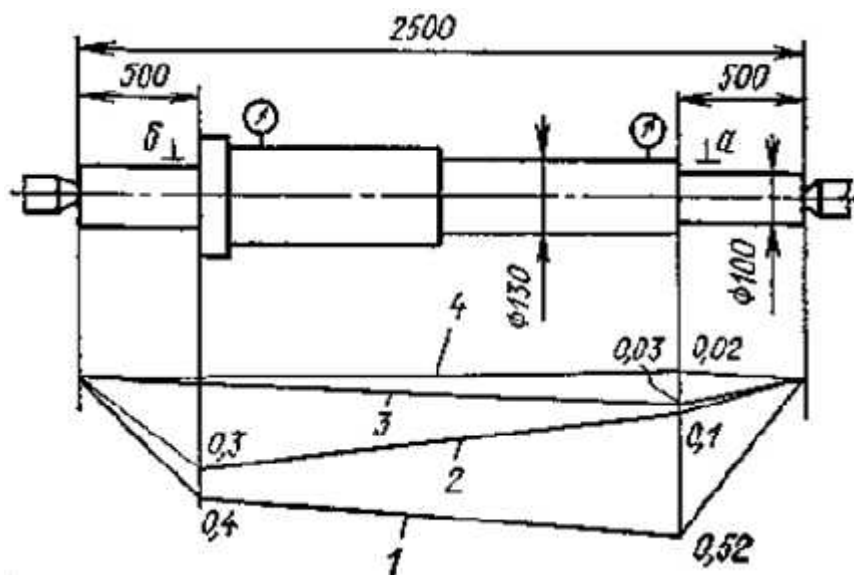
13.1.3-rasm. Valni qizdirib to'g'rilash
