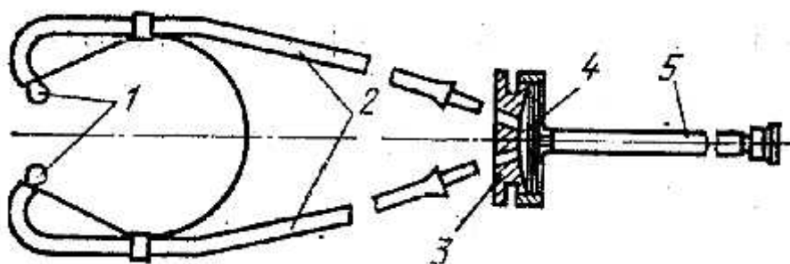
4.2.1-rasm. Stetoskop
