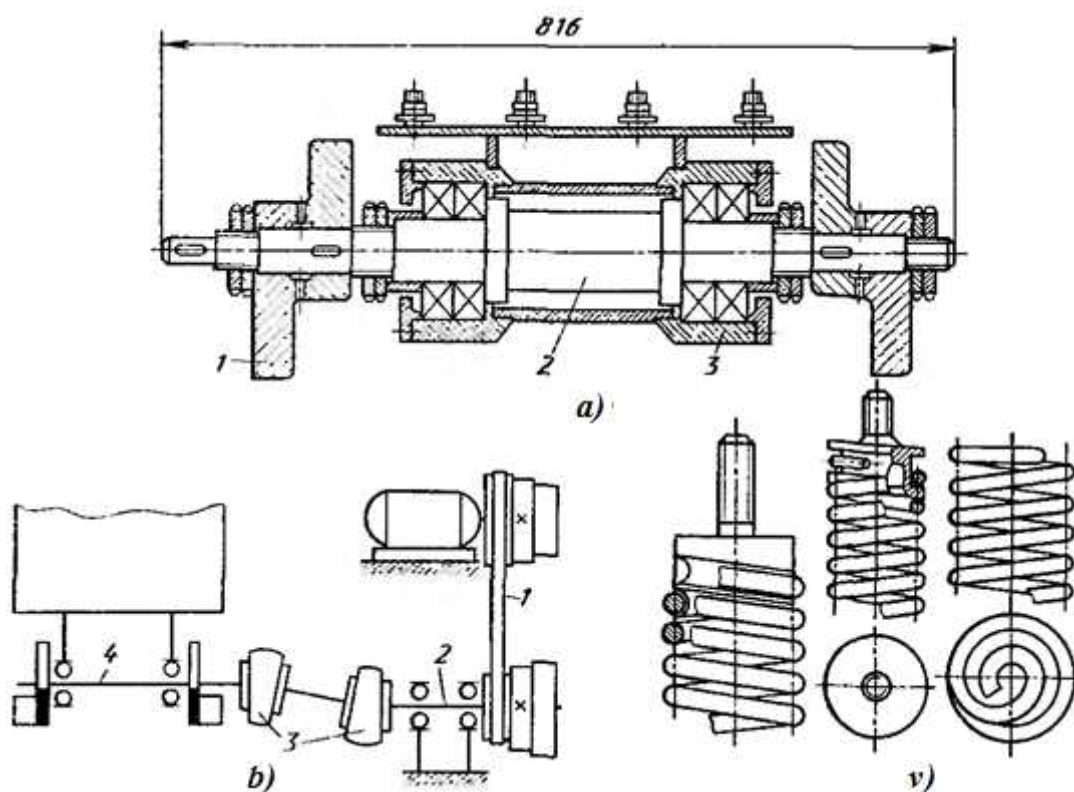
14.3.4-rasm. Vibratsion stanoklarning asosiy uzellarini tayyorlashga misollar: a - muvozanatlashtirilmagan titratgich; b – yuritma; v – elastik elementlar
