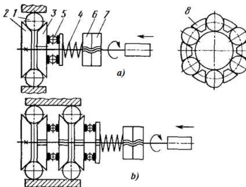
14.1.12-rasm. Zoldirlar tayanchi prujinalangan konusda joylashgan elastik dumalatgichlar:
