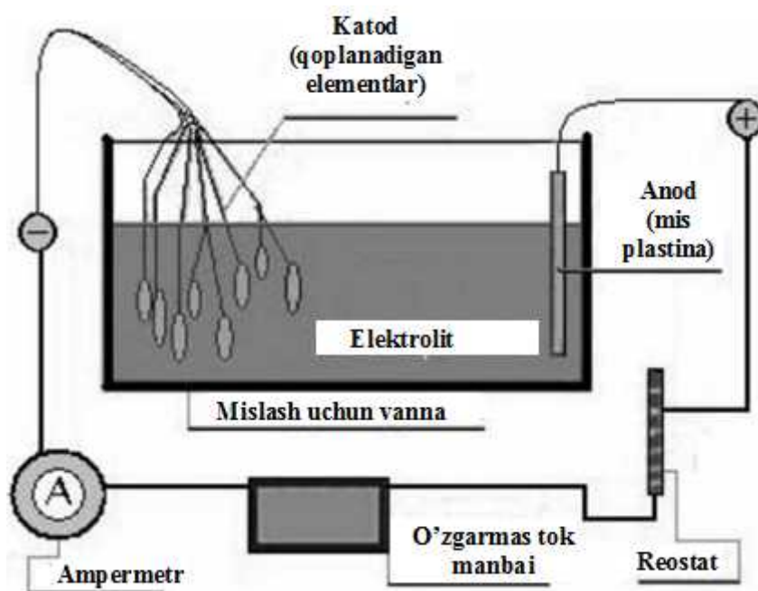
11.3.5-rasm Detalni elektrolitda cho'ktirib mislash
