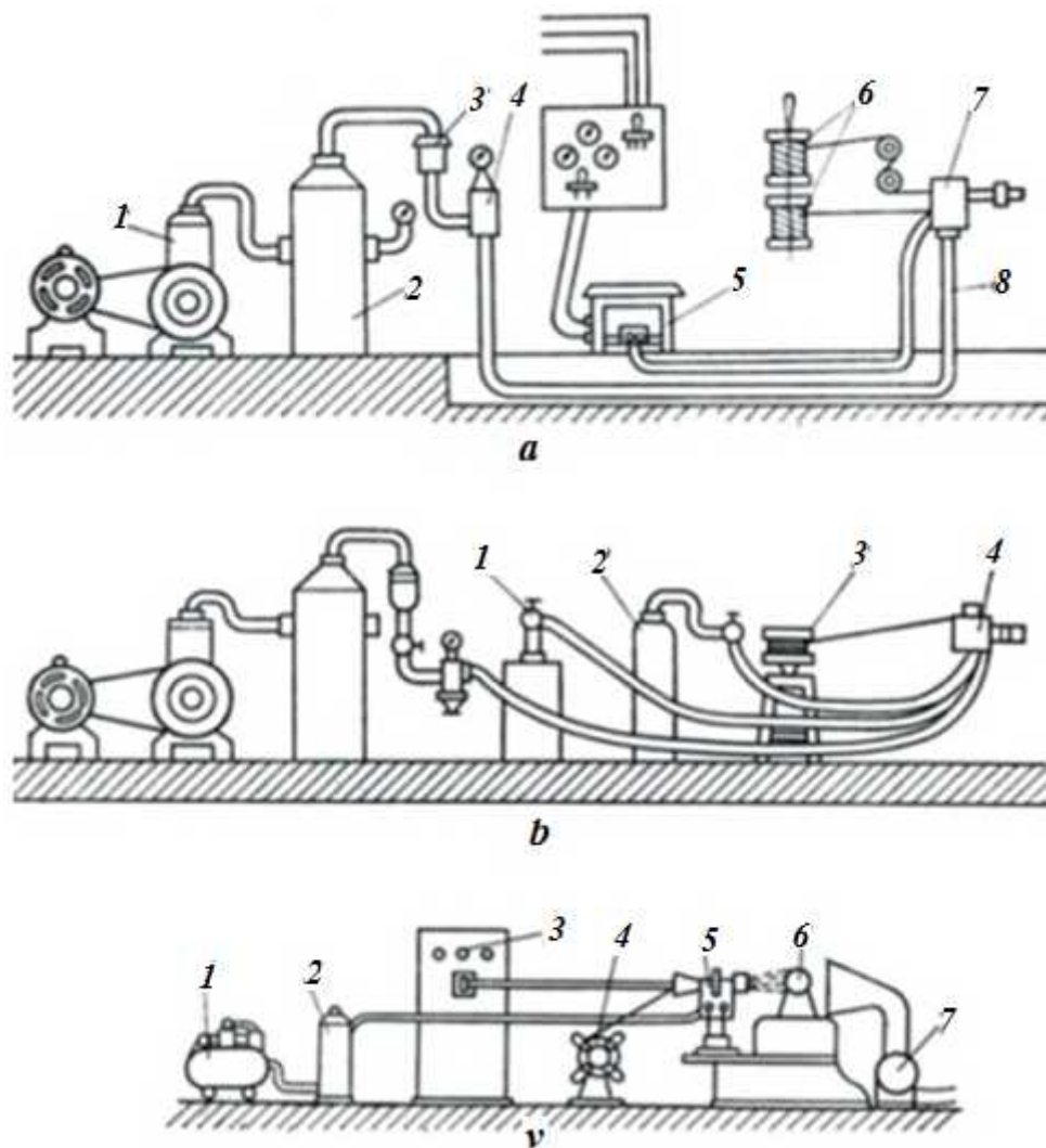
12.1.3-rasm. Gazotermik purkash uchun qurilmalar sxemasi:
