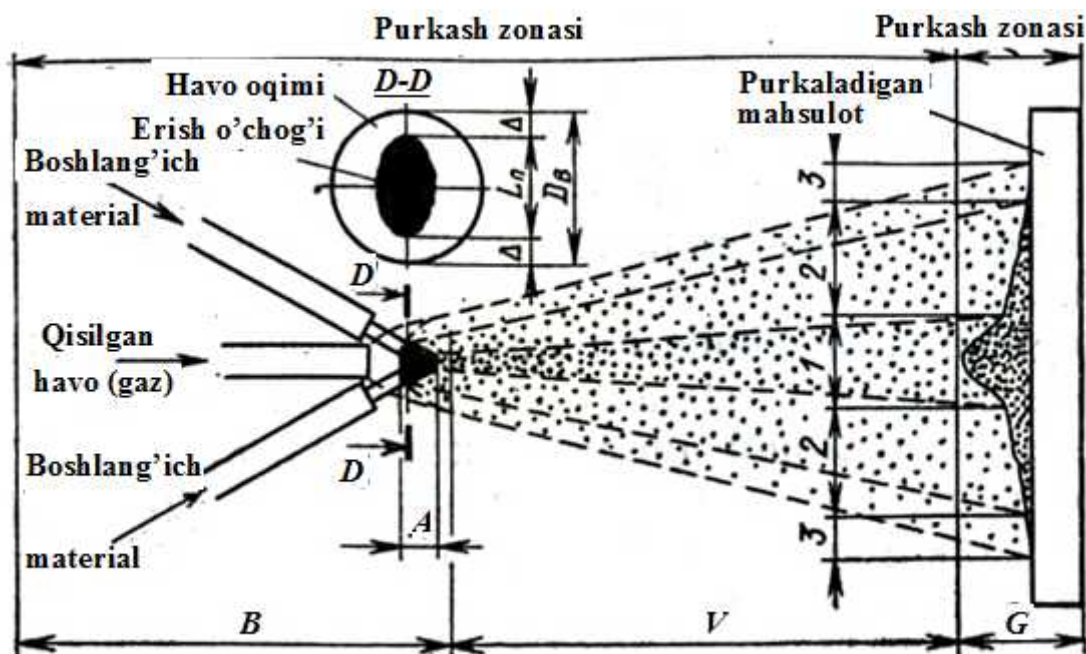
12.1.1-rasm. Materiallarni gazotermik purkashning printsipl sxemasi:
