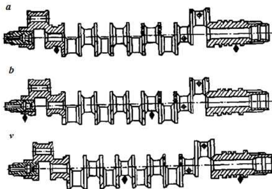
13.1.5-rasm. Tirsakli valni to'g'rilash sxemasi:
