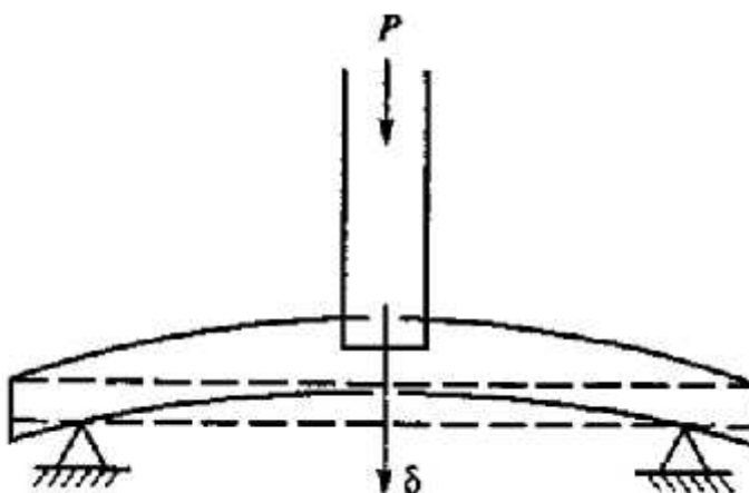
10.2.3-rasm. To'g'rilash sxemasi.
