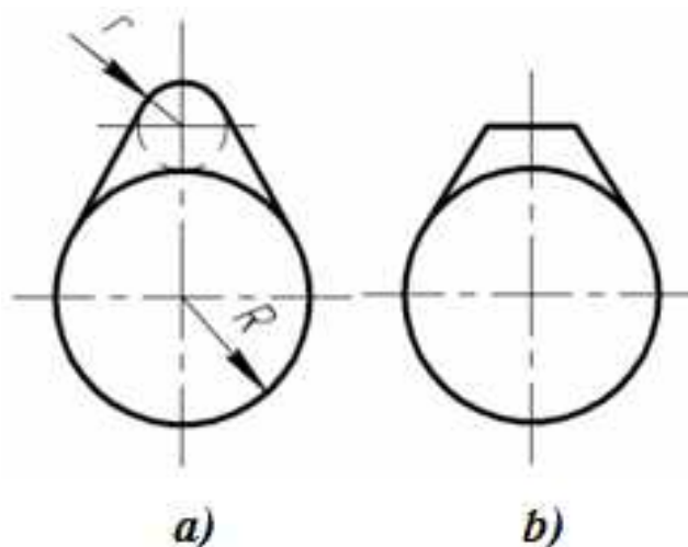
13.3.1-rasm. Boshlang'ich (a) va yeyilgan (b) kulachoklar
