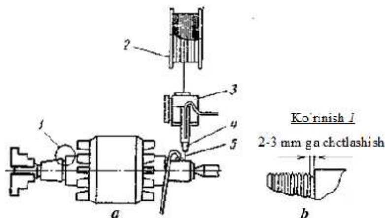
11.1.3-rasm. Detallarni suyultirib qoplash uchun qurilmaning sxemasi: a) suyultirib qoplash uchun kurilmaning sxemasi; b) suyultirib qoplashdan oldin detal sirtini tayyorlash
