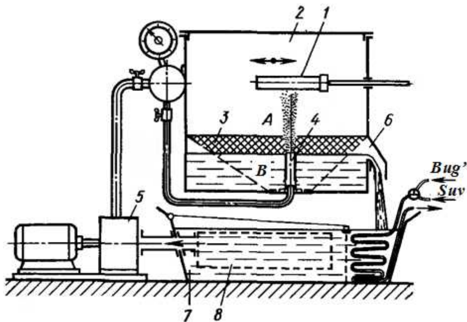
14.4.6-rasm. Gidropitraoqimli ejektorli qurilmaning sxemasi:
