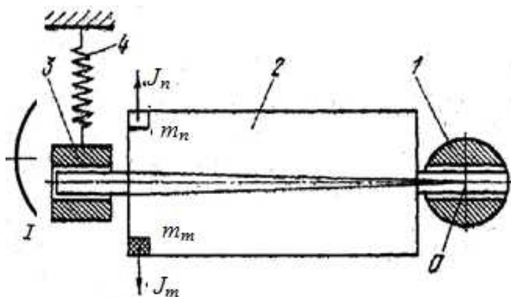
9.4.5-rasm. Dinamik muvozanatlash uchun qurilma sxemasi:
