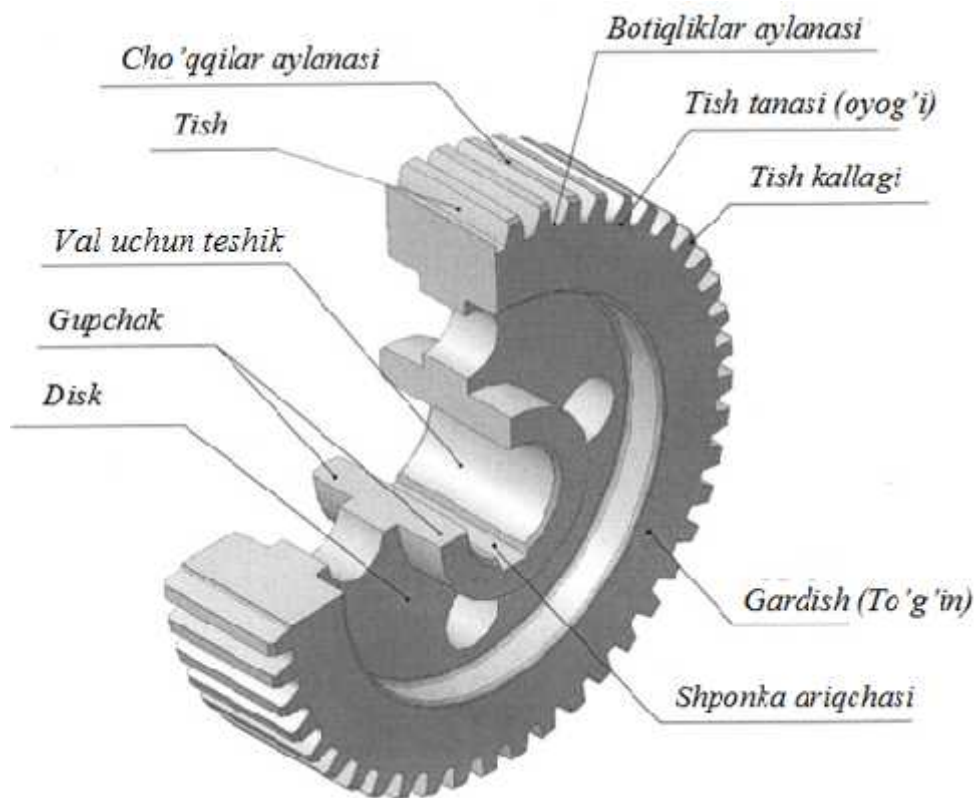
13.4.1-rasm. Tishli g'ildirak sxemasi
