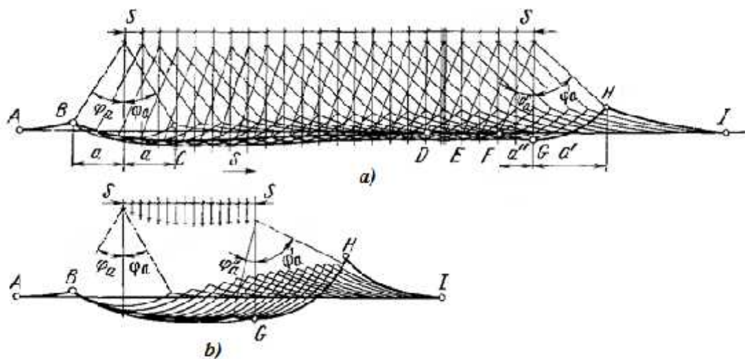
14.2.3-rasm. Ishlov berilayotgan sirtni S bo'ylama uzatish bilan rolik yordamida dumalatishda ketma-ket deformatsiyalanish sxemasi a – me'yordagi jarayonda; b – nobarqaror jarayonda
