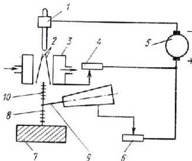
12.2.1-rasm. Sim yoki sterjen bilan plazmali qoplash qurilmasining sxemasi:
