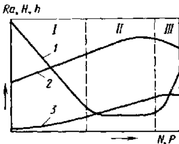
14.2.4-rasm. Yuklash tsikllari soni N va dumalatish kuchi P ning ta'sir etish xarakteri:
