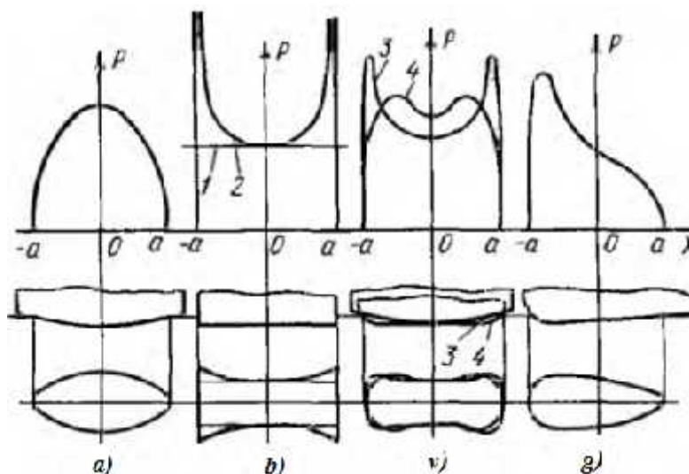
14.2.2-rasm. Dumalatish paytida deformatsiyalanish nuqtasida bosimlar epyurasi va roliklar izining xarakterli shakllari:
