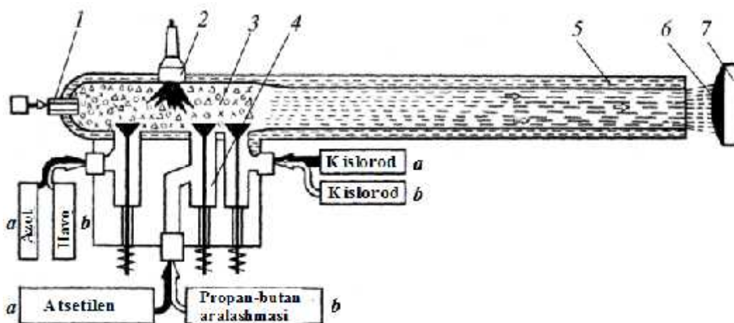
12.3.1-rasm. Purkash texnologiyasidagi detonatsiyalash qurilmasining sxemasi:
