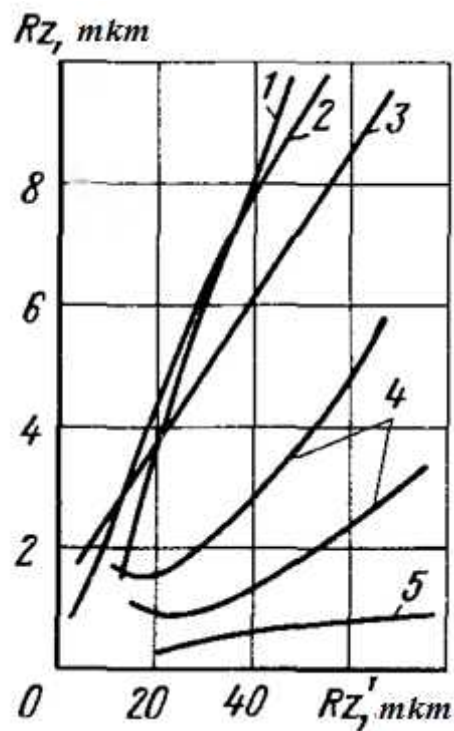
14.2.6-rasm. Har xil materiallar uchun dumalatishda hosil qilingan Rz parametrining boshlang'ich Rz' parametrdan bog'liqligi:
