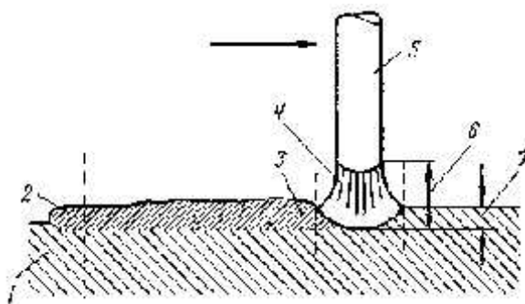
11.1.2-rasm. Suyultirib qoplash jarayoni sxemasi.
