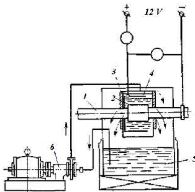
11.3.5-rasm. Vannasiz xromlash va po'latlash sxemasi:
