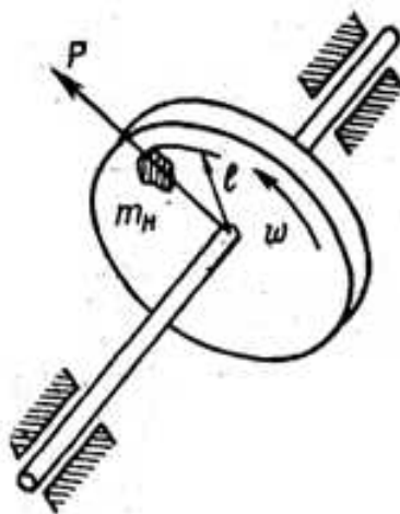
9.4.2-rasm. Nomuvozanat massaning yo'nalishi va joylashuvi.
