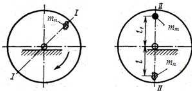
9.4.3-rasm. Statik nomuvozanatlik sxemasi.
