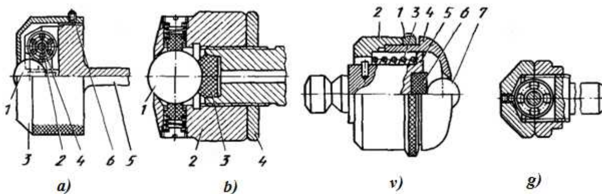
14.1.3-rasm. Zoldirli kallaklar:
