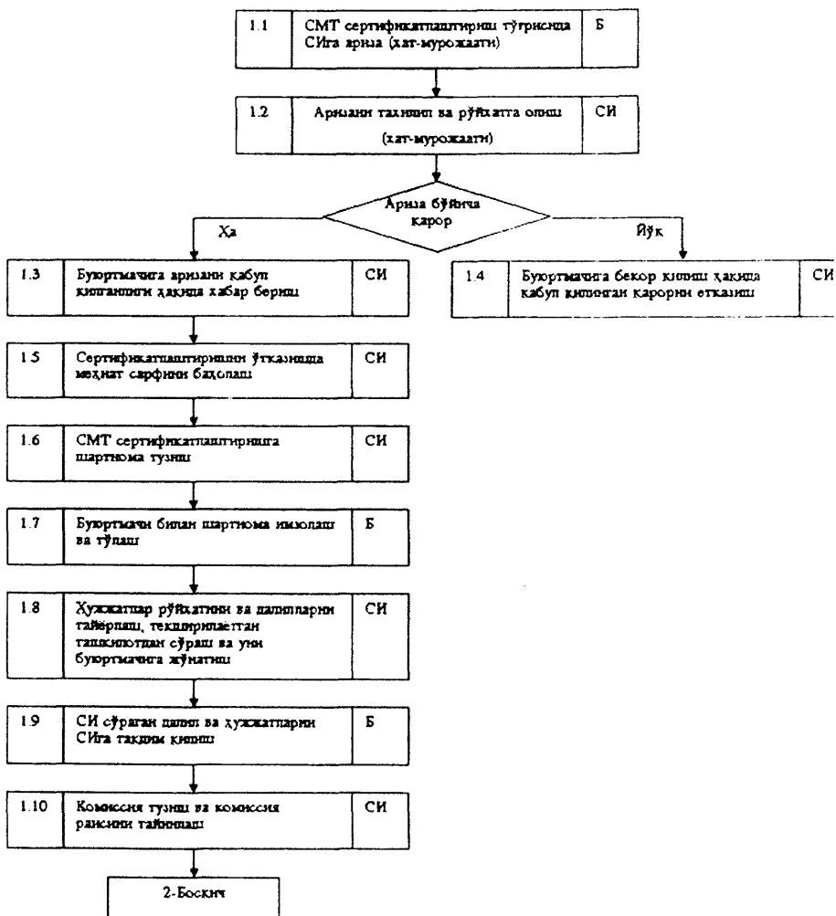
Расм. 3.1. Ишларни ташкиллаштириш (1-босқич)
