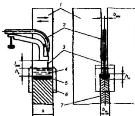
6.1-rasm. Elektr-shlak payvandiash chizmasi:
