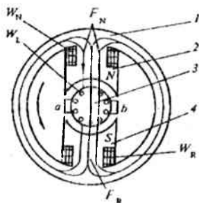
5.10-rasm. Kollektorli payvandlash generatorining (ko'ndalang kesimi) tuzilishi:
