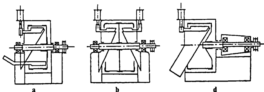
14-rasm. ФГН tipidagi sentrifugalarda rotorning joylashish sxemasi:
