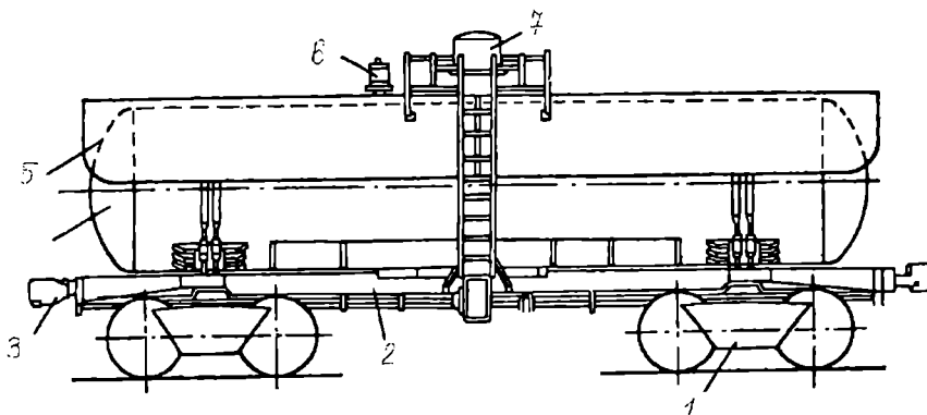
44-rasm. Siqilgan gazni tashish uchun sisterna:
