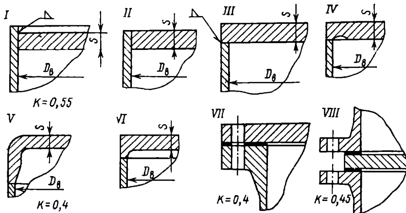
94-rasm. Obechaykalar yassi (tekis) tublarni biriktirish varianti va tub konstruksiyasi koeffitsienti K ning ahamiyati
