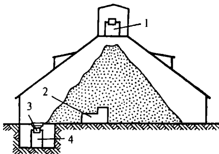
70-rasm. Maydalangan material saqlanadigan ombor:
