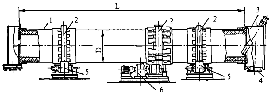
34-rasm. Ikki tayanchli suriladigan kallakli aylanma pech: 1 – korpus; 2 – belbog‘ (bandaj); 3 – suriladigan kallak; 4 – patrubok; 5 – roliklar; 6 – reduktorli elektr yuritgich.
