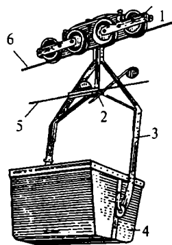
45-rasm. Osma arqonli yo'l vagonetkasi:
