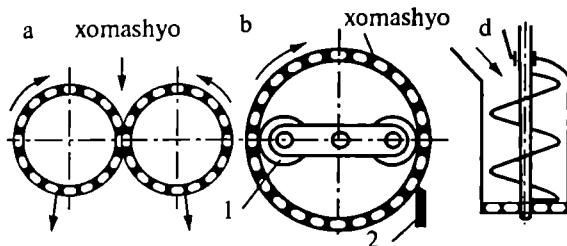
32-rasm. Ekstruzion tipdagi donalagichlar:
