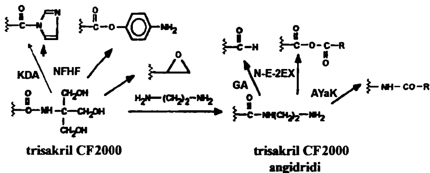
48-rasm. Affin xromatografiyasi uchun trisakril CF 2000 asosida ba'zi sorbentlarni olish. KDA – karbonildiimidazol.
