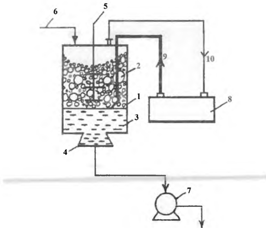
13-rasm. Suyuqlik-gaz tizimida fazalarning ajratuvchi yuzasida immobillangan, zamburug'li organizmlar yordamida uglevod saqlovchi xomashyolarni biyg'itish uchun fermentator:
