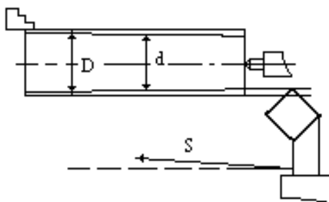
2.10-rasm. Dastgoh geometrik noaniqligiga misollar
