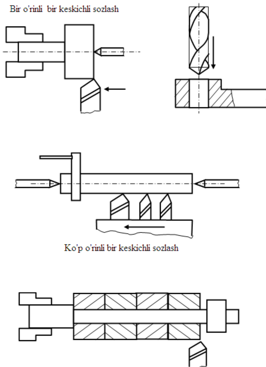
5.4-rasm. Detallarni turli sozlash sxemalari
