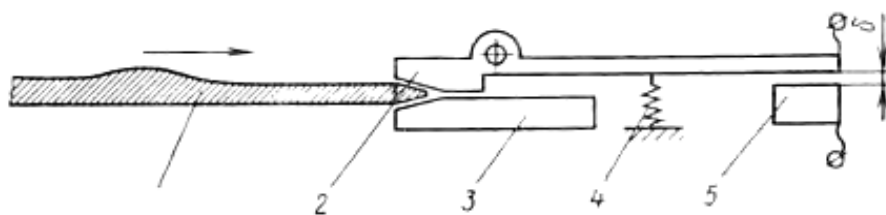
10.6-rasm.Konusni charxlash operatsiyasini nazorat qiluvchi qurilma
