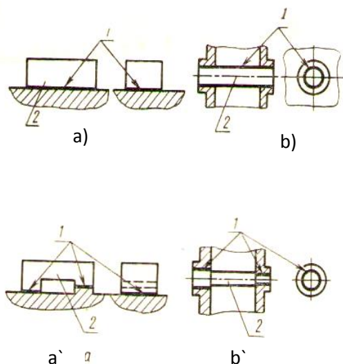
2.11- rasm. Asos turlari
