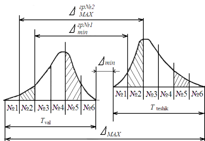
6.2- rasm. Tutashuvchi detallar o'lchamlarini taqsimlash qonunlarini qarama-qarshi assimetriyali bo'lgan birikmalarni selektiv yig'ish sxemasi.
