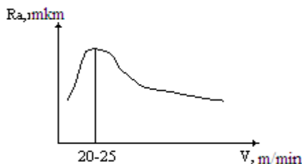
3.9-rasm. Kesish tezligini yuza gʻadir-budurligiga taʼsiri
