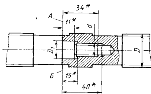
8.9-rasm. Sirpanish podshipniklariga o'rnatilgan cho'zuvchi ssilindrlar o'lchamlari
