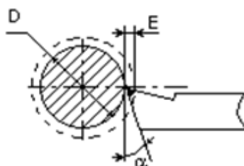
2.6 – rasm. Kesuvchi asbob eyilishini aniqlikka ta'siri
