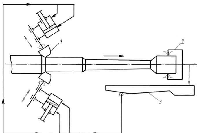
8.4-rasm. SHpindellar uchun tayyorlamalarni davriy prokatlash sxemasi 1-konik g‘o‘lacha; 2-o‘zimarkazlanuvchi patron; 3-nusxa olish chizig‘i.
