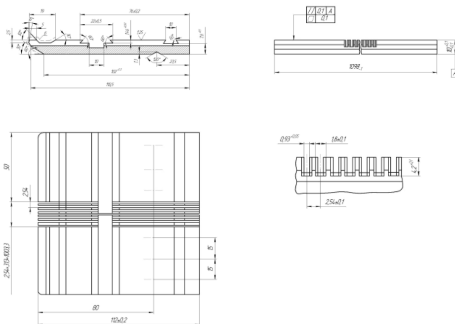
10.1-rasm Trikotaj mashinasini yassi to'quv ignadoni
