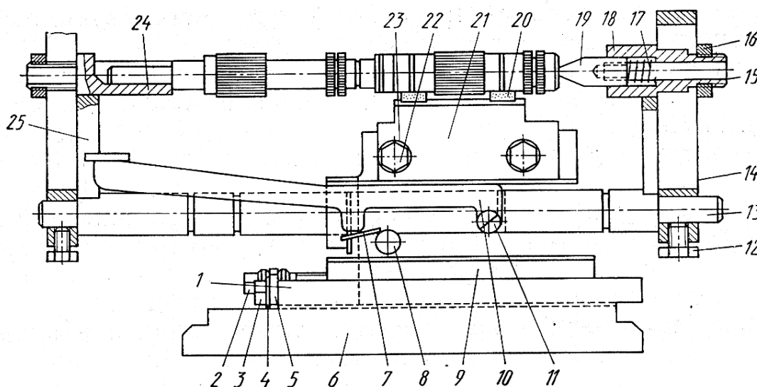
8.11-rasm. Cho'zuvchissilindrlar oraliq bo'yinchalarini juvalash uchun moslama
