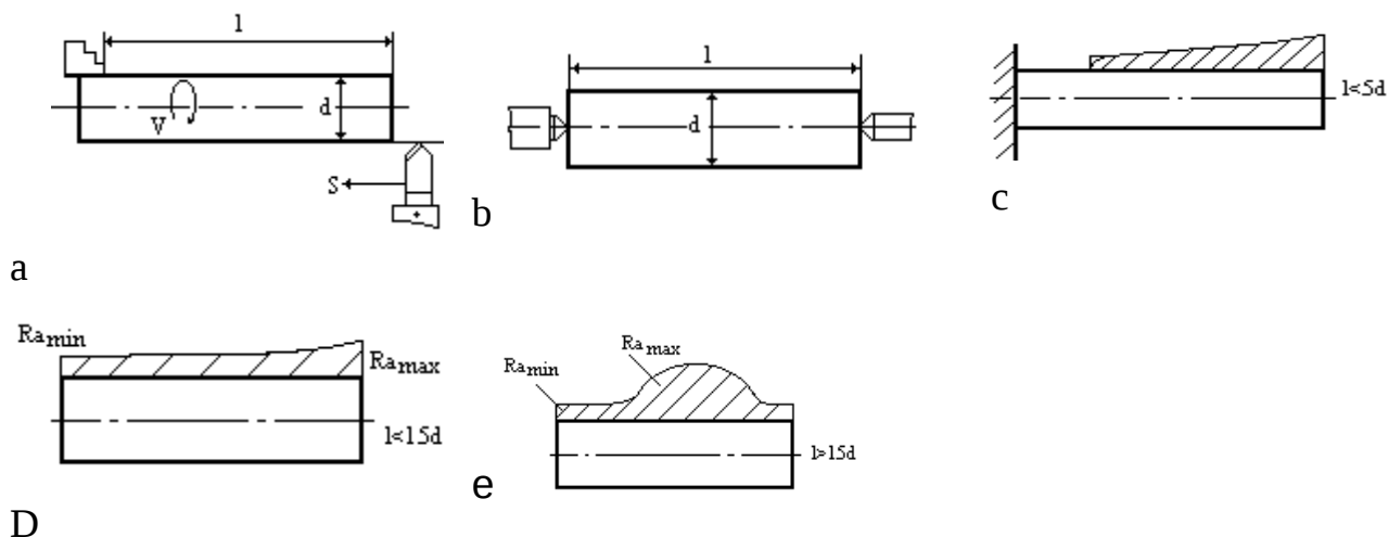
3.12 – rasm. DMAD tizimini gʻadir-budurligiga taʼsiri
