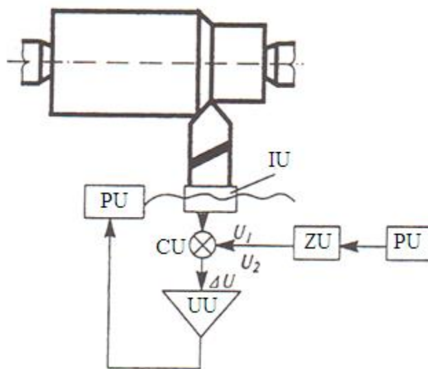
2.22-rasm. Kesuvchi kuchni doimiyligini ta'minlovchi qurilma sxemasi
