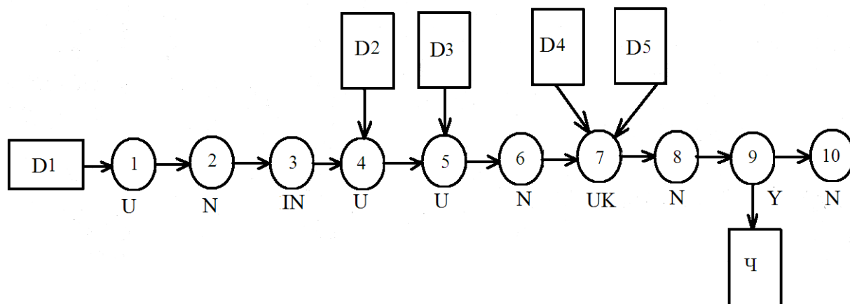
6.6- rasm. Avtomatik qismli yig'ishni texnologik sxemasi
