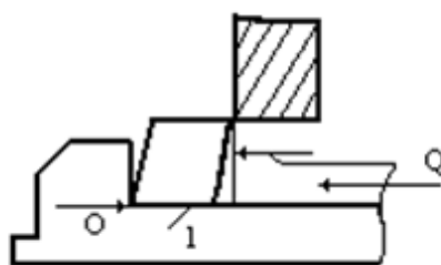
2.21 – rasm. Siquvchi kuch ta'sirida tayyorlamani siljishi
