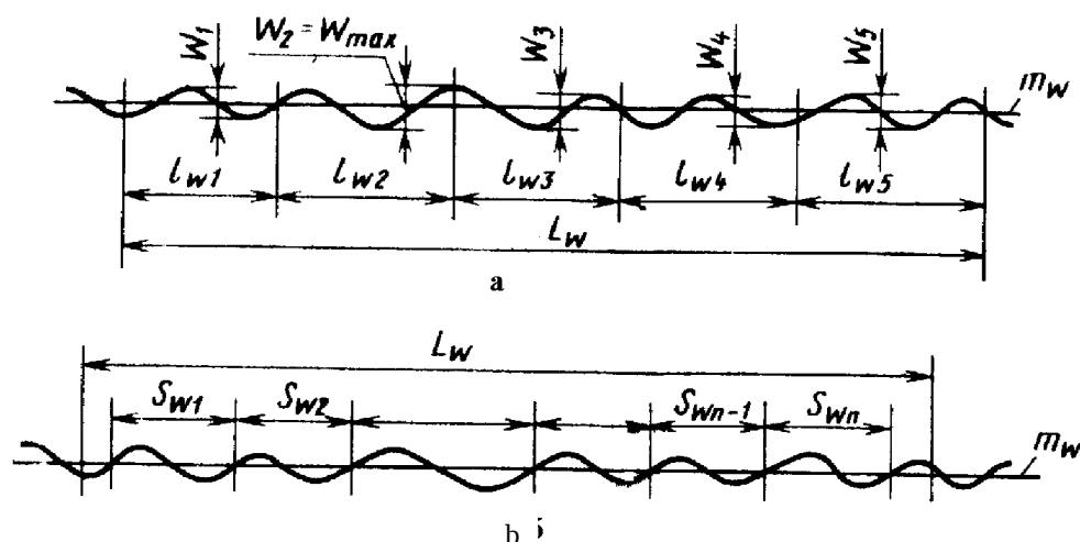
3.7-rasm. Yuza to'liqsimonligi to'liqining balandligi (a) va qadamini (b) o'lchash.
