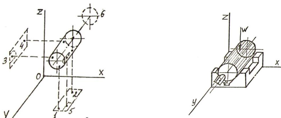
2.16-rasm ssilindr detallarni asoslash
