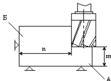
2.14-rasm O'lcham asoslari
