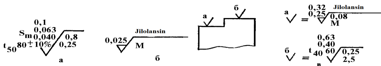
3.4-rasm. Yuza gʻadir-budurligini belgilash misollari.
