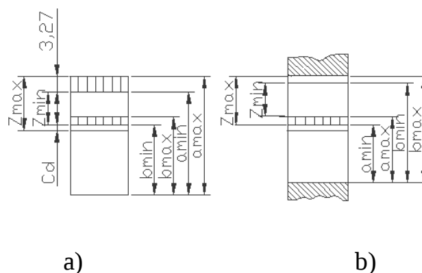
4.2-rasm. Ishlab berish va joizliklarga operatsiyalararo quyimni joylashuv sxemasi: a-val uchun; b-teshik uchun
