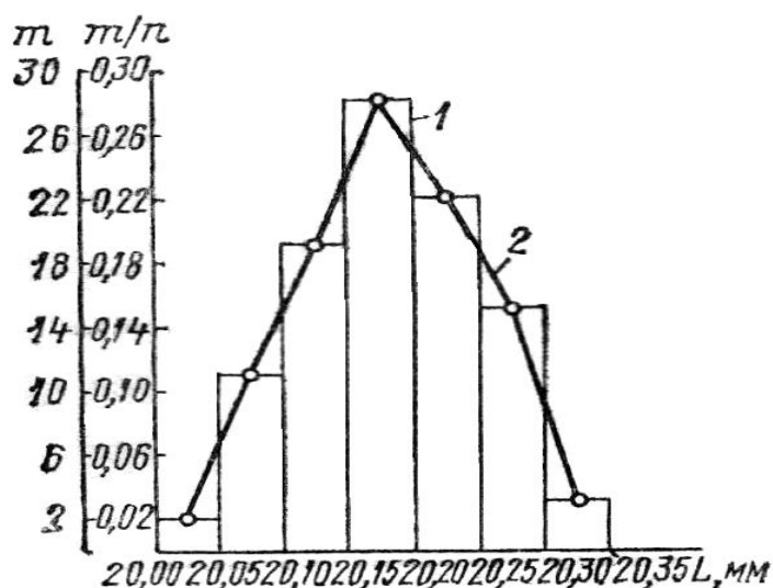
2.24-rasm. Tayyorlamani o'lchamlarini taqsimlanishi va egrisi.
