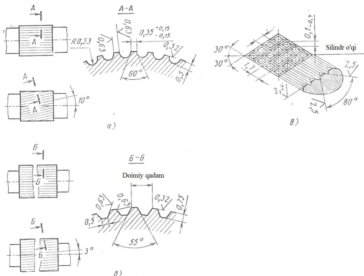
8.8-rasm. Cho'zuvchissilindrlarni bajarilishi, profili va o'lchamlari
