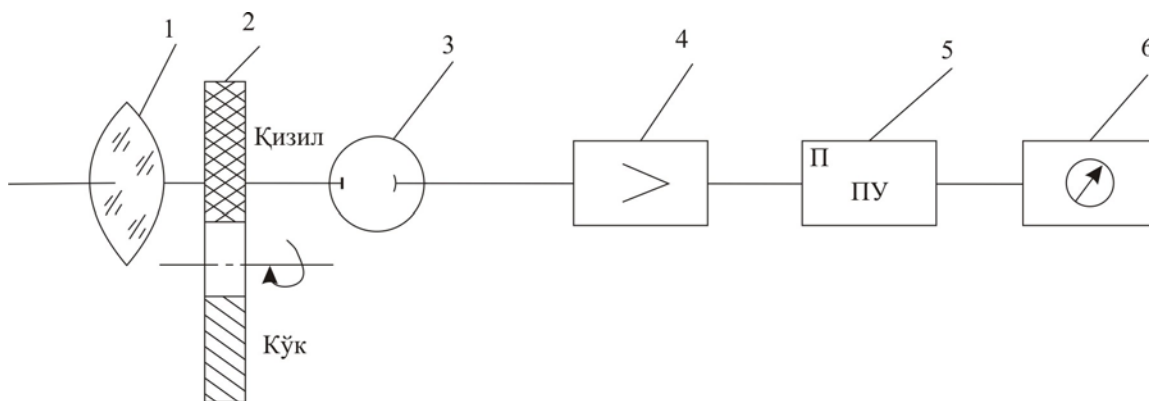
2.26 – расм. Фотоэлементли рангли пирометрнинг принципиал схемаси.
