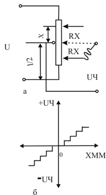
7.2 – расм. Икки тақтли потенциалрик датчик:
