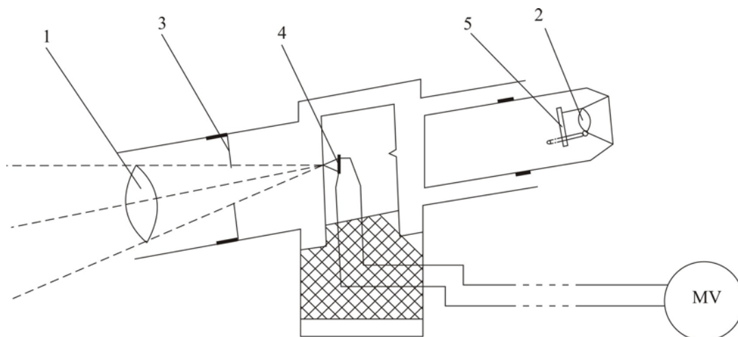
2.27 – расм. Радиацион пирометрнинг принципиал схемаси.
