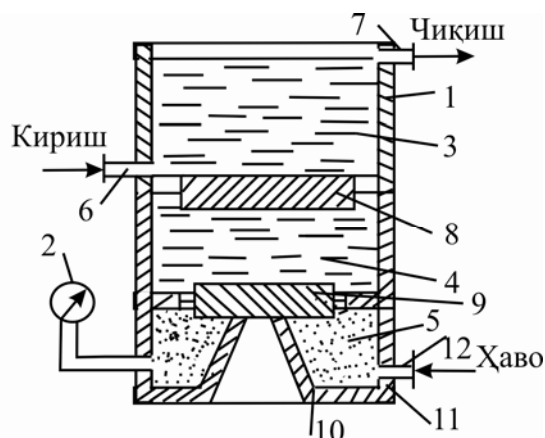
6.35 – расм. Мембрана – вазнли зичлик ўлчагичнинг
