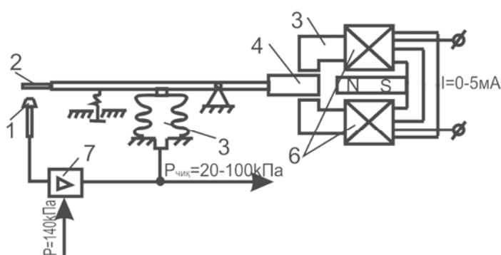
8.13 – расм. Электр – пневматик ўзгарткичнинг принципаал схемаси.
