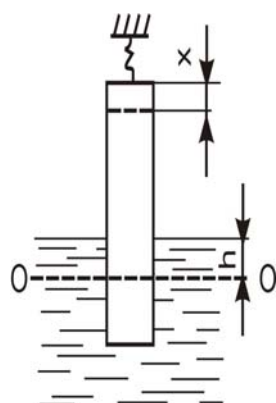
5.4 – расм. Ўзгарувчан ботишли цилиндрик қалқович силжишини
