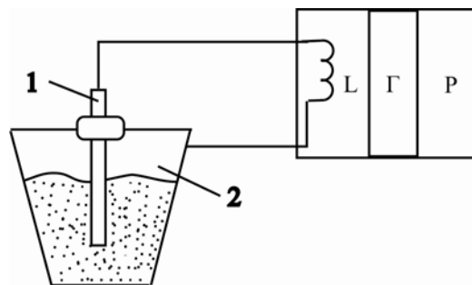
5.16 – расм. Сифимли сатҳ сигнализаторининг схемаси
