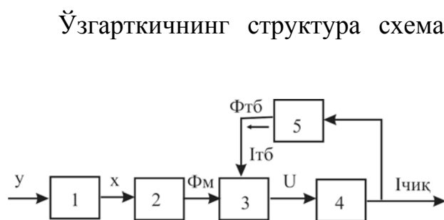
8.6 – расм. Ўзгарткичнинг магнит компенсацияли структурали схемаси.
