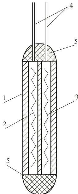
2.14 – расм. Платинали қаршилик термометрининг соғир элемент
