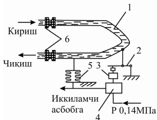
6.34-расм. Пневматик ўзгарткичи вазнли зичлик ўлчагичнинг схемаси
