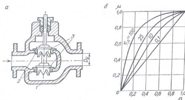
20.4-расм. Икки эгарли ростлаш клапани. а-конструктив схемаси; б-сарф тавсифи ( \xi_{\pi o}=5\text{у/н} ).
