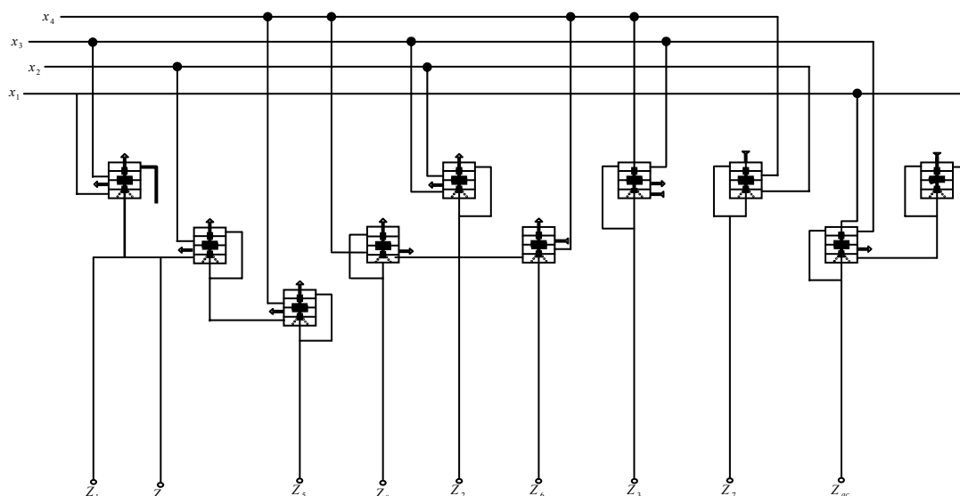
19.12-расм. Кўп функционал \Pi P.3 мантикий элемент асосидаги комбинацион автоматнинг принципл схемаси.
