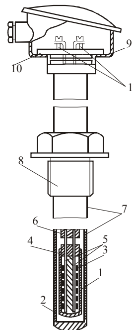
2.15 – расм. Қаршилик термометрин
