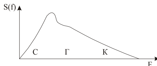
4.18 – расм. Ўлчаш ўзгарткичи датчиги сигнаlining ўзига хос частота спектри.
