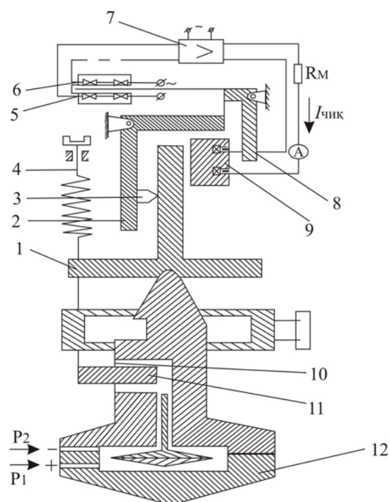
3.6 – расм. Юмшоқ мембранали дифманометрнинг
