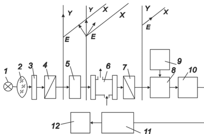
6.29 – расм. Автоматик поляриметрнинг схемаси.
