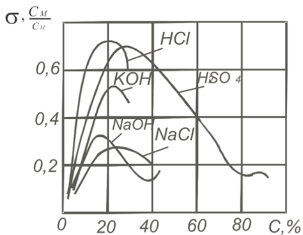
6.17 – расм. 18 0 С температурада баъзи моддаларнинг сувдаги эритмаларининг солиштирама электр ўтказувчанлигининг улар
