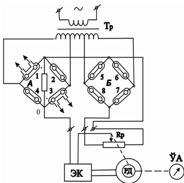
6.2 – расм. ТП туридаги автоматик газ таҳсилаторининг схемаси.
