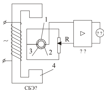
4.8 – расм. Ўзгарувчан магнит майдонли индукцион сарф
