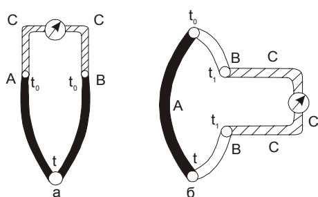
2.3 –расм. Учинчи ўтказгич(ўлчаш асбоби)ни термодуфт
