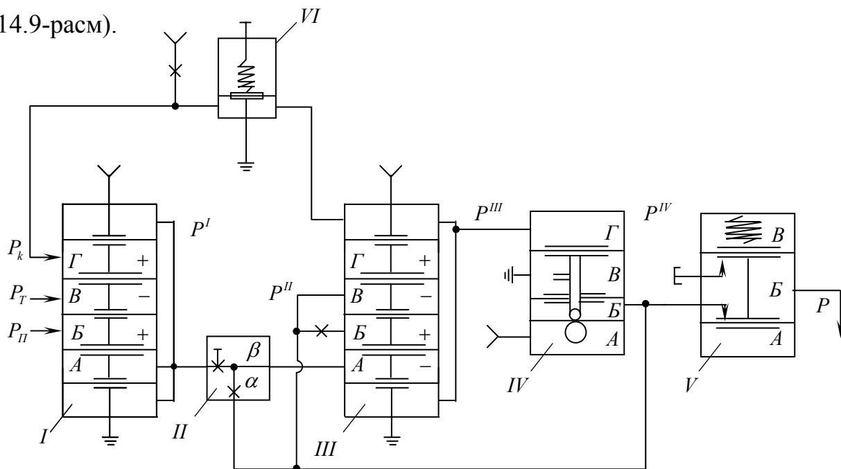
14.9-расм ПР2.5 мутаносиб ростлагичнинг принциал схемаси.
