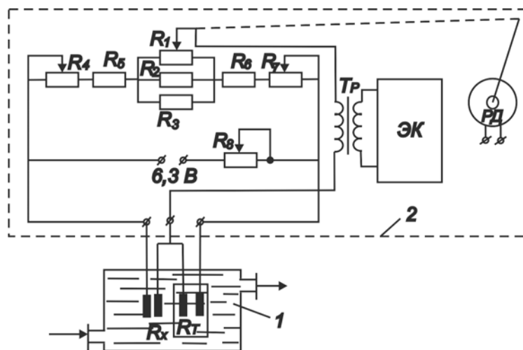
6.20-расм. Сульфат кислота концентратомерининг принципиал схемаси.
