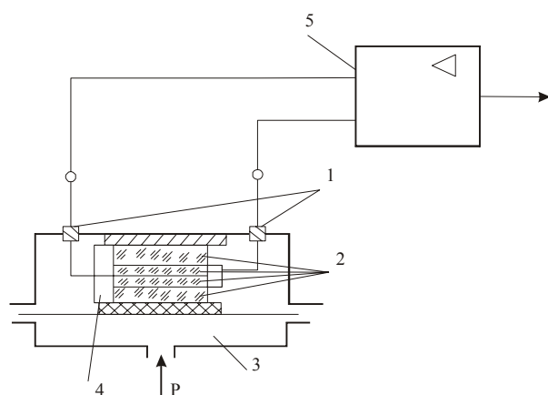
3.10 – расм. Пьезоэлектрик
