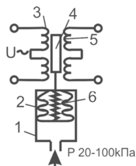
8.14 – расм. Пневмо – электрик ўзгарткичнинг принципаал схемаси.
