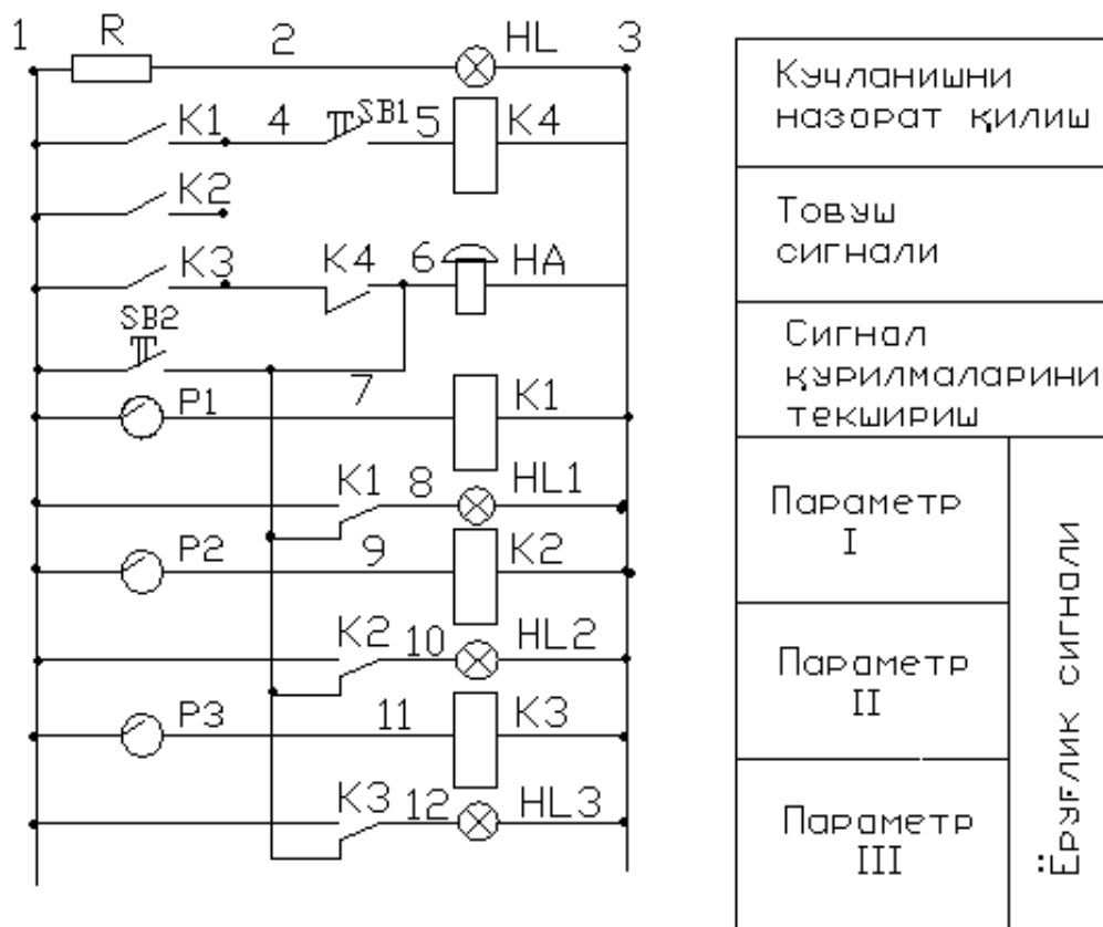
21.11-рasm. Технологик сигнализациянинг принципиал электр схемаси.
