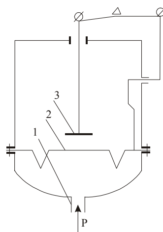
3.8 — расм. Сифимли
