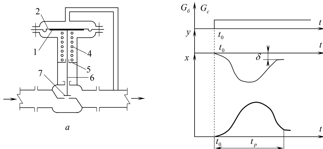
14.5-расм. Бевосита таъсир қилувчи статик босим ростлагичнинг принципал схемаси (а) ва унинг вақт характеристикаси (б).
