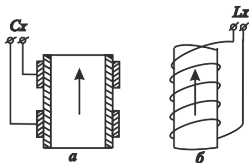
6.22-расм. Контактсиз юқори частотали кондуктометрнинг ўзгарткичлари:
