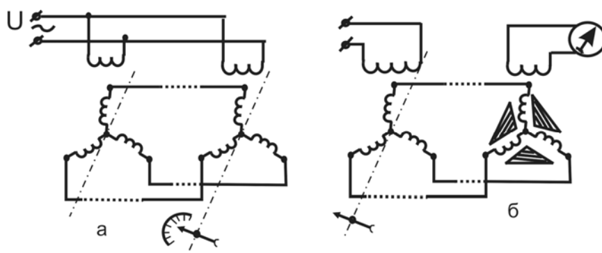
8.8 – расм. Сельсинли масофага узатиш тизимининг принцинал схемаси:
