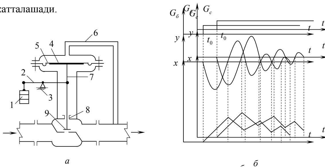
14.6-расм. Бевосита таъсир қилувчи астатик босим ростлагичнинг принципиал схемаси (а) ва унинг вақт характеристикаси (б).
