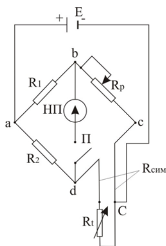
2.18 – рasm. Уч симли улаш схемаси.
