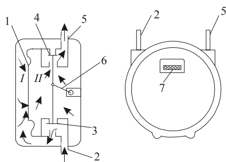
4.12 – расм. ГФК туридаги газ ҳисоблагич
