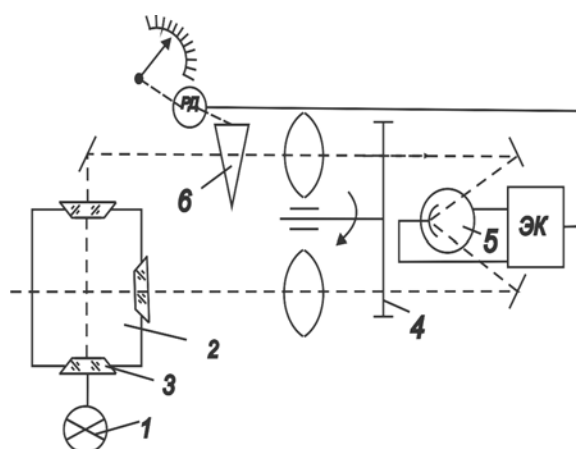
6.28 – расм. Нефелометрнинг принципаал схемаси.
