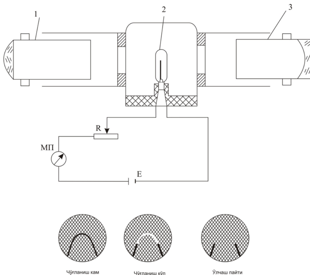
2.24 – расм. Оптик пирометрнинг принципиал схемаси
