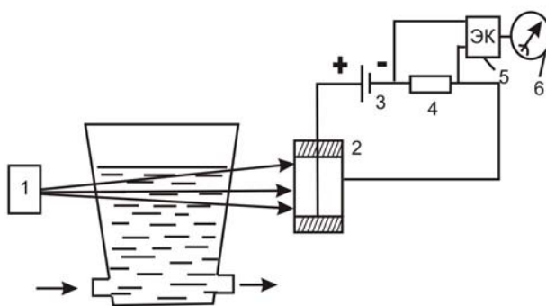
5.12 – расм. Радиоизотопли сатҳ ўлчагичнинг принципиал схемаси.
