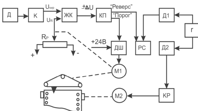
8.16 – расм. РП 160 иккиламчи асбобнинг структура
