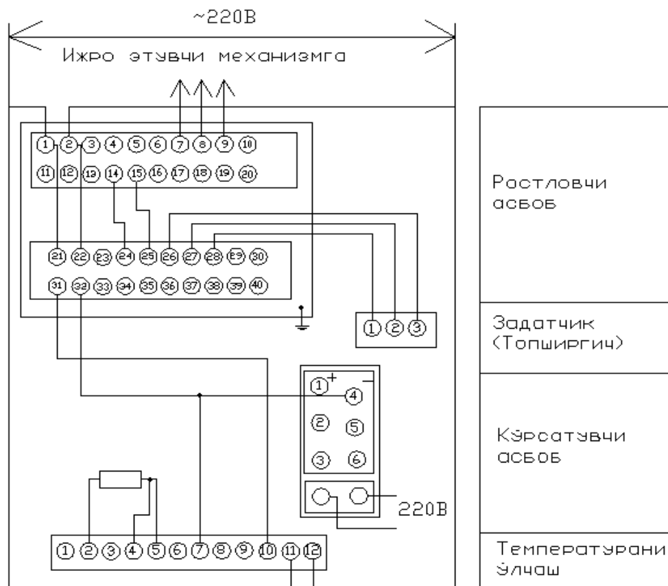
21.12-расм. Назорат ва ростлаш тизимларининг принцинал электр схемаси.
