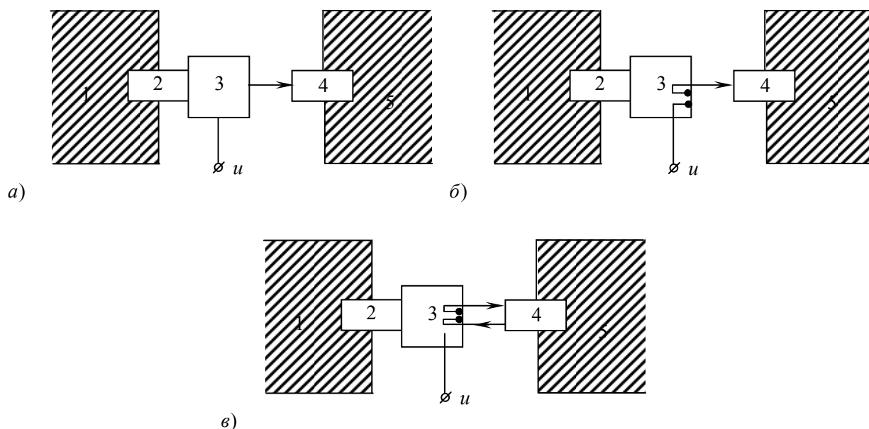
15.1-расм. Контактсиз ва контактли датчикларнинг тизим билан боғланиш схемалари.
