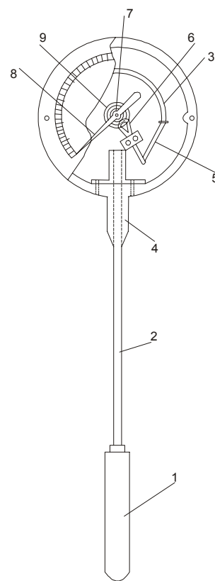
2.1 – расм. Манометрик
