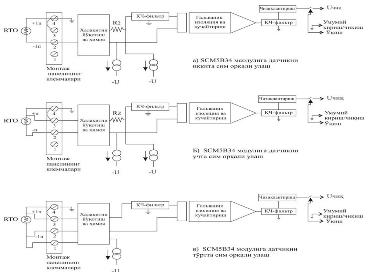
2.28 – расм. Датчикнинг SCM5B35 модулига улаш вариантлари
