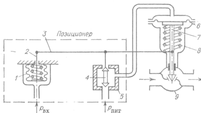
20. 2 расм. Позиционер
