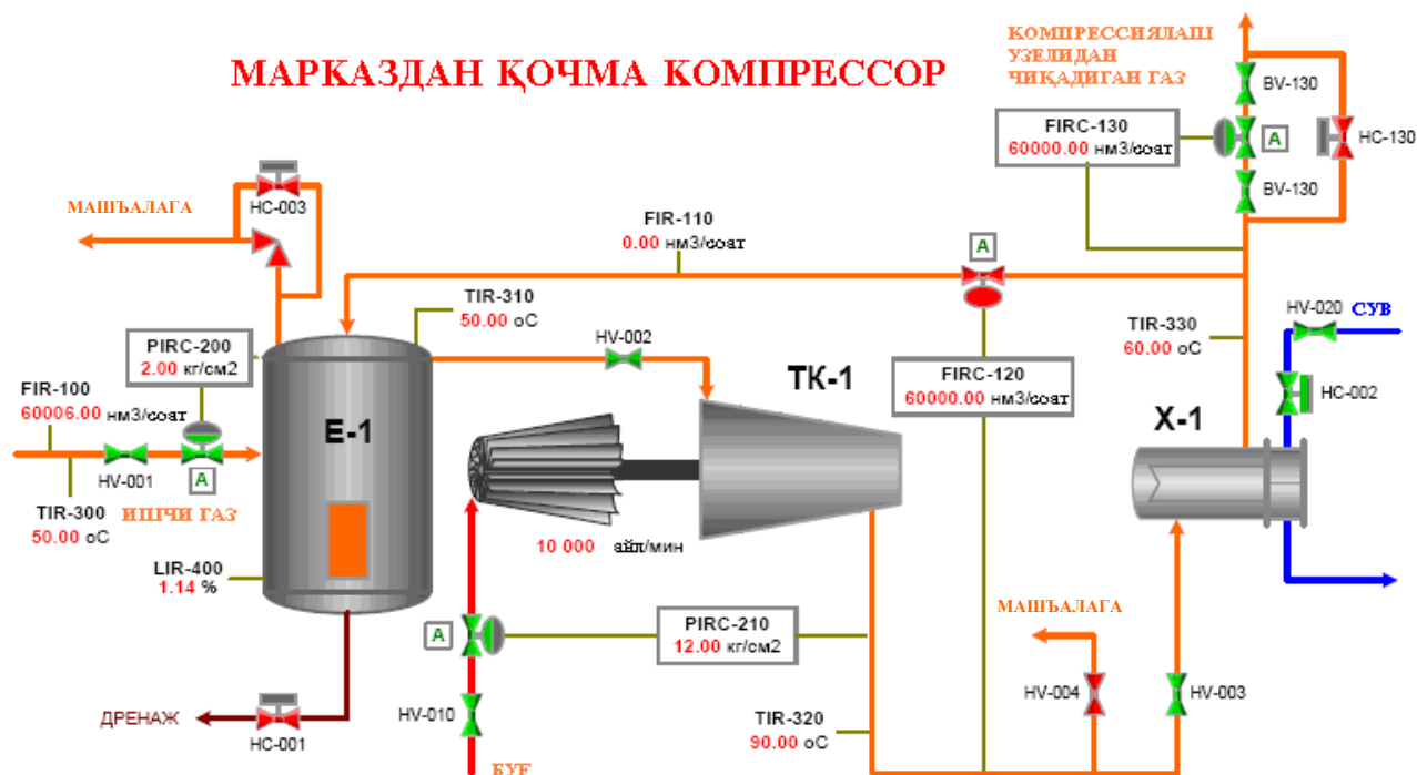
22.1-рasm. Компрессиялаш узели схемаси.
