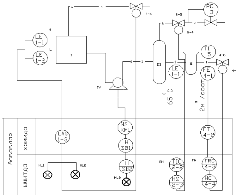
22.4- расм. Технологик жараённи автоматлаштириш схемаси.
