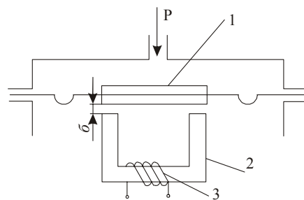
3.7 – расм. Индуктив манометр схемаси
