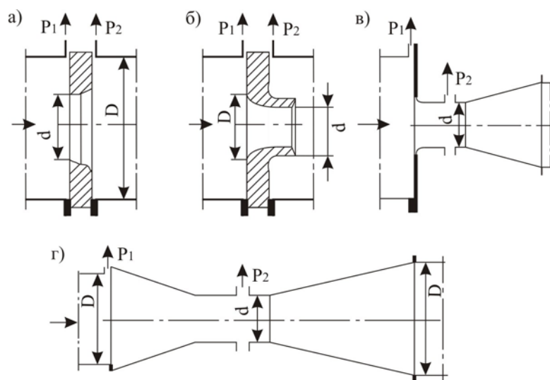
4.1 расм. Стандарт торайтирувчи қурилмалар схемаси: а – диафрагма, б – сопло, в – Вентури соплоси, г – Вентури кувури.
