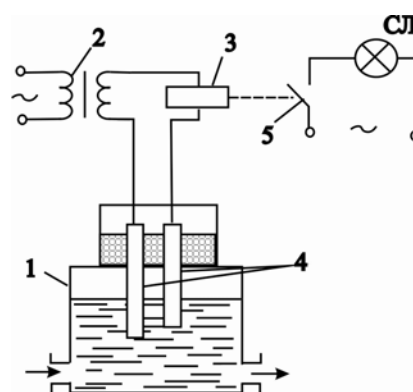
5.11 – расм. Сатҳ сигнализаторининг схемаси
