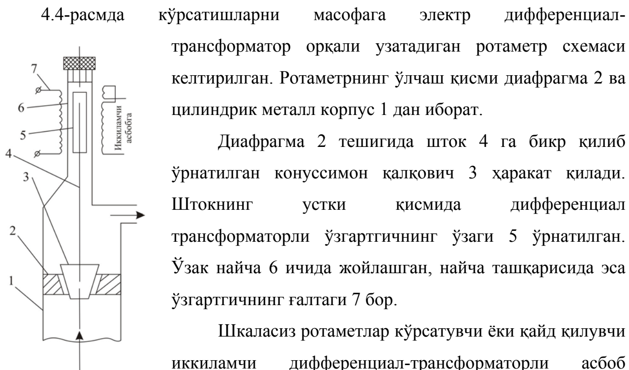
4.4 – расм. Кўрсатишларни масофага электр дифференциал – трансформатор
