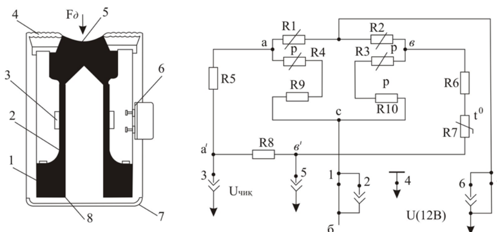
4.16 – расм. ДЕДВУ тензорезисторли ўзгарткичнинг схемаси:
