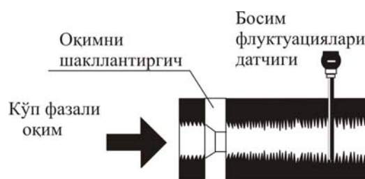
4.17 – расм. Оқим ўлчаш ўсули
