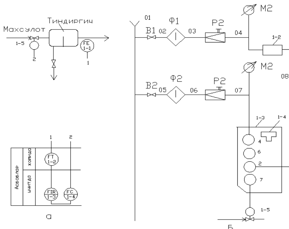
21.13-расм. Суюқ маҳсулот сарфини ростлаш схемаси:
