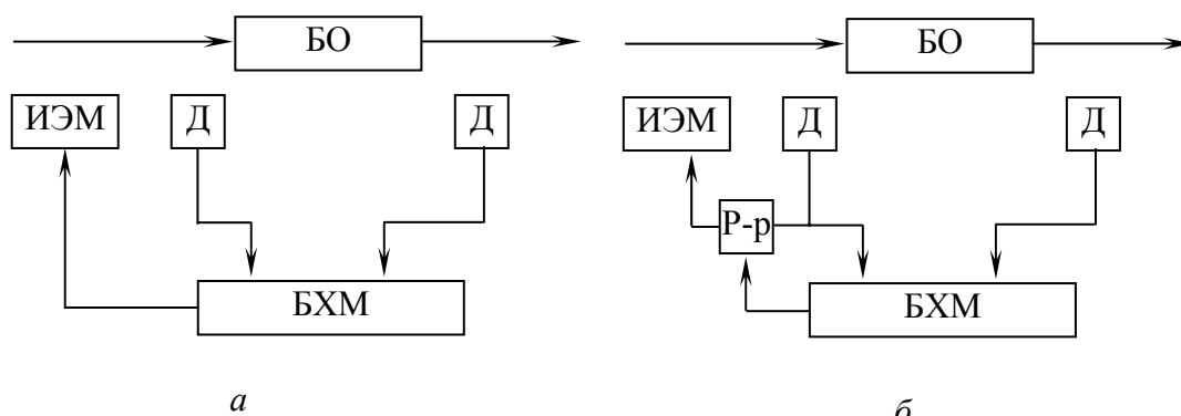
17.2-расм. Автоматлаштирилган бошқаришни марказлаштиришнинг турли даражаларига мисол.
