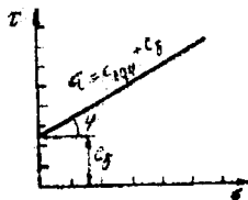
2.5-rasm. Qattiq loylarni siljishga sinash
