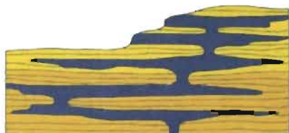
105-расм. Кўп ярусли силлар.
