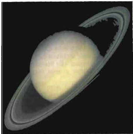
12-расм. Сатурн атрофидаги ҳалқалар тизими. www.gafspace.spb.ru .
