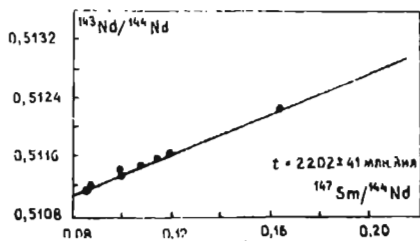
43-расм. Асосли таркибли дайдалар учун самарий-неодимийли эволюцион диаграмма.
