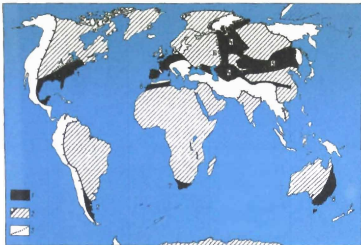
214-расм. Герцинидларнинг ҳозираи структурада тутган ўрни. 1-эпигерцин платформалари: 1-Аппалача, 2-Жанубий Америка, 3-Ғарбий Европа, 4-Урол-тиёношон, 5-Мугул-Охота, 6-Шимолий Африка, 7-Жанубий Африка, 8-Шарқий Австралия; 2-олдинги консолидация вилоятлари; 3-олд ботиқликлар: А-Аппалачиолди, Б-Урололди.
