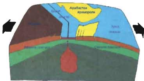
57-расм. Қизил денгиз рифтимина ривожланиши.
