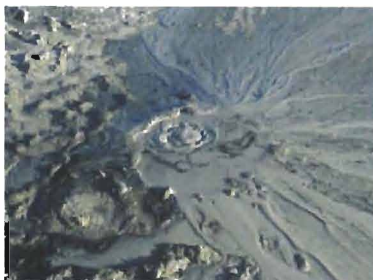
98-расм. Балчиқ вулкан кратери. http://travel.gala.net
