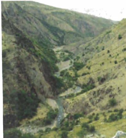
128- расм. Асимметрик дарё водийси.
