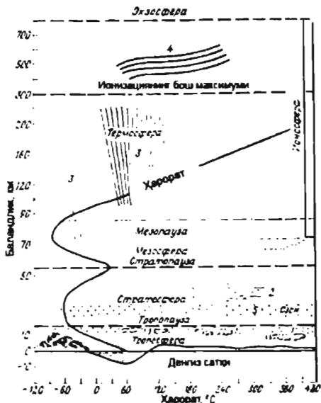
20-рasm. Атмосферанинг вертикал кесмаси.
