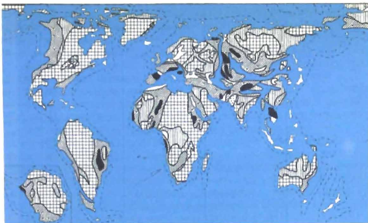
197-расм. Кечки рифейина ҳозирги географик асосдаги палеогеографик элементлари. Шартли белгилар 196-расмда берилган.
