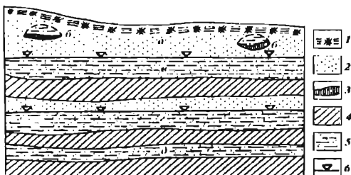
137-расм. Ер пўстида турли ерости суварларининг жойлашиш схемаси: а - сизот суварлари; б - верховодка; в - грунт суварлари; г, д - қатлам суварлари; 1 - тупроқ-ўсимлик қатлами; 2 - сув ўтказувчи қатлам; 3 - ярим сув ўтказувчи жинслар; 4 - сув ўтказмайдиган қатлам; 5 - гравитацион сув; 6 - грунт суварларининг сатҳи.
