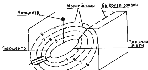
62-расм. Зилзила ўчоғининг тузилиш схемаси.
