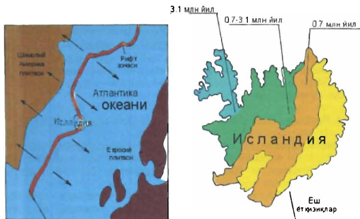
61-расм. Литосфера плиталарининг ҳаракат тезлиги.
