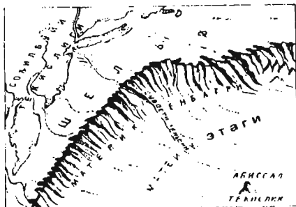
165-расм. Пассив континент чет элементлари.
