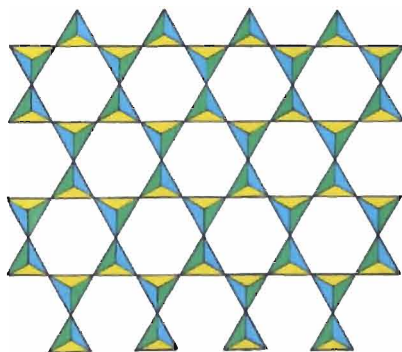
27-расм. Варақли силикатларнинг тузилиши.
