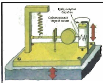
64-расм. Вертикал табранишларни қайд этувчи сейсмограф.
