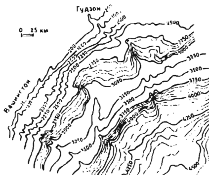
166-расм. Континент ёнбагининг топографияси.
