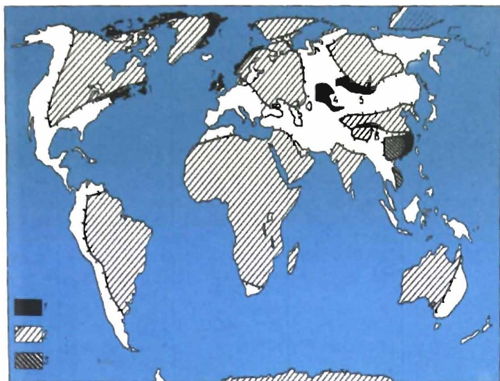
204-расм. Каледонидларнинг ҳозираги структурада тугъан ўрни. 1-эпикаледон платформалари: 1-Шимолий Гренландия, 2-Грампиан, 3-Иннуит, 4-Марказий Қозоғистон, 6-Наньшан, 7-Катоси, 2-илгари консолидацияланган вилоятлар, 3-қадимий Хитой платформасининг парчаланган палахсалари.
