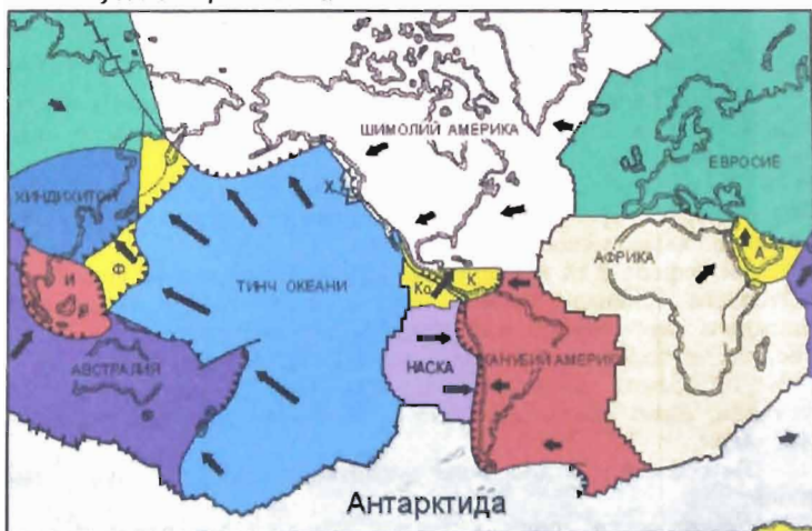
58-расм. Литосфера плиталарининг ўзаро жойлашува схемаси. 1-трансформали ер ёриқлари, 2-субдукция зоналари, 3-материклар чегаралари, литосфера плиталарининг ҳаракат йўналиши.
