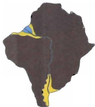
225-расм. Шарқий ва Ғарбий Гондвананинг ажрalliши.
