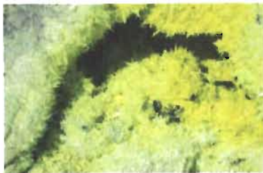
79-расм. Кратерда ҳосил бўлган олтингузурт кристаллари. www.ekosistema.ru
