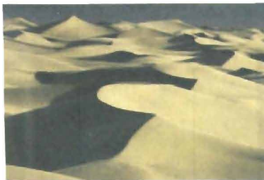
121-рasm. Саҳродаги барханлар.
