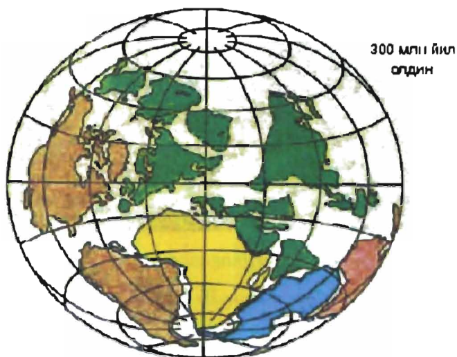
213- расм. Карбон даврида литосфера плиталарининг тутган ўрни.
