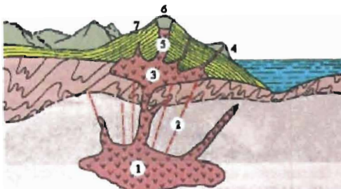
73-расм. Вулкан қурилмасининг тузилиши.
