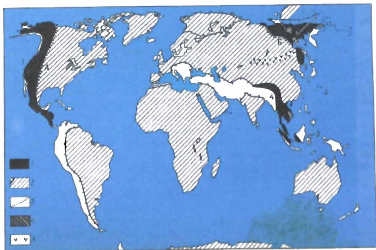
226-расм. Мезозойларнинг ҳозирги структурада тугаган ўрни. 1-платформалар: 1-Кордильера, 2-Верхоян-Калм, 3-Узоқ Шарқ, 4-Ҳиндихитой; 2- олдинаи консолидация вилоятлари; 3-олд ботиқликлар: А-Кордильераолди, Б-Верхоянолди; оралиқ массивлар – мезозойлар орасидаги барқарор вилоятлар: а-Колима, б-Омолон, в-Охота, г-Шарқий Чукотка, д-Ҳиндосиний; 5-Муғул-Охота қамбари.
