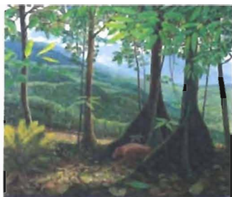
246-расм. Палеоген ладшафти. http://wwlife.ru
