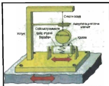
63-расм. Гризонтал табранишларни қайд этувчи сейсмограф.
