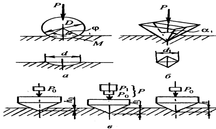
7.4-rasm. Qattiqlikni sinash usullari sxemalari. a-Brinell usuli, b-Vikkers usuli, v-Rokvell usuli.
