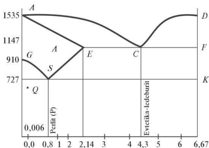
5.8-rasm Temir — uglerod qotishmalarining holat diagrammasi.
