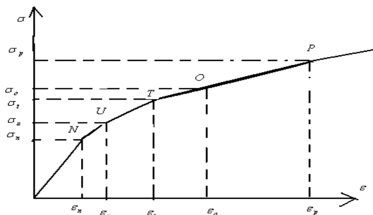
7.1-rasm. Nisbiy uzayishni deformatsiya \varepsilon
