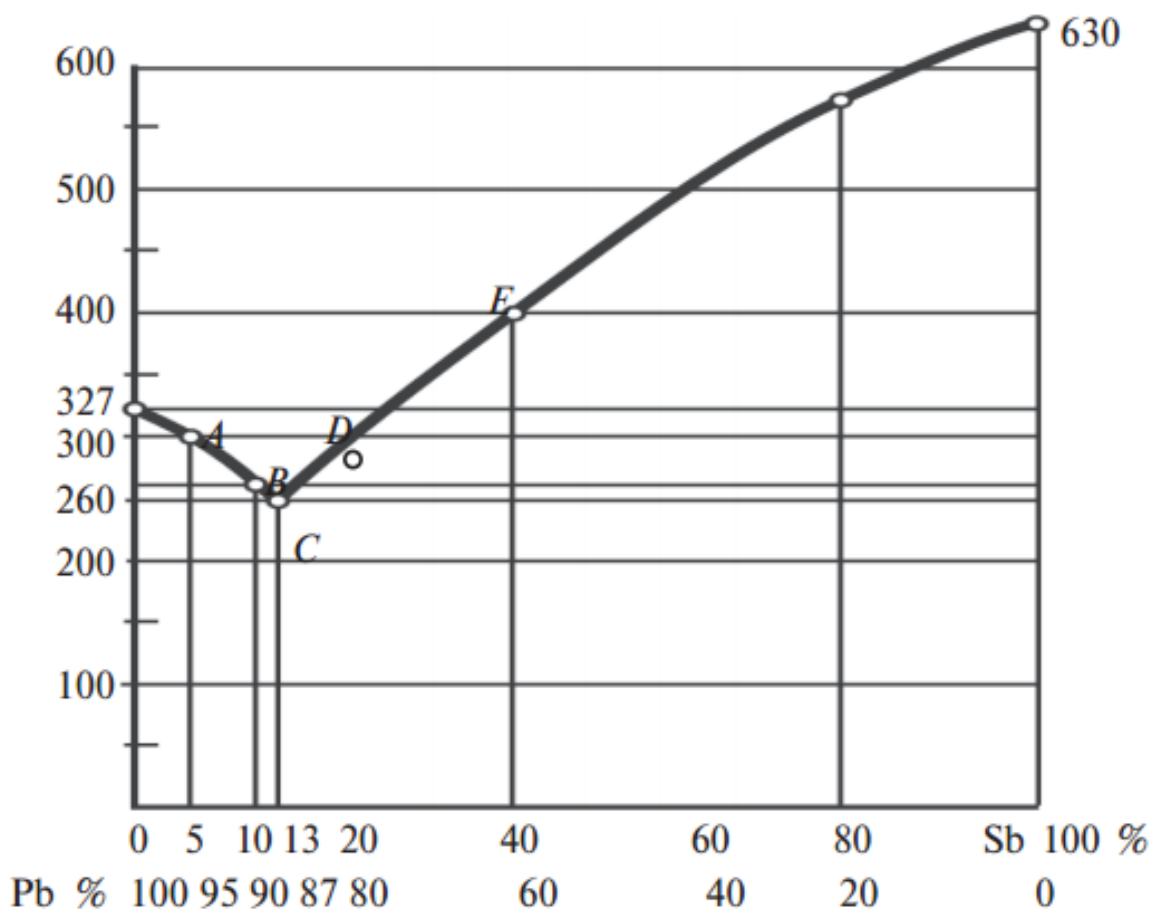
5.6-rasm. Qotishmalarning holat diagrammasi.
