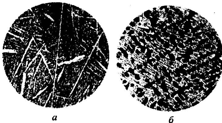
12.1-rasm. Qayta ishlanuvchi oq cho'yan mikrostrukturasi (x200). a) – evtektikadan keyingi oq cho'yan ( S=5,5\% ); b) – evtektikagachadagi oq cho'yan ( S=2,5\% ). Rasmdagi qora ranglilari bu perlit; oq ranglilari ledeburit.
