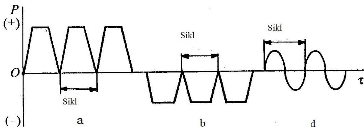
1.2- rasm. Siklik yuklama sxemasi.
