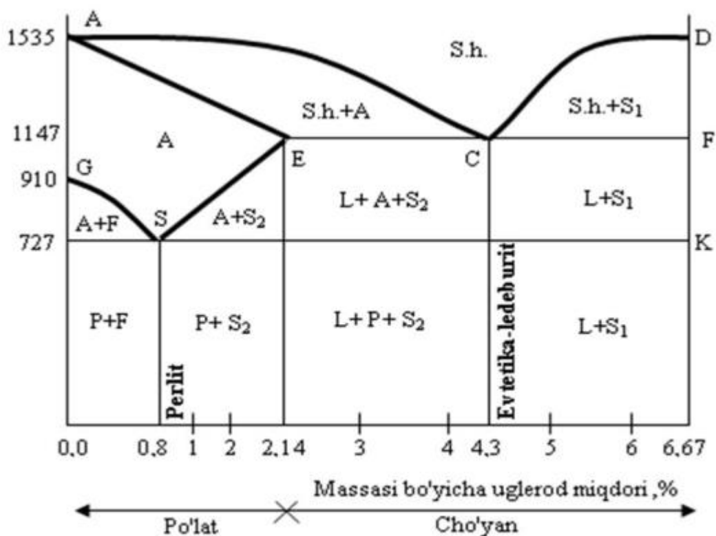
Temir-uglerod qotishmalarining holat diagrammasi
