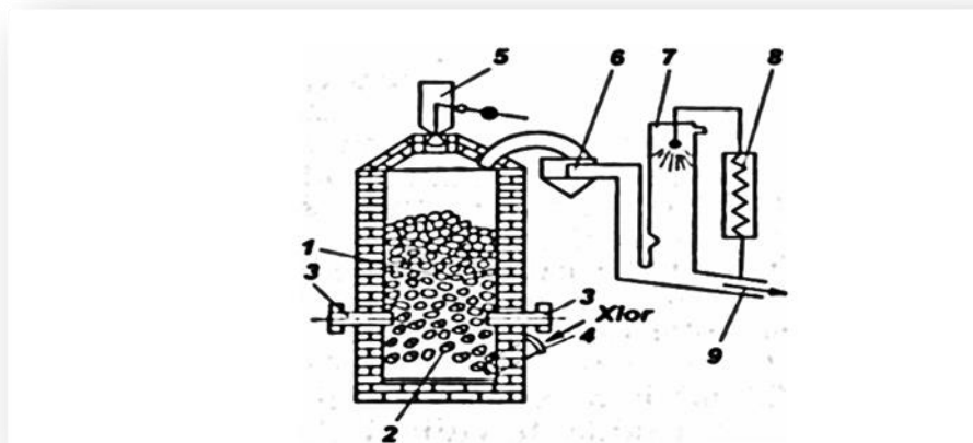
13.6-rasm. Rutil briketlariga xlor bilan ishlov berish qurilmasining sxemasi. 1-rutil briketlari; 2-qarshilik elementlari; 3-elektrodlar; 4-trubka; 5-bunker; 6-chang yutgich; 7-kondensat; 8-sovutgich(chapda).
