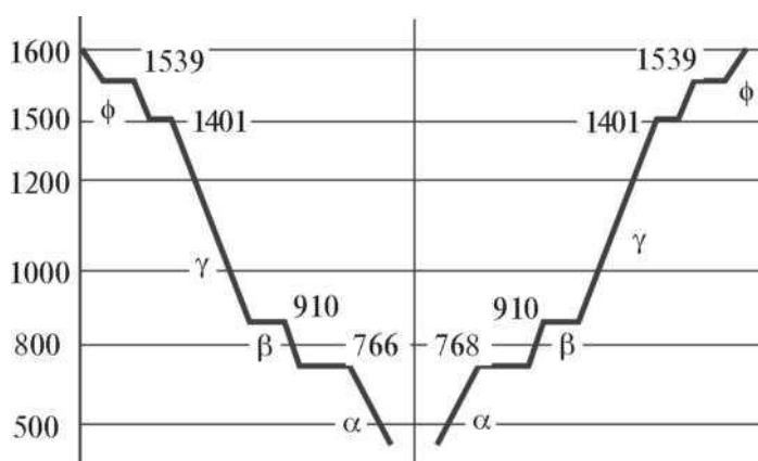
5.7-rasm Temirning sovish va erish grafigi.
