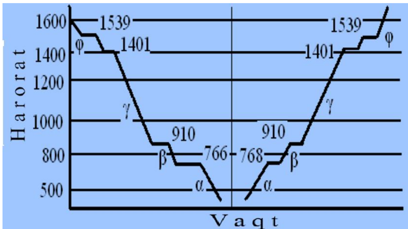
8.1rasm. Temirning sovish va erish grafigi
