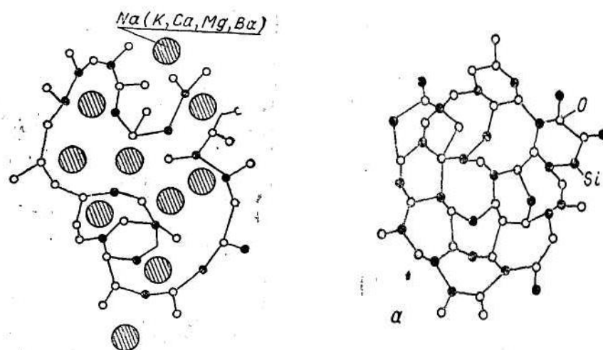
14.2-rasm. Anorganik shishalarning strukturasi:
