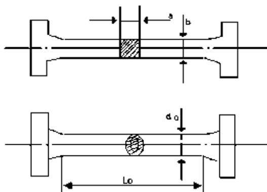
6.7-rasm. Tajriba uchun ishlatiladigan namunalarning sxematik tuzilishi
