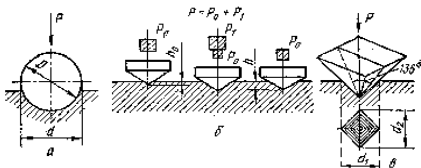
6.10-rasm. Qattiqlikni o'lchash: a) Brinel usuli b) Rokvell usuli v) Vickers usuli
