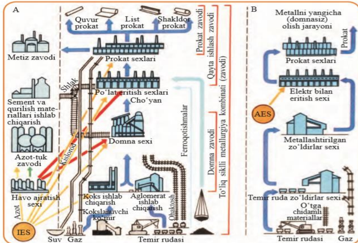
6-rasm. Metallurgiya kombinatidagi sexlar sxemasi
