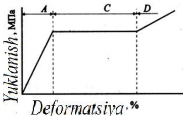
16.9-rasm. Kristallik polimerni choʻzish diagrammasi.
