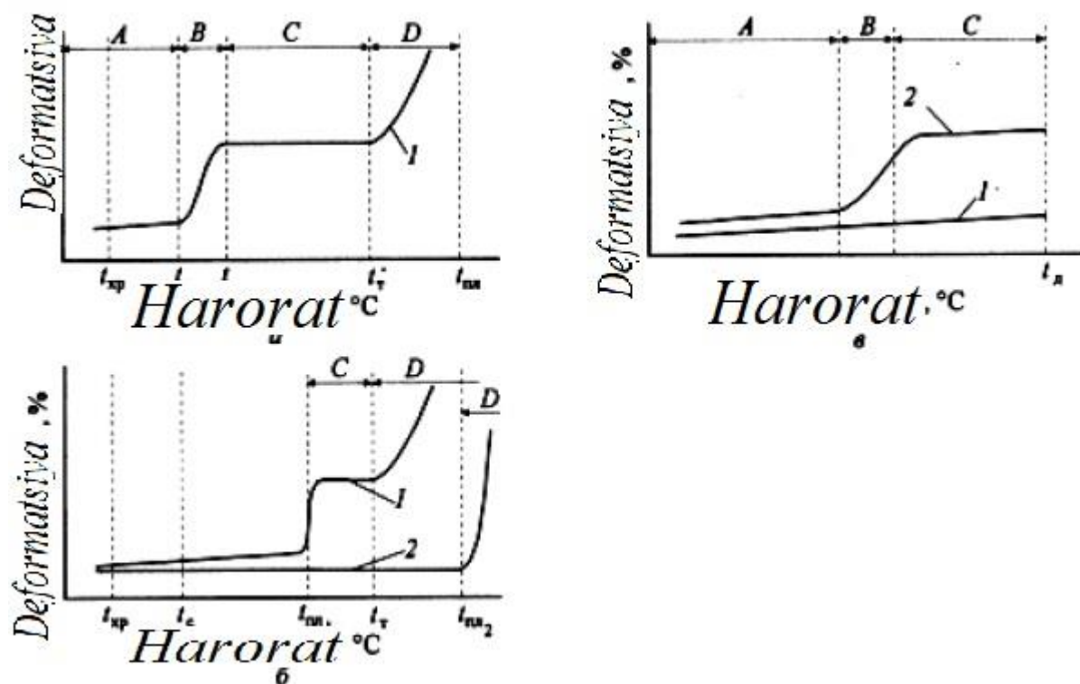
16.7-rasm. Termomexanik grafiklar:
