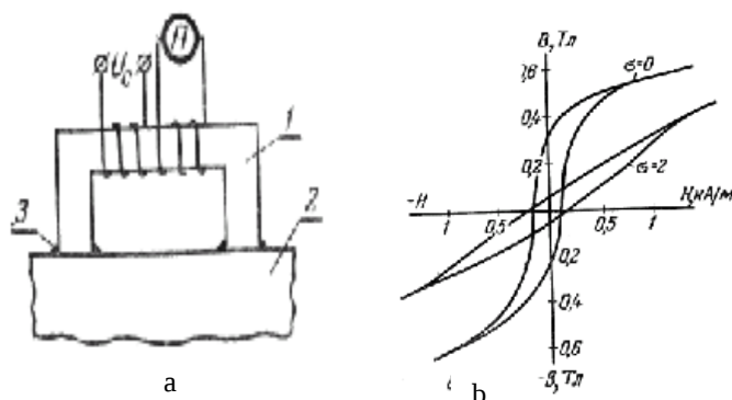
2.8- rasm. Magnitoelastikli datchikning sxemasi va tavsifnomasi.
