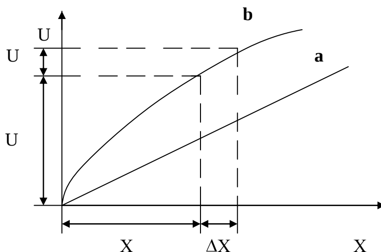
2.2-rasm. Datchiklarning statik tavsifnomalari.
