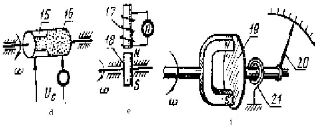
2.22-rasm. Elektrik tezlik datchiklari.
