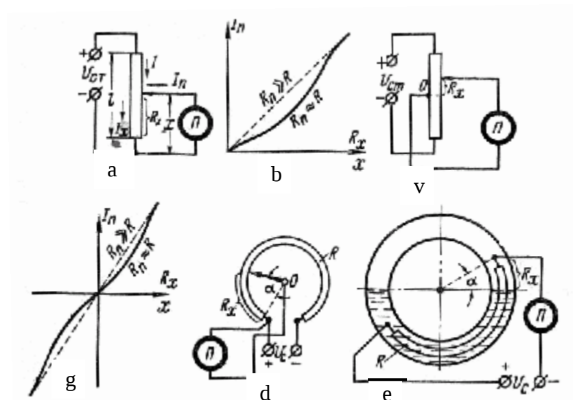
2.3-rasm. Potensiometrik datchiklar va ularning tavsifnomalari.
