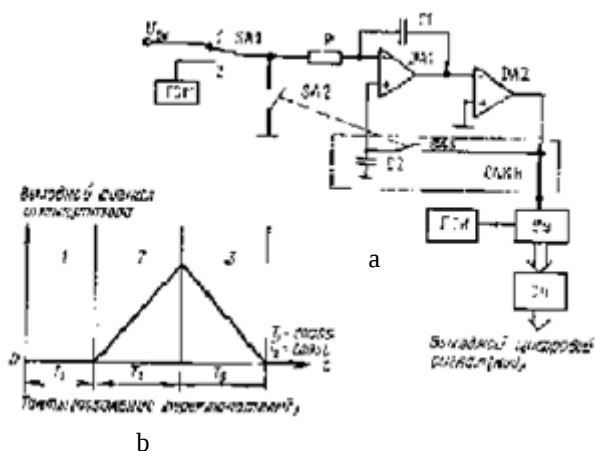
5.5.- rasm. Ikki qiyalik integrallash ARU si.
