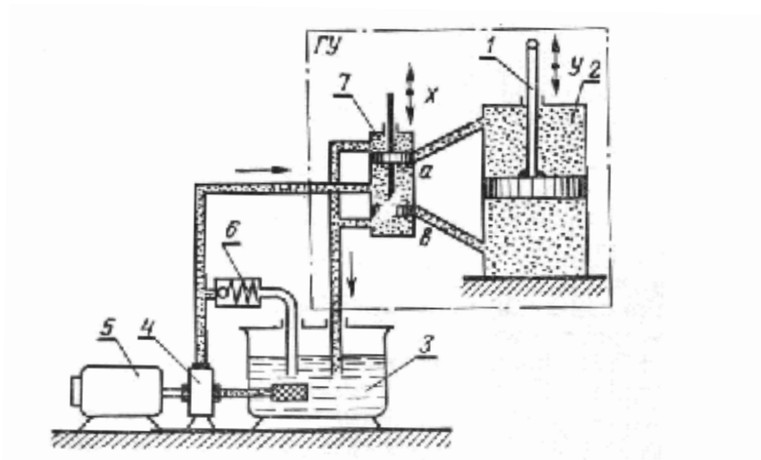
6.9 -rasm. Zolotnikli gidravlik kuchaytirgichning sxemasi va uning statik tavsifnomasi.
