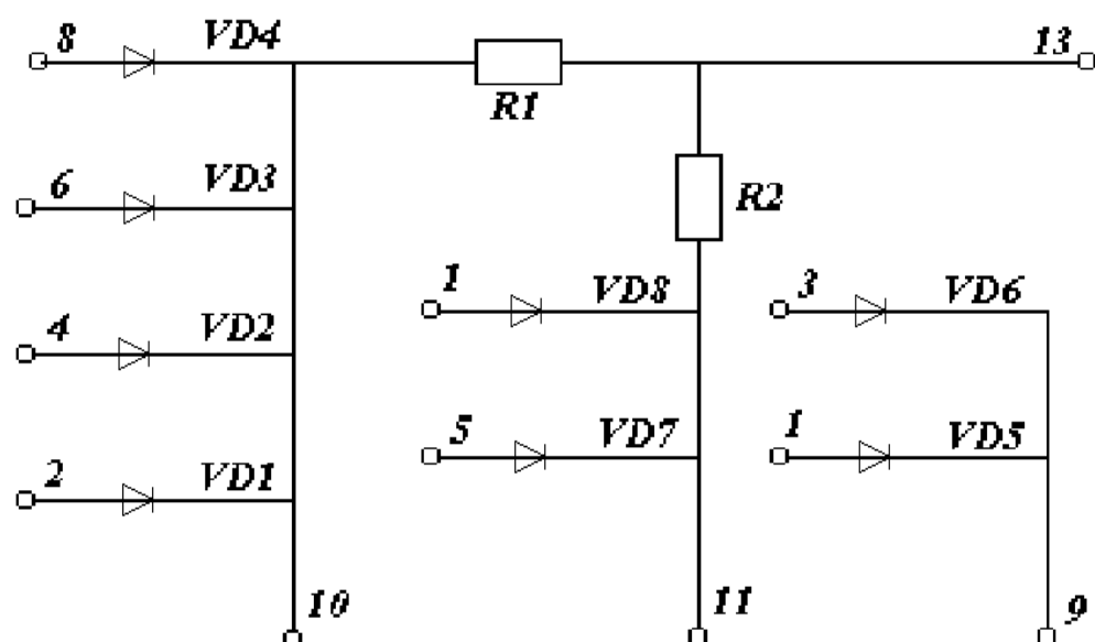
4.12-расм. T-107 rusumli yarim o'tkazgichli mantiy elementning sxemasi.
