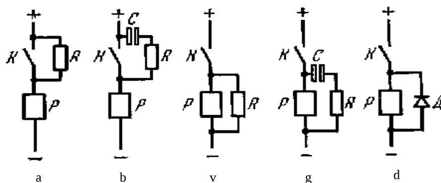
3.2.-rasm. Rele kontaktlari ishini yengillashtiruvchi sxemalar.
