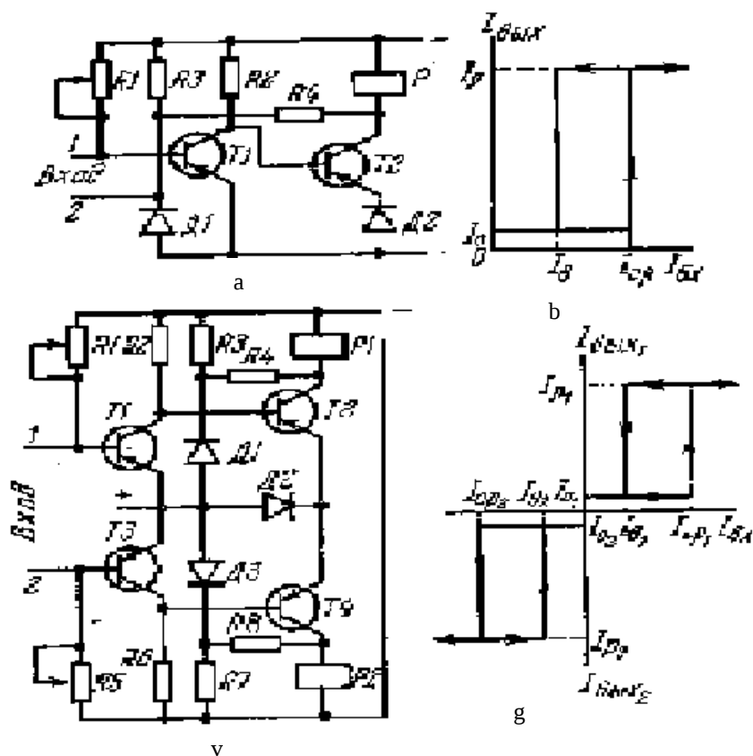
5.2-rasm. Nol-indikatorli taqqoslash elementining sxemalari va xarakteristikalari
