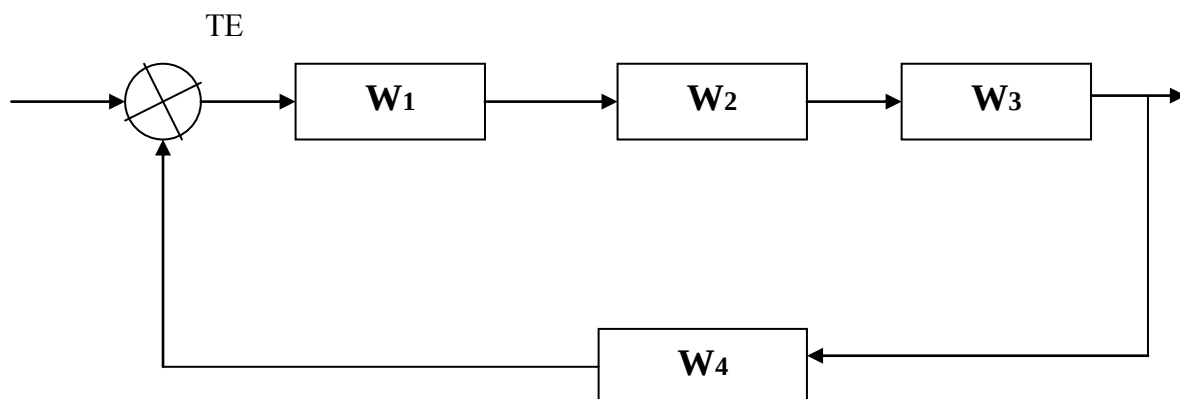
1.4. - rasm. Avtomatikaning strukturaviy sxemasi.
