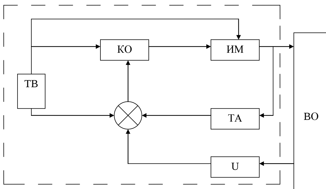
8.1-rasmd. Xaroratni avtomatik rostlagichlarning funktsional-strukturabiy sxemasi: BO-boshqarish ob'ekti, U-uzgartirgich (xarorat datchigi), TO-taqqoslash va topshirish organi, TA-teskari aloqa, KO-kuchaytirish organi, IM-Ijro mehanizmi, TB-ta'minot bloki
