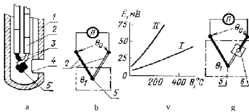
2.33-rasm. Termoelektrik termometrning prinsipial sxemasi.
