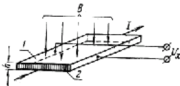
2.9- rasm. Xoll elementining sxemasi.
