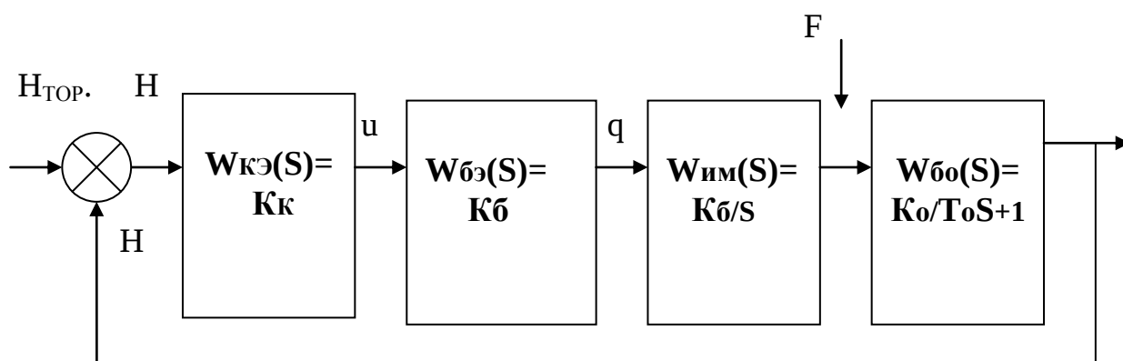
1.5 - rasm. Xaydov chuqurligini avtomatik rostlashning strukturaviy sxemasi.
