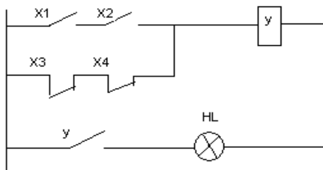
Rele ekvivalent sxemasi
