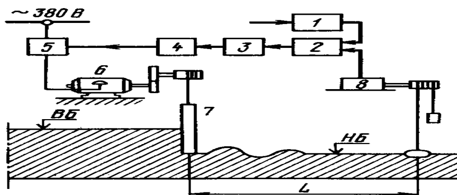
8.6. – rasm. Suvni satxi pastki bef bo'yicha stabillovchi regulyatorning tartibiy sxemasi.
