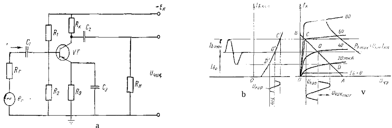
6.3- rasm. Umumiy emmitterli (UE) kuchaytirish kaskadining sxemasi.
