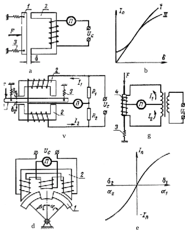
2.6- rasm. Induktiv va transformator datchiklarining sxemalari va ularning tavsifnomalari
