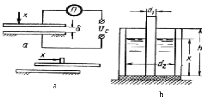
2.10- rasm. Sig'im datchiklarining turlari.
