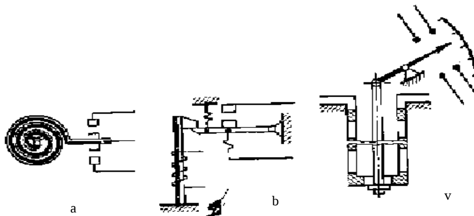
2.13-rasm. Dilatometrik va bimetallik datchiklarning sxemalari.
