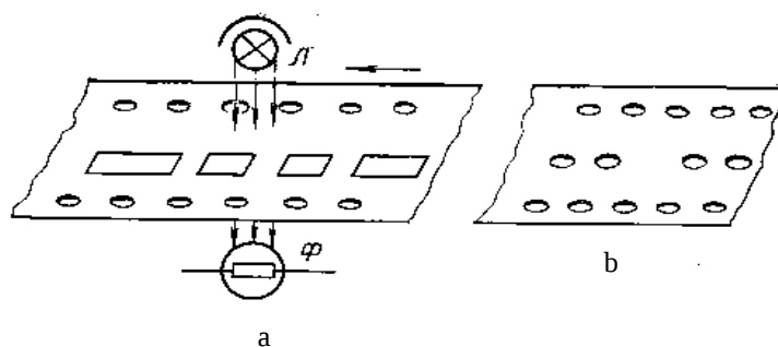
5.3.-rasm. Perforatsiyalangan lenta
