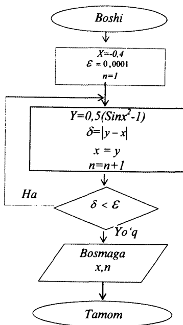
10-rasm. Iteratsiya metodi blok-sxemasini.
