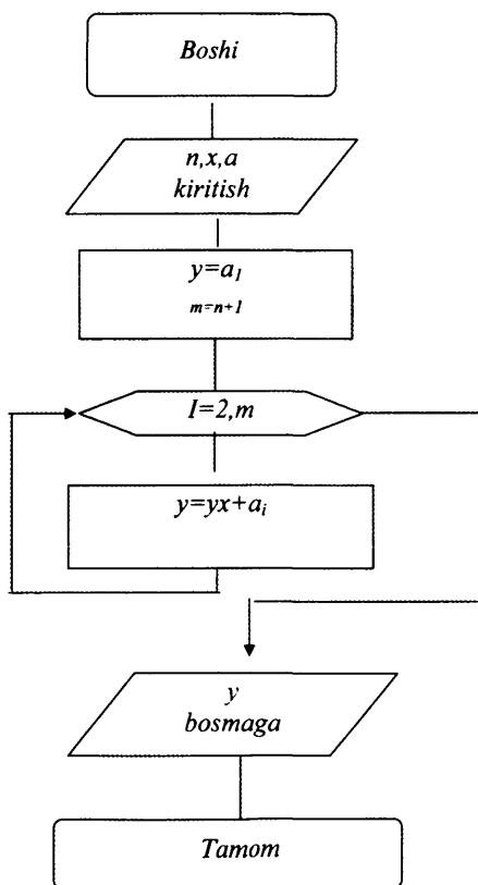
18-rasm. Gornier sxemasi yordamida hisoblash algoritmining blok-sxemasi.
