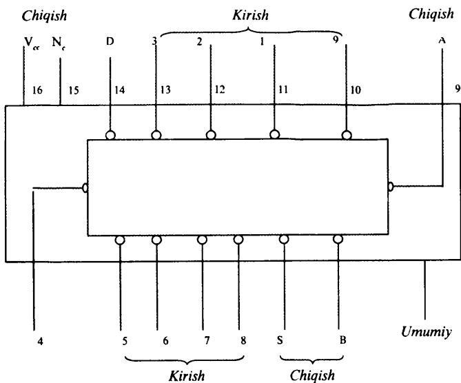
6-rasm. 74147 shifratorning ulash sxemasi.
