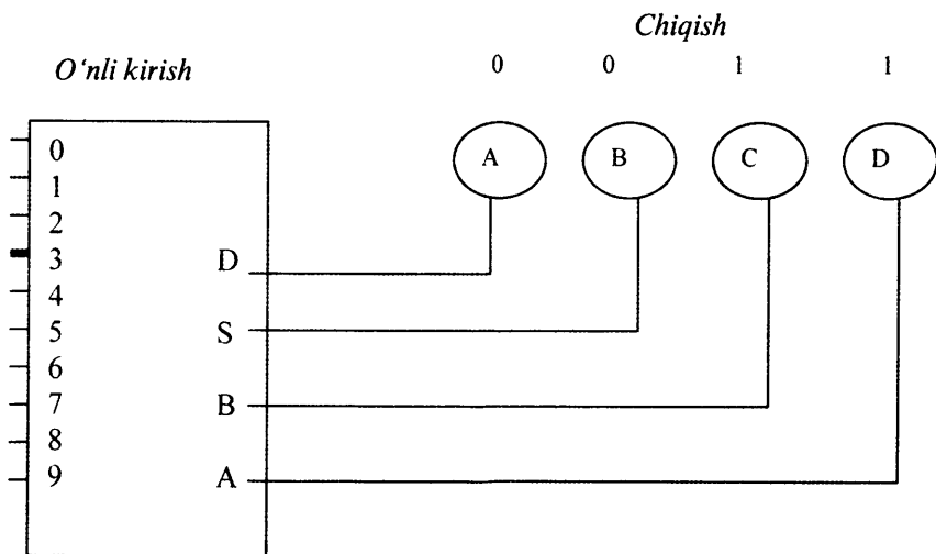
5-rasm. 10 kirishli, 4 chiqishli shifраторning blok-sxemasi.
