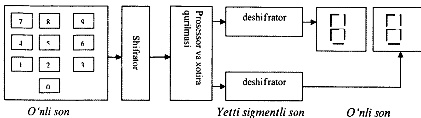
4-rasm. Shifратор qo'llaniladigan raqamli sistema.
