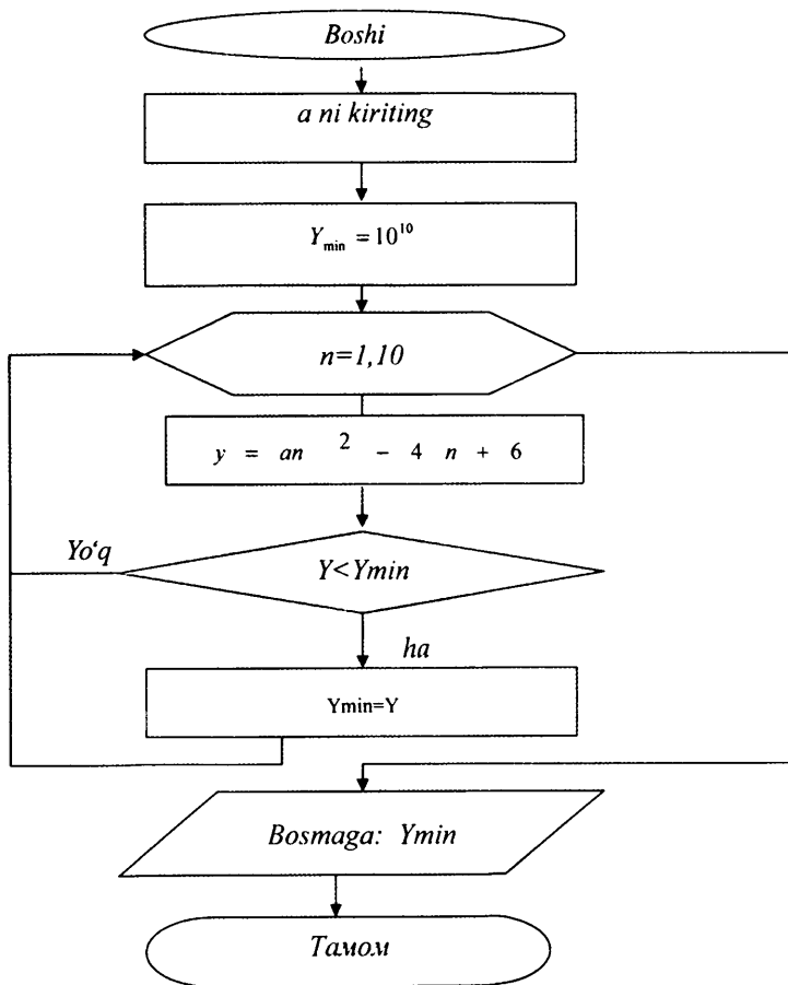
19-rasm. Funksiyaning eng kichik qiymatini topish blok-sxemasi.
