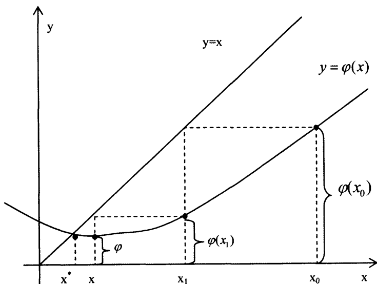
9-rasm. Iteratsiya metodining geometrik ma'nosi.
