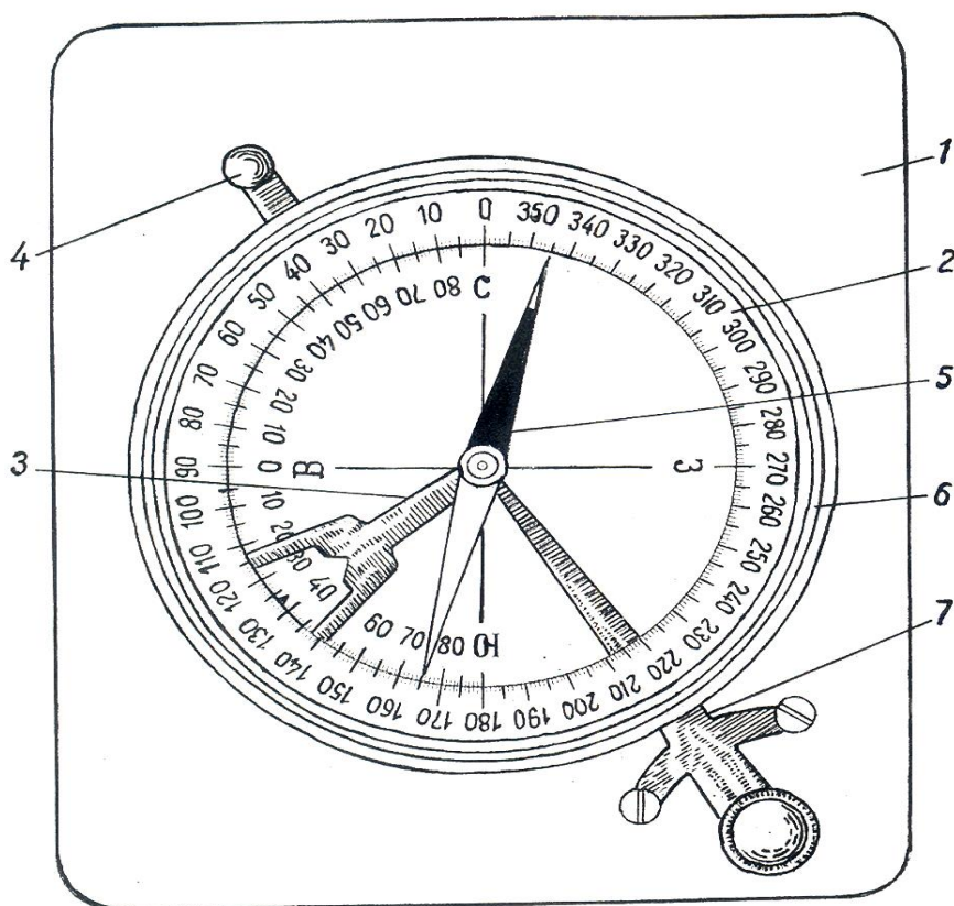
27-rasm. Tog' kompasi: 1-kompas asosi; 2-limbli kompas qutisi; 3-klinometr; 4-klinometrni mahkamlash mexanizmi; 5-magnit mili; 6-qoplovchi oynani tutib turuvchi prujina; 7-magnit milini mahkamlash mexanizmi.
