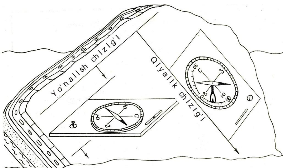
28-rasm. Yo'tish elementlarini tog' kompasi yordamida aniqlash
