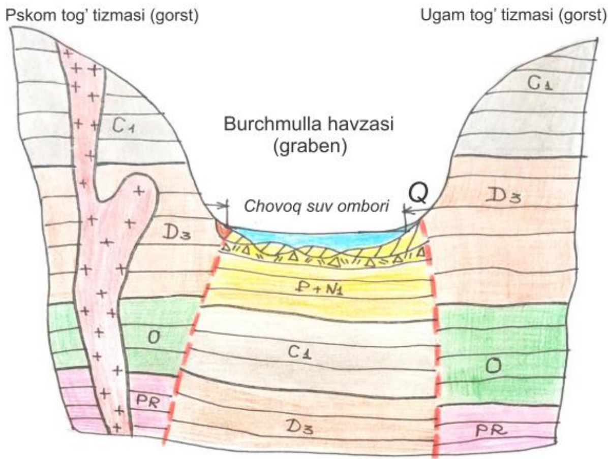
4-rasm. Hududning tektonikasi
