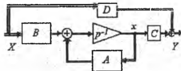
2.48-rasm. Obyekt modeling algoritmik sxemasi.
