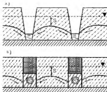
21.3-расм. Зовурларга ер ости сувини оқиб келиш жараёни (В.П.Анапьев, Л.В.Переделский-лар бўйича). А-очиқ зовур, Б-ёпиқ зовур
