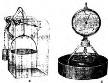
6.7-расм. Гил ва гилли жинслар ивувчанлигини (а) ва кўпчувчанлигини (б) аниқлаш асбобларининг умумий кўриниши
