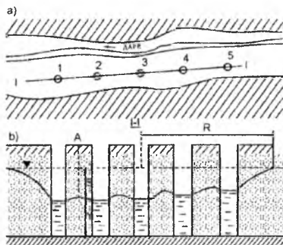
21.2-расм. Дарё водийси бўйлаб, бир нуналинида жойлаштирилган сув чиқариш қудукларининг ўзаро таъсир этиш чизмаси
