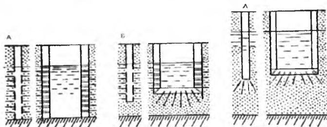
15.9-расм. Сув чиқариш иншоотлари грунт қудуклари ва шурфларининг умумий қўриғи. А-мукаммал қудуклар ва шурфлар, Б-тубидан ва ер томонларидан сувни ўтказиши мумкин бўлган номукаммал қудук ва шурфлар, Д-фақат туб томонидан сувни ўтказиши мумкин бўлган қудук ва шурфлар
