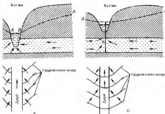
10.9-расм. Босимли сувларни ер усти сув хавзалари билан ўзаро алоқаси (У.Богомолов). а-босимли сувлар оқимининг дарё сувлари оқими бўйича таъминланиши; б-дарё сувлари оқимини босимли сувлар оқими билан таъминланиши; АА-пъезометрик юза
