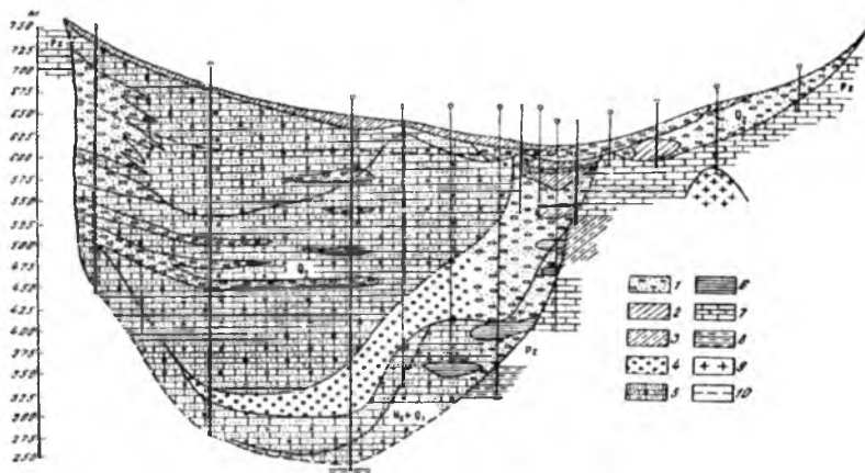
19.3-расм. Нурота марказий чўкмасининг (ботигининг) гидрогеологик кўндаланг кесмаси (В.А.Борисов ва С.Ш.Мирзаевлар буйича). 1-пагаллар, 2-суплиноклар (соз туپроқлар), 3-конгломератлар; 4-супеслар (қумоқ туپроқлар); 5-майда шағалли қумтошлар; 6-гитлар; 7-оҳақтошлар, 8-гилли сланецлар; 9-гранитлар; 10-грунт сувларининг сатҳи
