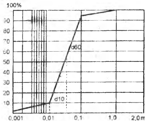
15.4-расм. Қум жинслари таъсир этувчи диаметрини (x) ( d_{10} ) аниқловчи гранулометрик таркиби эгри чизиги (Й.Э.Эргашевдан)
