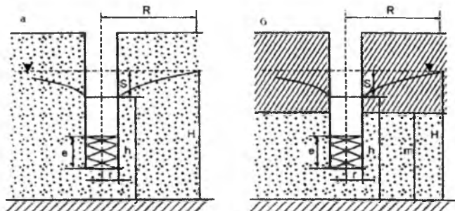
21.4-расм. Мўкаммал бўлмаган бурғу қудуқлари: а-босимсиз ер ости сувлари учун; б-босимли сувлар учун
