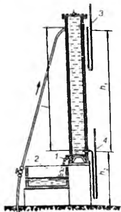
15.3-расм. Дарси қурilmасининг умумий кўрinishи
