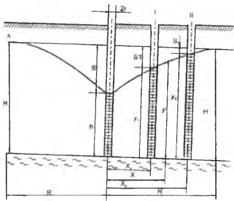
15.12-расм. Грунт қудуқларидан сувни сўриб олиш жараёнида сув сарфини (дебитини) аниқлаш схемаси (М.В.Седенқодан)
