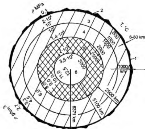
5.1-расм. Ер геосфералари ва уларнинг миқдори қийматлари (Ф.Ю.Зингель бўйича) 1-қобик (литосфера); 2-Мохорович юзаси; 3-юқори мантия; 4-мантия; 5-ташқи ядро; 6-ядро
