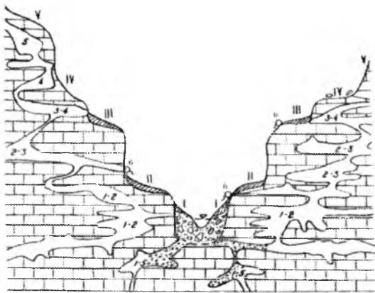
11.3-расм. Оҳақтош қатламларида карст бўшлиқларининг (горларининг) вужудга келиш чизмаси. I-V-тўртамчи давр мобайнида ҳосил бўлган «ювилган» ва «Цоколь» террасалар, 1-5-«ювилган» ва «Цоколь» террасалар пайдо бўлиш даври билан, ана шу даврлар мобайнида тектоник-кўтарилиш ҳаракатлари билан боғлиқ ҳолда пайдо бўлган карстлар (горлар), 6-карст булоқлари
