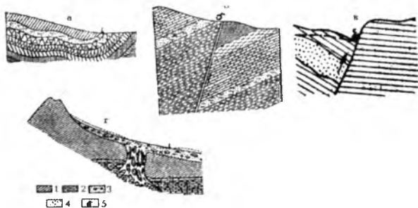
13.2-расм. Пастдан юқорига отилиб чиқувчи булоқлар (М.В.Альтовский ва бошқа мавжуд маълумотлар бўйича) а-дарё водийларидан оқиб чиқувчи эрозиявий булоқлар; б,в-тектоник экранланган булоқлар; г-босимли сув таъсири натижасида сув ўтказмайдиган қатламнинг бузилиши ёки грунт сувлари оқими таъсири остида босимли сувларнинг ҳаракатга келиши оқибатида пайдо бўлган булоқлар; 1-сув ўтказмайдиган жинс қатлами, 2-сувли оҳактош, 3-босимли сув ҳаракати натижасида сув ўтказмайдиган қатламни ёриб чиқиб жараёни; 4-сувли кум қатлами, 5-ер ости сувларининг пастдан юқорига ҳаракат қилиши натижасида вужудга келган булоқлар
