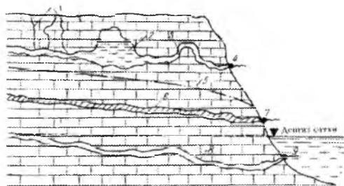
11.4-расм. Карст булоқлари: 1-ер юзасига чикувчи ёриқлар; 2-карстли ер юзаси; 3-сифон туридаги букилган каналлар; 5-карст сувли горизонтлардаги доимий сув сағхи; 6-карст каналлари; 7-доимий булоқ; 8-сув ости булоқлари
