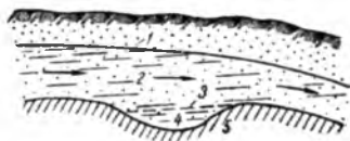
9.5-расм. Грунт сувлари оқими ҳавзаларининг бир-галикдаги қўриниши: 1-грунт сувлари сатҳи, 2-грунт сувлари оқими, 3-грунт сувлари оқимининг ҳавзалари ўртасидаги чегара, 4-грунт сувлари ҳавзаси, 5-сув тўсғич
