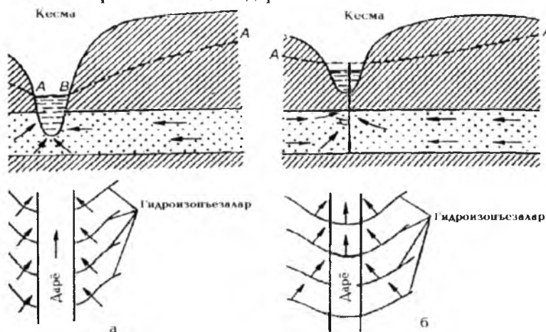
10.3-расм. Босимли сувларнинг ер усти сув хавзалари билан ўзаро алоқаси (У.Богомолов): а-босимли сувлар оқимининг дарё сувлари оқими бўйича таъминланиши; б-дарё сувлари оқимининг босимли сувлар оқими билан таъминланиши, А-пъезометрик юза
