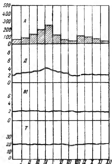
13.3-расм. Булоқлар режимини тавсифловчи чизма (В.М.Максимов ва Д.И.Пересунколардан). А-атмосфера ёғини, мм; Д-булоқ-нинг дебити, л/сек; М-сувнинг минераллашдиш даражаси, г/л; Т-сувнинг ҳарорати, °С.
