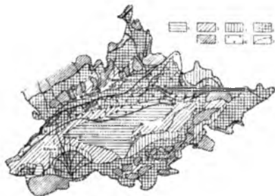
19.6-расм. Фарғона артезиан ҳавзаси тўртламчи давр юқорини юз метрлик қатлами жинсларинини сув ўтказувчанлик хусусияти ўзгаришини кўрсатувчи чизма (В.А.Гейнц, А.Н.Султонхўжаевлар бўйича).
