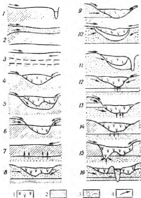
20.2-расм. Сувни қочирилатётган ерларнинг гидрогеологик шаройтларининг турлари (1-16). 1-торф; 2-гил тупрок; 3-кум (кум тупрок, майда шағал), ёриқоли (коча жинслар), 4-ер усти ва ер ости сувлари ҳаракати
