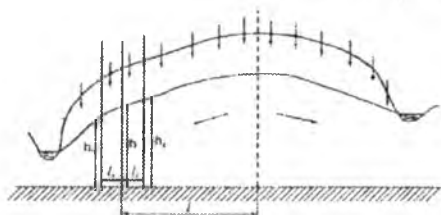
17.2-расм. Грунт сувларини миқдорини инфильтрация йўли билан озиқлаштириш аниқлаш чизмаси
