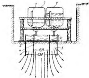
19.4-расм. Дала тажриба филтрацион ишларини олиб боришда қўлланиладиган Н.С.Нестерев асбобини пиллаш жараёнидаги кўриниши. 1-ўлчаш линейкаси; 2-бутиллар; 3-шурфни тоғ қисмига солинадиган майда пағал қатлами; 4-ички метал халқа; 5-тапқи метал халқа
