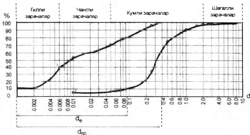
6.5-расм. Жинслар механик таркибининг логарифмик масштаблардаги жадвали: 1-соғуноқ; 2-қум
