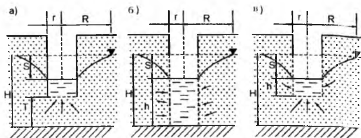
21.1-расм. Кон майдони шахта қудукларига ер ости сувларининг оқиб келиш чизмаси (Й.Э.Эргашевдан. 1990). а-тубидан, б-ён деворларидан, в-туби ва ён деворларидан
