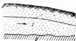
9.3-расм. Грунт сувлар оқимини чизмаси: 1-грунт сувлари юзаси, 2-сувли қумлар, 3-сув ўтказмайдиган жинслар
