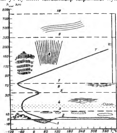
5.3-расм. Ер атмосферасининг тузилиши (Ф.Ю.Зшеддан, 1988)
