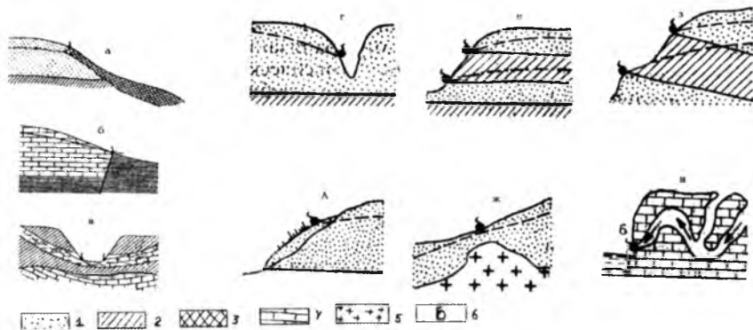
13.1-расм. Пастга эркин оқувчи булоқлар (М.Е.Альтовский ва бошқа мавжуд маълумотлар бўйича): а-литологик экранланган булоқлар, б-тектоник экранланган булоқлар; в,д,е,ж,з,и-дарё эрозия водийларидан оқиб чиқувчи (д-делювиал жинс ётқиқиқлари билан қопланган жойлардан); ж-она (магматик ва б.) тоғ жинслари унча-лик чуқурда ётмаган жойлардан ва з-маълум баландликлардан оқиб тушувчи; и-карстбулоқлар; 1-сувли кум қатламлари; 2-сув ўтказмас жинс қатлами, 3-сув оқими йўлини тўсувчи қатлам. 4-оҳактош қатлами, 5-она тоғ жинси, 6-пастга оқувчи булоқ
