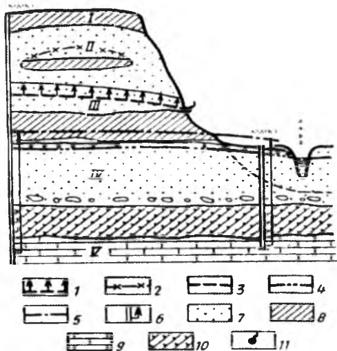
9.2-расм. Ер ости сувларини жойлашши шартини бўйича таснифи: I-гулрокдаги сувлар, II-юзак сувлар, III-грунт сувлари, IV-қатламлар оралигидаги босимсиз сувлар, V-босимли (артезиан) сувлар. 1-капитляр кайма, 2-юзак сувларни сатҳи, 3-грунт сувлар сатҳи, 4-қатламларо босимсиз сувлар сатҳи, 5-босимли сувларни пьезометрик сатҳи, 6-бургу қудугидаги босим ўлчами, 7-сув ўтказувчан тоғ жипси, 8-сувни ёмон ўтказувчи ва ўтказмайдиган жипслар, 9-сувни ўтказувчи жипслар, 10-сувни ўтказмайдиган жипслар, 11-булоқ
