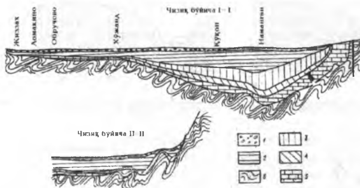
10.4-расм. Фарғона артезиан суви ҳавзасининг тузилмавий геологик кесмаси (А.Н.Султонхўжаев бўйича). Сувли тоғ жинс қатламлари: 1-тўртламчи давр (Q), 2-қуйи (Сўх) тўртламчи (Q 1 ) ва бактрий свитаси жинслари (N 2 ), 3-массагет свитаси жинслари (N 1 ), 4-палеоген даври жинслари (P), 5-бўр даври жинслари (K), 6-палеозой даври жинслари (Pz)
