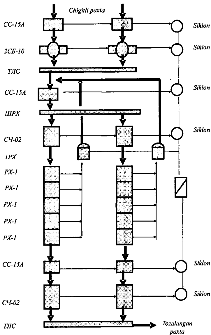
19-rasm. JII-IC-uskunalar majmuasining texnologik jarayon sxemasi.
