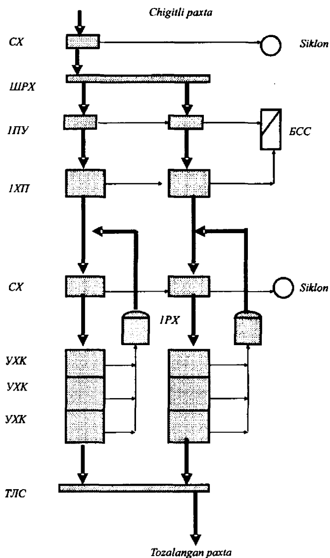
12-rasm. 2ЛПО-uskunalar majmuasining texnologik jarayon sxemasi.
