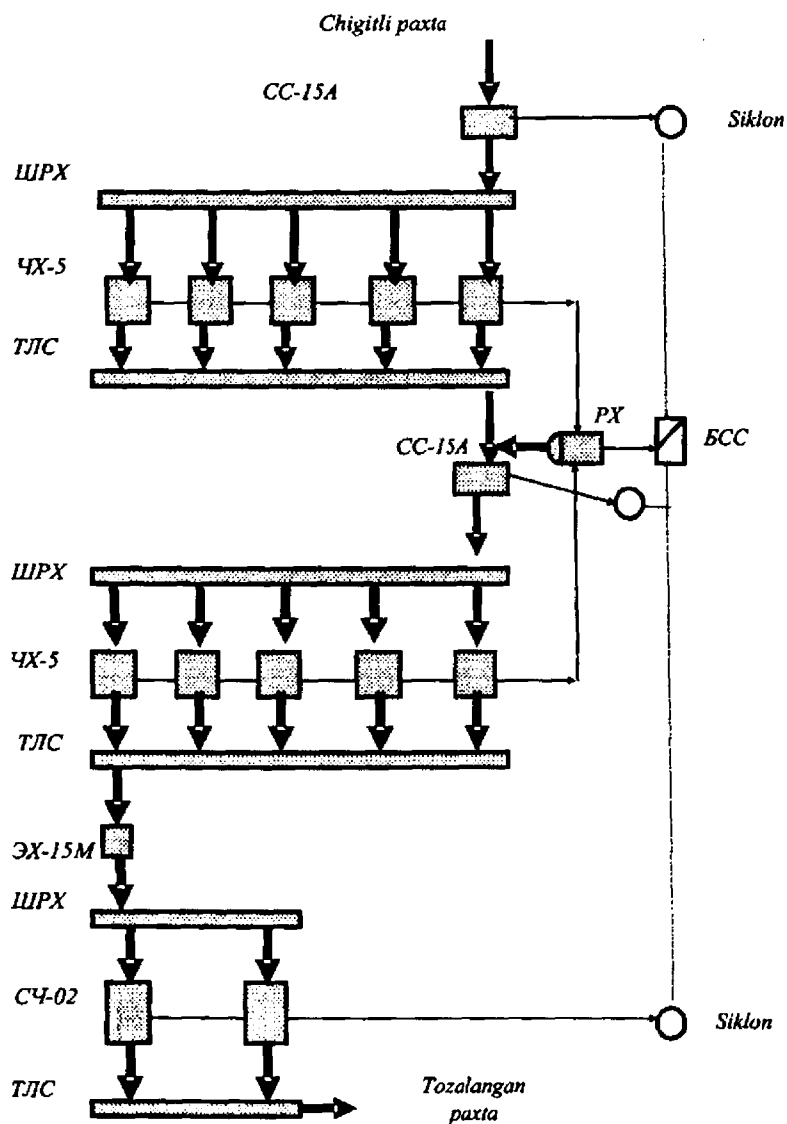
24-rasm. BKO-T uskunalarining texnologik jarayon sxemasi.
