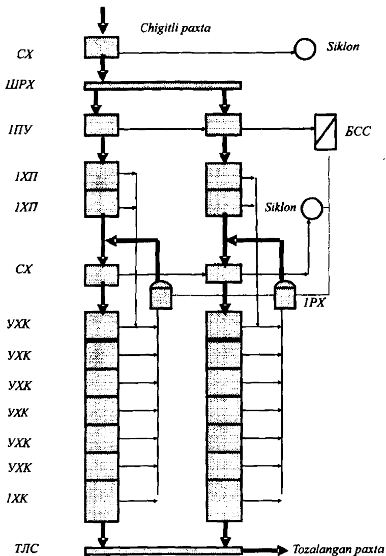
18-rasm. KOFI-ushkunalari majmuasining texnologik jarayon sxemasi.
