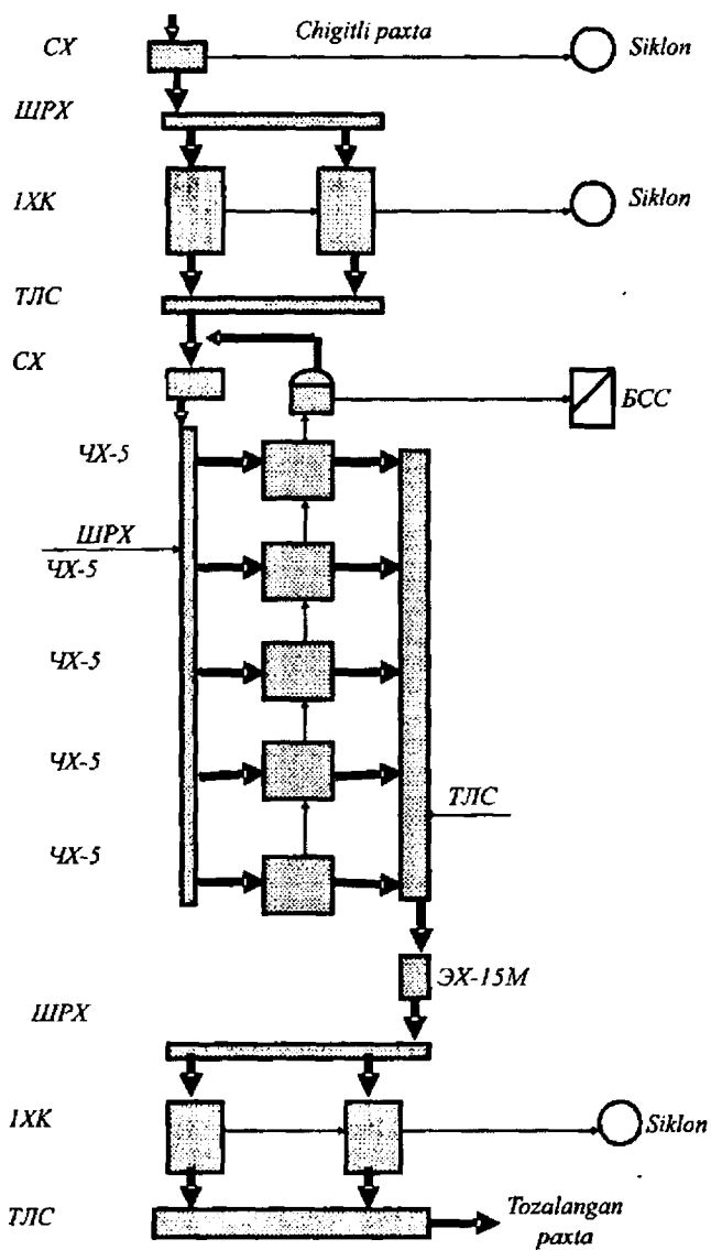
13-rasm. 2KOH uskunar majmuasining texnologik jarayon sxemasi.
