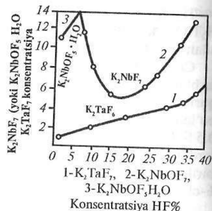
2- grafik. Turli konsentratsiyali plavik kislotalarda tantal va niobiyning fluor komplekslarining (25°C da) erishi.
