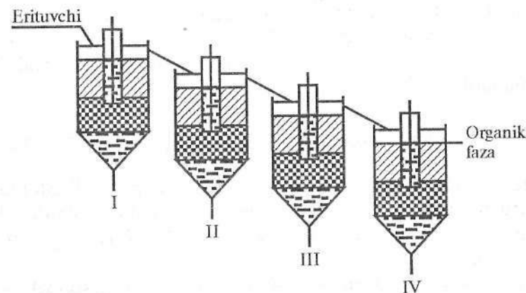
9-rasm. Yarim teskari oqimda ekstraksiyalash I, II, III, IV suvli eritma fraksiyalari: 1— aralashtirish kamerasi; 2— tindirish kamerasi.
