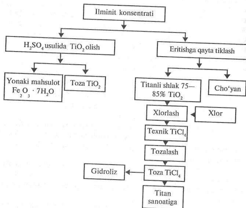
5-chizma. Ilminiti konsentratidan TiCl 4 yoki TiO 2 ni olish.
