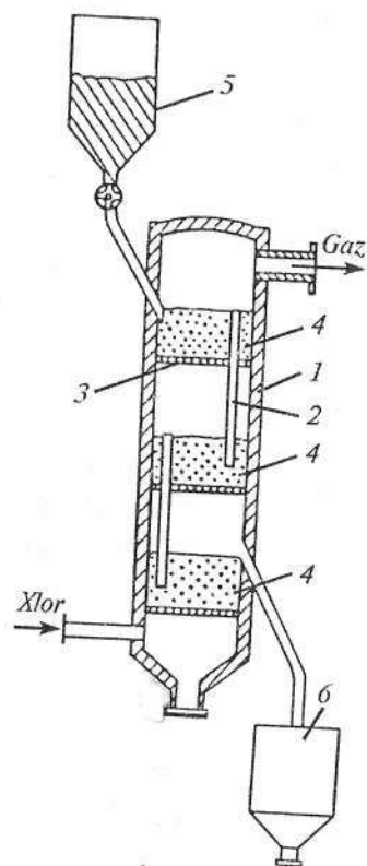
1-rasm. Qaynovchi qavatlarda xlorldash.
