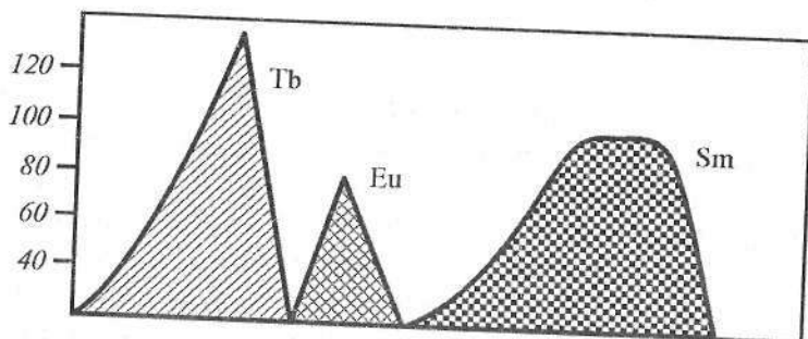
8- rasm. Smolada yutilgan terbiy, yevropiy va samariy elementlarini pN = 3,62 da 0,26 molarli ETDS eritmasi bilan ajratib (yuvib) olish egri chiziqlari.
