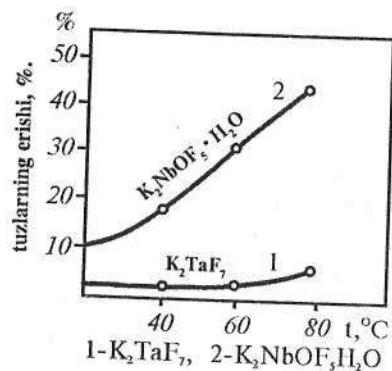
1- grafik. Kaliy fiortantalat fluoroksiniobat tuzlarining 1% li plavik kislotasi va harorat o'zgarishi.
