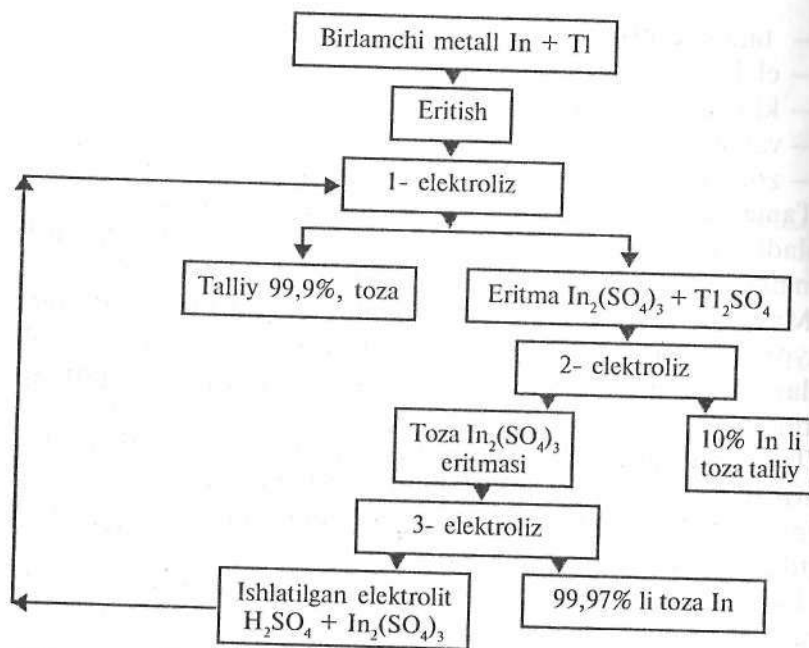
14-chizma. Indiyi elektrokimyoviy usulda olish.
