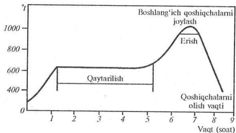
3- grafik. \text{GeO}_2 ni qaytarish sharoiti va undagi germaniyli qoshiqchaning o'choqda harakatlanishi.
