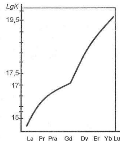
4- grafik. KYEE larining tartib raqami barqarorlik konstantasiga nisbatan oshishi.
