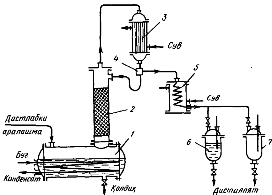
15.7-расм. Даврий ишлайдиган ректификацион қурилма схемаси:
