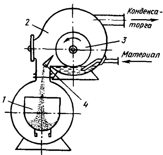
18.29-расм. Вальцовка куриткичлар:
