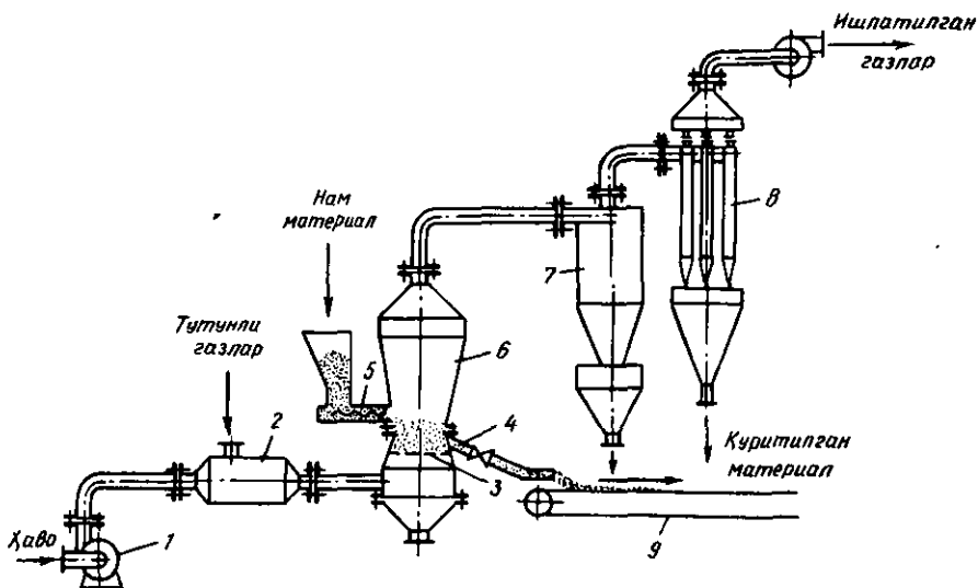
18.20-рasm. Мавхум қайнаш қатламли қуриткич:
