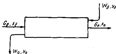
9.10-расм. Экстракторнинг моддий балансини аниқлашга доир.
