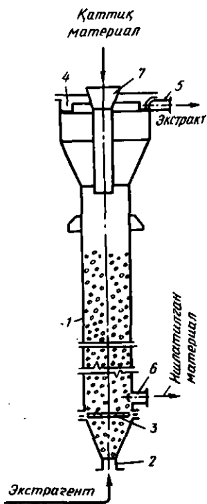
19.9-рисм. Мавхум қайнаш қатламли экстрактор:
