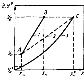
14.2-расм. Абсорбция процессининг иш на мувозанат чизиклари: 1 — абсорбентнинг сарфи L бўлгандаги иш чизиги; 2 — абсорбентнинг сарфи L_{\text{мин}} бўлгандаги иш чизиги; 3 — мувозанат чизиги Y^* = f(X) .
