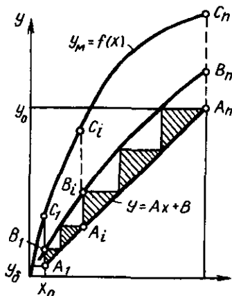
16.21-расм. Қарама-қарши окимли экстракторларда тарелкалар сони аниқлаш.
