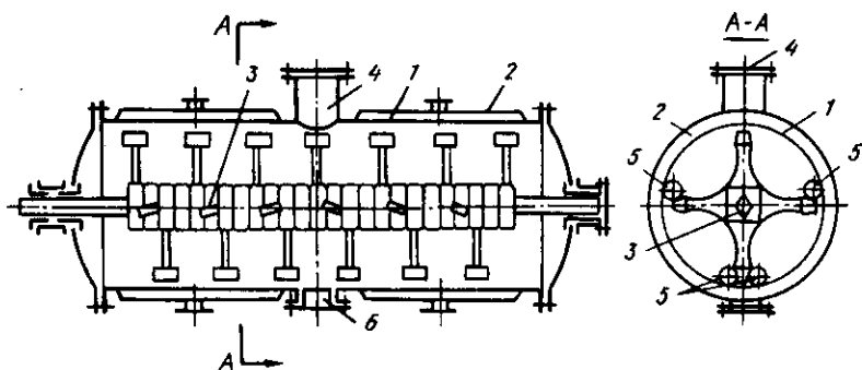
18.28-расм. Тарокли вакуум — қуритгич:
