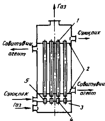
14.8-расм. Суюқликнинг юпка қатлами кўтарилма ҳаракат қилувчи абсорбер:
