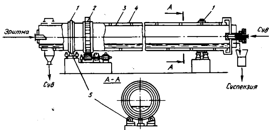
20.3-расм. Барабанли кристаллизатор:
