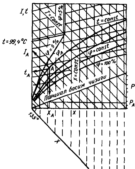
18.1-расм. Нам ҳавонинг I-x диаграммаси.
