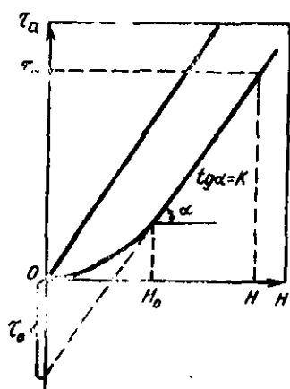
17.11-расм. Қатламни адсорбцион химоя қилиш вақти \tau_a нинг адсорбент қатлами баландлиги H дан боглиқлиги.
