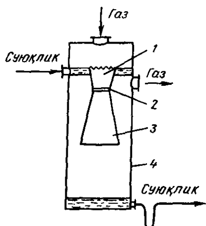
14.23-расм. Вентури абсорбери: 1 — конфузор; 2 — диффузорнинг бўған; 3 — диффузор; 4 — ажратиш камераси.
