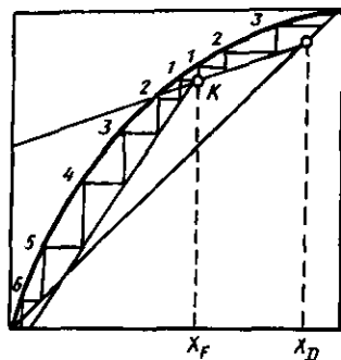
15.11-расм. Концентрация погонялари сонини график усул билан аниқлаш.
