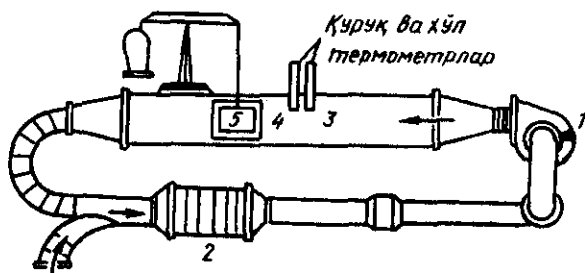
18.6-расм. Қуришти процессини ўрганишга мўлжалланган лаборатория қурилмасининг схемаси:
