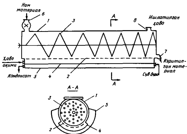
18.24-расм. Шнекли қуриткич:
