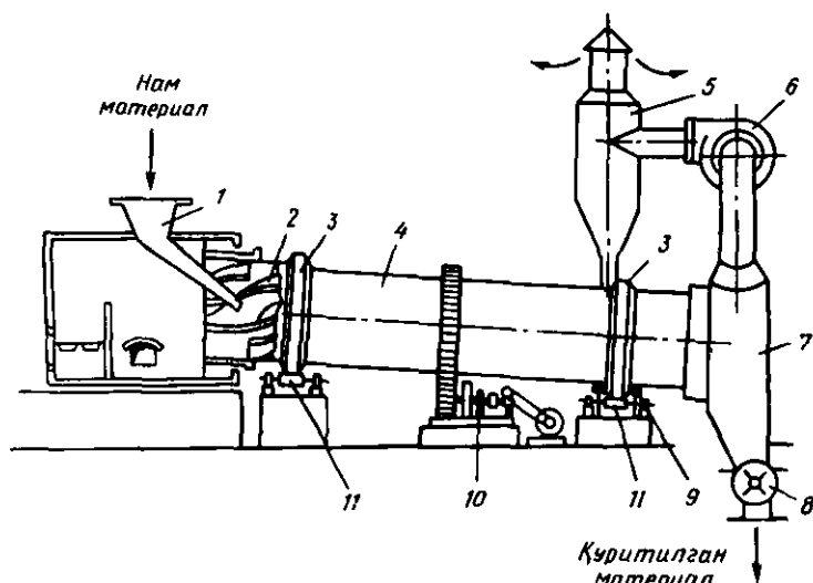
18.18-расм. Барабанли қуритгич:
