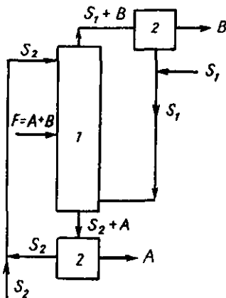
16.9-расм. Икки хил эритувчи ва флегмадан фойдаланишга асосланган қарама-қарши оқимли экстракциялаш схемаси:
