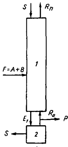
16.8-расм. Флегмадан фойдаланадиган кўп погона ва қарама-қарши оқимли экстракциялашнинг схемаси:
