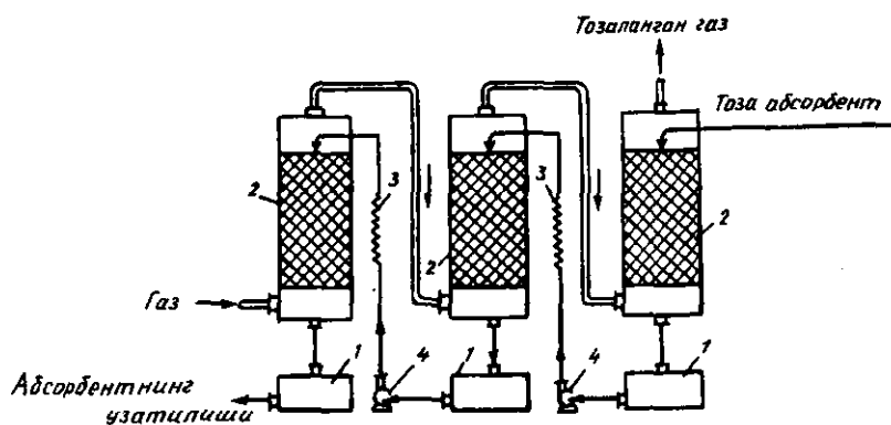
14.4-рasm. Карама-қарши йўналишли абсорбция қурилмасининг схемаси:
