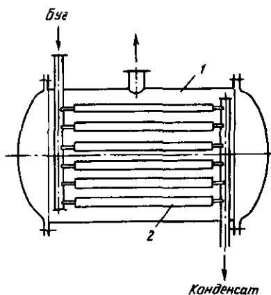
18.27-расм. Вакуум — куриштиш шкафи: 1 — куриштиш камераси; 2 — ичи бўш токчалар.
