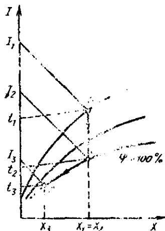
18.3-расм. Ҳавонинг совитиш жараёни I - x диаграммада тасвирлаш.
