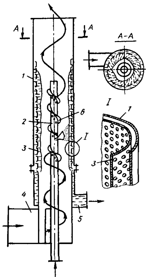
14.30-расм. Суюқликнинг винтли юза бўйлаб конуссимон ҳолатда отилиб чиқинв усули билан намланадиган уюрмалли модда алмашиниш аппарати:
