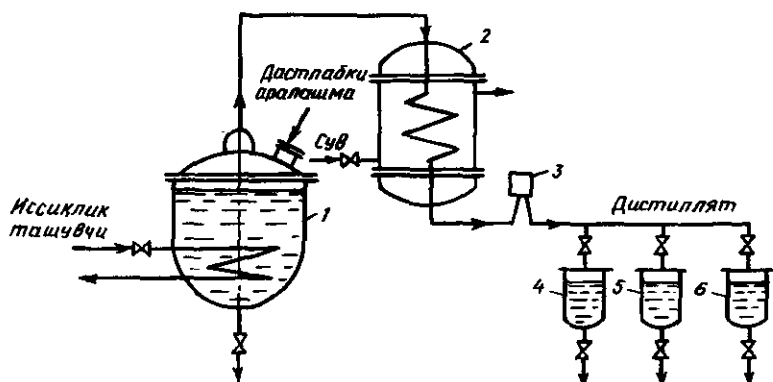
15.3-расм. Оддий хайдаш қурилмасининг схемаси:
