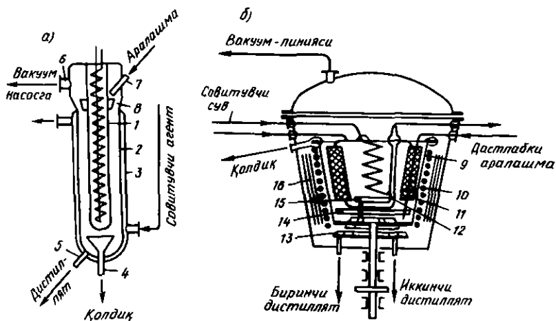
15.15-расм. Молекуляр дистиллаш аппаратлари:
