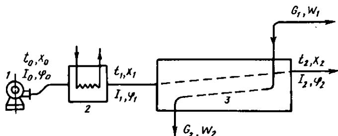
18.9-расм. Нормал қуриштиш процессининг схемаси:
