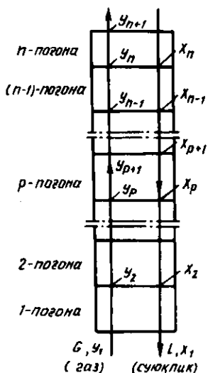
13.10-расм. Карама-қарши йўналган n -погона-ли модда алмашиниш апаратынинг схемаси.
