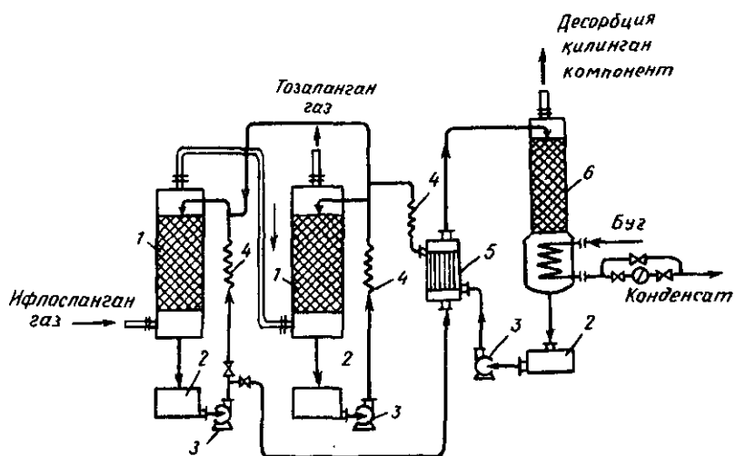
14.5-рasm. Рециркуляцияли абсорбция — десорбция қурилмасининг схемаси:
