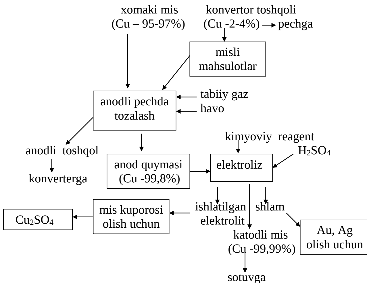
4-rasm. Olmalik sharoitida mis olish texnologiyasi.
