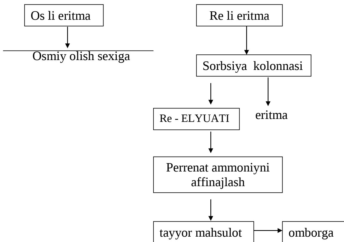
11-rasm. Reniyli perrenat ammoniy olish texnologiyasi.
