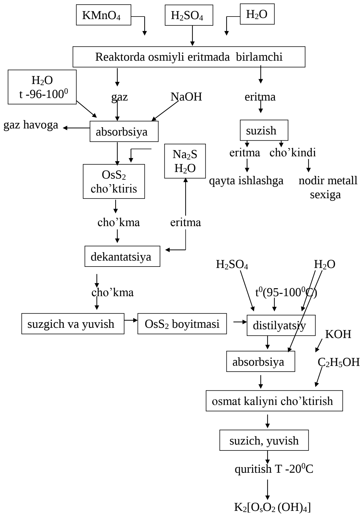
12- rasm. Osmiyni kukun holida olish texnologik tasviri.
