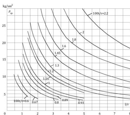
1.1-rasm Tashqi bosim ta'sirida bakning silindr qismiga tushadigan kiritik bosim
