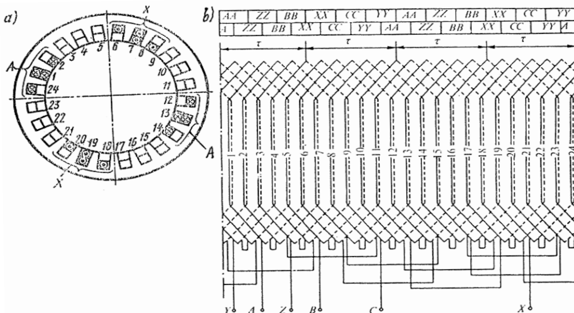
4.2-rasm. Uch fazali ikki qatlamli cho'lg'am g'altaklarining statorda joylashishi (a) va sirtmoqsimon cho'lg'amning ( Z=24 , m=3 , 2p=4 , y=5 ) yoyma sxemasi (b)
