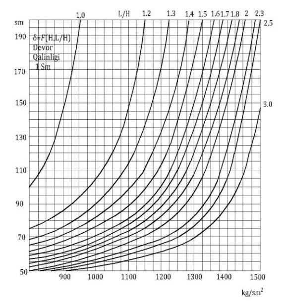
1.1-rasm Tashqi bosim ta'sirida bakning silindr qismiga tushadigan kiritik bosim
