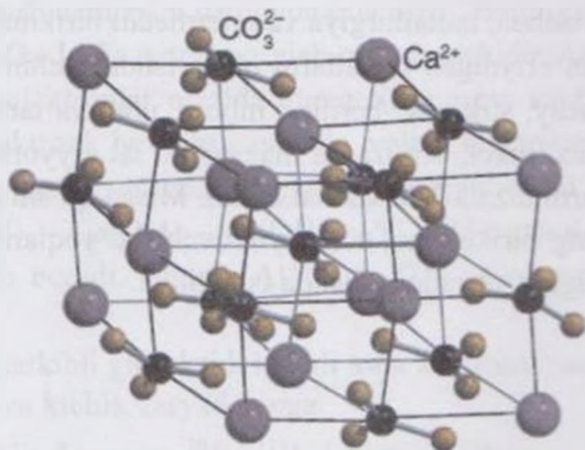
10.13-rasm. \text{CaCO}_3 ning strukturaviy koʻrinishi.
