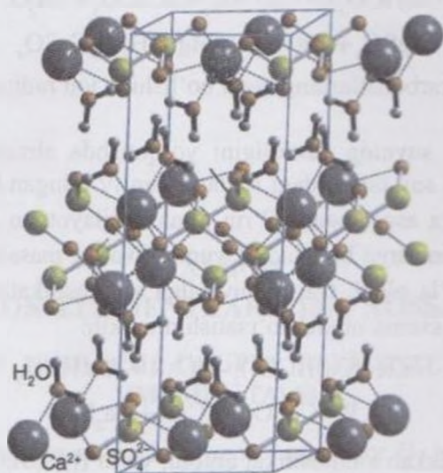
10.12-rasm. Gips ( \text{CaSO}_4 \cdot 2\text{H}_2\text{O} )ning strukturası.
