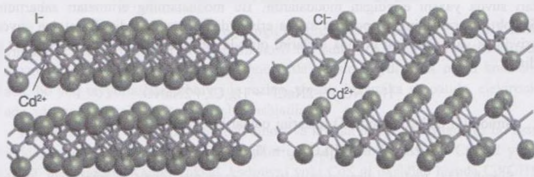
15.15-rasm. \text{CdJ}_2 va \text{CdCl}_2 ning strukturasi.
