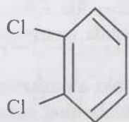
ortodixlorenzol
