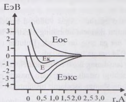
4.10-rasm. Vodorod molekulası potensial energiyasining o'zgarishi.
