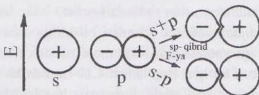
4.13-rasm. p – gibrirlangan orbitalning shakllanishi.
