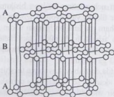
\alpha - Gaphit
