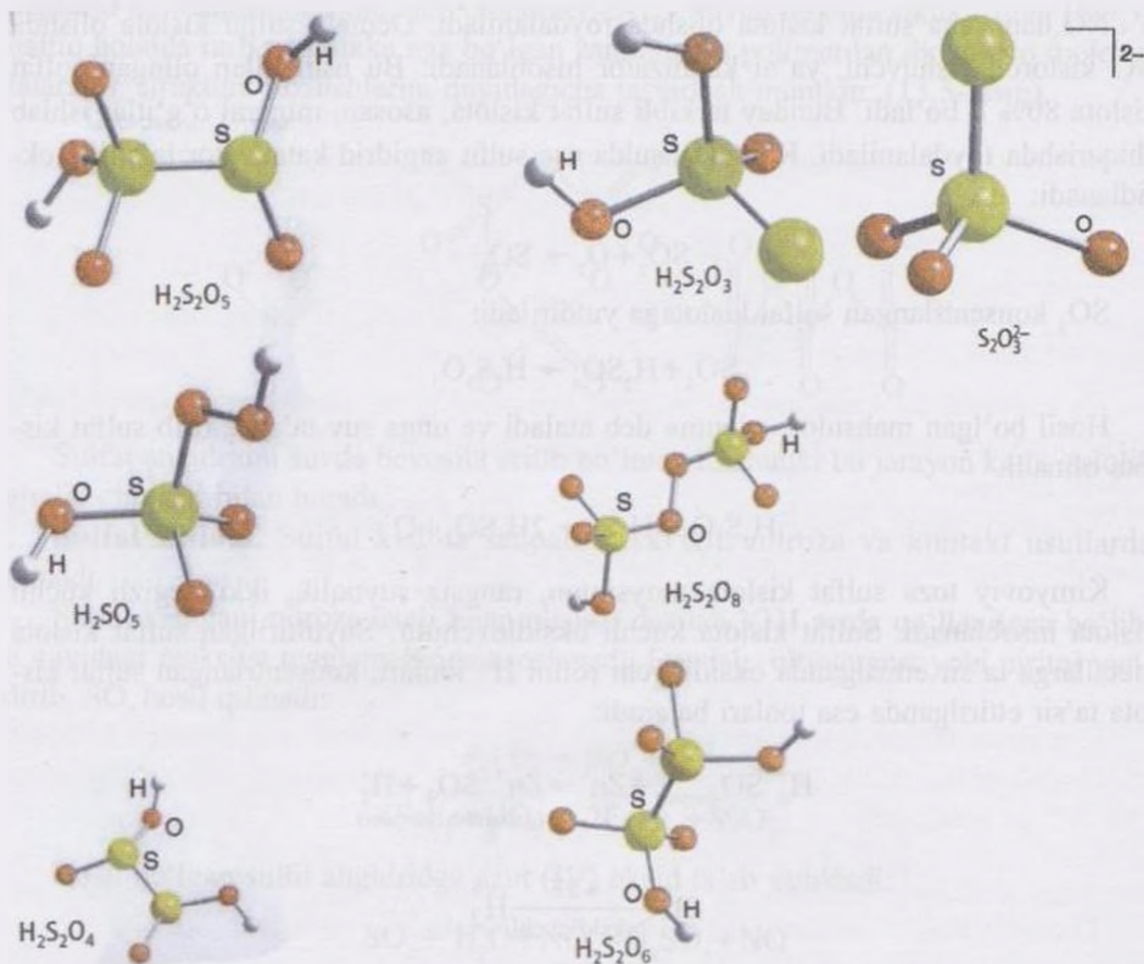
13.6-rasm. Oltingugurt polikislotalari strukturasi.
