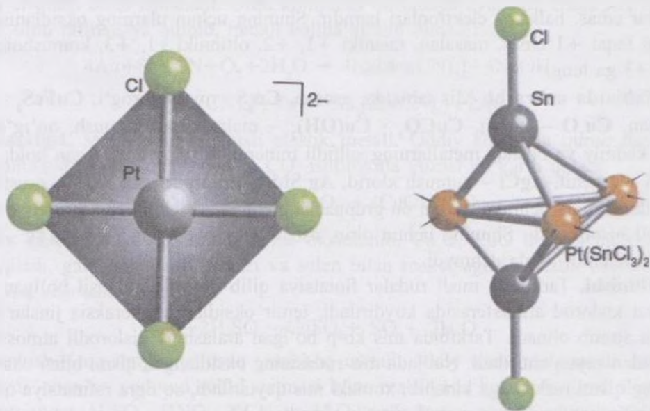
15.9-rasm. Platina kompleks ioni [\text{PtCl}_4]^{2-} ko‘rinishi.
