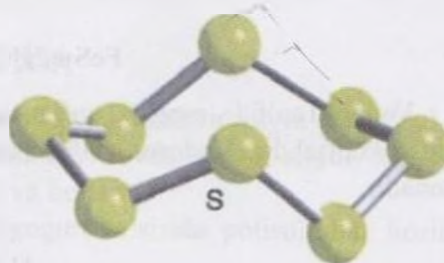
13.3-rasm. Oltingugurt molekulasida \text{S}_8 ning struktura ko'rinishi.
