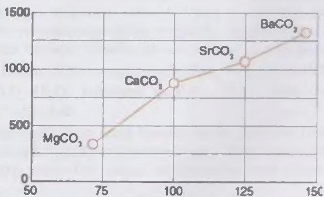
10.14-rasm. Karbonatlar hosil boʻlishi haroratlarning ion radiusiga bogʻliqligi.
