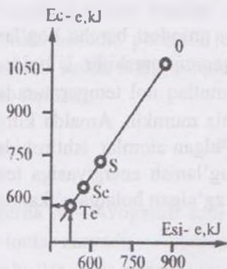
4.6-rasm. Kremniy va uglerod birikmalarining bog'lanish energiyalari grafi.
