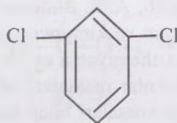
metadixlorbenzol
