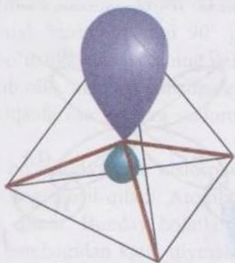
4.14- rasm. sp^3 - gibrirlanishi.
