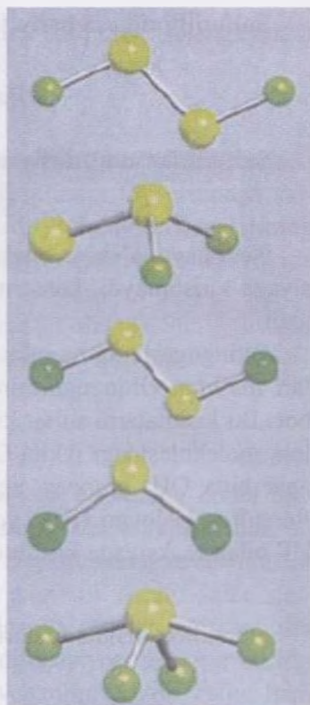
13.7-rasm. Oltingugurtning galogenli birikmalari.
