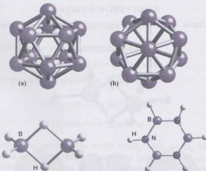
10.16-rasm. B_{12} -ning gorizont (a) va vertikal (b), diboran B_2H_6 va borazol B_3N_3H_6 ning strukturalari.
