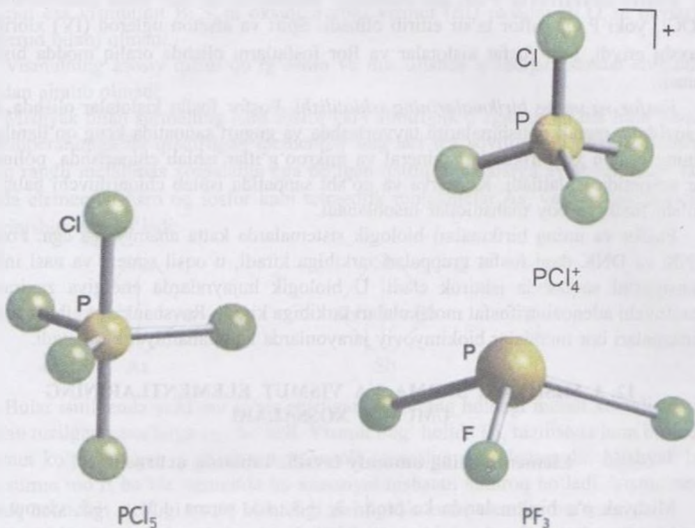
12.7- rasm. \text{PCl}_5 va \text{PF}_3 molekulası ko'rinishi.
