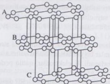
\beta - Gaphit
