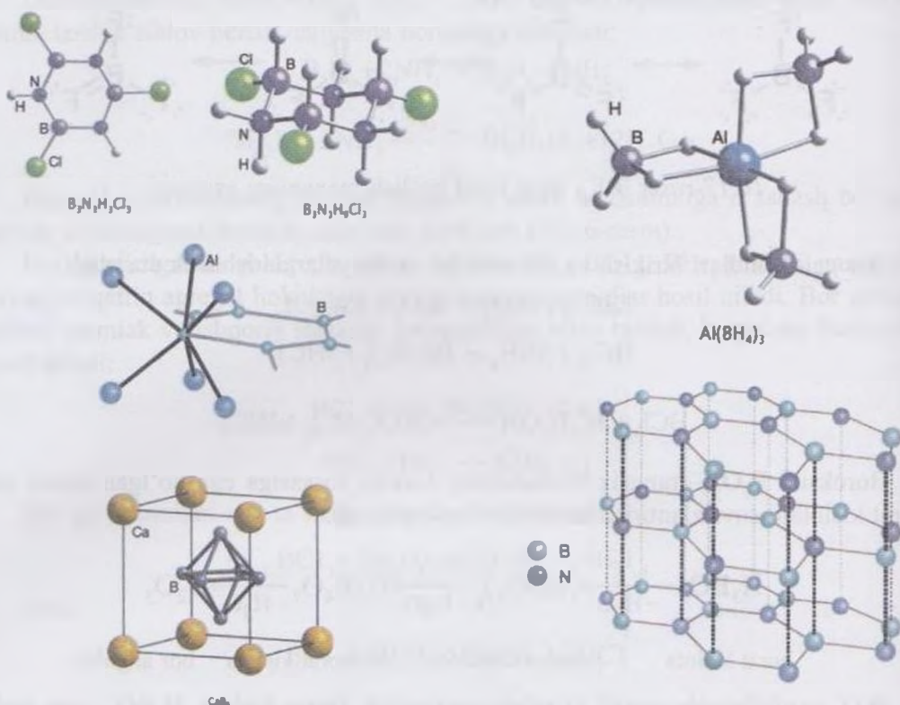
10.18-rasm. Borning alumiiniy, kalsiy va azotli birikmalari strukturasi.
