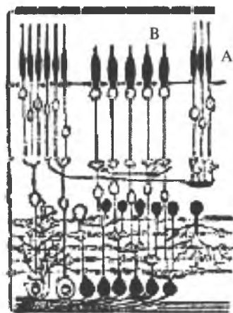
13-rasm. Ko'z to'r pardasi- ning tuzilishi:
