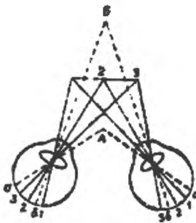
26-rasm. Ikkala ko'z pardasida nuqtalarning mos va nomoslik sxemasi.
