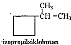
izopropilsiklobutan
