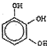
pirogallol
