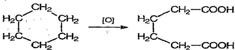
siklogeksan
