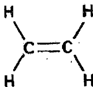
eten (etilen)
