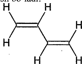
butadiyen-1,3
