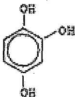
oksigidroxinon
