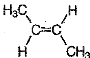
trans-buten-2
