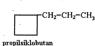
propilsiklobutan
