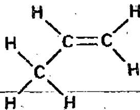
propen (propilen)
