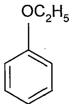
etilfenil efir
