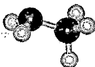
Metilamin
