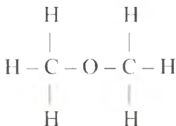
dimetil efir
