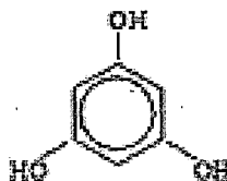
floroglutsin
