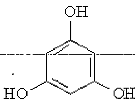
floroglutsin
