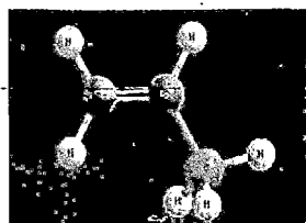
31-rasm. Etilen va propilen molekulalarining modellari.
