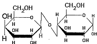
Laktoza
