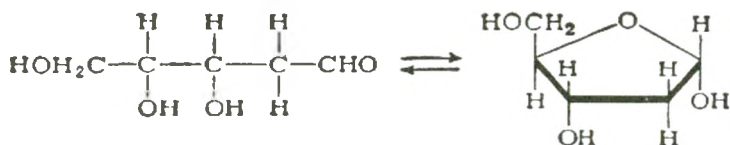
dezoksiriboza
