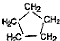
siklopentan
