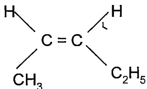
sis-penten-2
