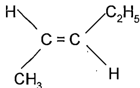
trans-buten-2
