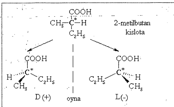
42- rasm. 2-metilbutan kislotaning D(+) va L(-) optik antipodlari.
