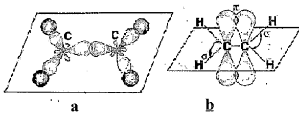
23-rasm. Etilen molekulasida \sigma -bog'lar (a) va \pi -bog'lar(b) ning hosil bo'lishi.
