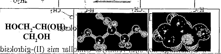
41-rasm. Glitserinning: A struktura formulasi; B va C sharsterjenli va yarimsharsimon modeli.
