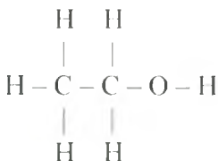
etil spirti
