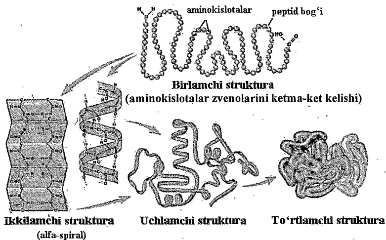
51-rasm. Oqsil molekulasining I, II, III va IV strukturalari.
