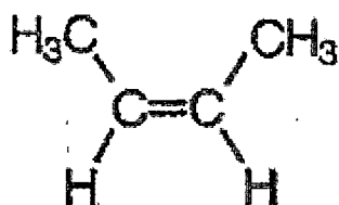
sis-buten-2
