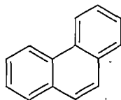
fenantren
