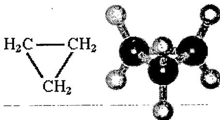
Siklopropan
