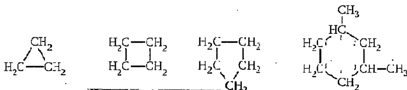
siklopropan
