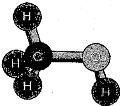
39- rasm. A) Spirt molekulasining geometriyasi; B) metanolning fazoviy tuzilishi.
