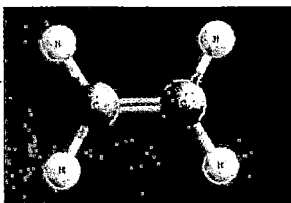
31-rasm. Etilen va propilen molekulalarining modellari.
