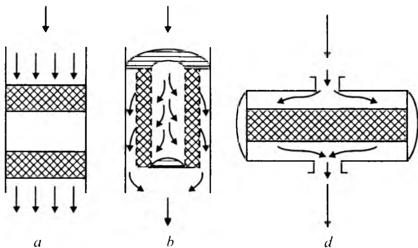
5.42-rasm. Katalizator aksial (a), radial (b) va gorizontaal (d) qatlamlar tarzida joylashuvchi reaktor.
