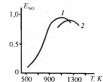
4.43-rasm. T haroratni ammiakni 0,1 MPa (1) va 0,7 MPa (2) bosimlarda azot oksidi hosil bo'lish miqdori E_{NO} ga ta'siri.
