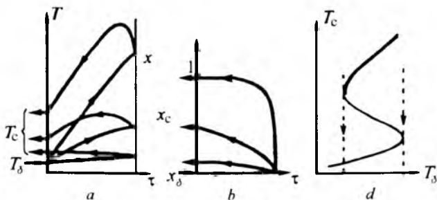
2.70-rasm. Avtotermik reaktordagi statsionar rejimlar.
