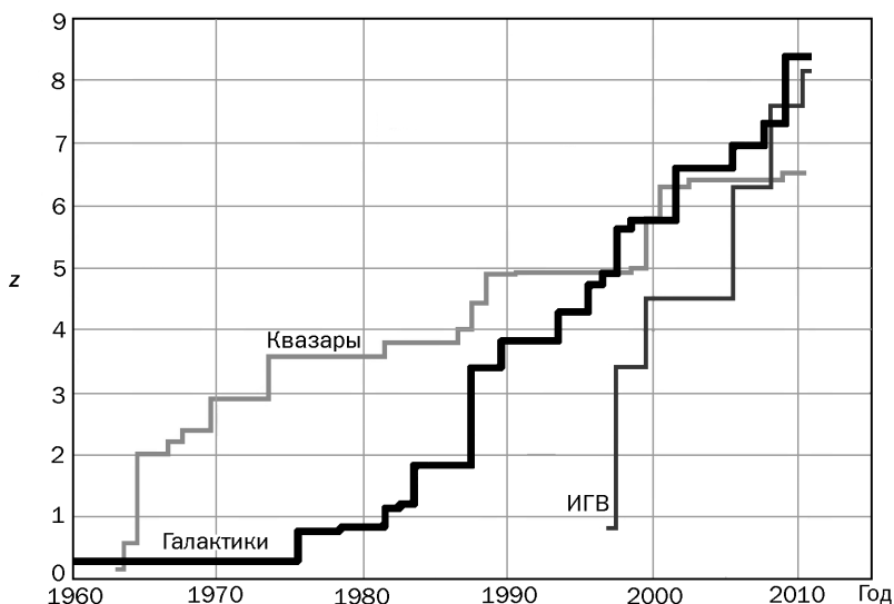
Рис. 9.33. Максимальное красное смещение ( z ) галактик, квазаров и источников гамма-всплесков (ИГВ), открытых к указанному году.
