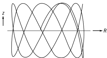
Рис. 3.21. Ящикообразная орбита в проекции на сопутствующую плоскость.
