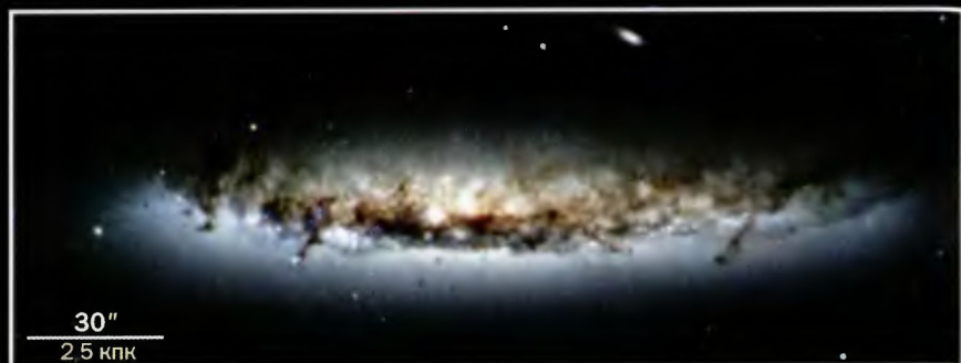
Галактика NGC 4402, наблюдаемая недалеко от центра скопления Virgo и испытывающая динамический напор межгалактического газа.
