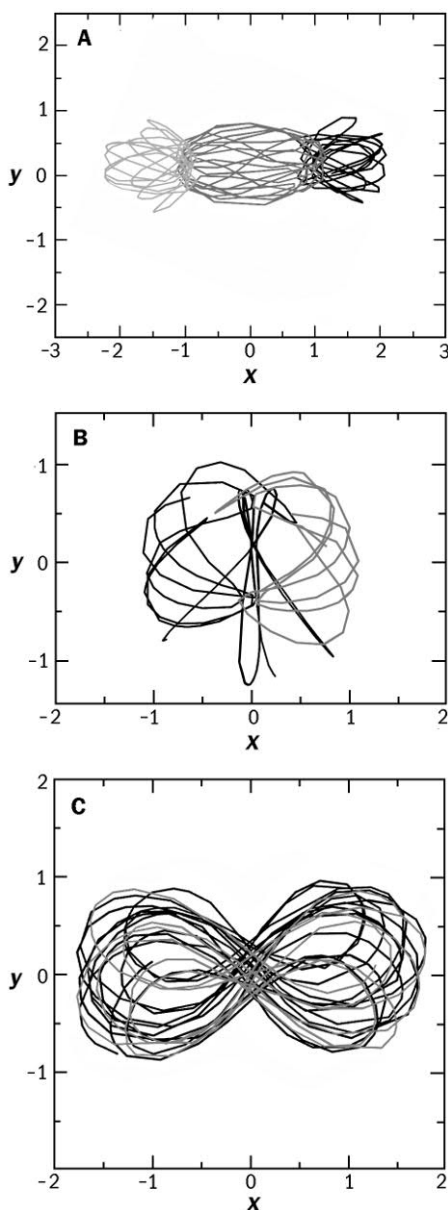
Рис. 2.5. Фрагменты «прилипания» траекторий к периодическим орбитам Шубарта (А), Брука (В) и к «восьмерке» (С), показанным на рис. 2.4.
