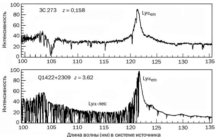
Рис. 9.24. Типичные спектры относительно близкого ( z = 0,158 ) и значительно более далекого ( z = 3,62 ) квазаров. Отдельные линии поглощения Ly в спектре далекого квазара превращаются в «густой лес».
