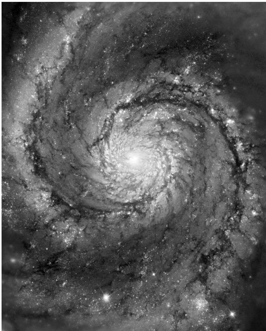
Рис. 6.2. Современное фото центральной части галактики М51 демонстрирует почти идеально симметричную двухрукавную спираль, образованную яркими областями звездообразования и оконтуренную с внутренней стороны рукавов темными прожилками холодных газовой-пылевых облаков.
