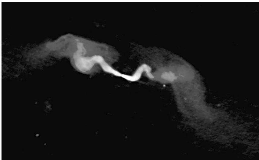
Рис. 9.18. Радиогалактика 3C 31 с двумя протяженными компонентами, яркость которых уменьшается по мере удаления от ядра (тип FRI).
