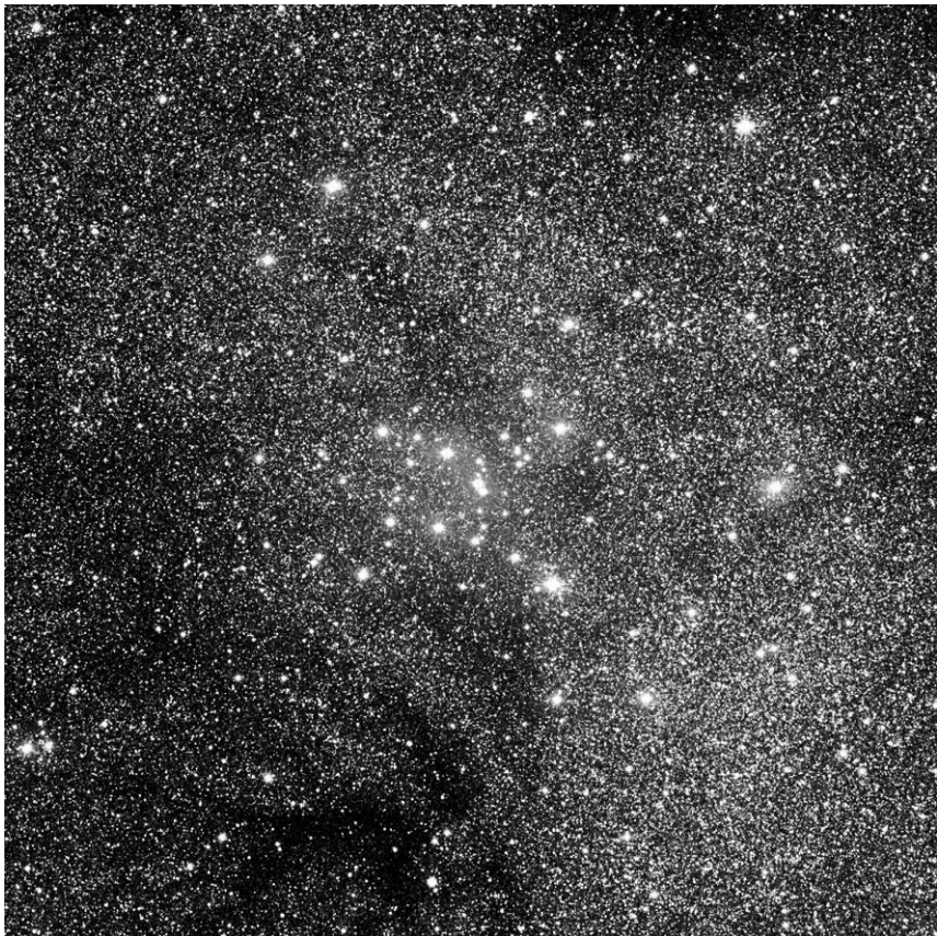
Рис. 7.23. Рассеянное скопление Мессье 7 в созвездии Скорпион наблюдается на фоне более далеких звезд центральной области Галактики. Возраст этого скопления около 250 млн лет, вполне зрелый для рассеянного скопления.
