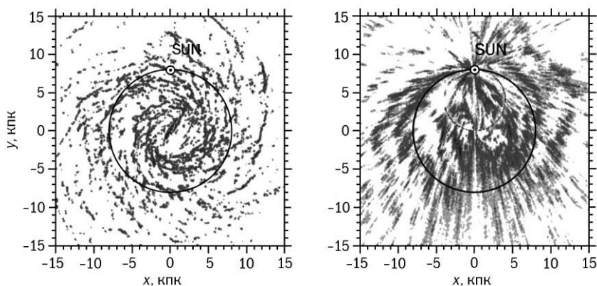
Рис. 6.16. Численная модель галактики Ваба и др. (2009) при ее условном возрасте 2 млрд лет. SUN — положение Солнца; R_0 = 8 кпк; v_0 = 162 км/с. Большая ось бара ориентирована под углом 25^\circ к направлению на Солнце. Слева: истинное распределение холодного ( T \sim 100 K) газа в диске. Справа: такой результат для распределения холодного газа получит наблюдатель, применив кинематический метод оценки расстояний и предполагая, что газ обращается вокруг центра галактики по круговым орбитам.
