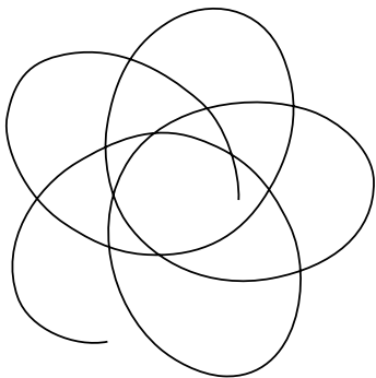
Рис. 3.18. Орбита частицы в поле с силой F \propto r^{-1,5} (Сурдин, 2009).
