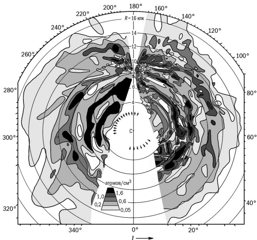
Рис. 6.12. Карта распределения плотности нейтрального водорода по наблюдениям в линии 21 см, построенная Оортом, Керром и Вестерхаутом (Oort et al., 1958) на основе модели Шмидта 1956 г. (см. рис. 6.7). В направлении на центр и антицентр Галактики кинематический метод не работает.
