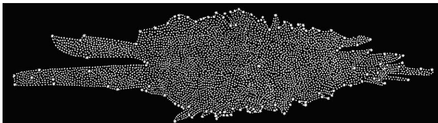
Рис. 4.2. Карта меридионального (т. е. перпендикулярного плоскости экватора) сечения галактического диска, построенная Вильямом Гершелем на основе «звездных черпков». Здесь она показана в негативе. Солнце — жирная точка — оказалось почти в центре звездного острова.
