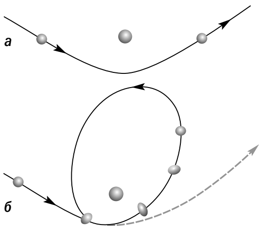
Рис. 7.26. Приливный захват при тесном сближении двух звезд (одна из них для простоты показана неподвижной и абсолютно жесткой). Если бы звезды не деформировались гравитацией соседа (а), то пролет был бы симметричным, и захват не произошел. В действительности (б) приливная деформация звезды отбирает у нее часть механической энергии, поэтому звезда переходит на связанную орбиту — образуется двойная система.
