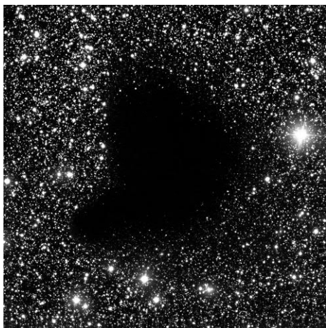
Рис. 7.28. Два препятствия в Млечном Пути мешают поиску далеких звездных скоплений — непрозрачные для света облака и богатый звездный фон в промежутках между ними. На снимке: газово-пылевое облако B68 (Barnard 68) в созвездии Змееносец, удаленное от Земли всего на 150 пк; поэтому перед ним не оказалось ни одной яркой звезды, а за ним вообще ничего не видно. Фото: телескоп VLT обсерватории ESO (Чили).
