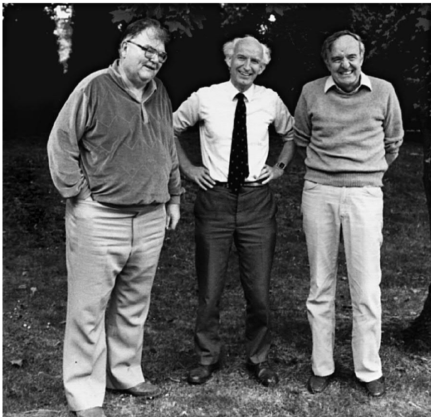
Рис. 5.3. Эгген, Линден-Белл и Сэндидж — авторы бессмертной работы ELS, посвященной формированию Галактики и кинематике ее старейших звезд. Снимок сделан на обсерватории Серро-Тололо в 1995 г.
