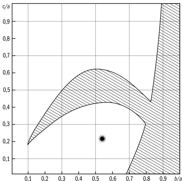
Рис. 3.28. Области устойчивости и неустойчивости (заштрихована) для моделей трехосных эллипсоидов Фримена. По осям отложены отношения осей эллипсоида. Звездочка соответствует галактике NGC 4027.
