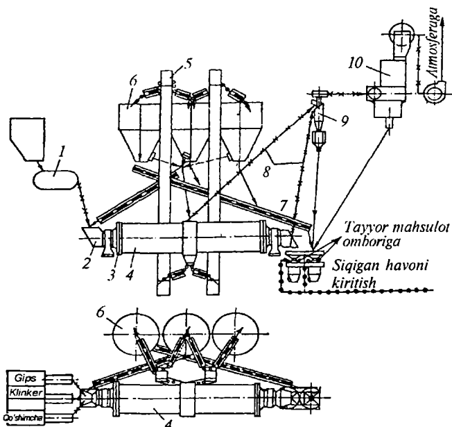
13-rasm. Separator tegirmon qurilmasining chizmasi.
