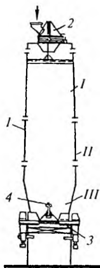
4-rasm. Shaxta pech tasviri.
