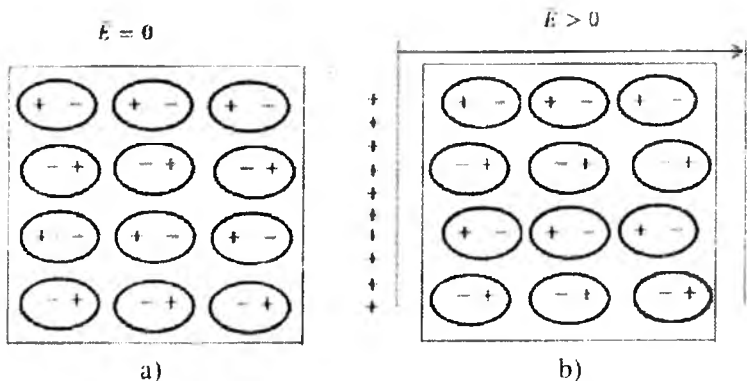
17.3-rasm. Ionli dielektriklar. a) qutblanishdan oldin, b) qutblanishdan keyin
