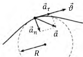
1.4-rasm. Egri chiziqli harakatda tezlik va tezlanish
