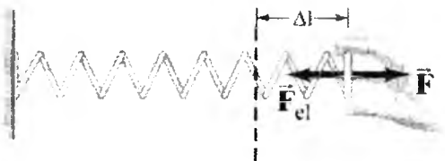
3.1-rasm. Elastik kuchining vujudga kelish sxemasi
