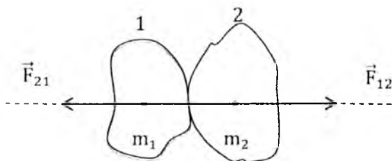
2.3-rasm. Ikki jism ta'sirlashganda vujudga keluvchi kuchlar
