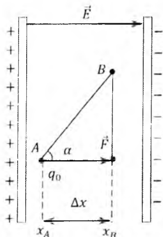
15.1-rasm. Sinovchi q_0 zaryadning elektrostatik maydondagi harakat trayektoriyasi
