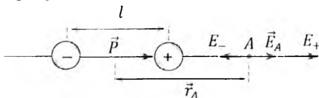
16.8-rasm. Elektr dipoli yelkasi bo'ylab yo'nalgan o'qdagi elektr maydon kuchlanganligi
