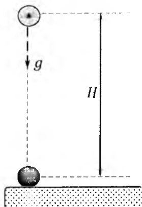
4.3-rasm. Yerdan H balandlikdagi jism holati
