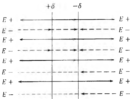
16.6-rasm. Ikki xil ishorali zaryadlangan tekisliklar orasidagi va tashqarisidagi maydon
