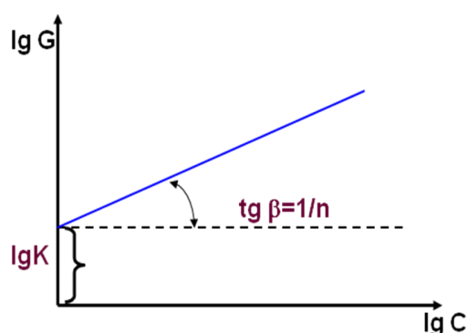
16-rasm. Freydlix tenglamasi konstantalarini grafik usulda topish
