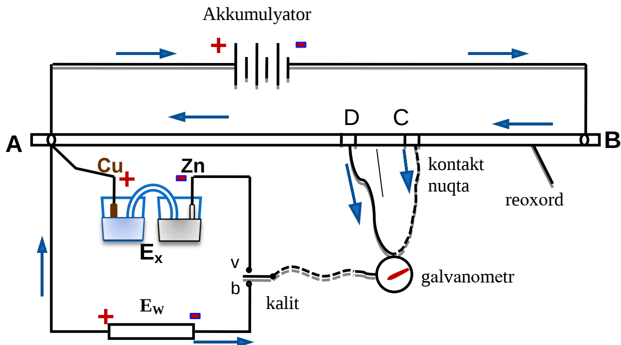
11-rasm. EYuK o'lchashni kompensatsion sxemasi
