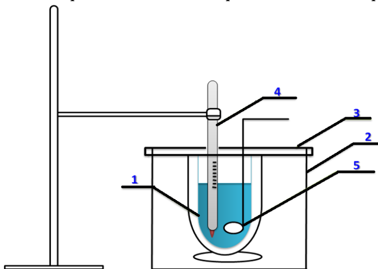
1-rasm. Laboratoriyada qo'llaniladigan oddiy kalorimetr qurilmasi
