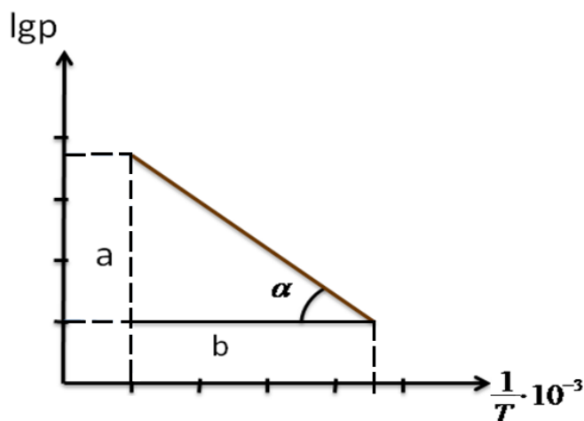
5-rasm. Haroratni bosim bilan bog'liqlik grafigi
