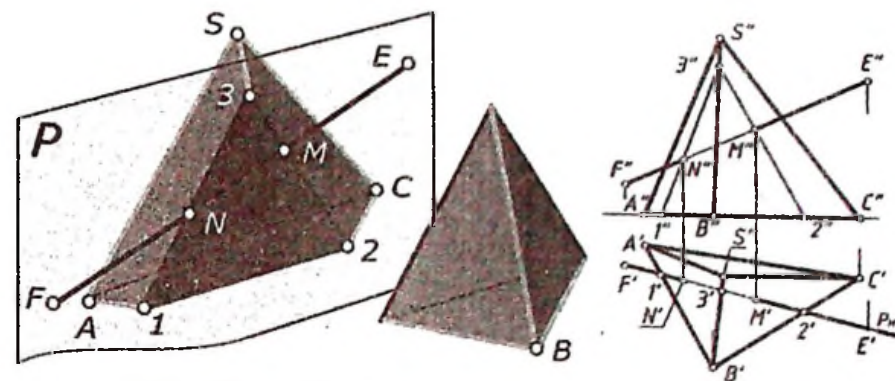
6.16 - chizma. Epyur.
