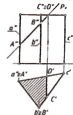
6.7 - chizma. Epyur.
