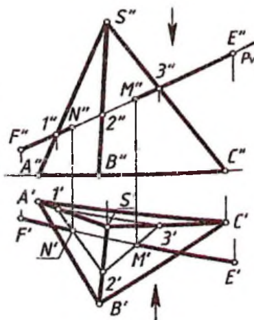
6.14 - chizma. Epyur.
