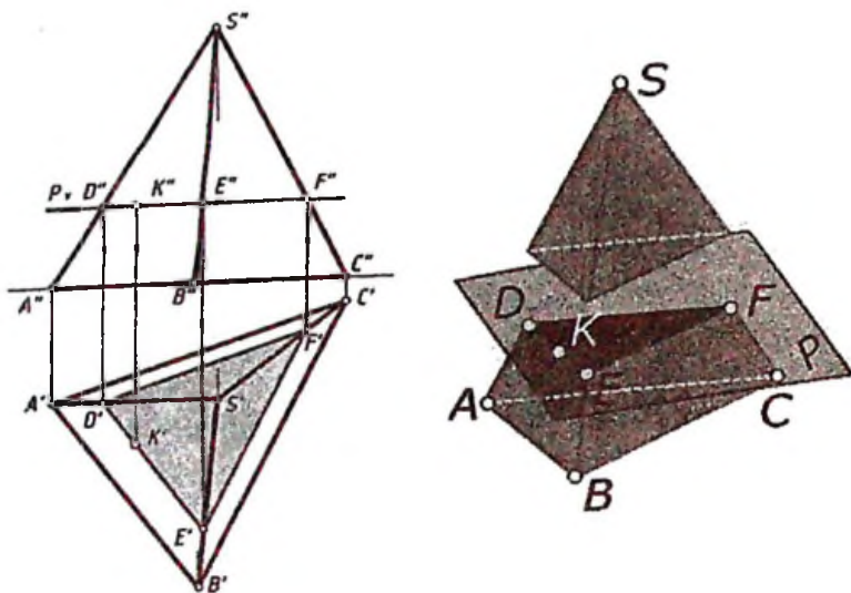
6.4 - chizma. Piramida sirtiga tegishli nuqtani aniqlash.
