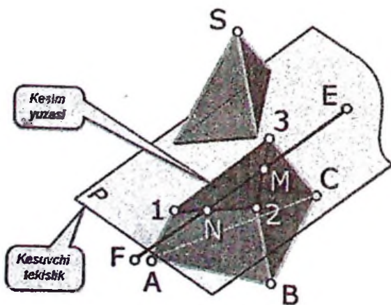
6.13 - chizma. Yaqqol tasvir.
