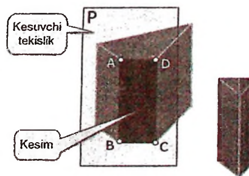
6.10 - chizma. Yaqqol tasvir.
