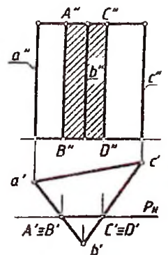
6.9 - chizma. Epyur.
