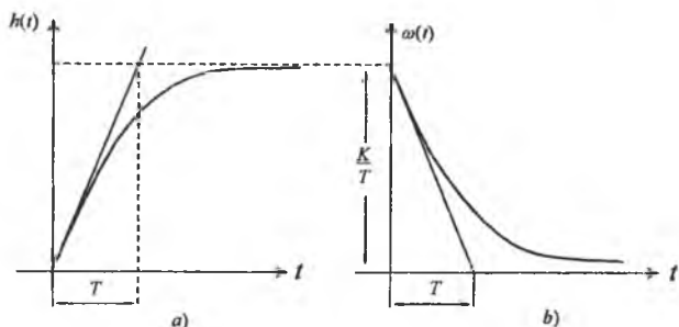
2.21-rasm. O'tkinchi xarakteristika (a); impulsli o'tkinchi xarakteristika (b).
