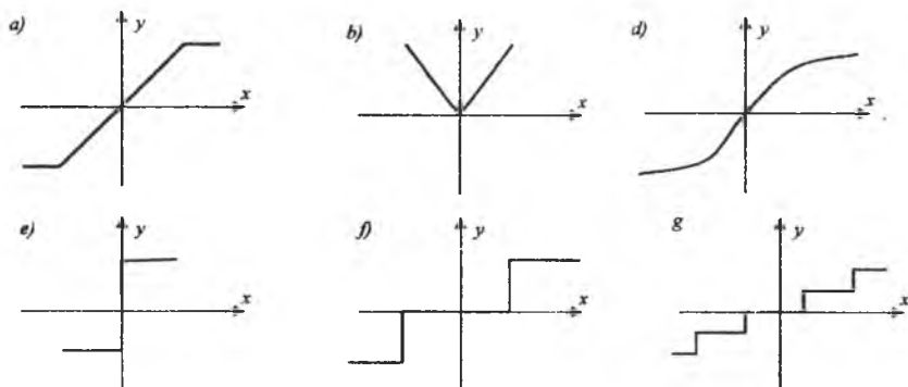
6.1-rasm. Nochiziqli elementlarning xarakteristikalar.
