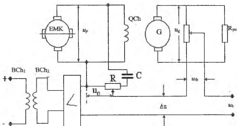
1.8-rasm. O‘zgarmas tok generatorining kuchlanishini avtomatik boshqarish tizimining prinsipial sxemasi.
