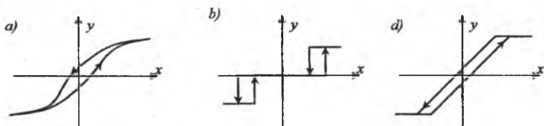
6.2-rasm. Ko'p qiymatli nochiziqli elementlarning xarakteristikalar.
