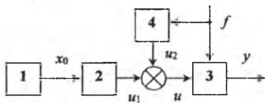
1.14-rasm. Kompensatsiyalash (g'alayon bo'yicha boshqarish) prinsipi.
