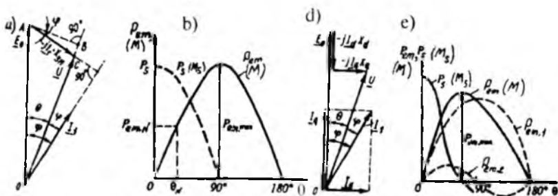
23.2-rasm. Noayon qutbli (a, b) va ayon qutbli (d, e) SGning elektromagnit quvvatini aniqlashga oid soddalashtirilgan vektor diagrammalar (a, d) va tegishli aktiv quvvatining burchak xarakteristikalar (b, e).
