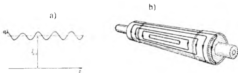
21.2-rasm. Sinxron generatorning nosimmetrik yuklamasida qo'zg'atish chulg'ami tokining o'zgarish shakli ( a ) va turbogenerator rotorida teskari ketma-ketlik maydoni hosil qilgan toklar o'tadigan yo'llar sxemasi ( b ).
