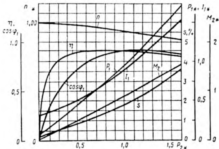
13.4-rasm. Quvvati 50 kW, 220/380 V, 1470 ayl./min boʻlgan qisqa tutashgan rotorli asinxron motorning ish xarakteristikalar.
