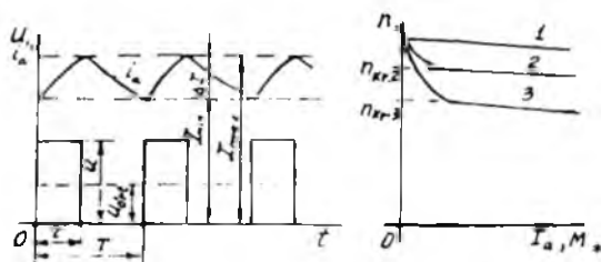
31.14-rasm. O'TM ing aylanish chastotasini impulsli rostlashda kuchlanish va toklarning (zgarish grafigi (a) va parallel qo'zg'atishli rotorni impulsli rostlashda tezlik va mexanik xarakteristikaları (b).
