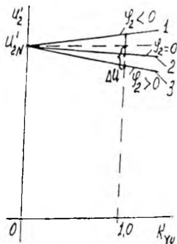
5.3-rasm. Transformatorning tashqi xarakteristikalari: 1 – aktiv-sig‘imiy; 2 – aktiv; 3 – aktiv-induktiv yuklamalar uchun.
