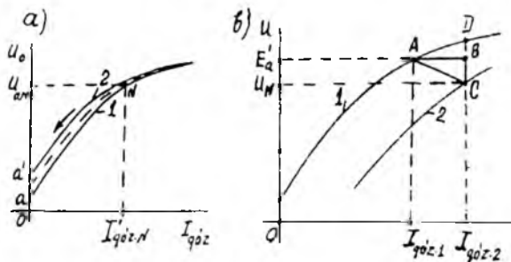
30.1-rasm. Mustaqil qo'zg'atishli o'zgarmas tok generatorining salt ishlash (a) va yuklanish (b) xarakteristikalar.
