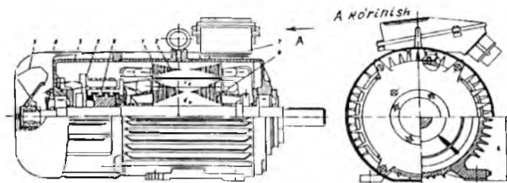
32.4-rasm. 4P seriyali o'zgaras tok motorining bo'ylama va ko'ndalang qirg'irlari:
