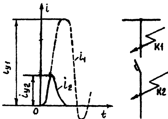
2.14-rasm. Qisqa tutashish tokini tok cheklovchi apparat yordamida kamaytirish: i_1 — apparat kirish qismidagi tok; i_2 — apparat chiqish qismidagi QT toki; I_{v1} va I_{v2} — apparatning kirish va chiqish qismlaridagi zarbaviy toklar.
