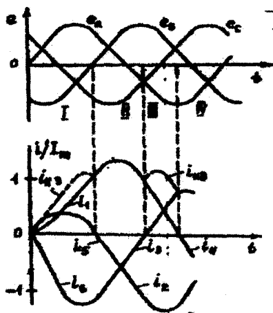
9.26-rasm. Tashqi qisqa tutashgan to'g'rilagichning EYUK ventil toklari diagrammalari; i_1 - i_B — ventil toklari; i_{kz} — qisqa tutashish zanjirini toki.
