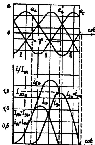
9.31-rasm. Uch fazali yarimo'tkazgichli ko'priq sxemali to'g'rilagichni ichki shikastlanganidagi EYUK va toklari diagrammalari.
