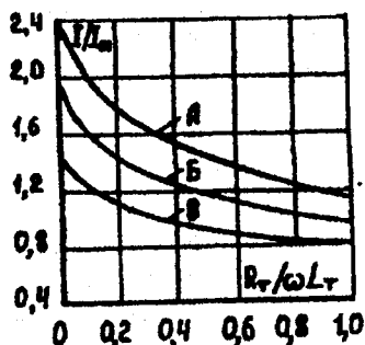
9.32-rasm. Boshqarilmaydigan to'g'rilagich avariya toki amplitudasining R_t/\omega t ga bog'liqlik diagrammalari; A — shikastlangan ventill zanjirida; B va V — shikastlanmagan ventillar zanjirlarida.
