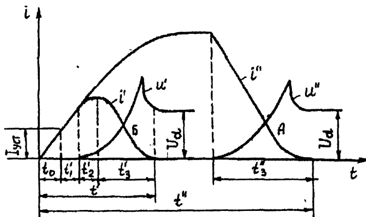
6.1-rasm. O'zgaras tok uzgichining qisqa tutashish davridagi uzishida tok va kuchlanishlar o'zgarish grafiklari.
