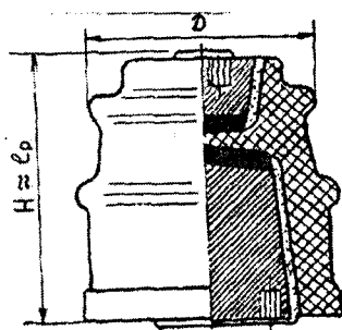
8.9-rasm. Armaturasidan ishlangan tayanch izolatori.
