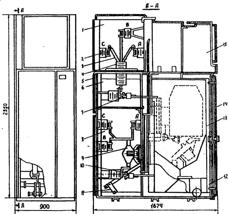
10.1-rasm. Elektr magnitli uzgich BEM-10Eli shkaf KRU-2 a 10E/E:
