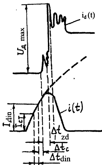
6.11-rasm. VAT—42 ( I_{nom} = 6300 A) turidagi uzgichning tok va kuchlanish ossilogrammalari.
