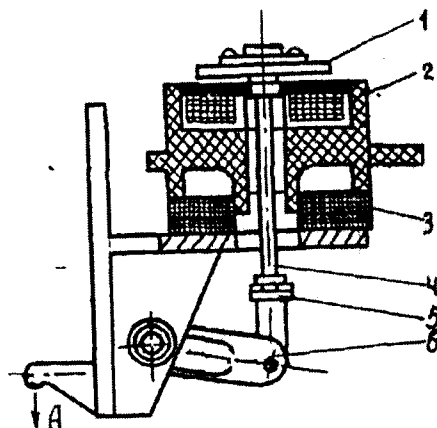
6.10-rasm. VAT—42 turdagi uzgichning induksiyali — dinamik yuritmasi: 1—disk; 2—g'altak; 3—qatlam; 4—tortgich; 5—gaykalar; 6—richag.
