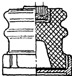
8.10-rasm. Armaturasini kombinatsiyali ishlangan tayanch izolatori.
