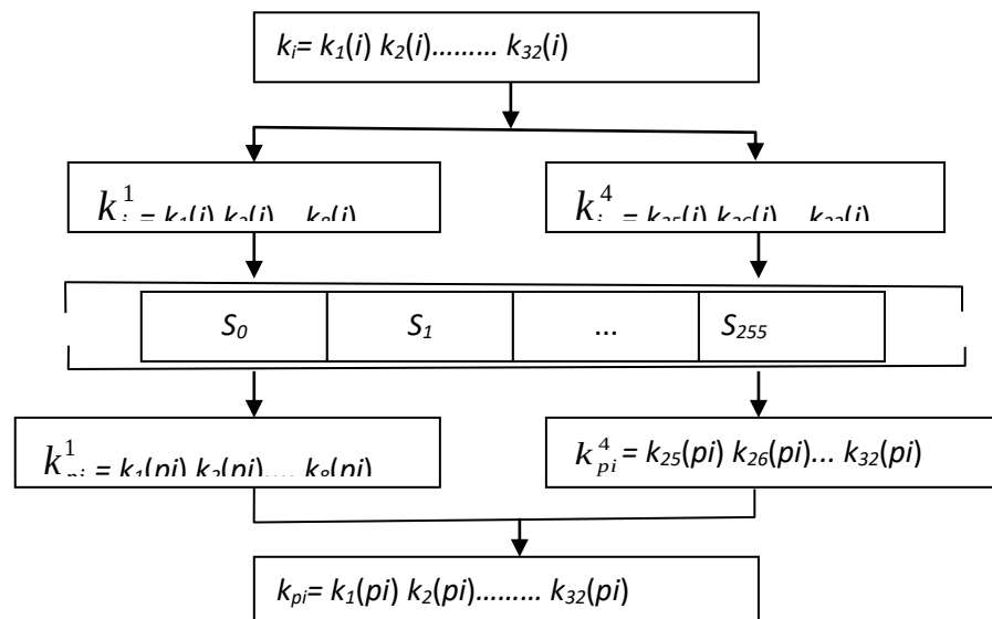
i – raund kaliti generatsiyasining blok sxemasi
