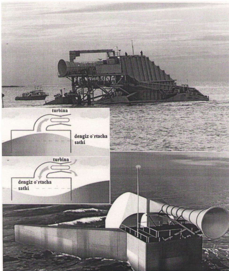
5.2 rasm To'liqin energiyasini olish prinsipi.
