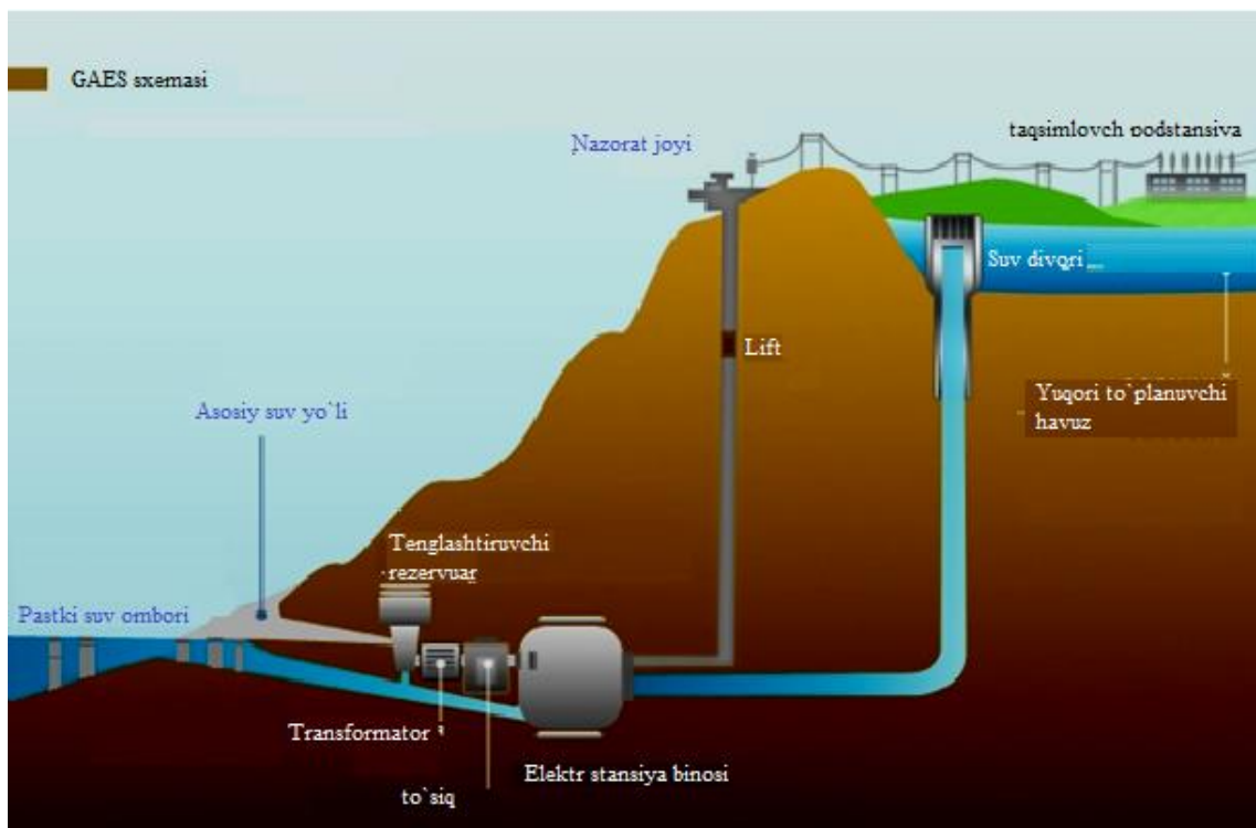
1.9 rasm GAESning prinsipial sxemasi
