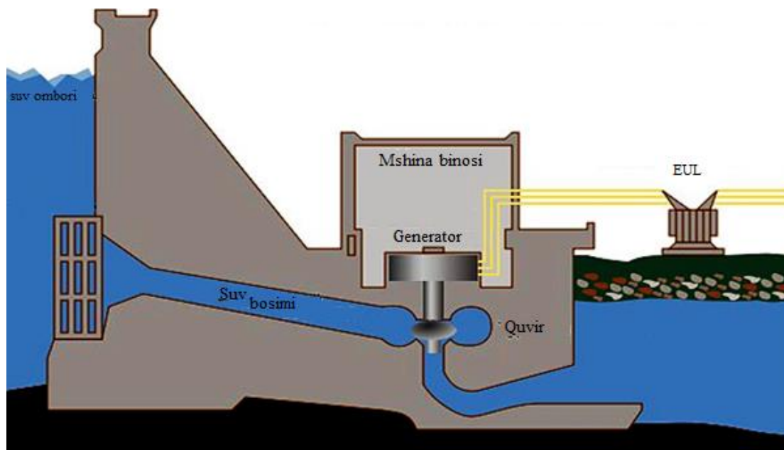
1.8 rasm GESni ishlash prinspi.
