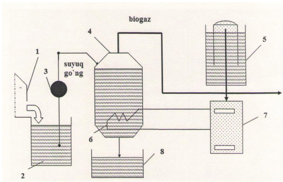
8.3-rasm Biogazni olish texnologik sxemasi
