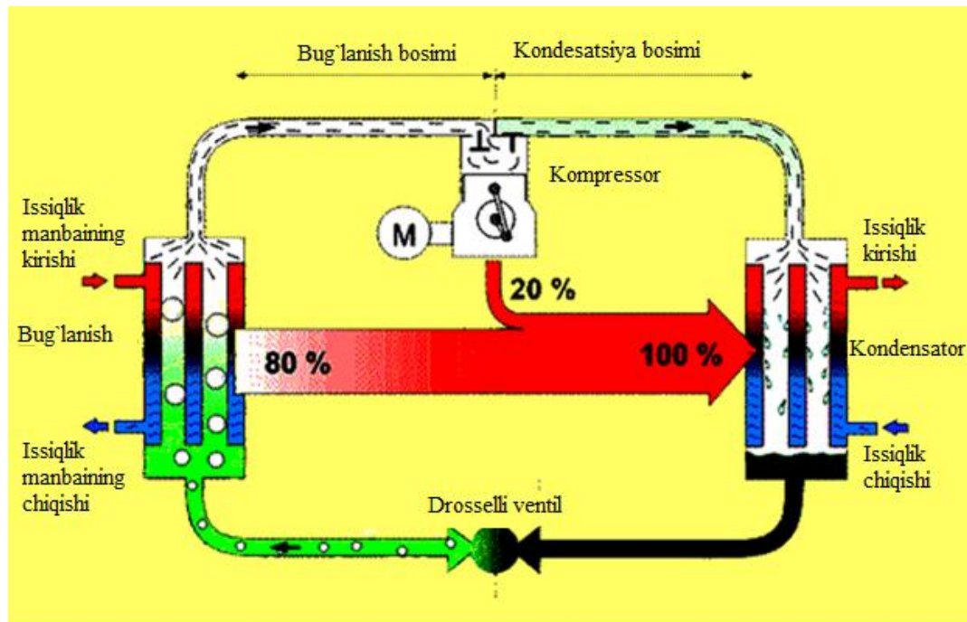
6.6-rasm Issiqlik nasosining ishlash prinspi.
