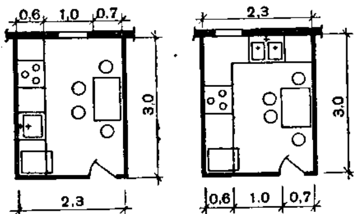
92 расм. Ошхона-ошхонанинг тархӣй ечимига доир мисол.
