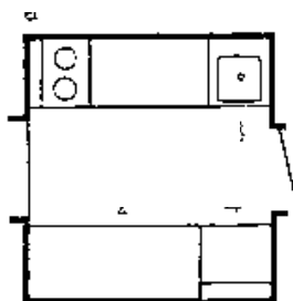
Ошхона жиҳозини икки қатор қилиб жойлаштиришга доир мисол
