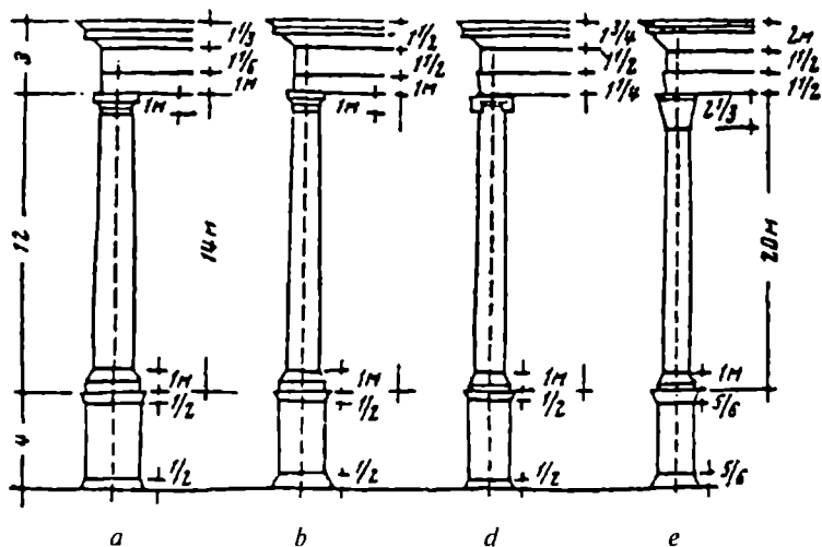
54-rasm. Rim orderlarining modullardagi o'lchamlari: a) toskan orderi; b) dor orderi; d) ion orderi; e) korinf orderi.
