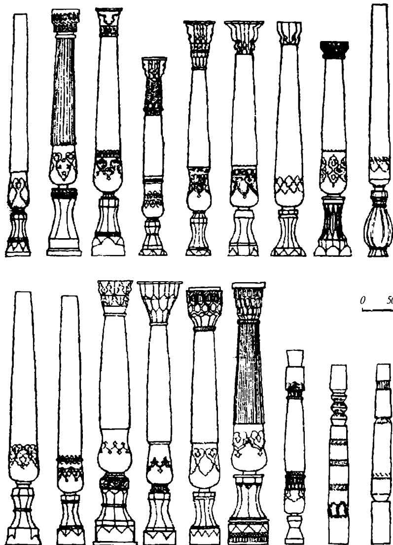
21-rasm. O'rta Osiyo ustunlarining Qashqadaryo viloyatidagi turlari. D. Nozilov bo'yicha.
