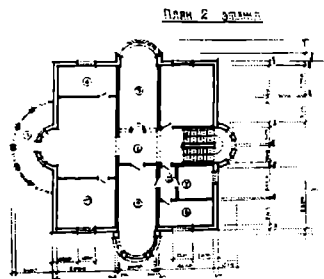
50-rasm. Grafikada tugatilgan loyihaga misol. (TAQI da bajarilgan kurs ishi.)
