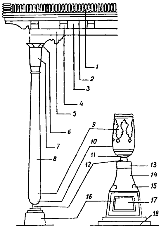
19-rasm. O'rta Osiyo orderlarining tarkibiy qismlari:
