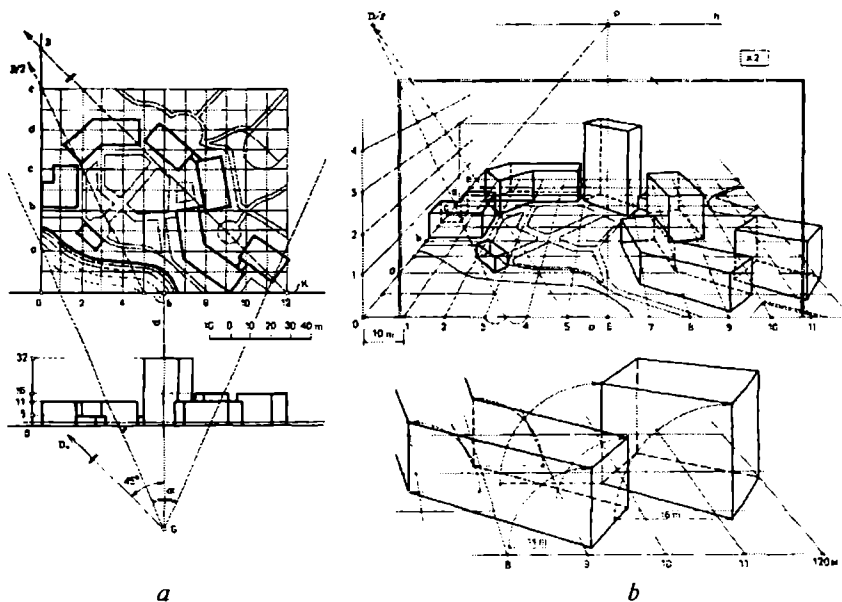
45-rasm. Perspektiva qurishning to'rt usuli:
