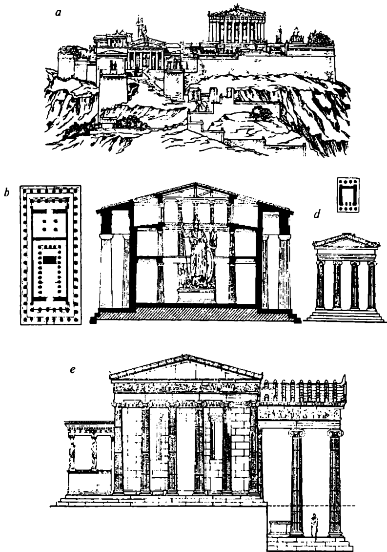
10-rasm. Qadimgi Yunonistonda qo'llanilgan orderlar (mil. avv. X asr) a) Afina akropoli majmuasi; b) Parfenon ehromi (tarhi va qirqimi); d) Niki ehromi (tarhi va tarzi); e) Erehteyon ehromi (tarzi).
