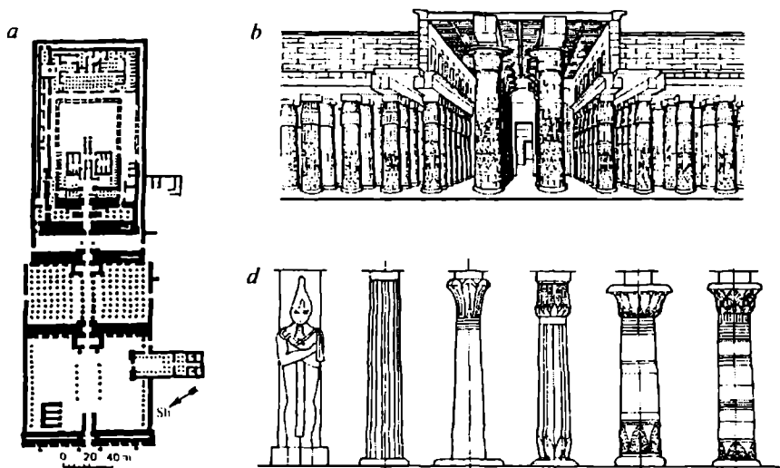
9-rasm. Qadimgi Misrda qo'llanilgan orderlar:
