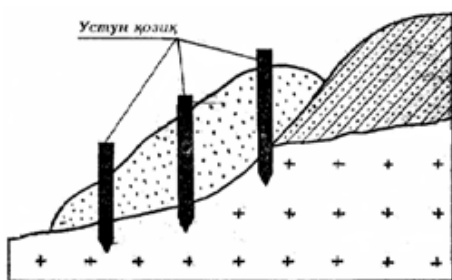
6.3-rasm. Suriladigan qiyalikni ustun qoziklar yordamida mustahkamlash (O.Mavlonov, S.Zohidov rasmi)
