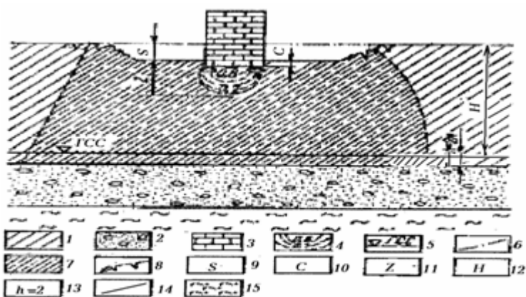
6.11-rasm. Cho'kish hodisasi tufayli lyossimon jinslarda liformatsiyalangan chegaralar sxemasi (Mavlonov va K.Pilatov): 1-mikro g'ovakli cho'kuvchan lyossimon jinslar (suv bilan namlangan); 2-toshli shag'allar; 3-jinsda chiqindidan keyin ko'rilgan inshoot; 4-tashqi kuch ta'sirida gruntlarda kuchlanishning tarqalish sxemasi (0,2 va 0,8 kuchlanishlar miqdori, 6,kgk/sm 2 ); 5-lyossimon jinslar namlanishga qadar grunt suvuning sathi; 7-bir oz cho'kkan va suv bilan namlangan jins; 8-cho'kish natijasida cho'kuvchan uchastkada hosil bo'lgan yoriqlar; 9-cho'kishning miqdori, sm; 10-qo'shimcha cho'kish miqdori, sm; 11-Inshoot og'irligi ta'sirida deformatsiyalangan zonaning qalinligi, m; 12-cho'kuvchan jinsning qalinligi, m; 13-grunt namlanishi natijasida kapilyar ko'tarilish miqdori; 14-cho'kishdan keyin yer yuzasining sathi; 15- gil qatlamlari
