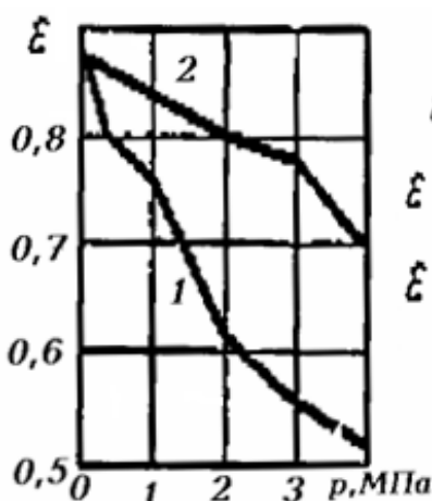
6.13-rasm. Oldindan ivitilgan (1) va tabiiy namlikdagi (2) lyossimon tog' jinsining zichlanish grafiği
