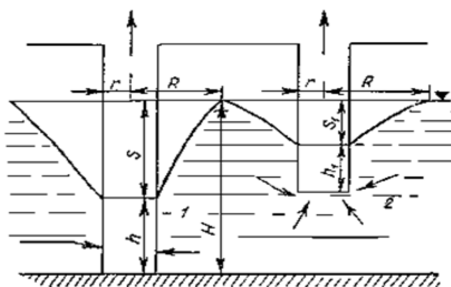
7.16-rasm. Suv yig'uvchi quduqlar 1-tugallanmagan 2-tugallanmagan ko'rinishi
