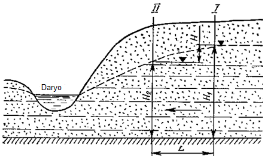
7.11-rasm. Grunt suvlarining sizish chizmasi
