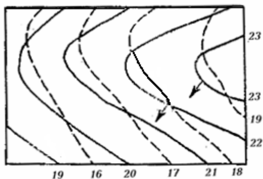
--- gorizontal chizig'i - - - gidroizogips chizig'i suv osti suvlari oqimining yo'nalishi 7.6-rasm. Gidroizgips haritasi: 1-gorizontal chiziq; 2-gidroizgips chizig'i; 3- yer osti suvlari oqimining yo'nalishi.
