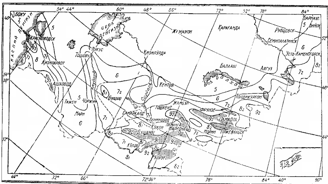
5.7-rasm. O'rta Osiyo va Qozog'iston seysmikrayonlashtirish haritasi.
