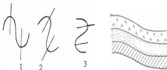
5.2-rasm. Bukilmalarning shakllari; 1-to'g'ri; 2-3-qiyalikda
