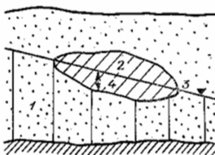
7.5-rasm. Mahalliy bosimning vujudga kelish chizmasi; 1-grunt suvi; 2-gilqatlamchasi; 3-grunt suvining yuzasi mahalliy bosimning balandligi.
