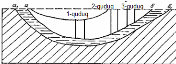
7.7-rasm. Artezian suvining yer yuzasiga chiqishi. Yer (muldasimon) shaklda bosimli suvli gorizontining yotishi, a_1a va b_1b - suvli gorizontining yer yuzasiga chiqishi.
