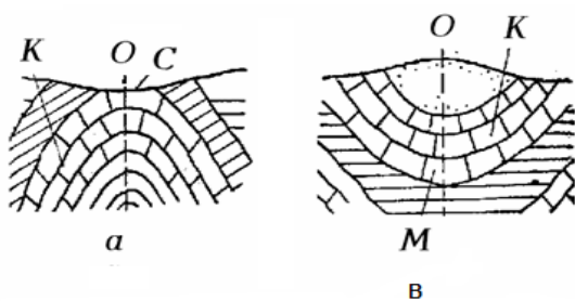
5.1-rasm. Bukilmalar va ularning elementlari: a-antiklinal; B-sinklinal; K-qanoti; O-bukilmalar o'qi; C-eg'ar; M-Mulda
