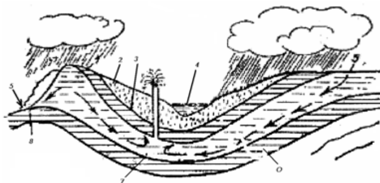
7.10-rasm. Artezian shavzaning qirgimi: 1-suv o'tkazmaydigan qatlam; 2-tuproq suvi; 3-grunt suvi; 4-daryo; 5-buloq; 6-qatlamlar orasidagi pastga tushuvchi yer osti suvi; 7-qatlamlar orasidagi ko'taruvchi yer osti suvi; 8-suv o'tkazmaydigan qatlam.
